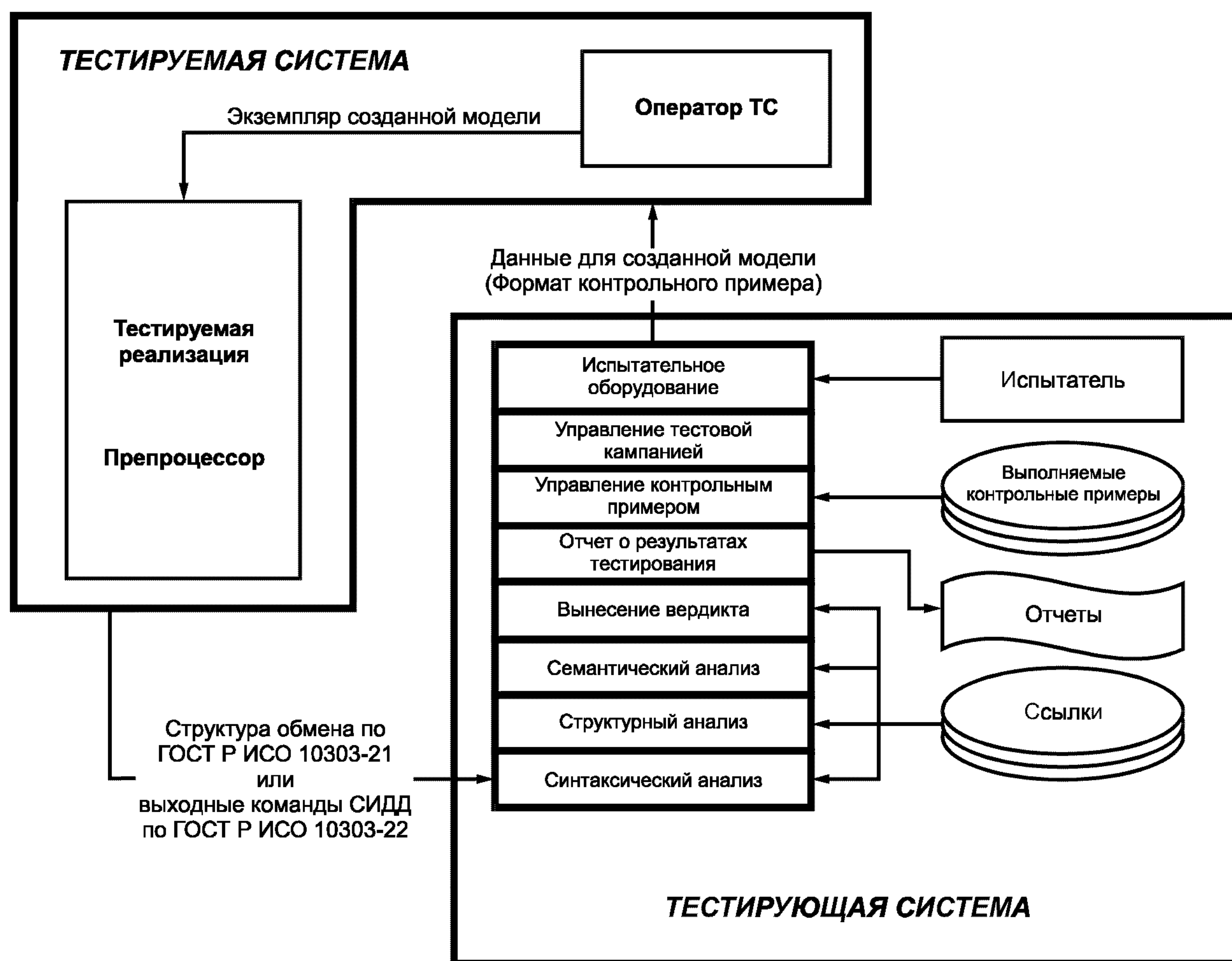
Рисунок 1 — Компоненты тестирования препроцессора
