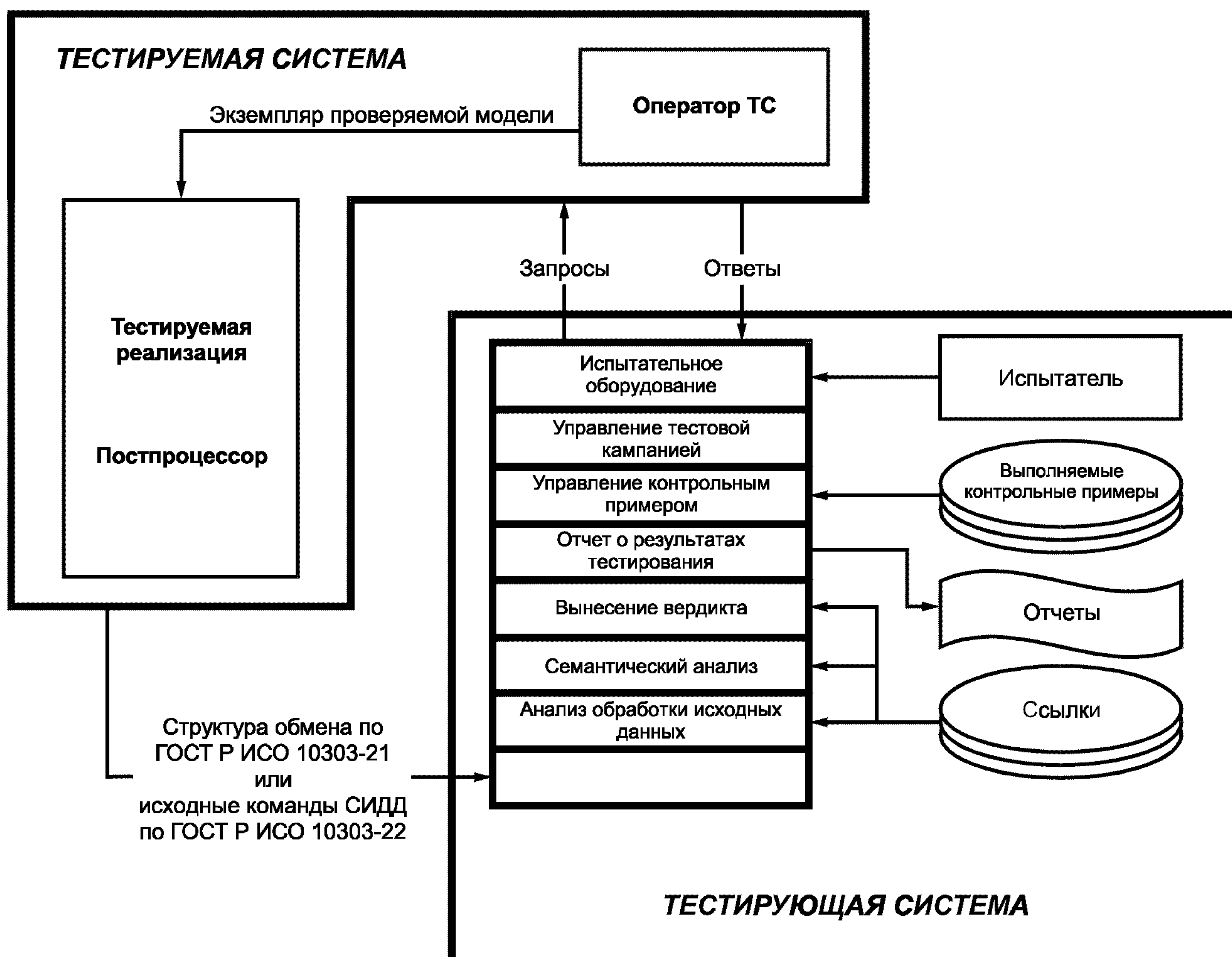
Рисунок 2 — Компоненты тестирования постпроцессора
