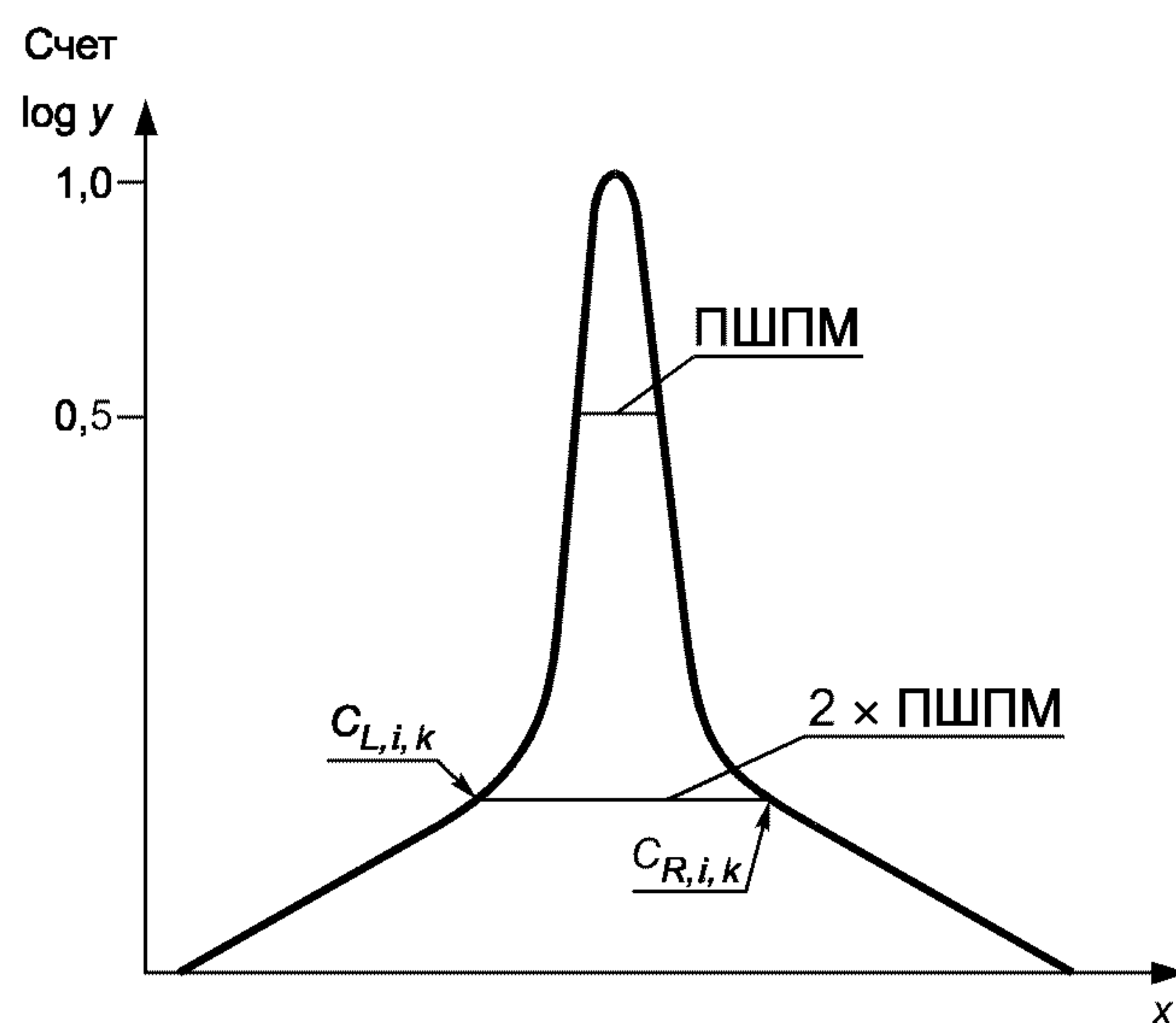
Рисунок 4 — Оценка ФРАКЦИИ РАССЕЯНИЯ
