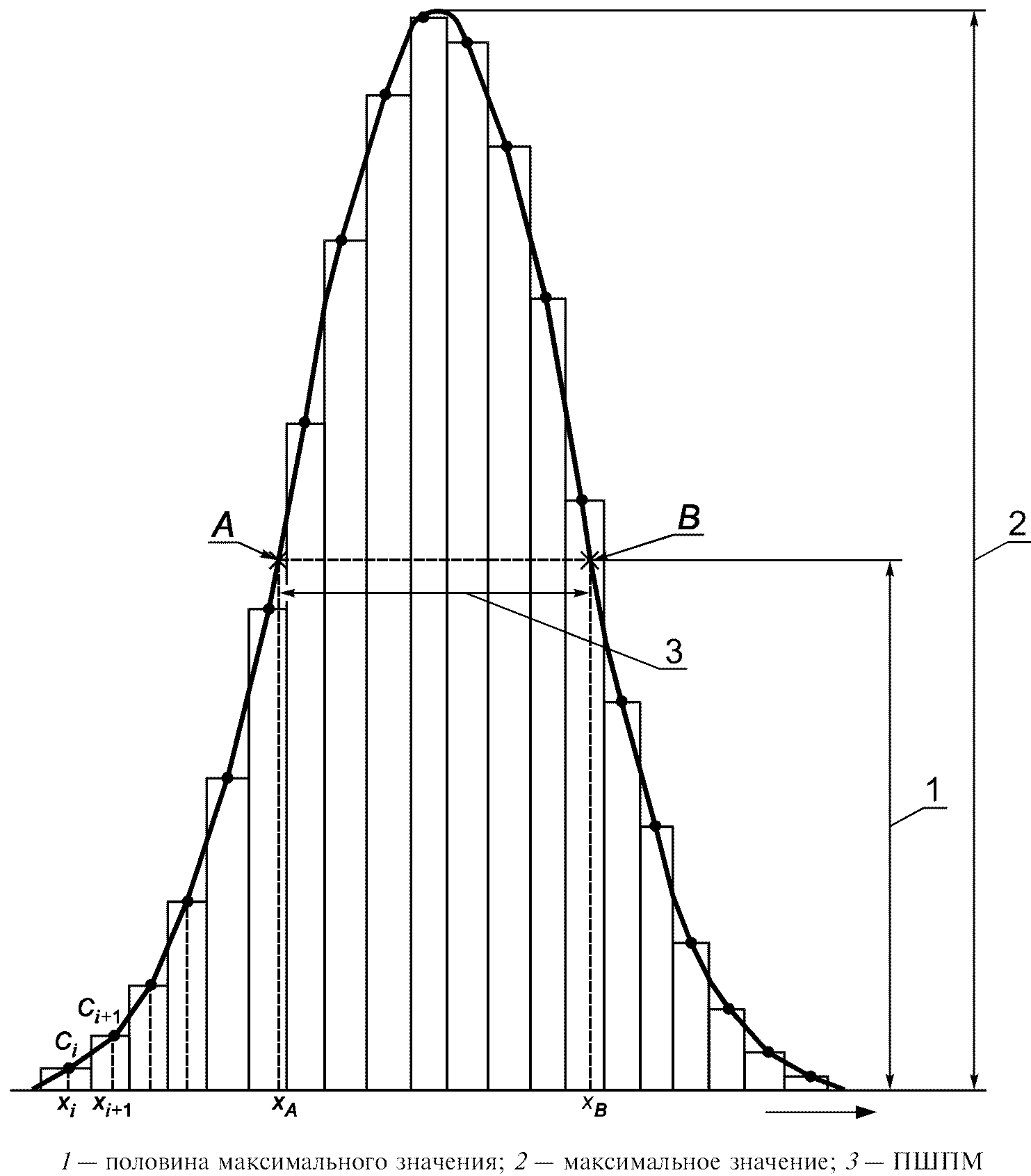
Рисунок 6 — Определение ПШПМ
