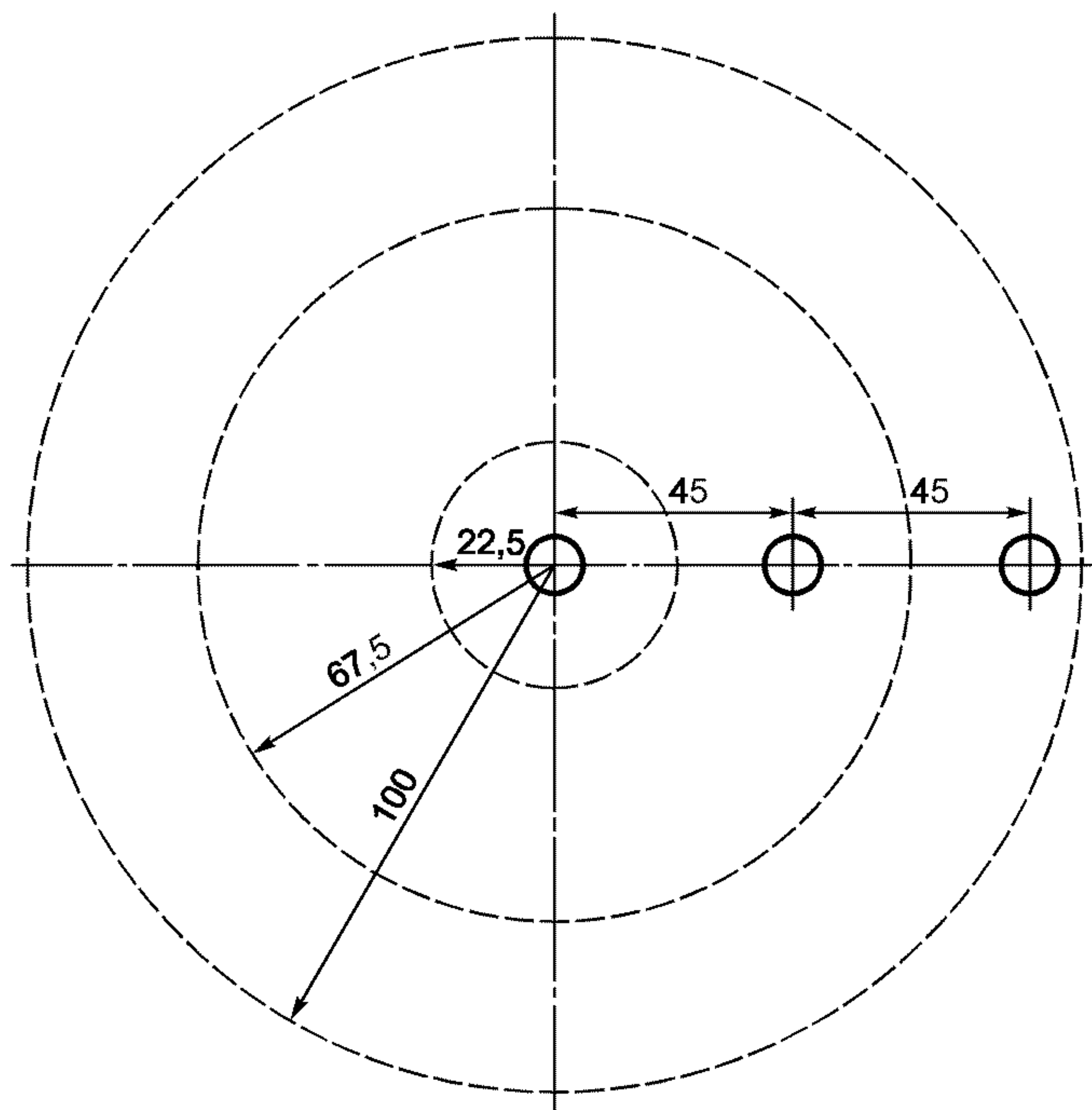
Рисунок 2 — Цилиндрический фантом головы
