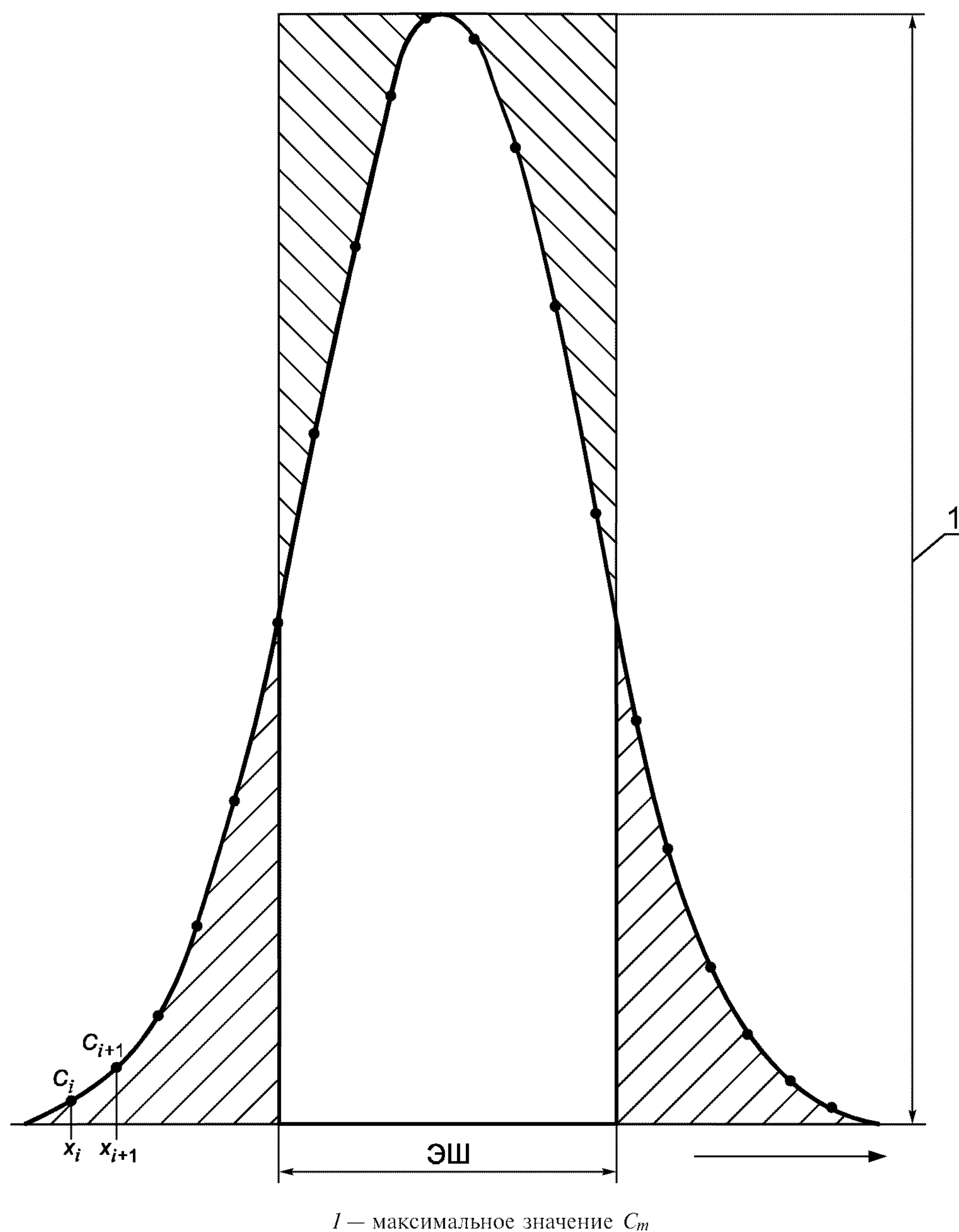
Рисунок 7 — Определение ЭКВИВАЛЕНТА ШИРИНЫ
