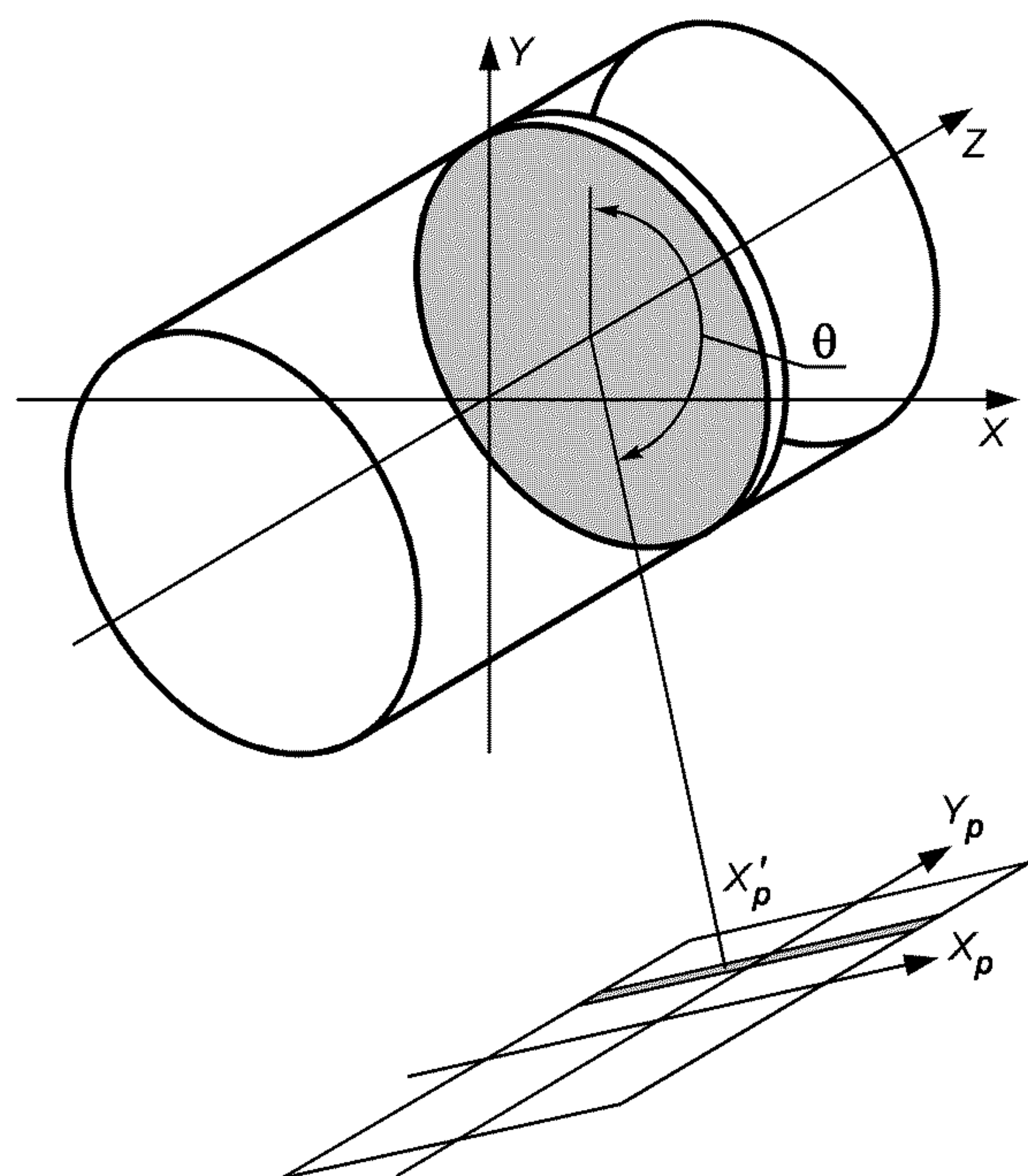
Рисунок 1 — Геометрия ПРОЕКЦИЙ
