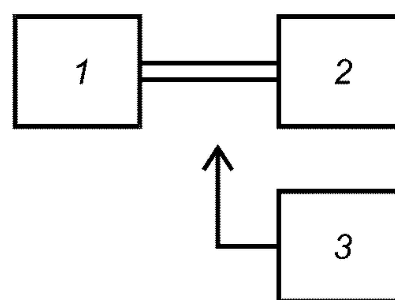
1 — приемник; 2 — эквивалент сети типа 4 по ГОСТ Р 51319; 3 — селективный микровольтметр
