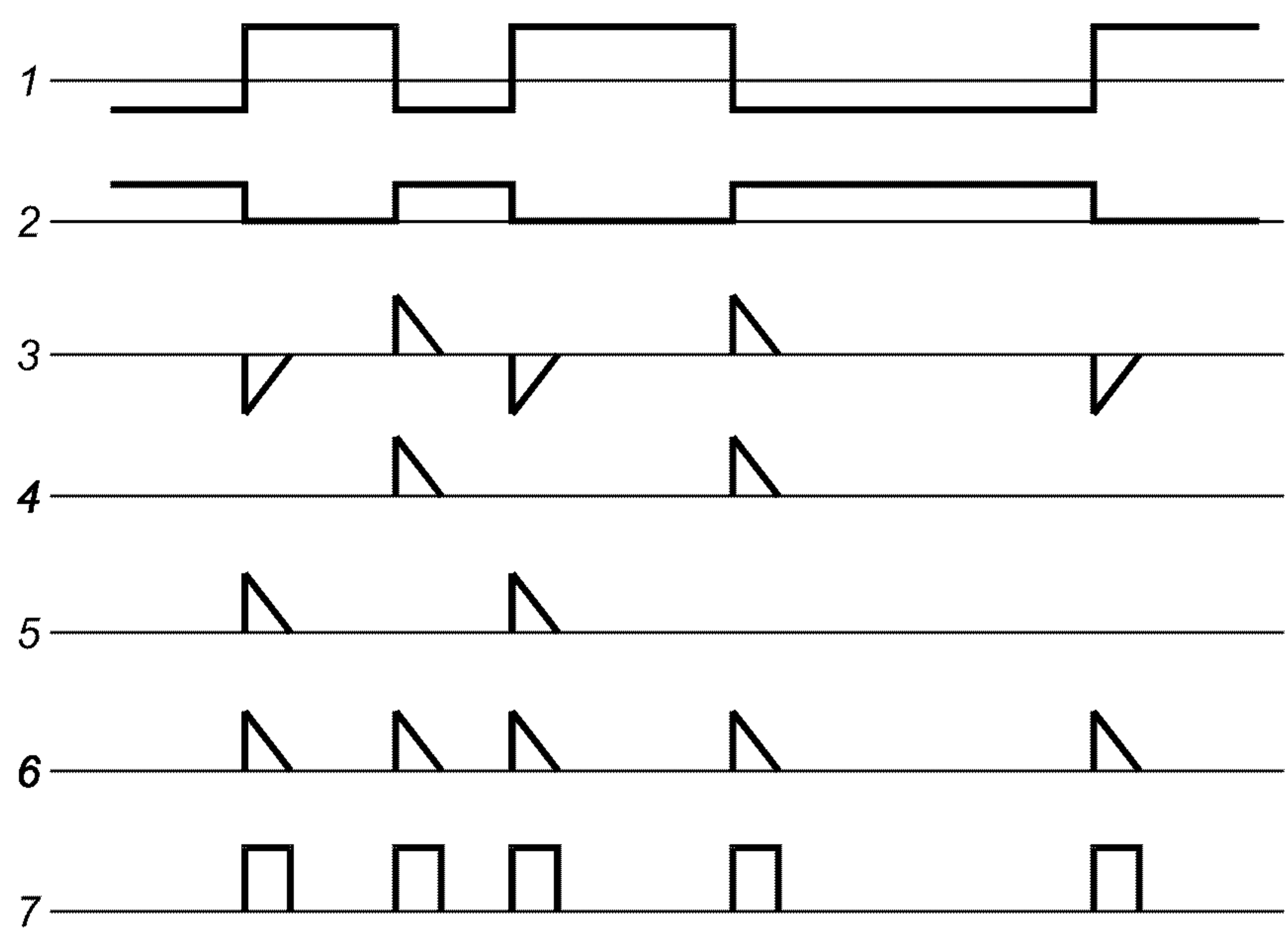
1 — входной сигнал; 2 — сигнал после формирователя однополярного сигнала; 3 — сигнал на выходе дифференцирующей цепи; 4 — неинвертируемые положительные импульсы; 5 — сигнал на выходе инвертора; 6 — сигнал на входе мультивибратора; 7 — выходные импульсы
