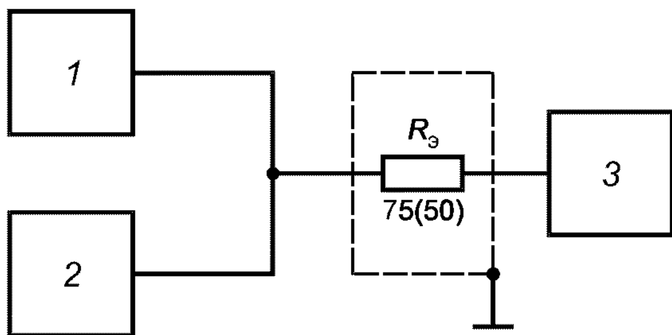
1 — генератор высокочастотных сигналов; 2 — универсальный вольтметр; 3 — приемник; R_э — эквивалент антенны мощностью не менее 200 Вт
