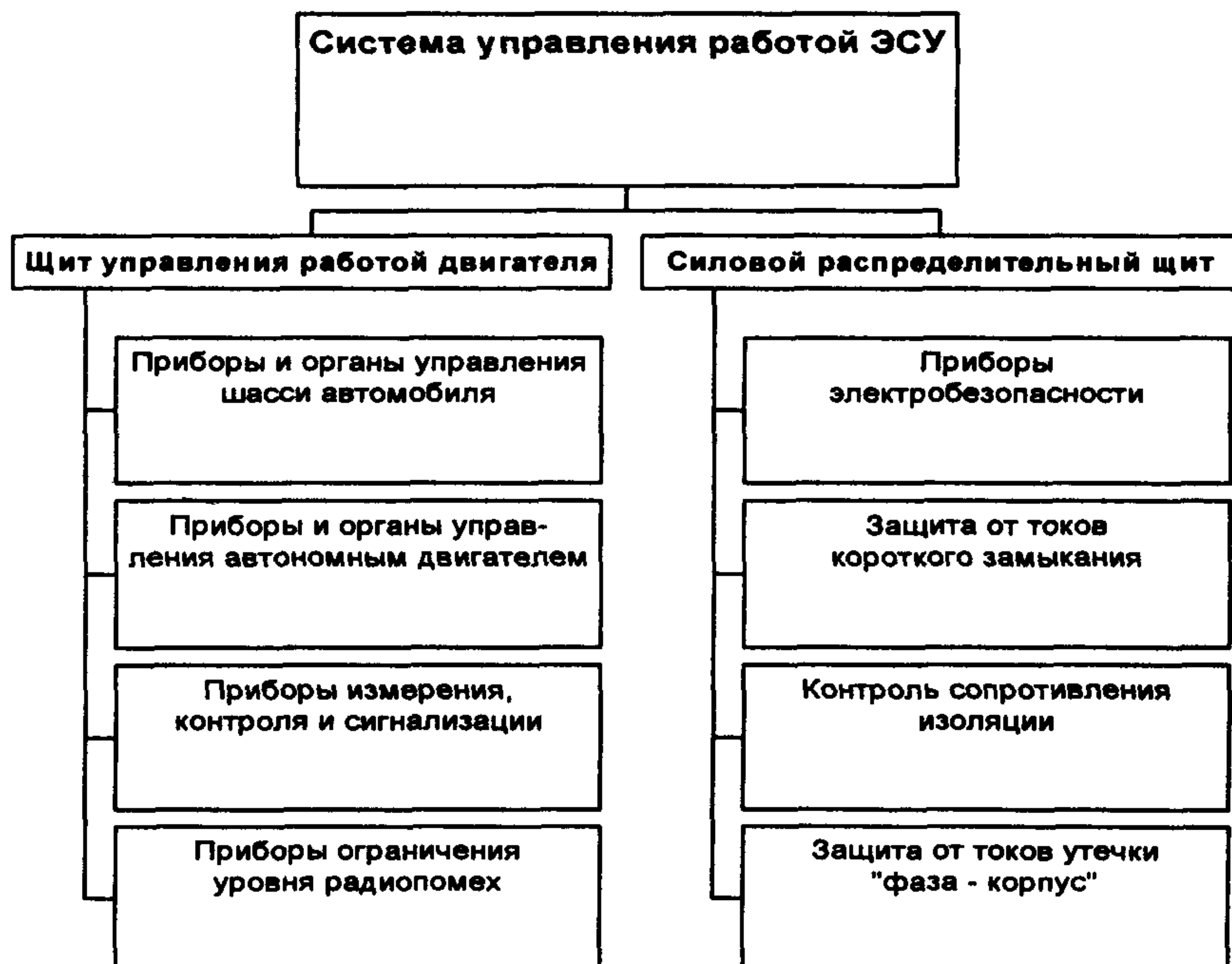
Структура системы управления работой ЭСУ АСА
