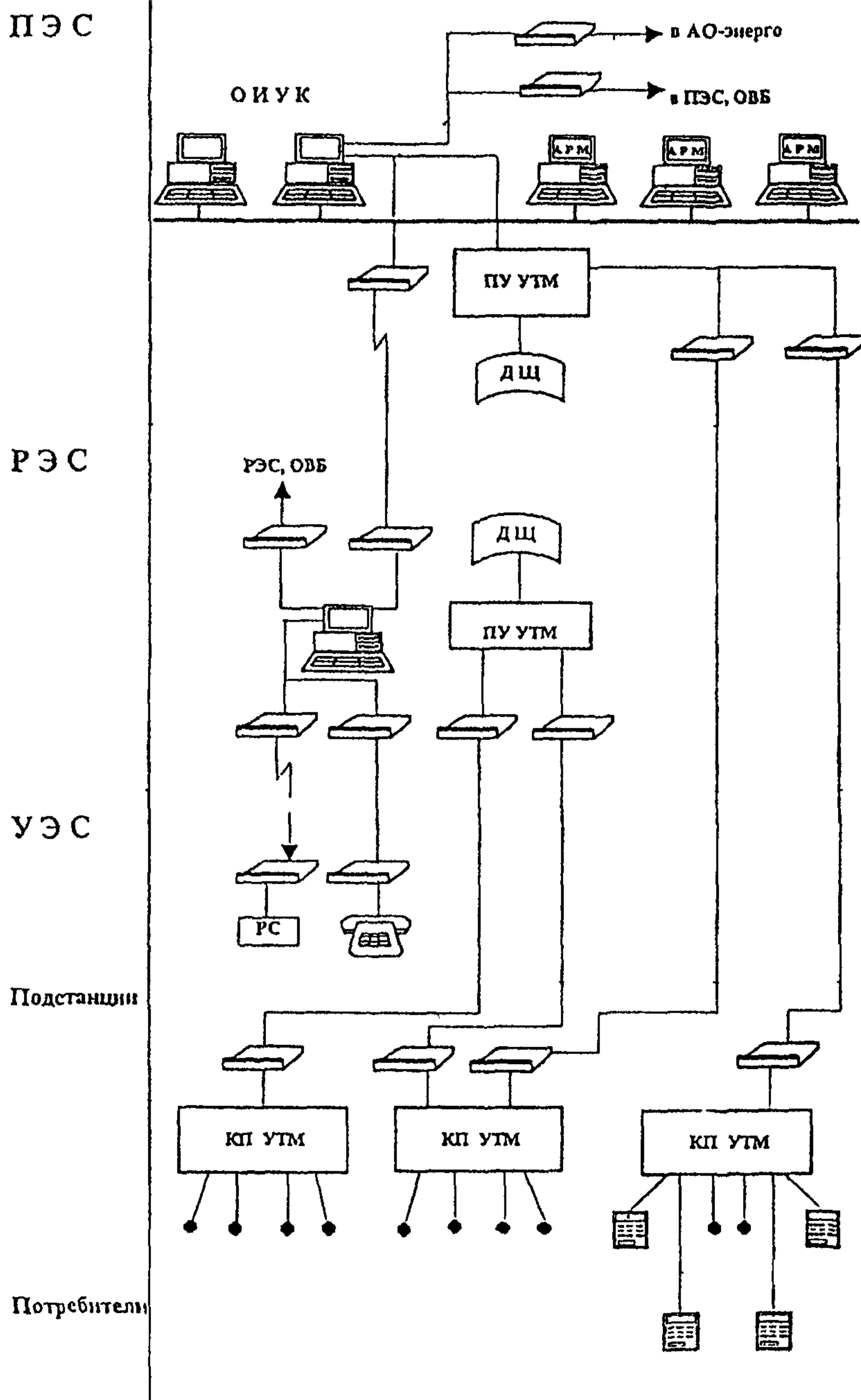
Рис 7 У. Архитектура первого этапа развития технических средств АСУ РЭС
