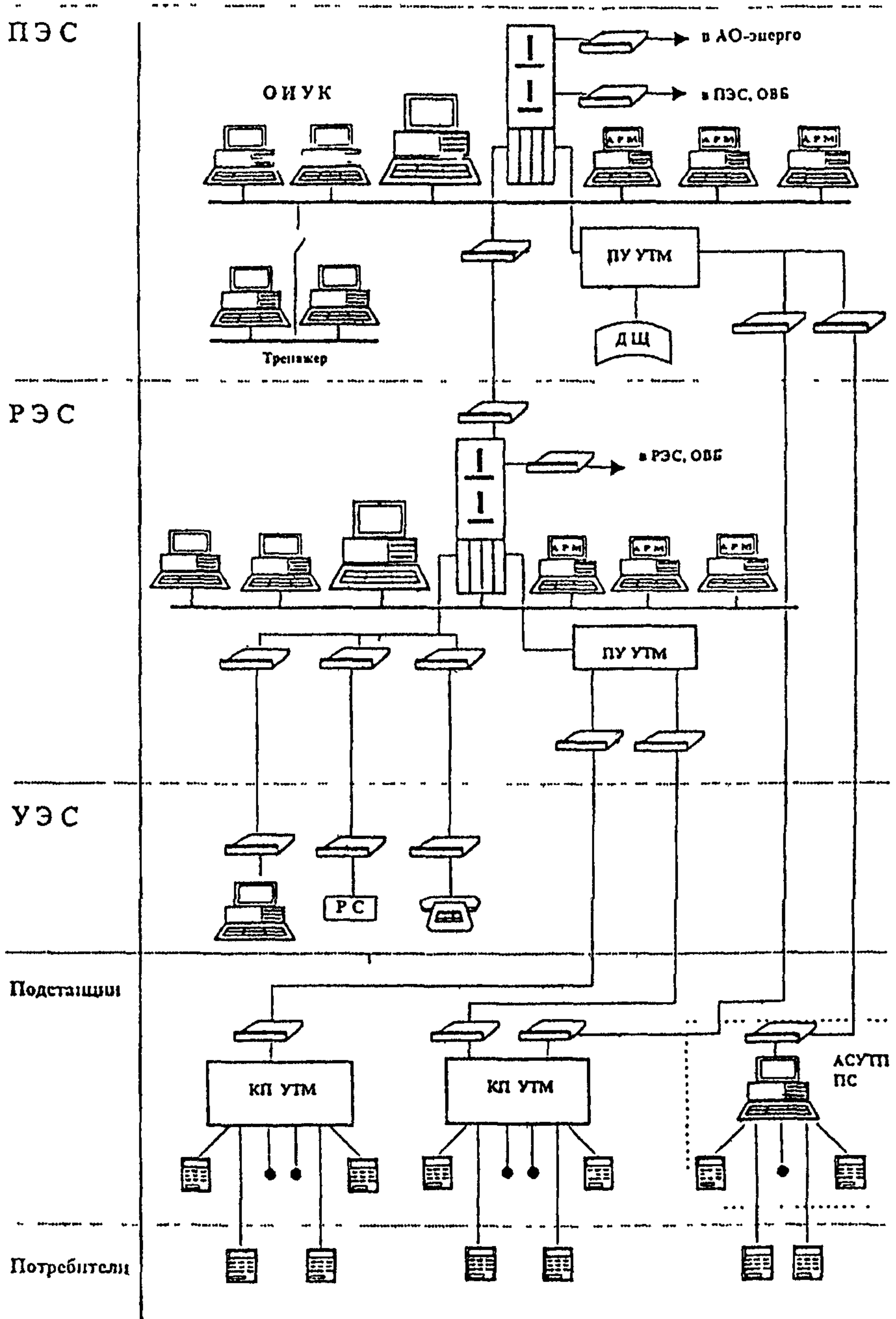
Рис 7.3. Архитектура третьего этапа технических средств АСУ РЭС
