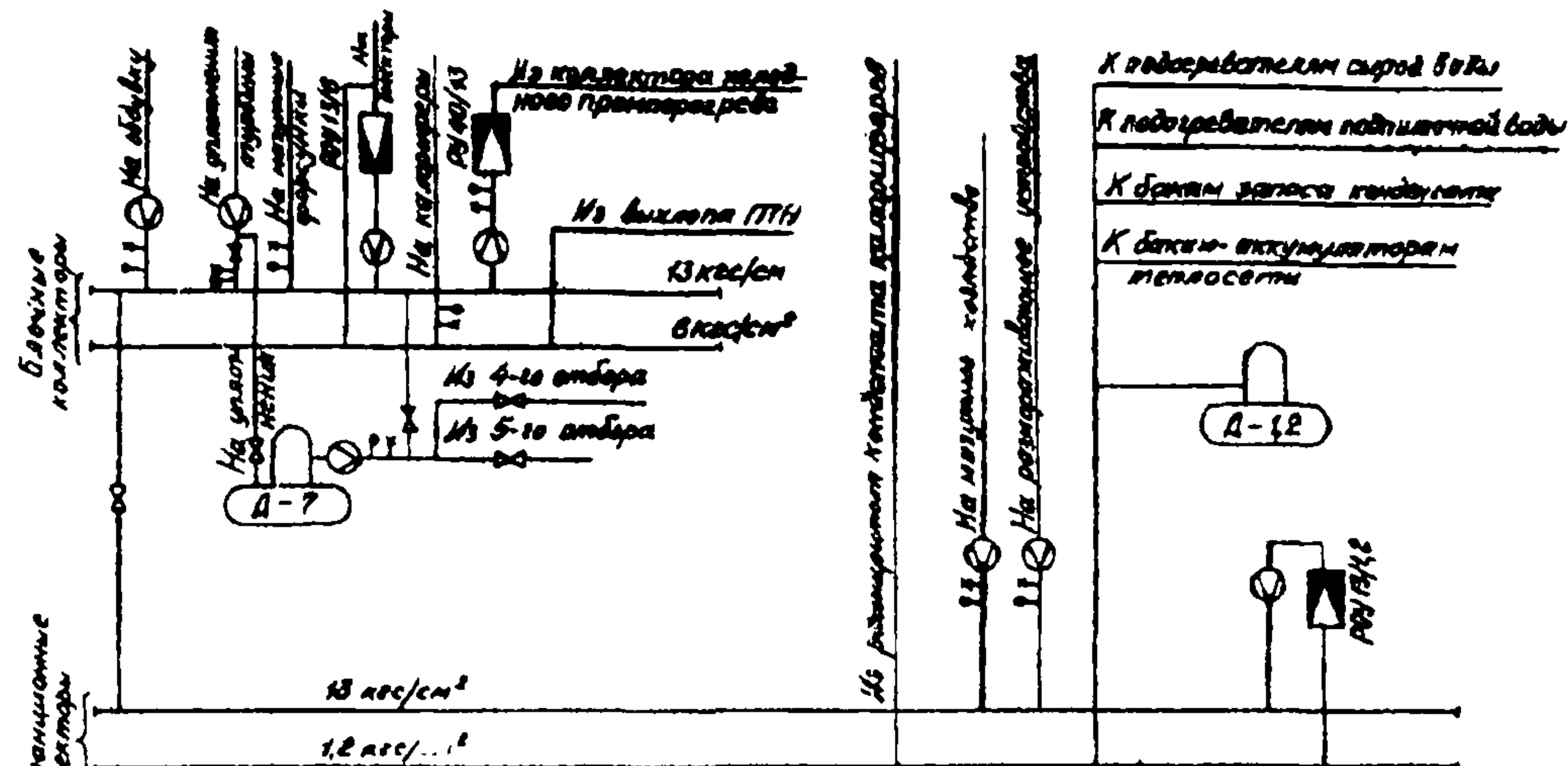
Рис. 6. Принципиальная схема тепловых СН энергоблока Т-250/300-240 для открытых систем теплоснабжения с точками измерений для расчета ТЭП. Обозначения см. рис. I
