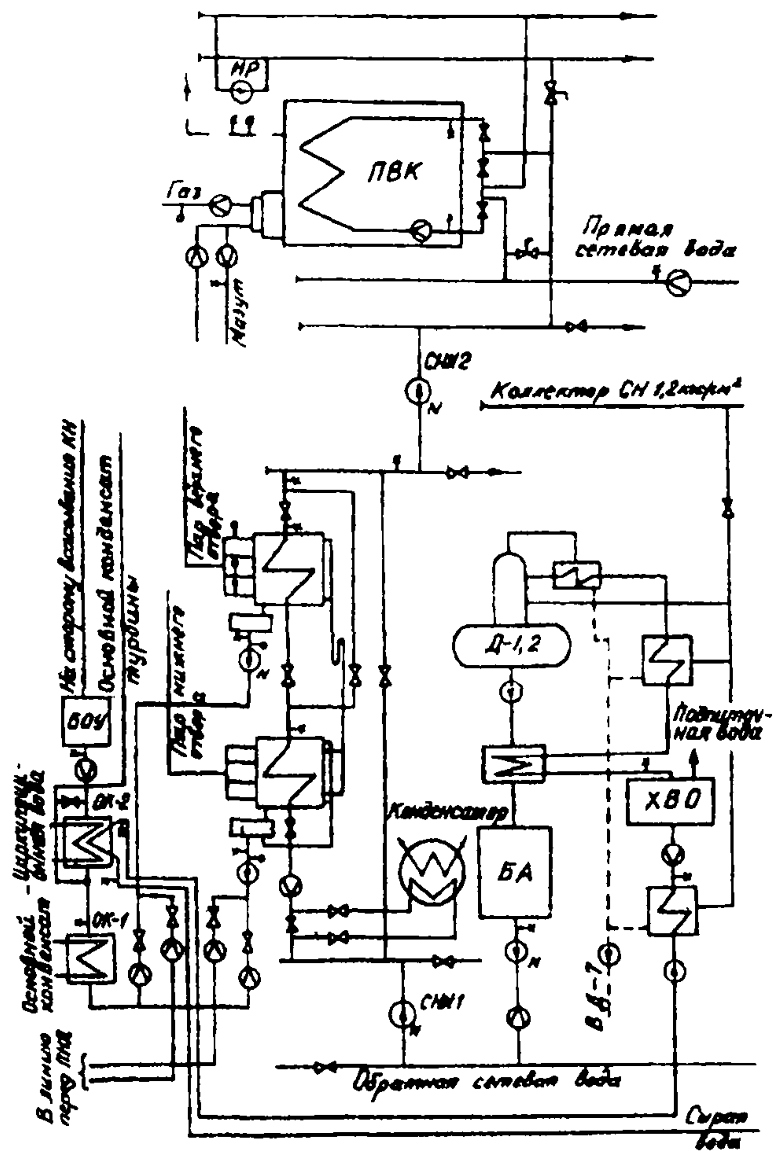
Рис. 5. Принципиальная схема сетевой установки для систем закрытого водоразбора Обозначения см. рис. I
