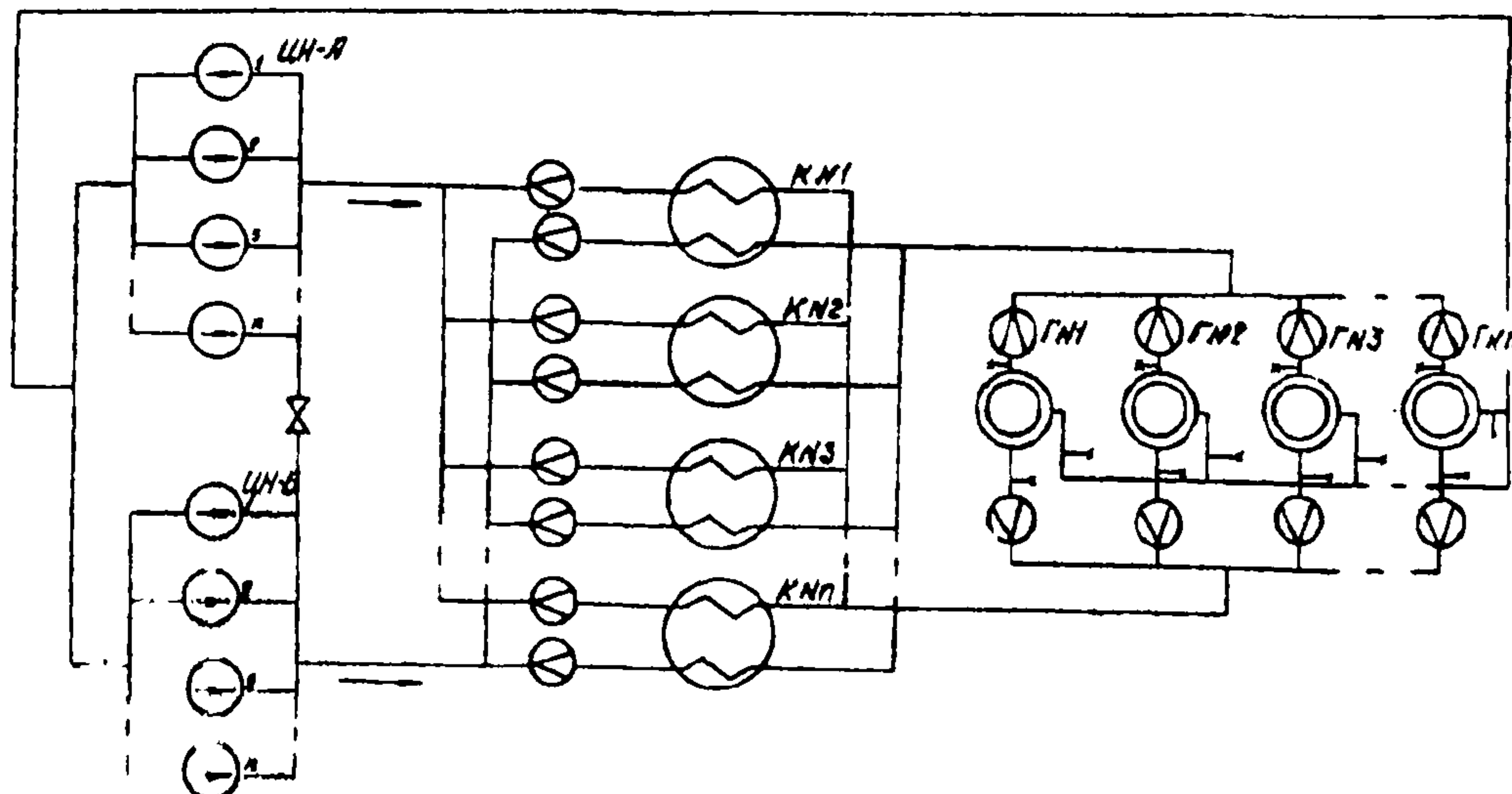
Рис. 7. Типовая схема циркуляционного водоснабжения ТЭЦ с центральной насосной. Обозначения см. рис. I
