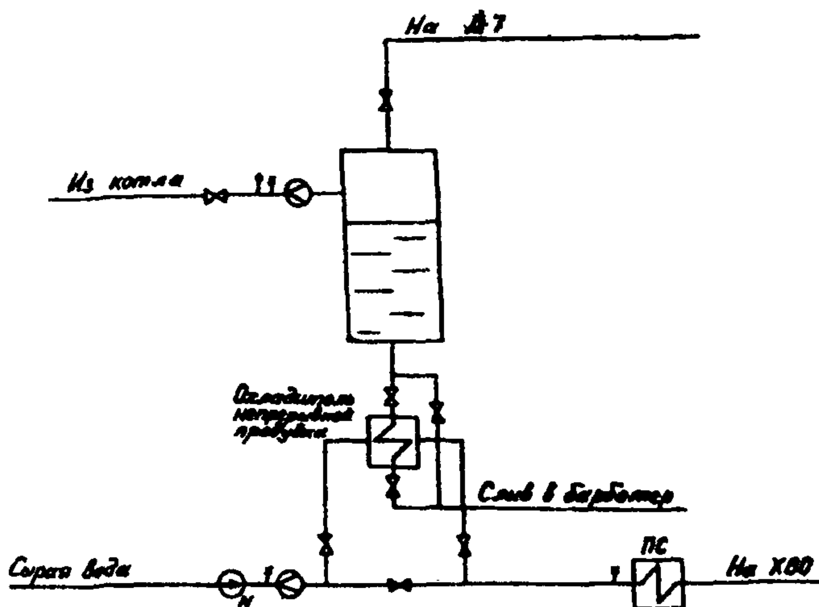
Рис. 4. Схема использования тепла непрерывной продувки барабанных котлов Обозначения см. рис. 1
