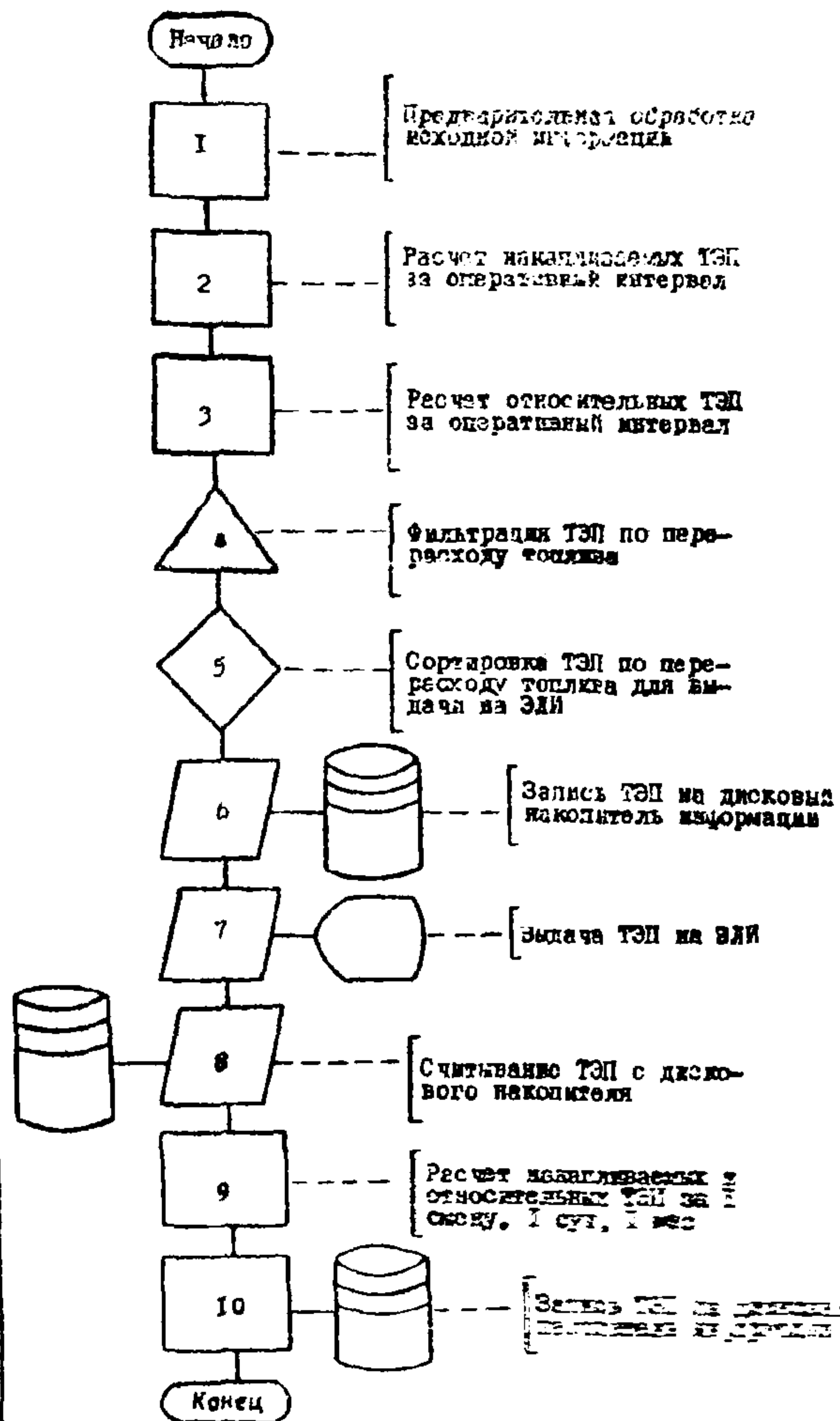
Рис. II. Блок-схема машинной программы расчета ТЭП для анализа оперативно-регулируемых параметров
