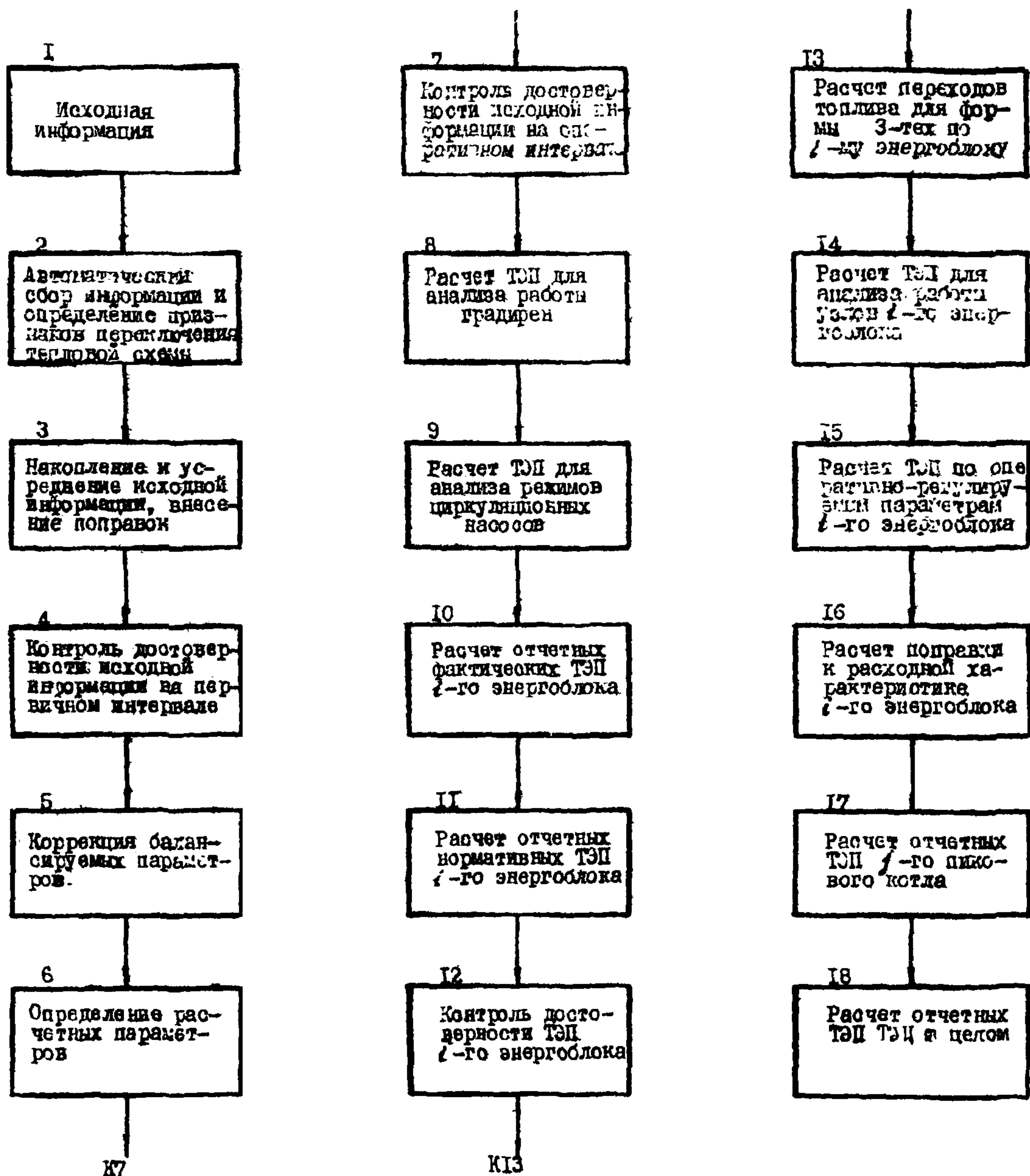
Рис.10. Технологическая последовательность обработки информации в Типовом алгоритме
