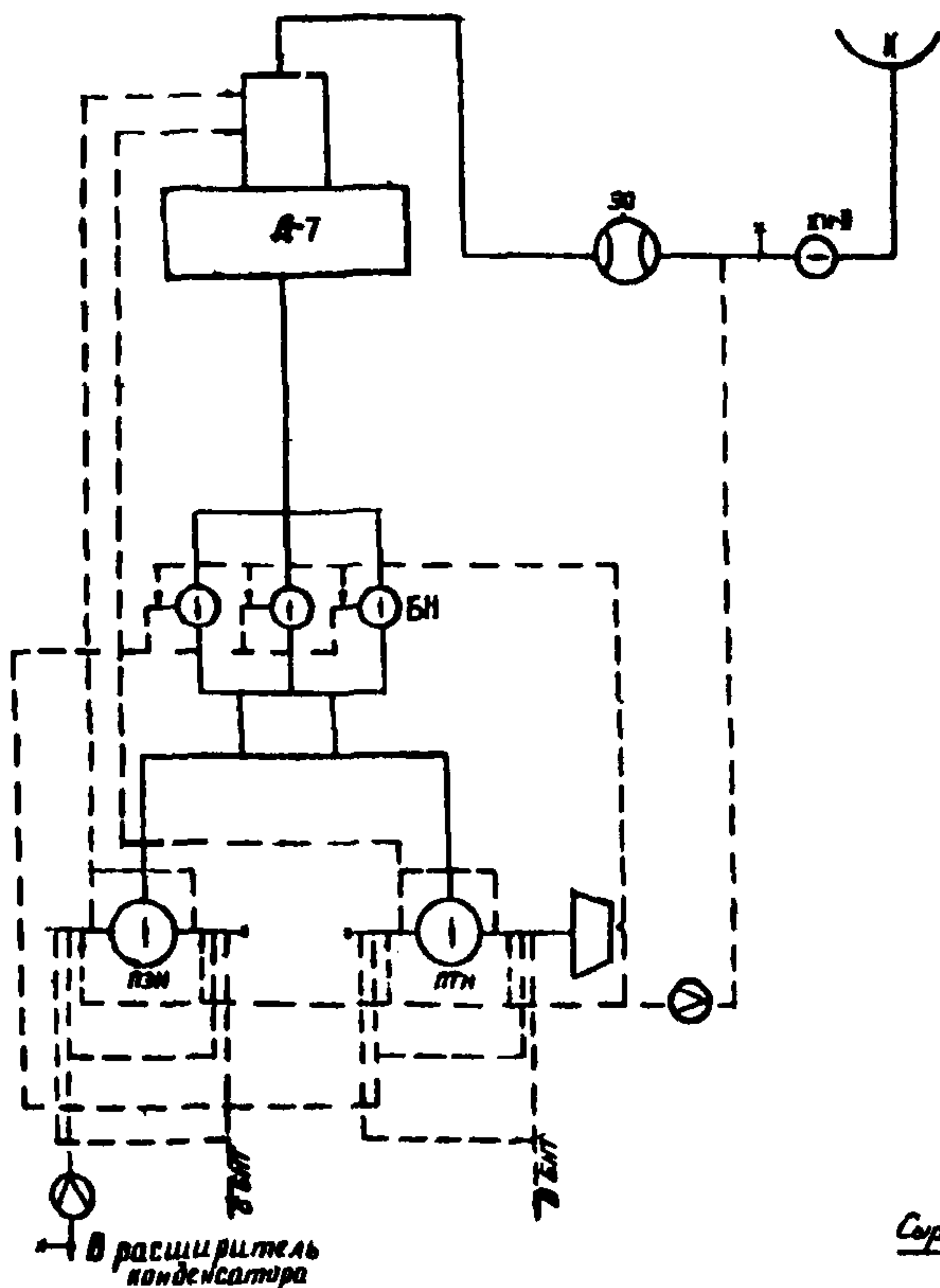
Рис. 3. Схема уплотнений питательных насосов турбины Т-250/300-240 с точками измерений для анализа их технического состояния. Обозначения см. рис. 1
