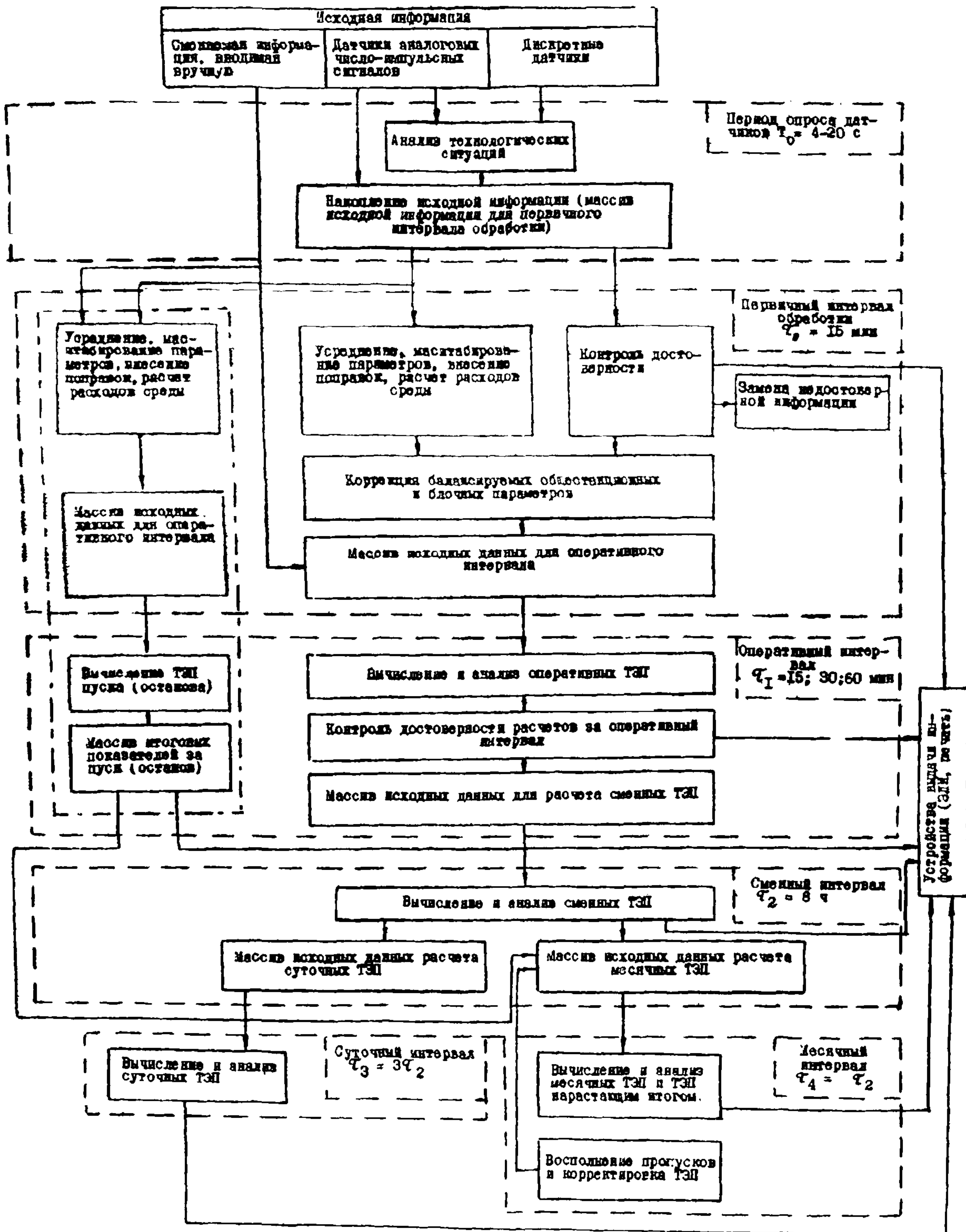
Рис. 9. Основные параметры расчета показателей энергоблоков и ТЭЦ в целом на различных временных интервалах: - - - - граница временных интервалов; -.-.-.- алгоритм расчета во время пуска (останова)
