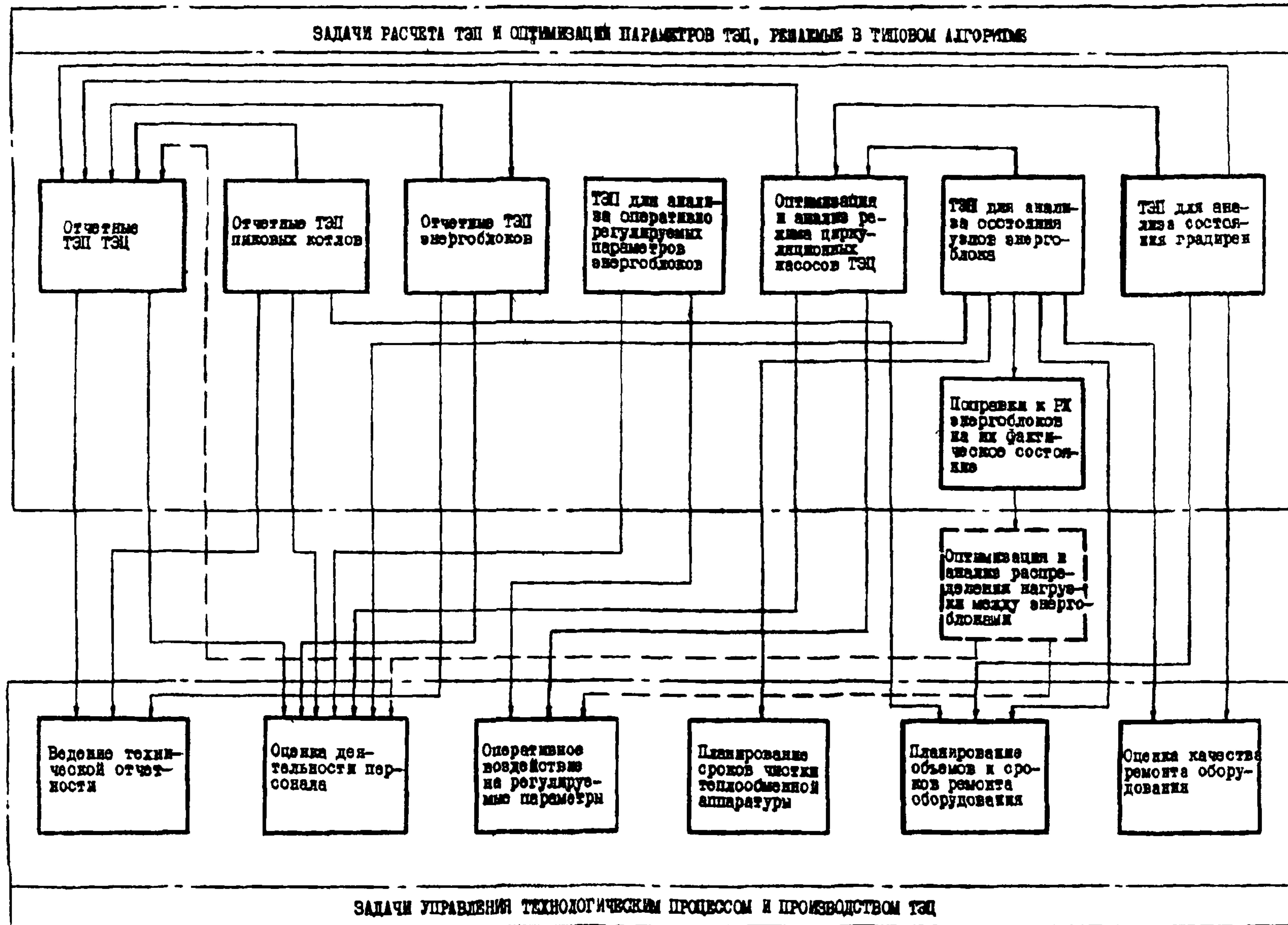
Рис. 8. Взаимосвязь задач расчета ТЭП и оптимизации параметров, решаемых в Типовом алгоритме, с задачами управления технологическим процессом и производственно-хозяйственной деятельностью ТЭЦ
