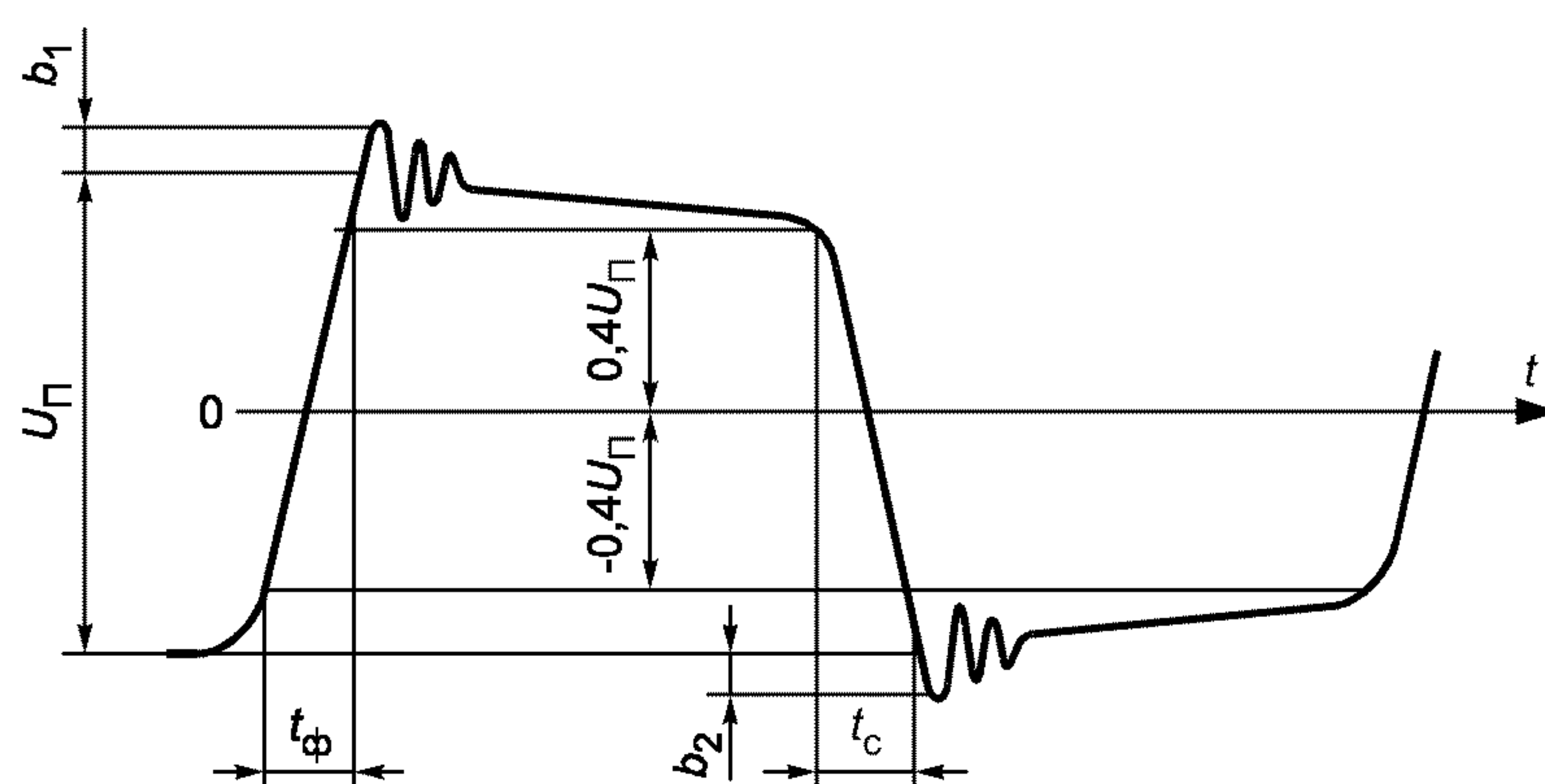
Рисунок 15 — Форма выходного сигнала устройства интерфейса
