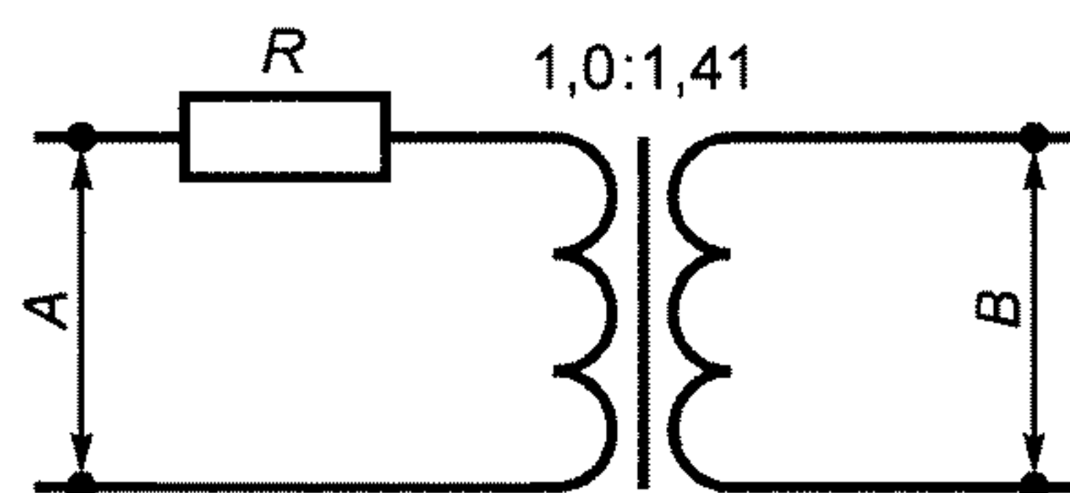
Рисунок 11 — Согласующий трансформатор
