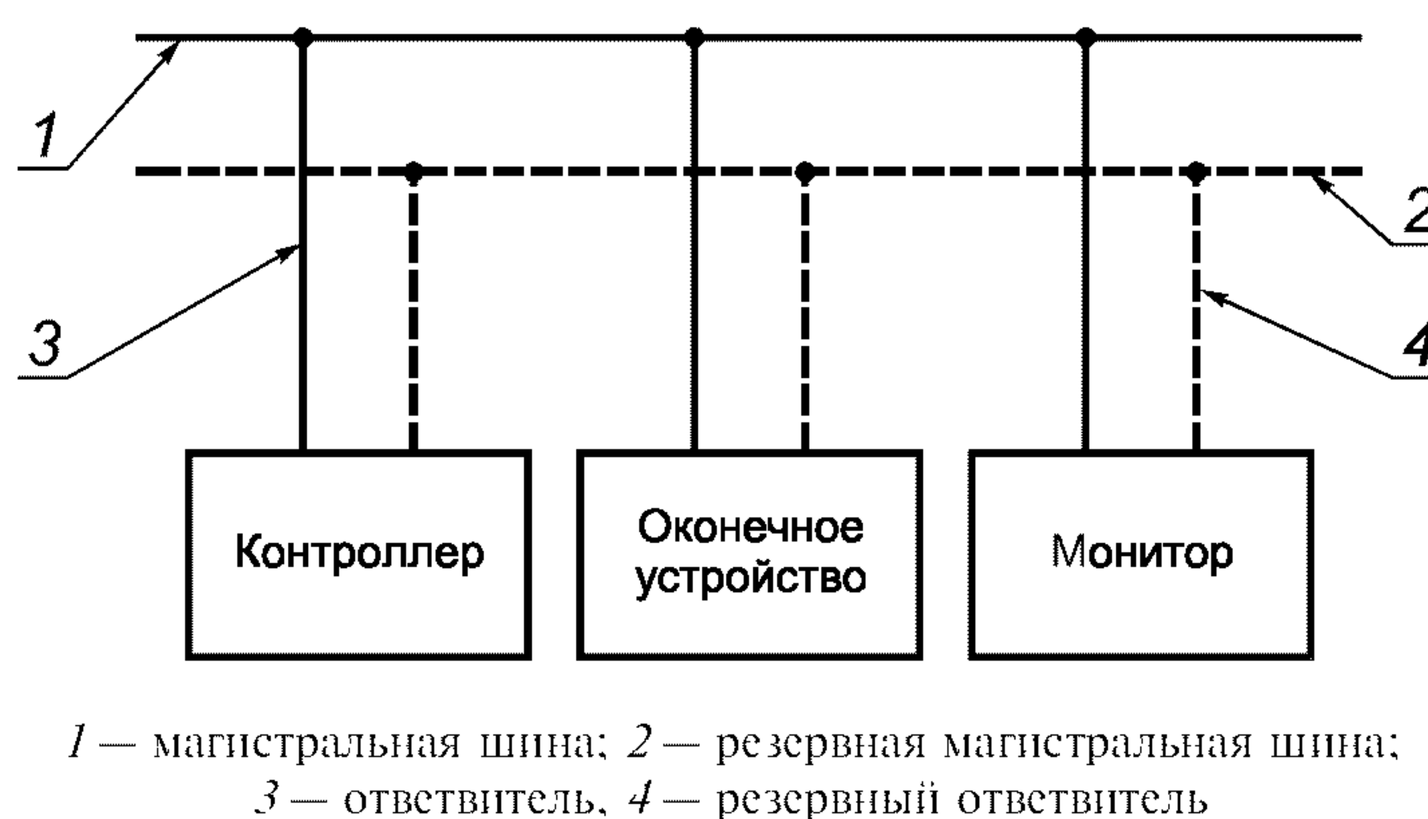
Рисунок 1 — Структурная схема технических средств интерфейса
