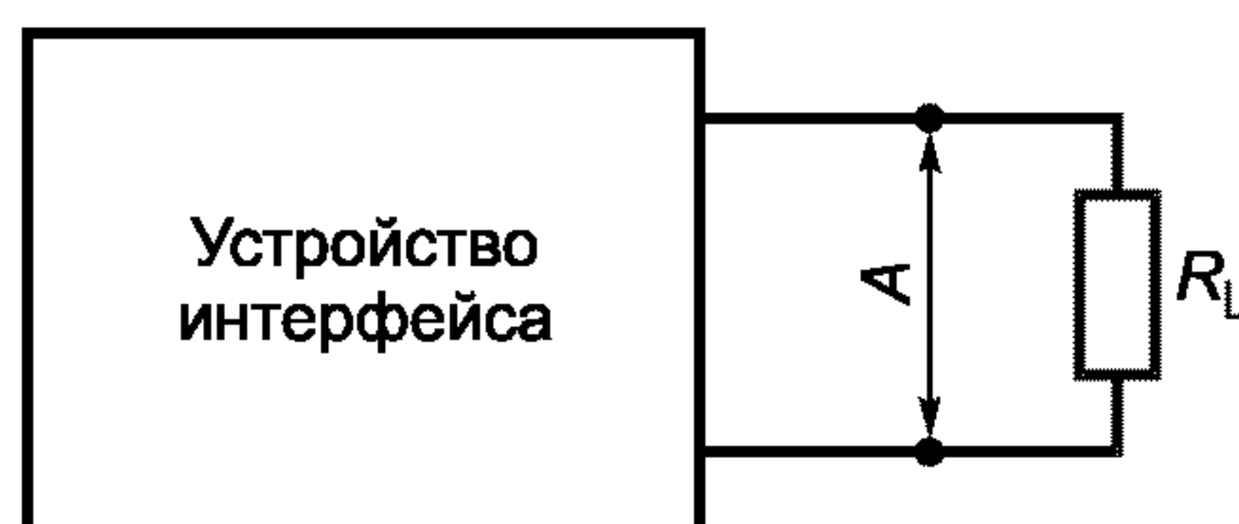
Рисунок 14 — Схема измерения выходных характеристик устройства интерфейса
