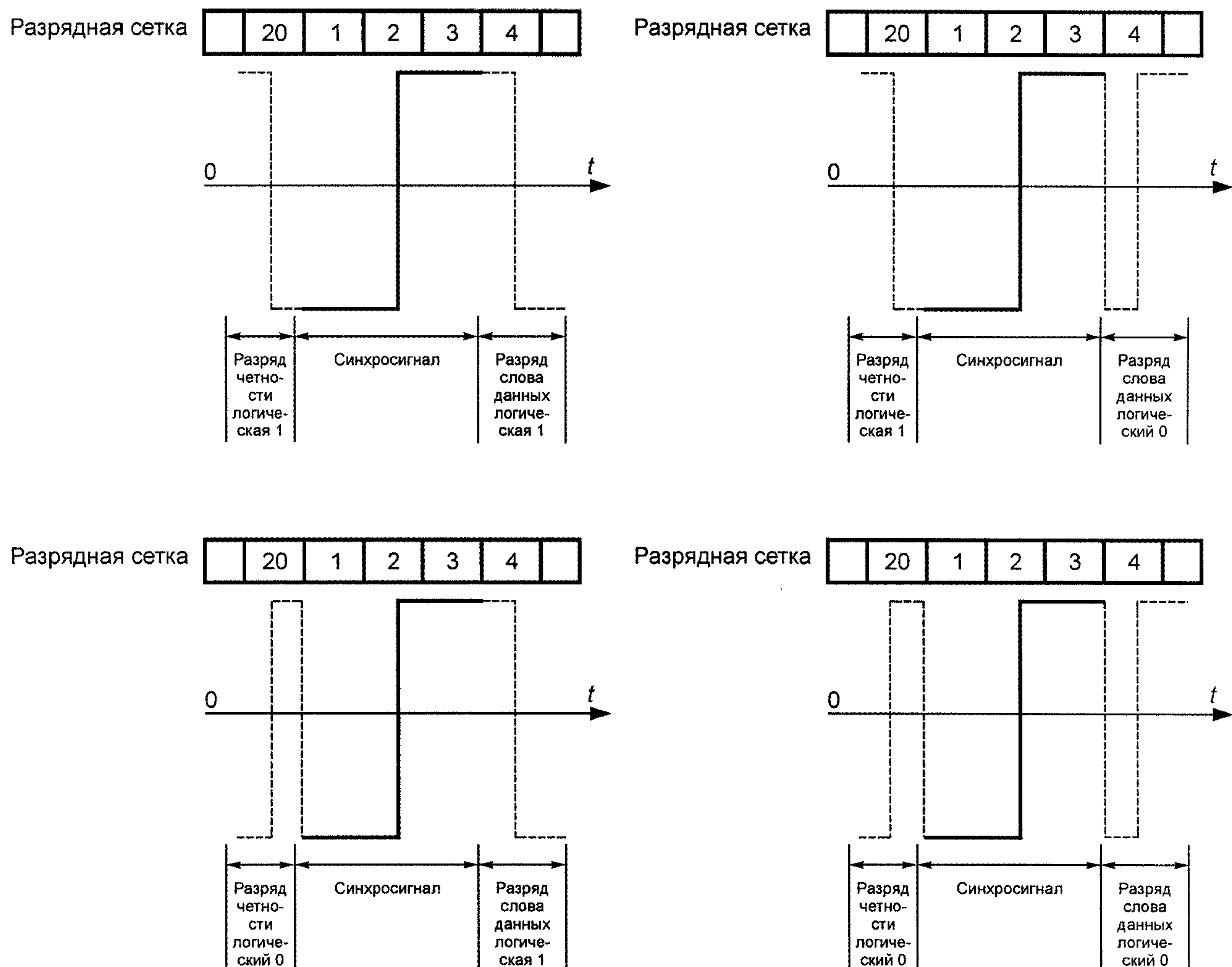
Рисунок 7 — Синхросигналы слов данных
