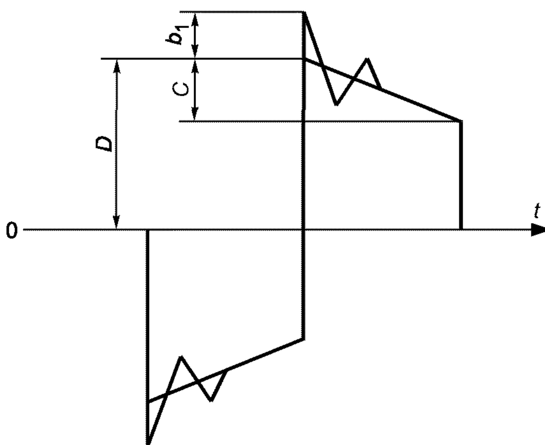
Рисунок 12 — Форма импульса на выходе согласующего трансформатора
