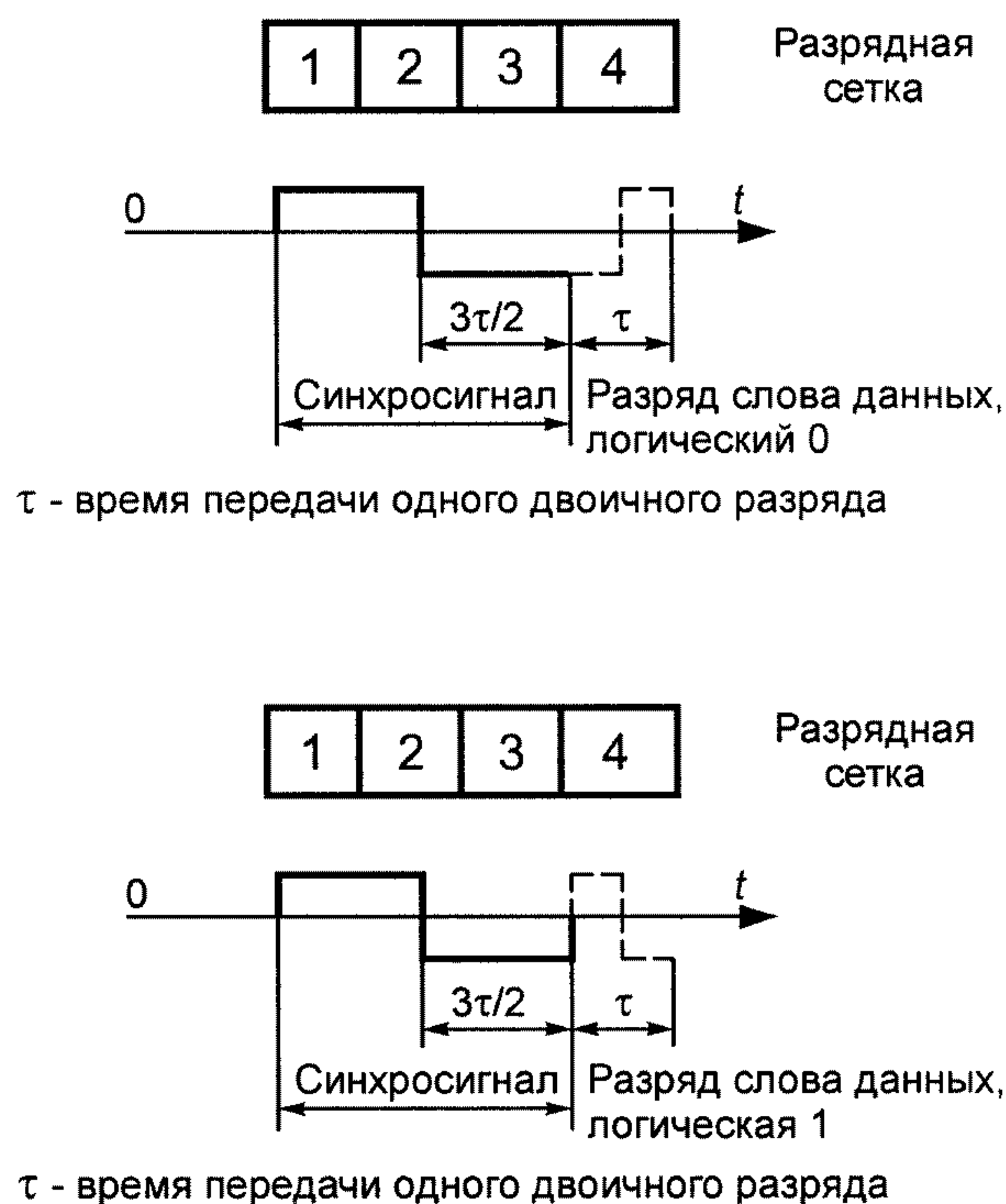
Рисунок 4 — Синхросигнал командного и ответного слов
