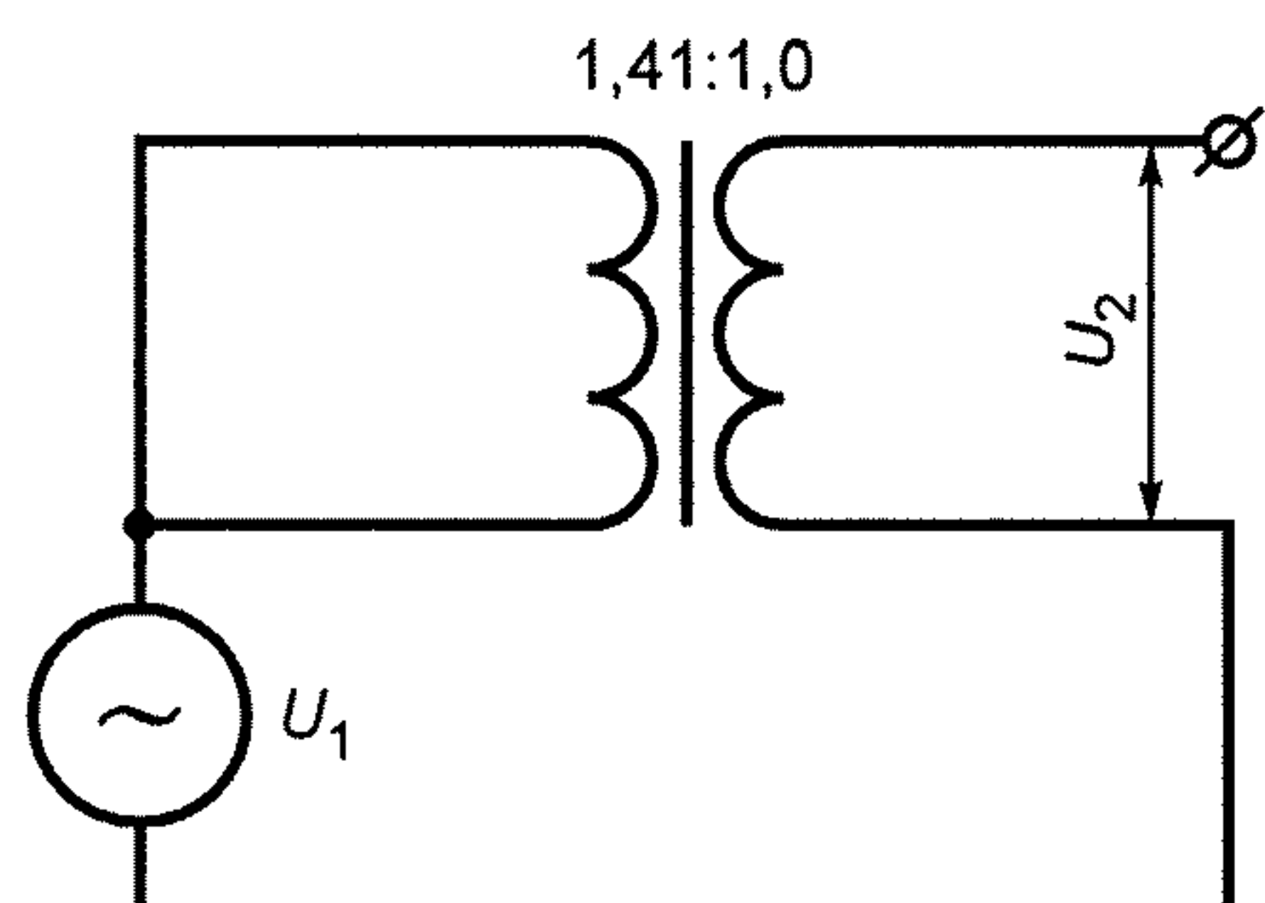
Рисунок 13 — Схема измерения ослабления синфазного сигнала согласующего трансформатора
