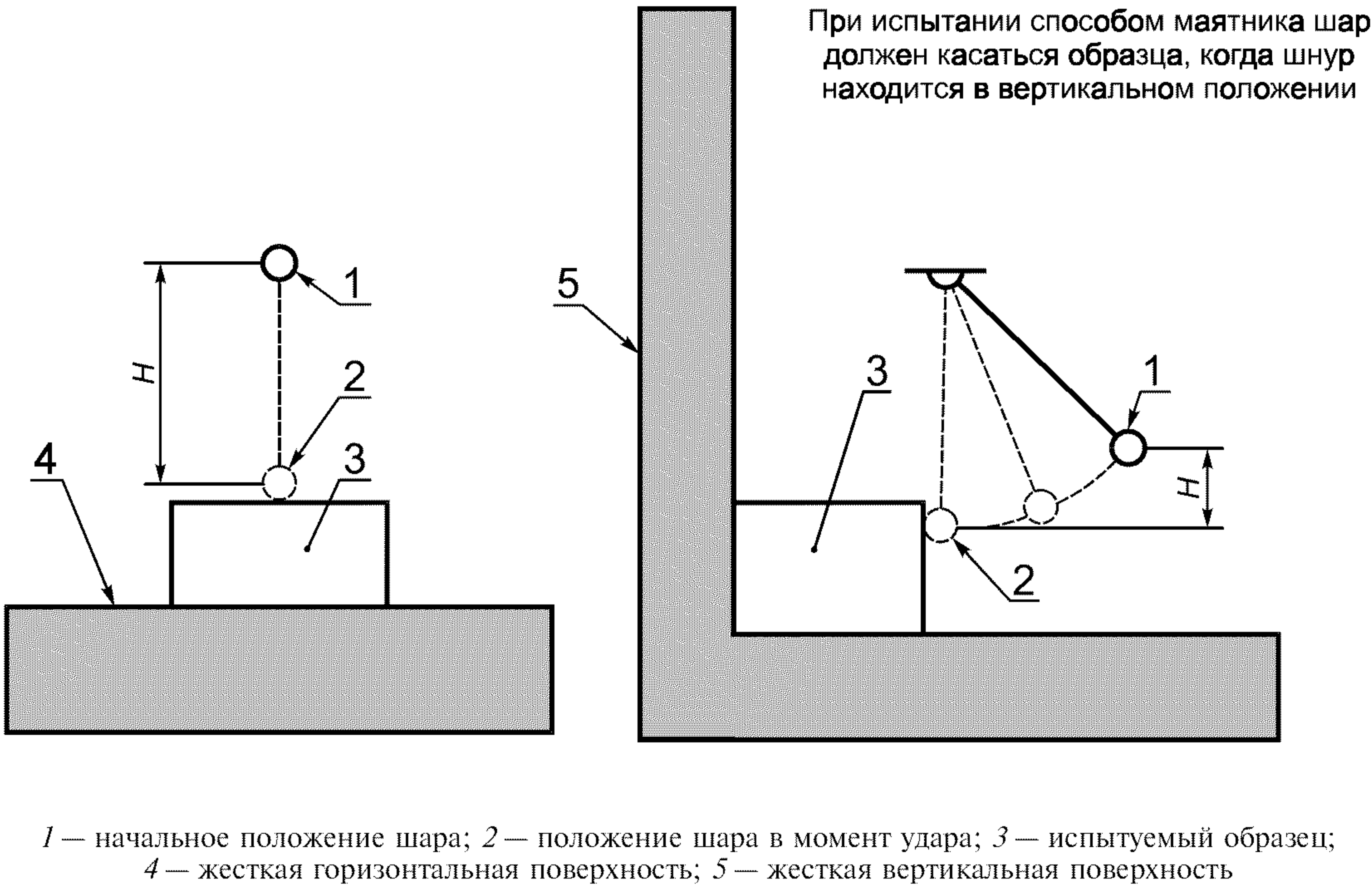
Рисунок 6 — Процедура испытаний на ударостойкость
