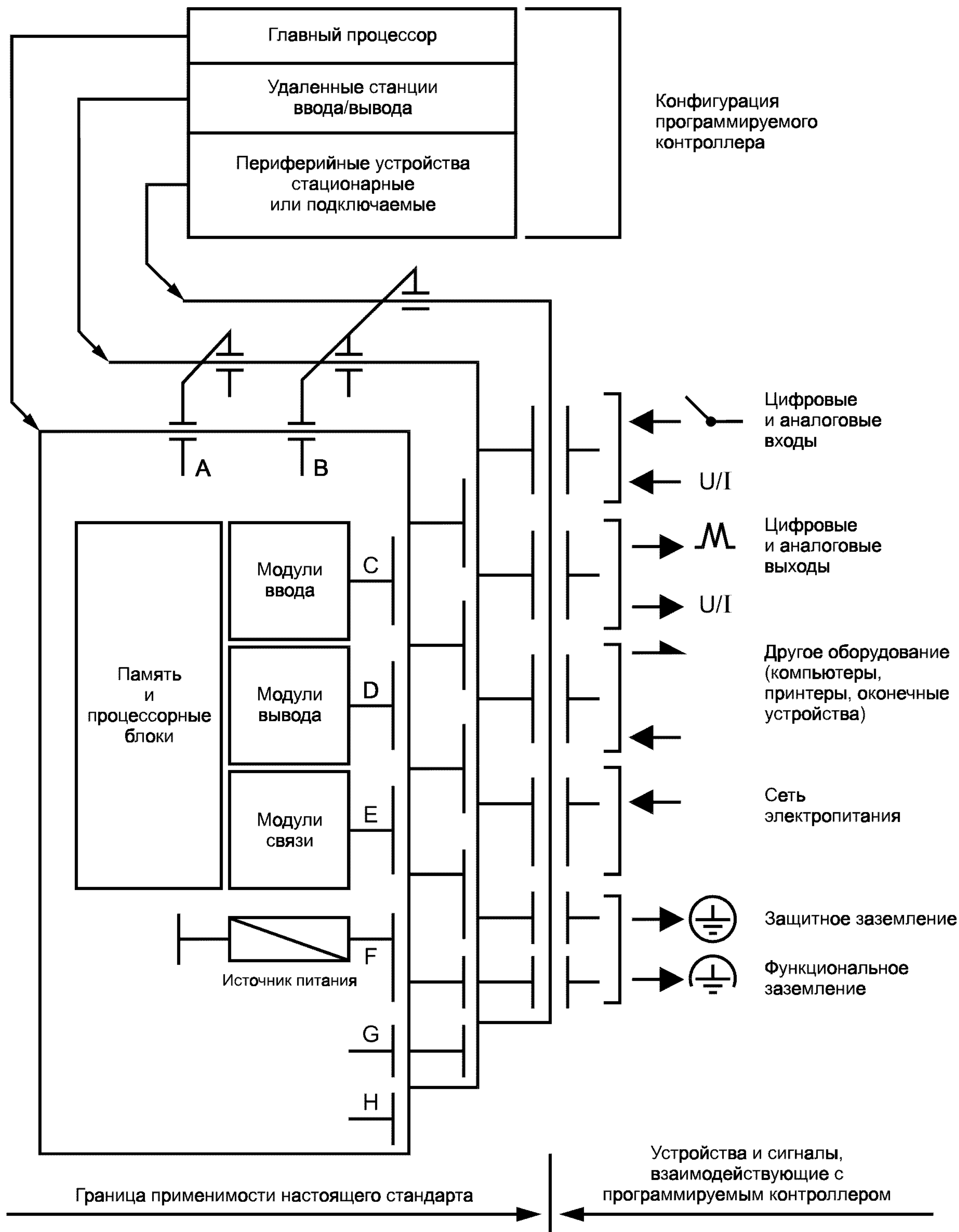
A — интерфейс для удаленных станций ввода/вывода; B — интерфейс для периферийных устройств; C — интерфейс для цифровых и аналоговых входных сигналов; D — интерфейс для цифровых и аналоговых выходных сигналов; E — последовательные или параллельные интерфейсы передачи данных другому оборудованию; F — интерфейс источников электропитания; G — интерфейс защитного заземления; H — интерфейс функционального заземления
