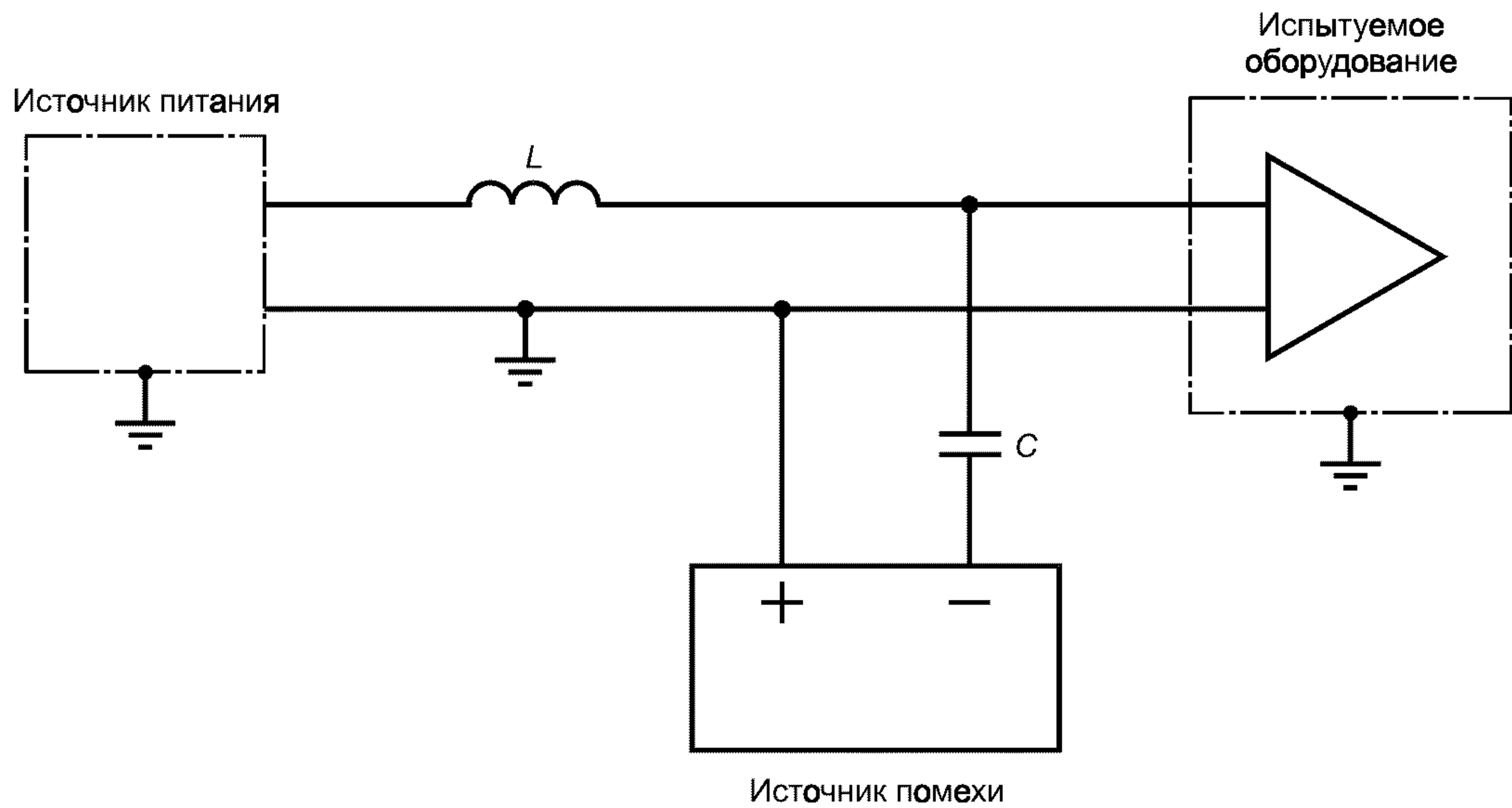
Рисунок 9 — Схема соединений при испытаниях на устойчивость к затухающему колебательному напряжению
