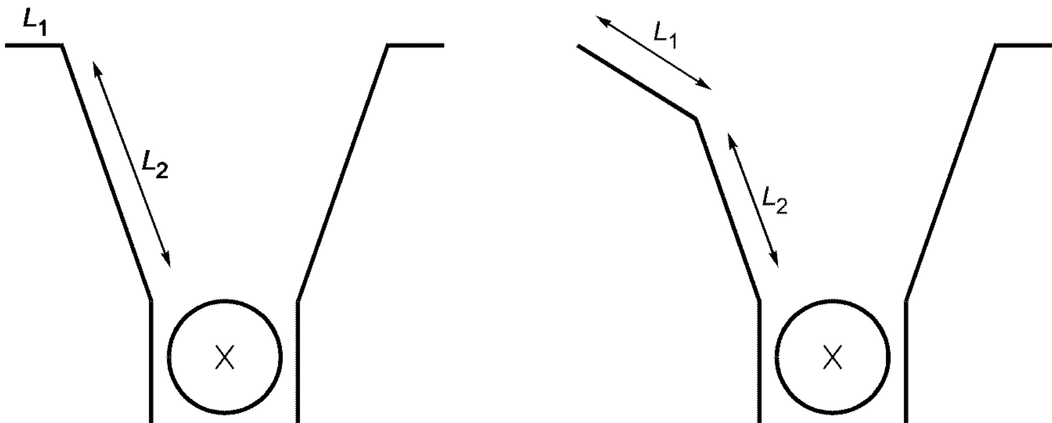
Рисунок 1 — Порядок измерений безопасного расстояния
