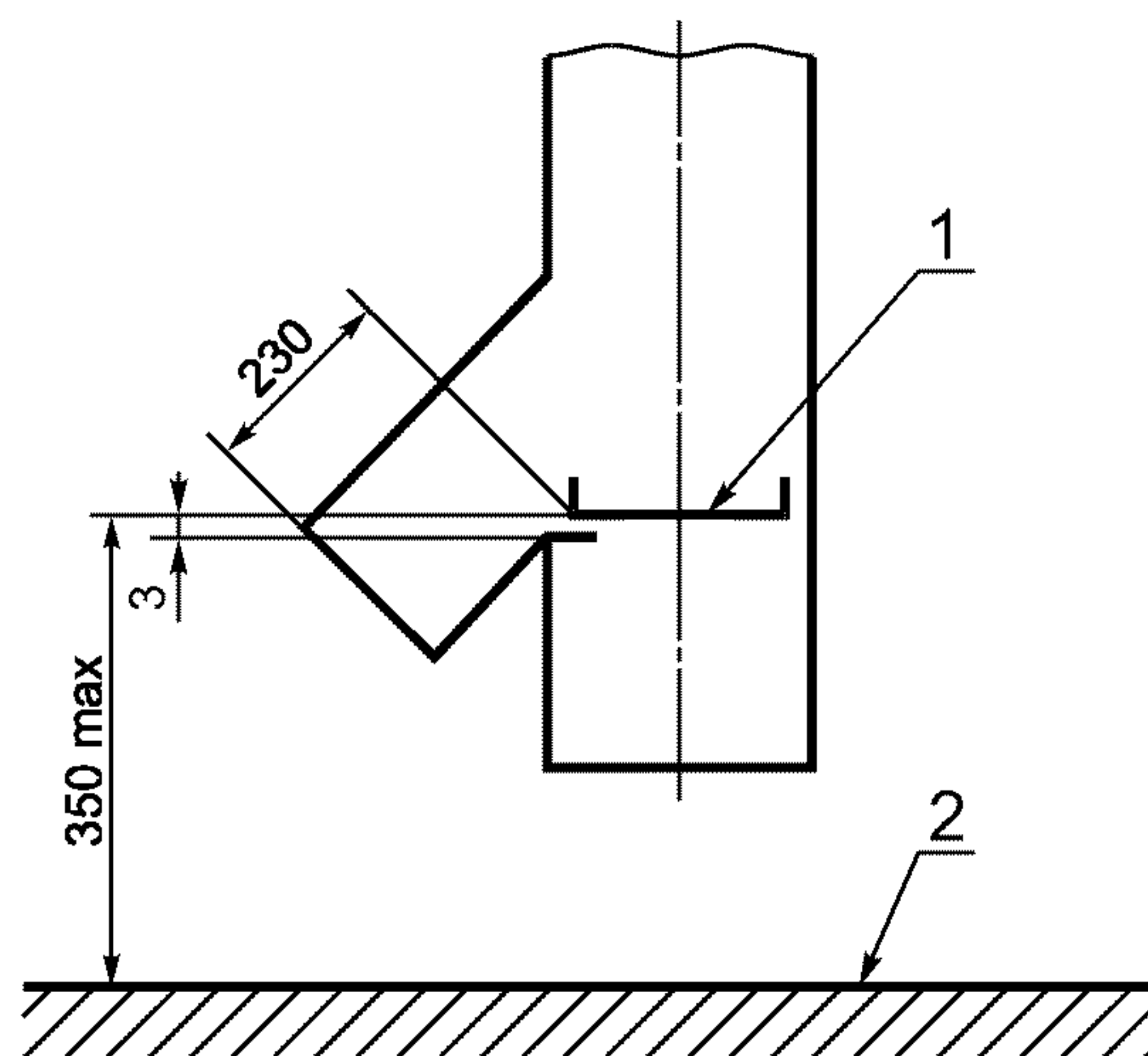
1 — режущий механизм; 2 — земля
