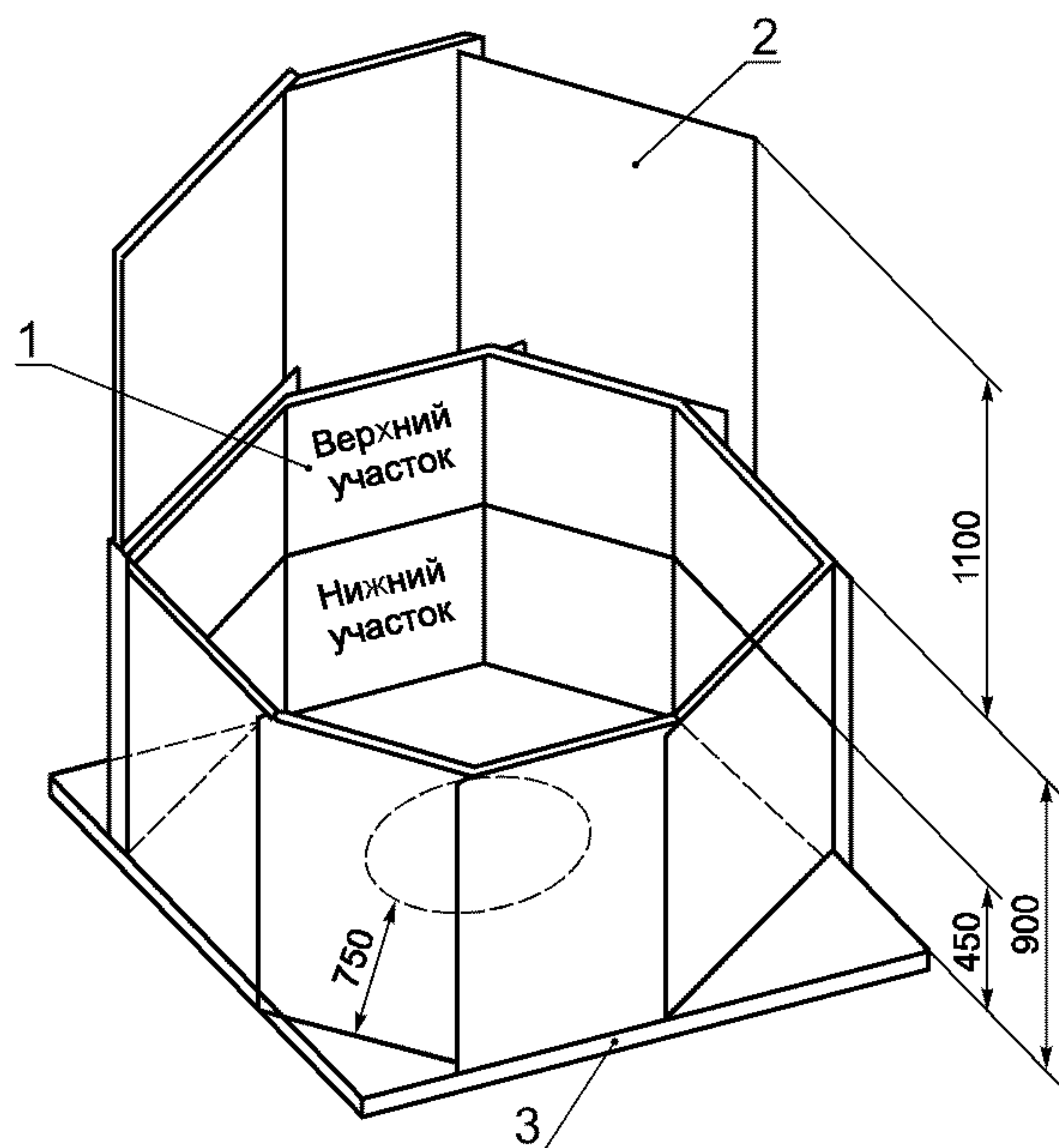
1 — панель с мишенью; 2 — листы крафт-бумаги; 3 — основание
