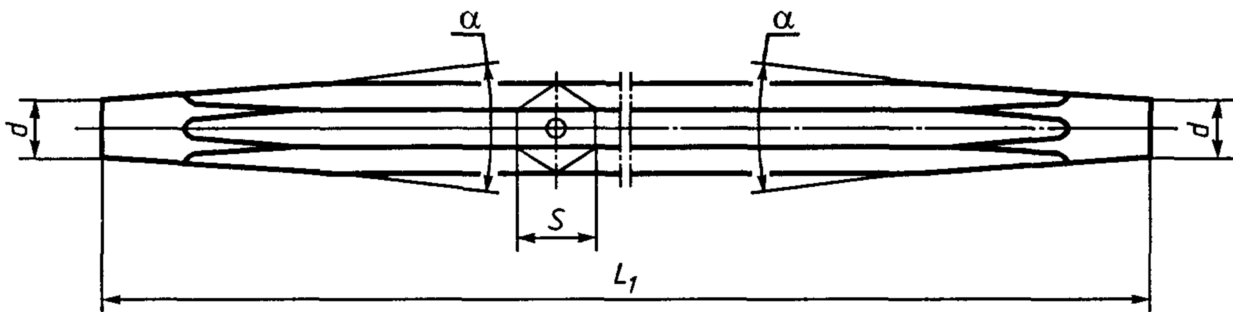
Рисунок 2 — Буровые и удлинительные штанги с конусом
