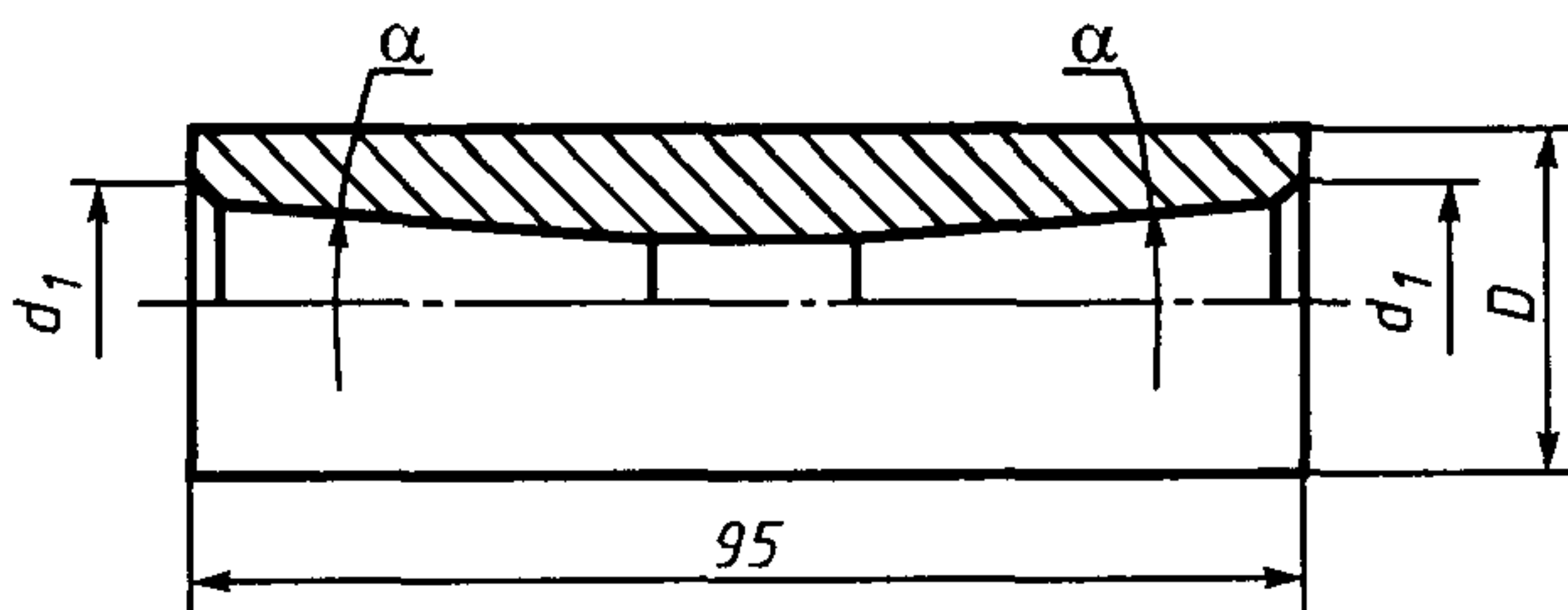
Рисунок 3 — Соединительная муфта
