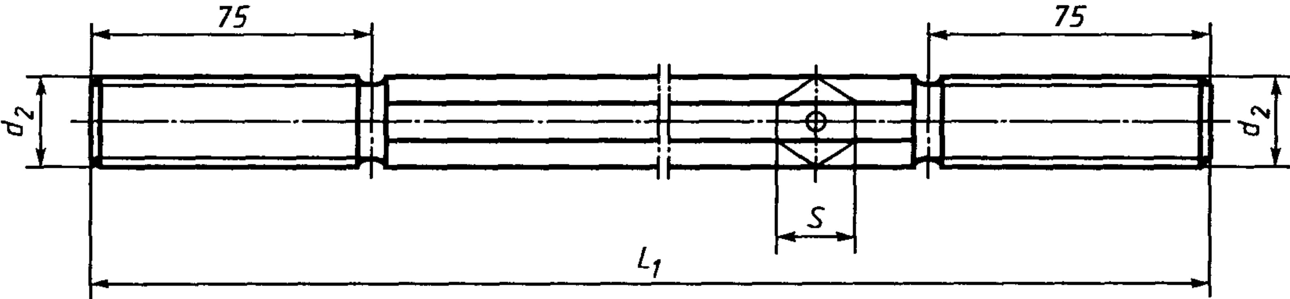
Рисунок 5 — Буровые и удлинительные штанги с резьбой
