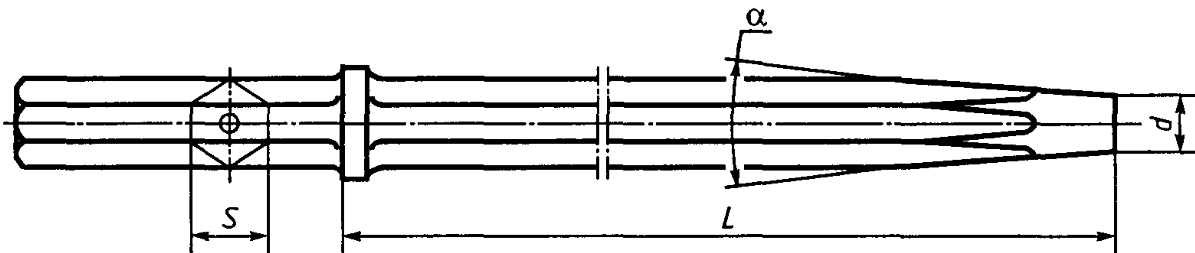
Рисунок 1 — Буровые штанги с конусом
