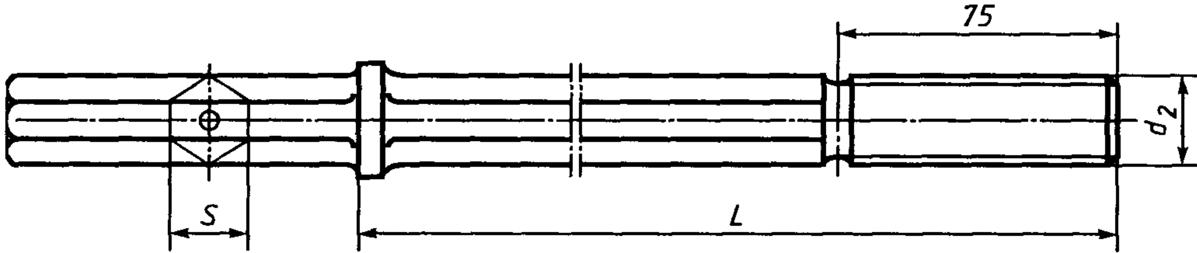
Рисунок 4 — Буровые штанги с резьбой
