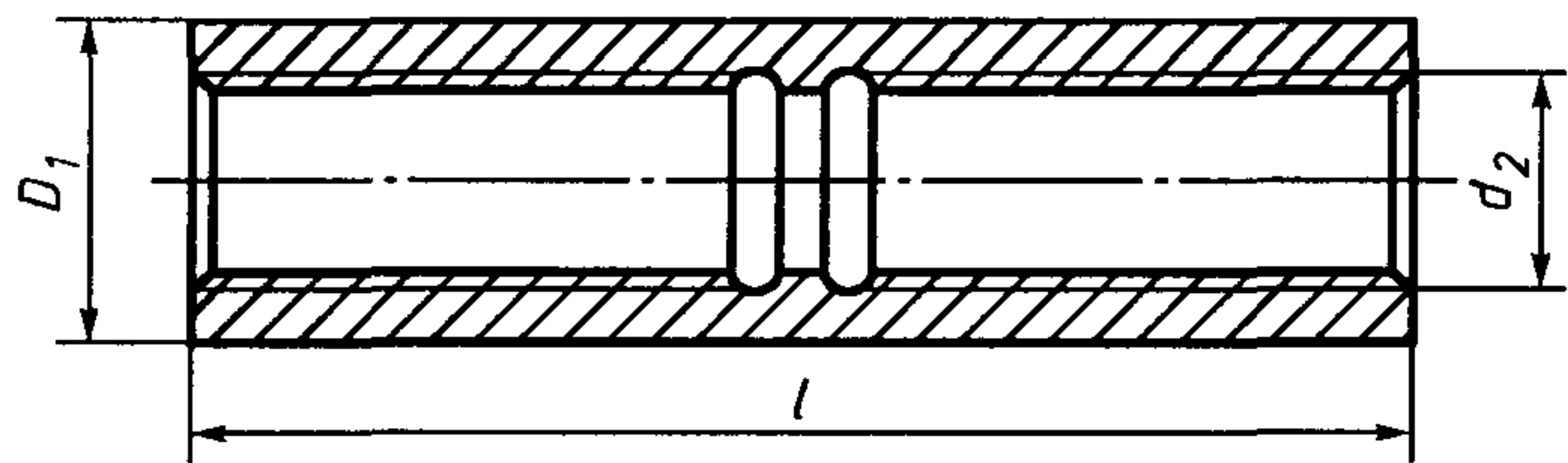
Рисунок 6 — Соединительная муфта
