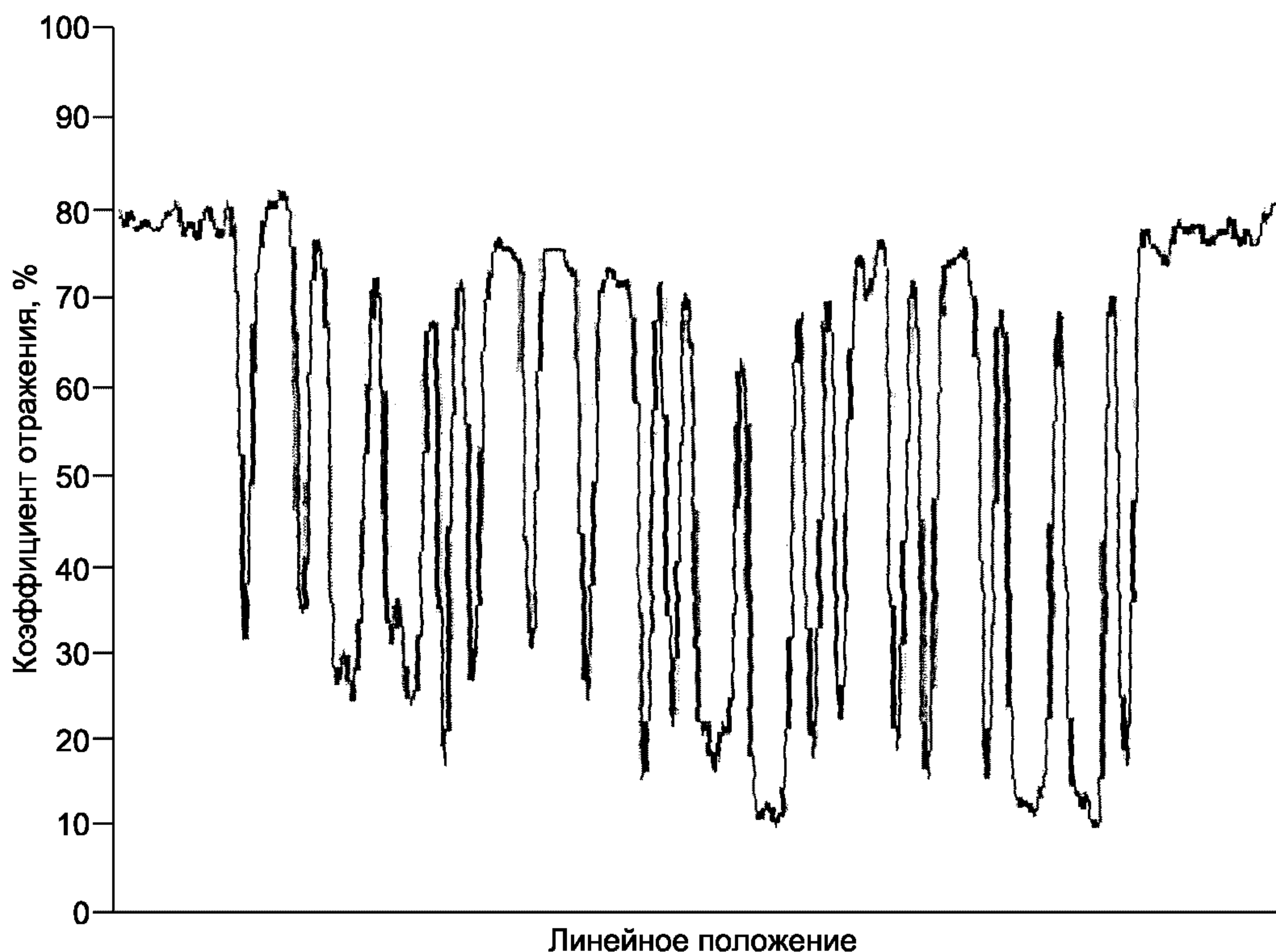
Рисунок 3 — Профиль отражения при сканировании
