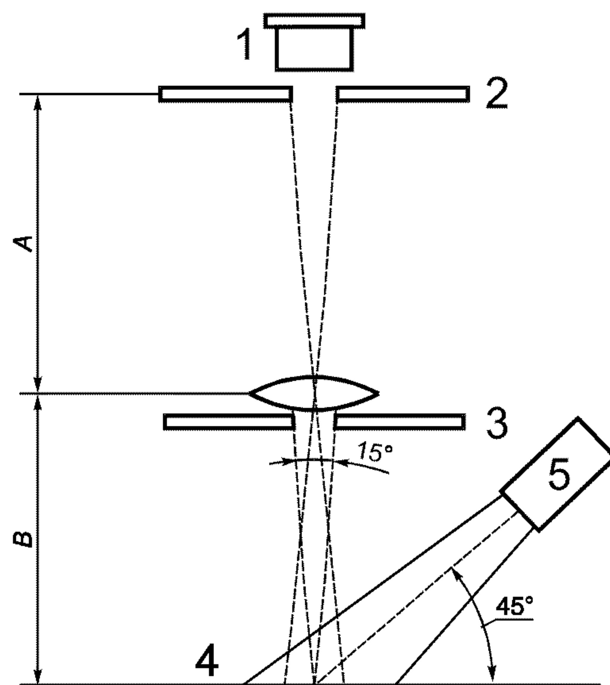
1 — фотоэlement; 2 — апертура при линейном увеличении 1:1 (размер A равен размеру B ); 3 — диафрагма; 4 — образец; 5 — источник оптического излучения
