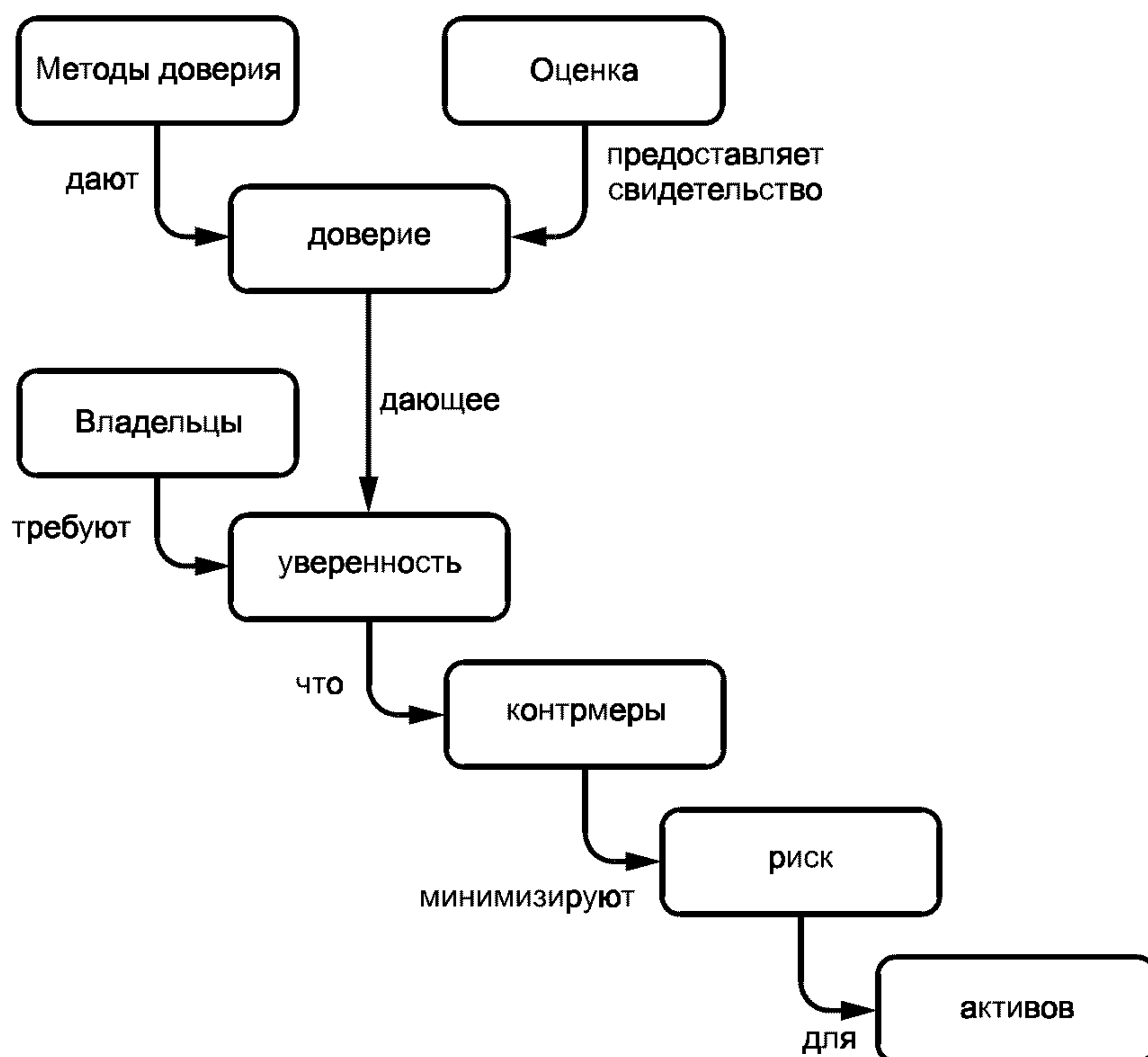
Рисунок 4.2 — Понятия, используемые при оценке, и их взаимосвязь
