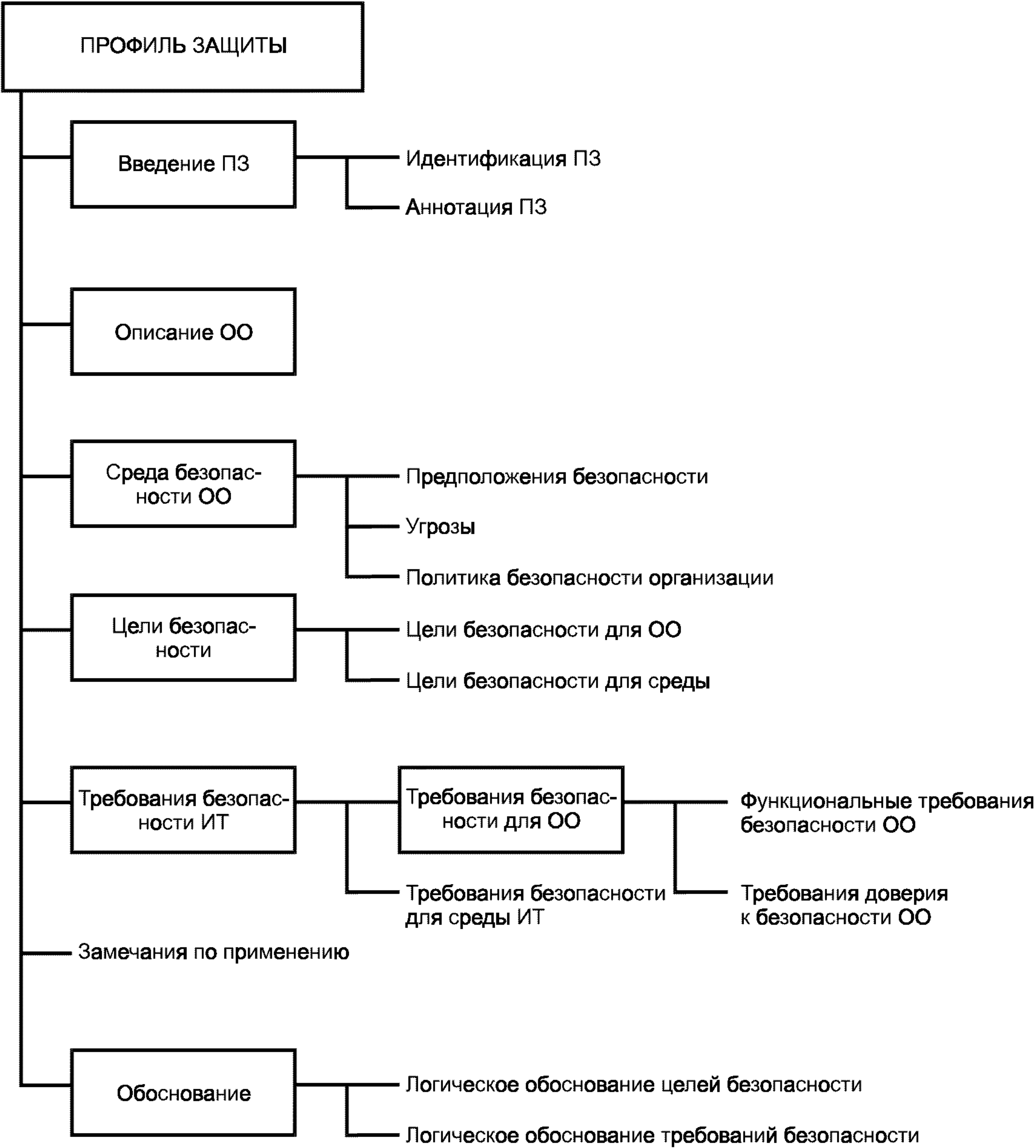
Рисунок Б.1 — Содержание профиля защиты
