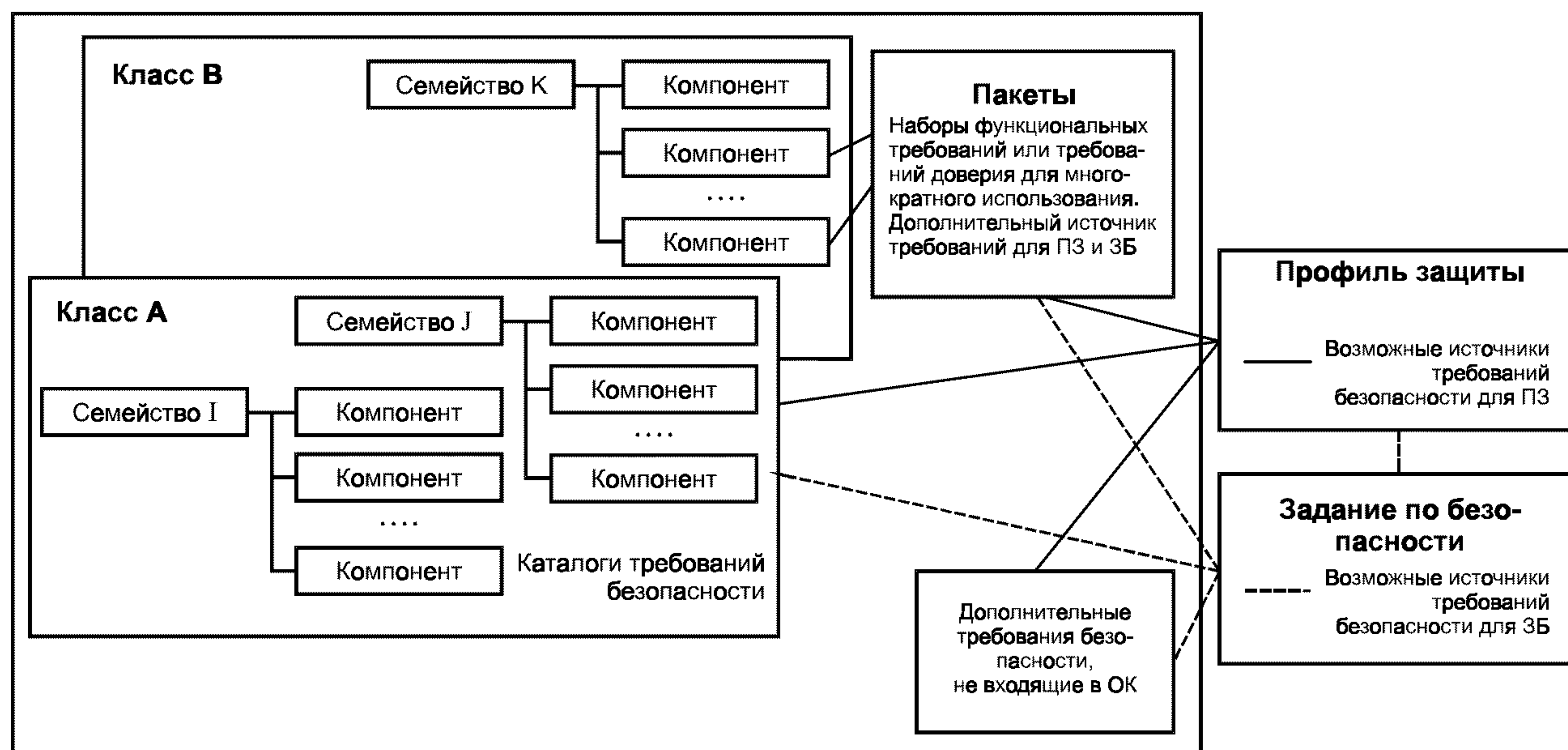
Рисунок 4.6 — Организация и структура требований
