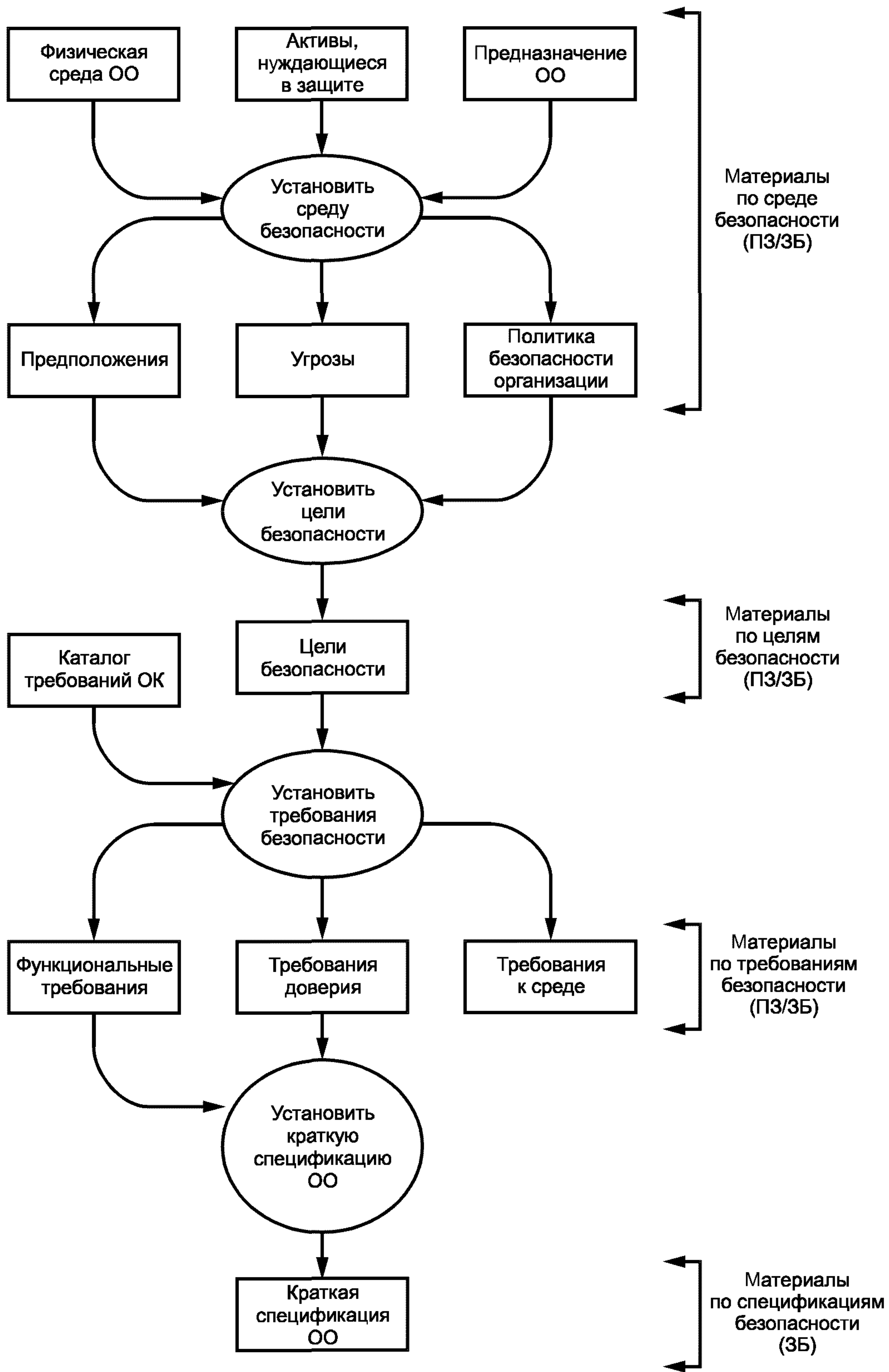
Рисунок 4.5 — Последовательное формирование требований и спецификаций
