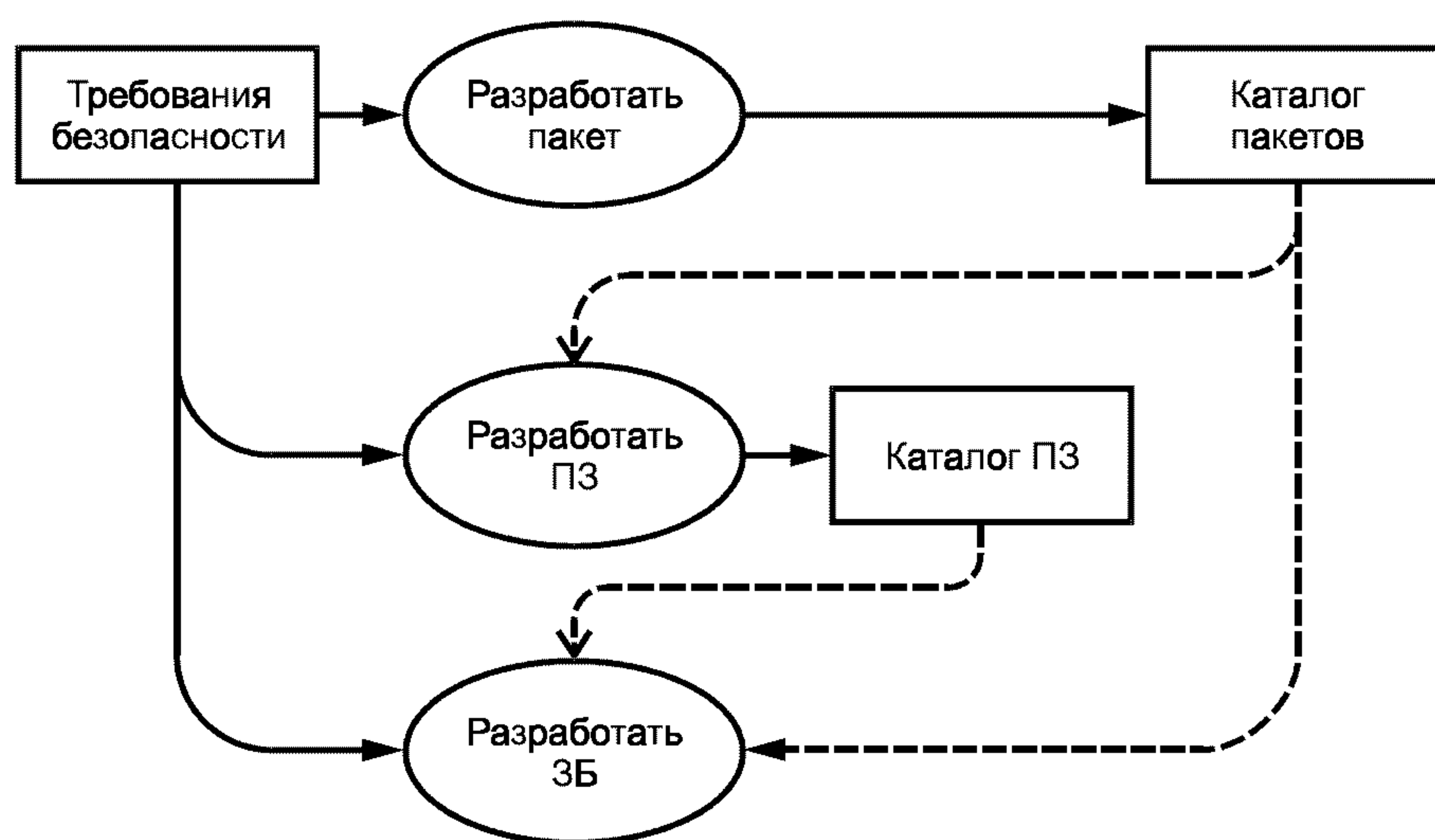
Рисунок 4.7 — Использование требований безопасности
