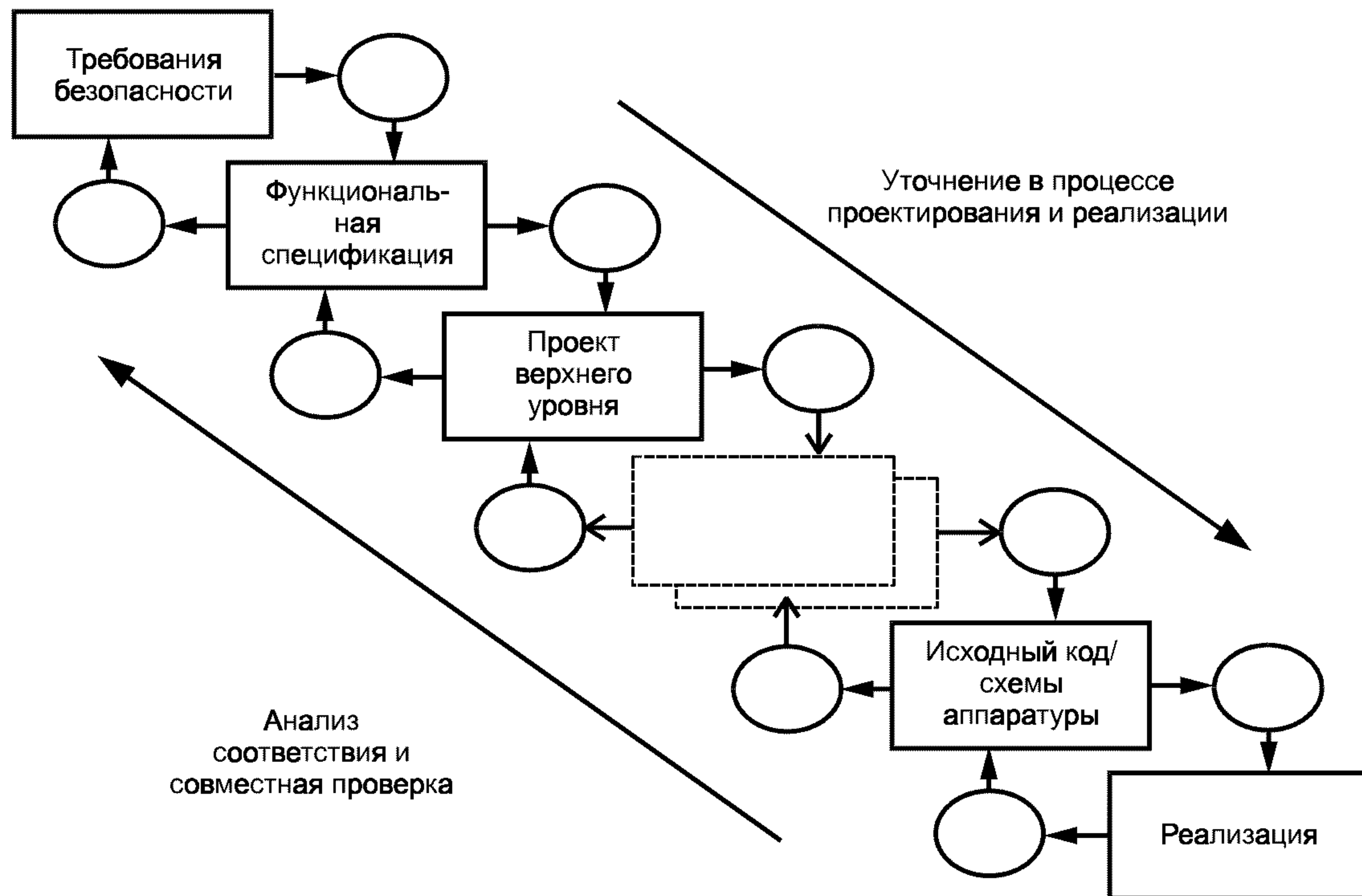
Рисунок 4.3 — Модель разработки ОО
