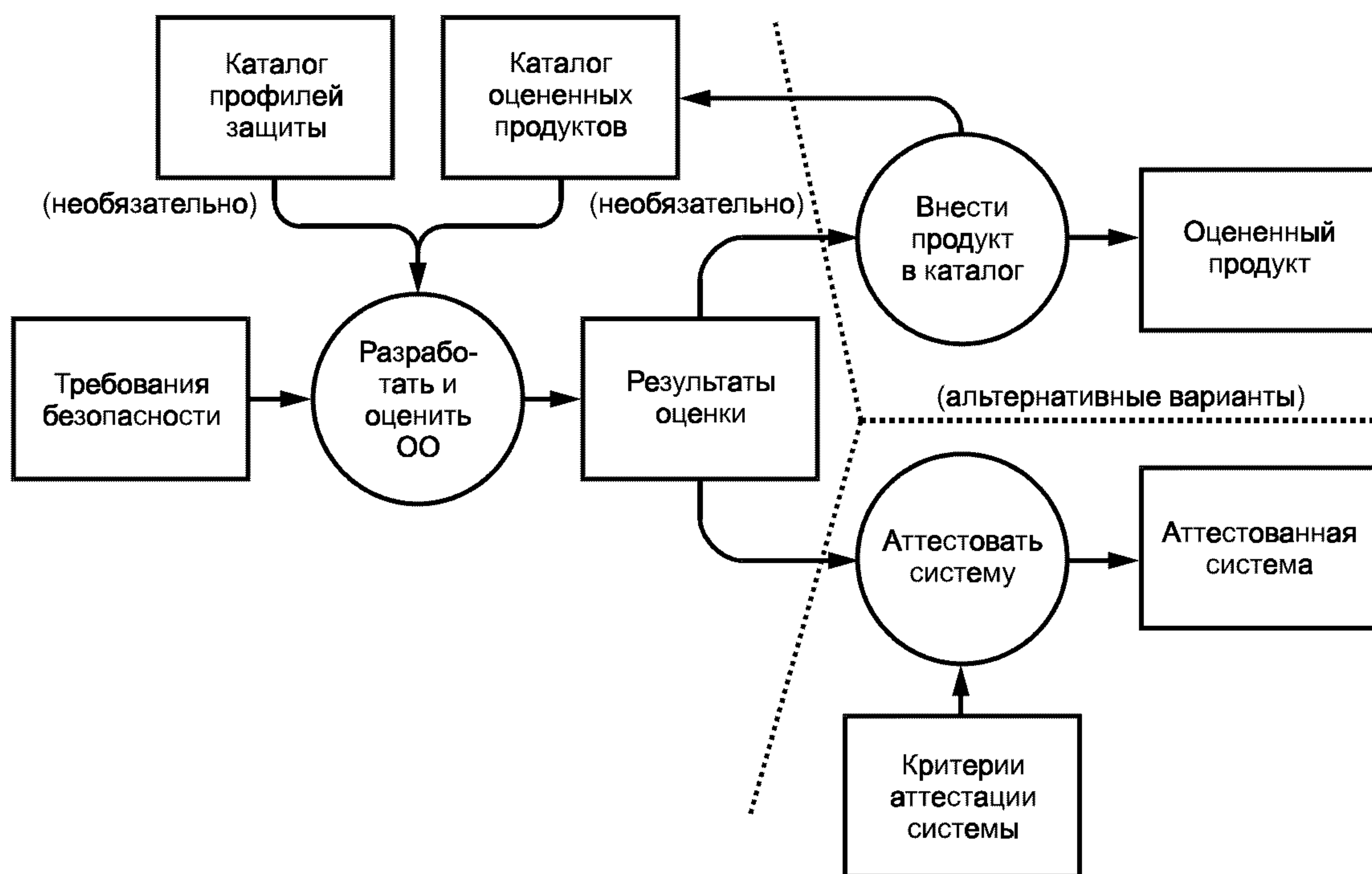
Рисунок 5.2 — Использование результатов оценки ОО
