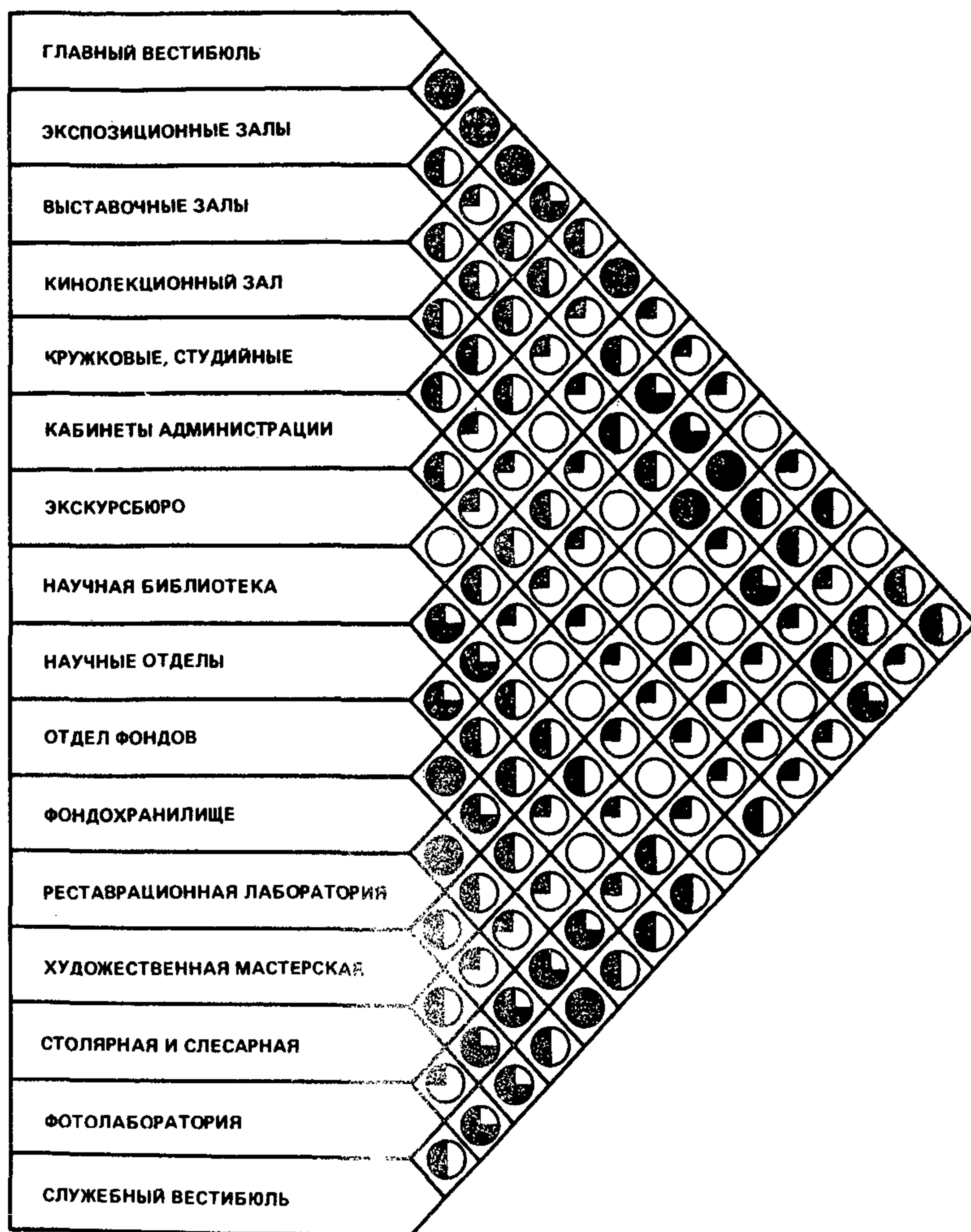
Рис. 2. Рекомендуемая степень взаимосвязи помещений
