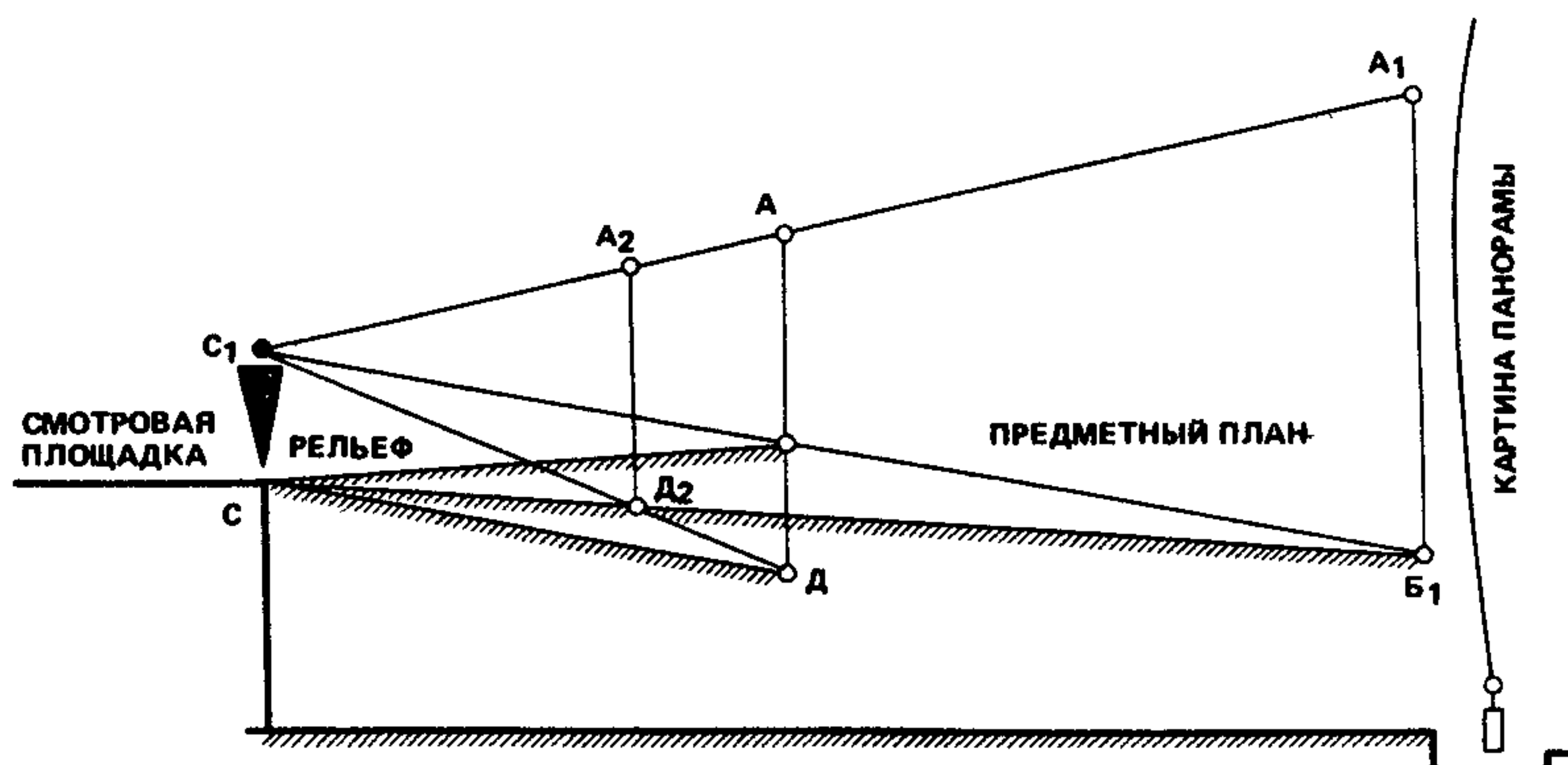
Рис. 17. Схема видимости на предметном плане
