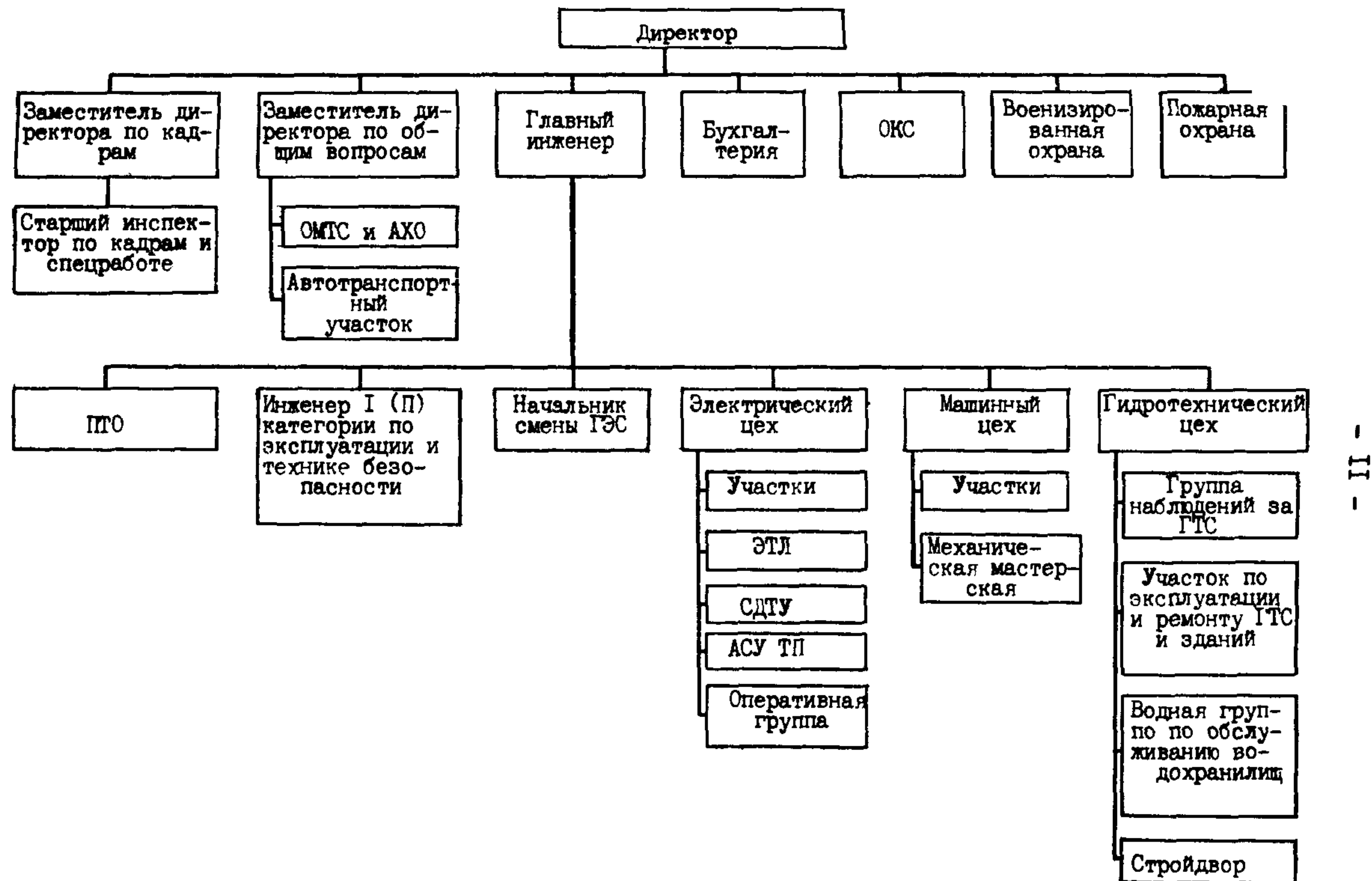
Рис.2. Организационная структура управления ГЭС мощностью свыше 1000 до 3000 тыс.кВт
