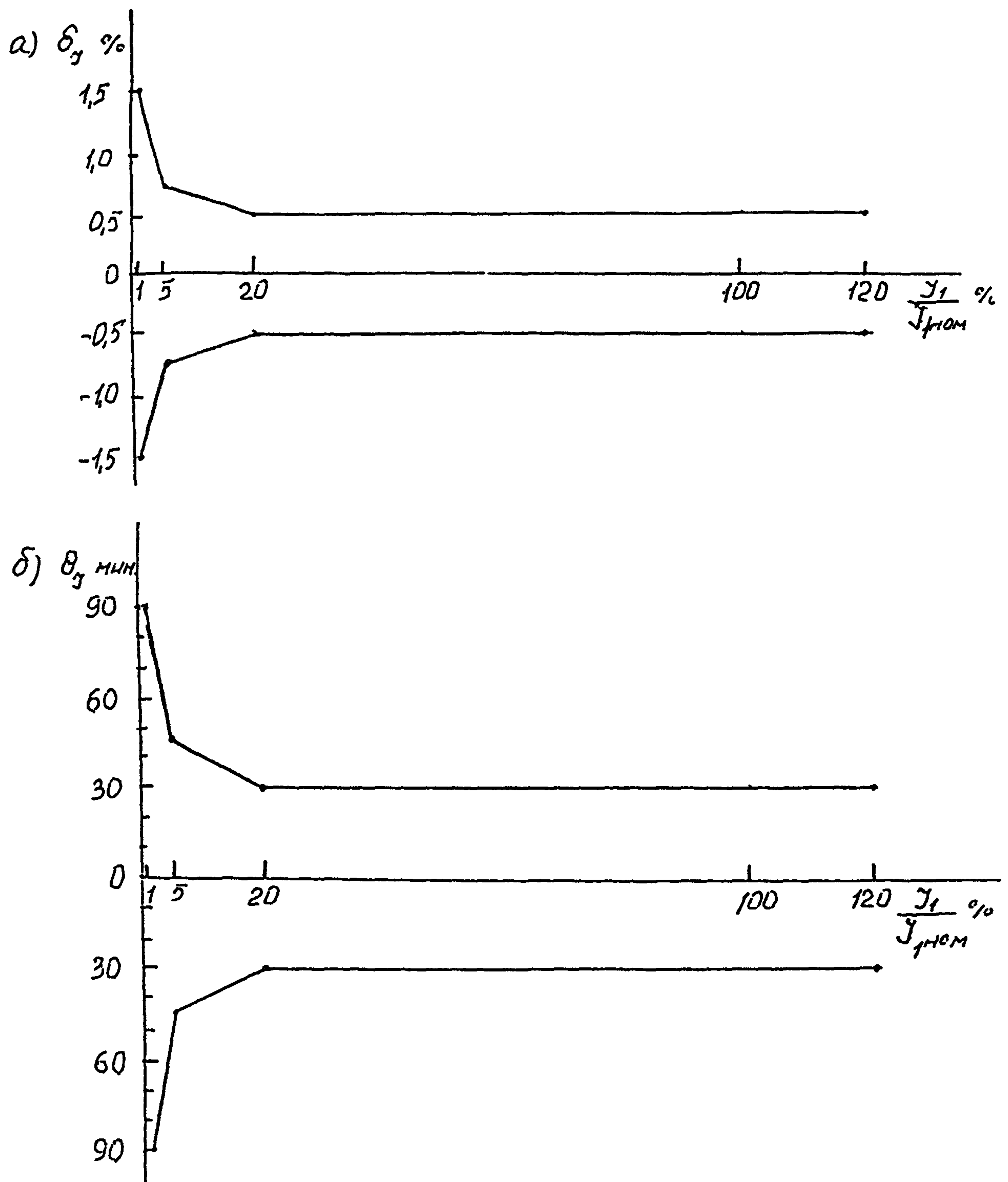
Рис П.2 6. Пределы допускаемых погрешностей трансформаторов тока класса точности 0,5 S по ГОСТ 7746-89: а) токовой; б) угловой.
