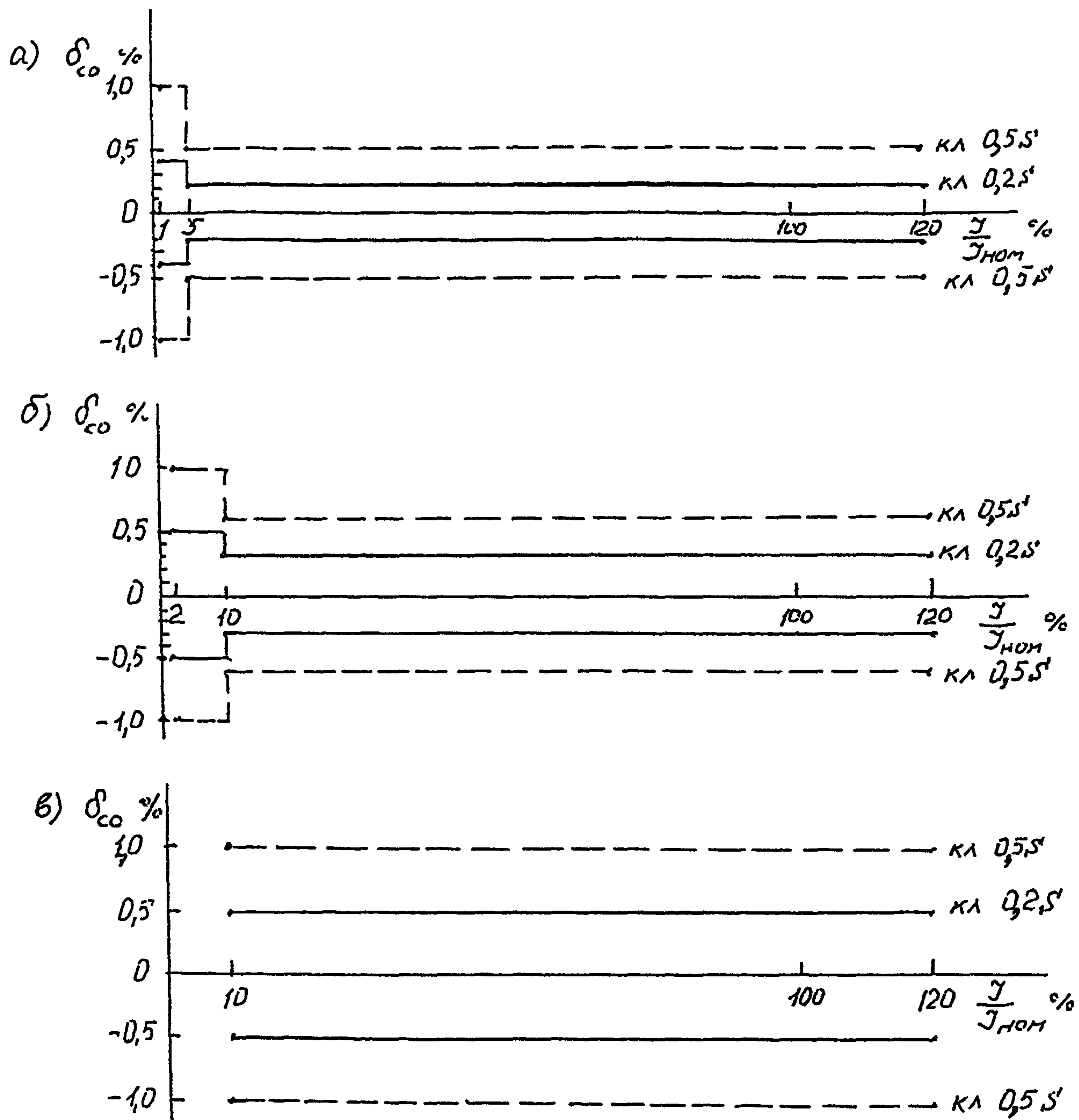
Рис. П.2.7 Предел допускаемой относительной погрешности электронных счетчиков активной энергии по ГОСТ 30206-94 (однофазные и многофазные счетчики с симметричными нагрузками):
