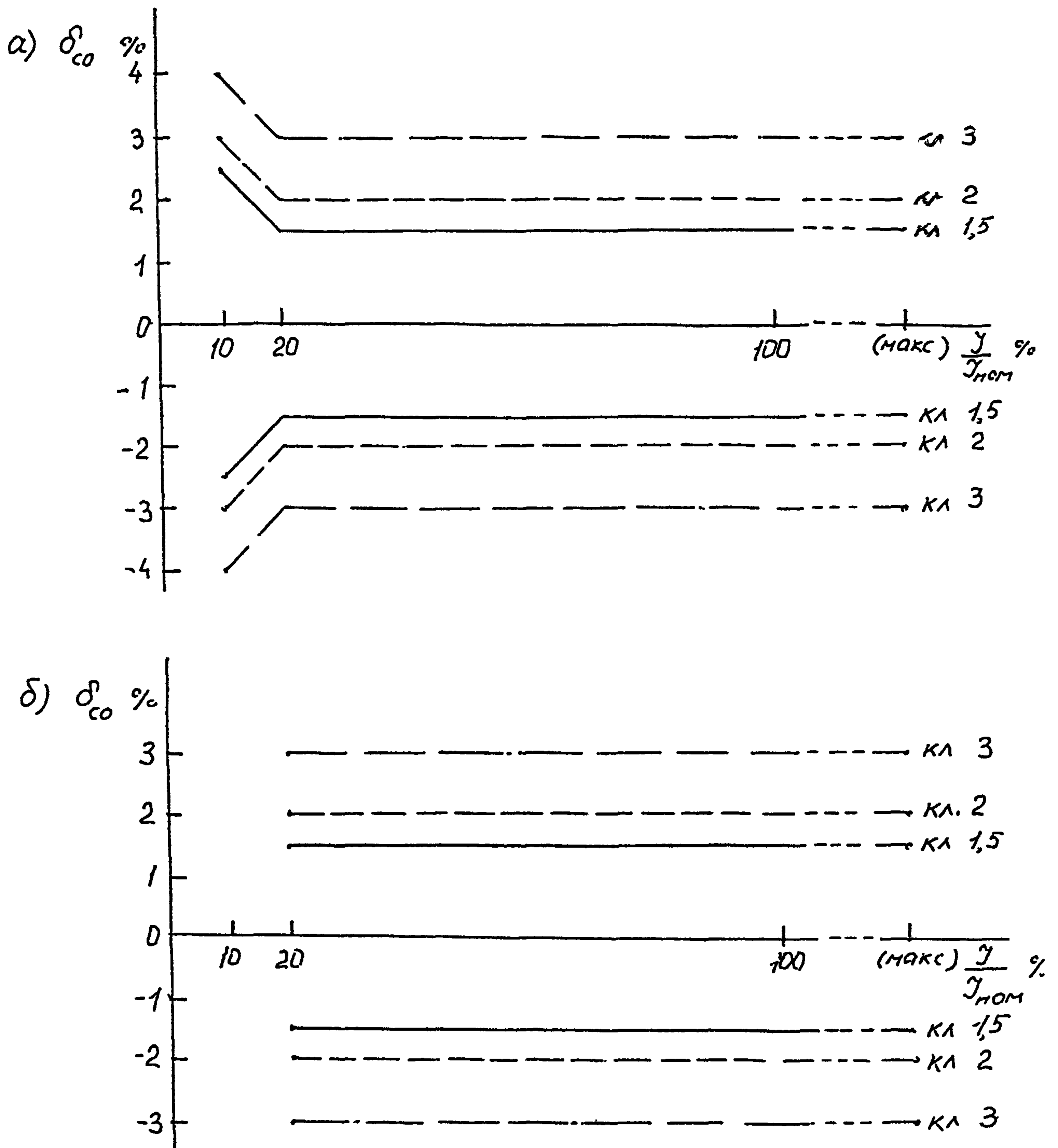
Рис П.2 13. Пределы допускаемой относительной погрешности индукционных счетчиков реактивной энергии по ГОСТ 6570-75:
