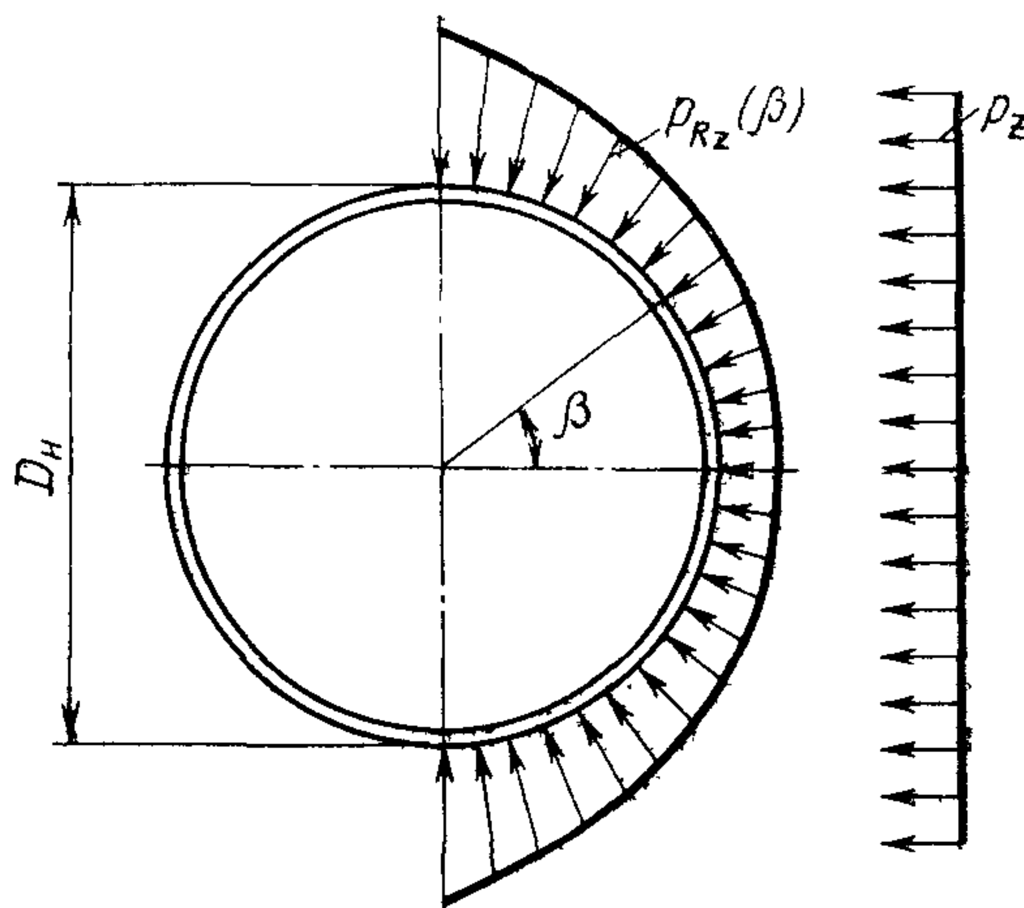
Рис. 6. Расчетная схема для определения волнового давления
