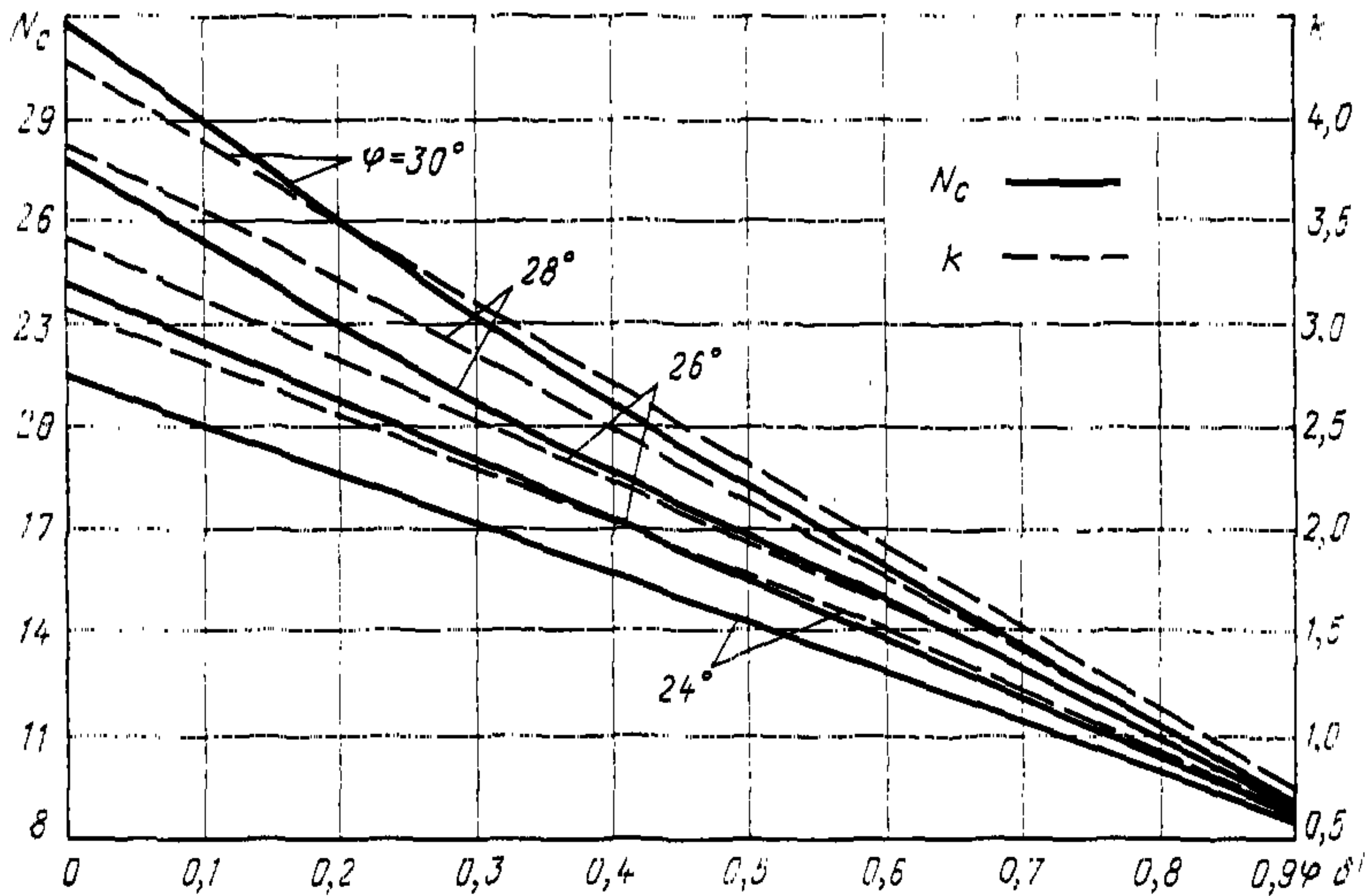
Рис. 17. График для определения безразмерных коэффициентов несущей способности N_c в зависимости от угла внутреннего трения \varphi и угла наклона \delta' силы R_{пр.р}
