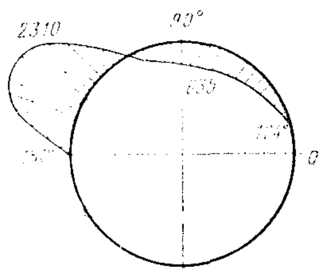
Рис. 25. Эпюра сдвигающих усилий в оболочке S, кН/м
