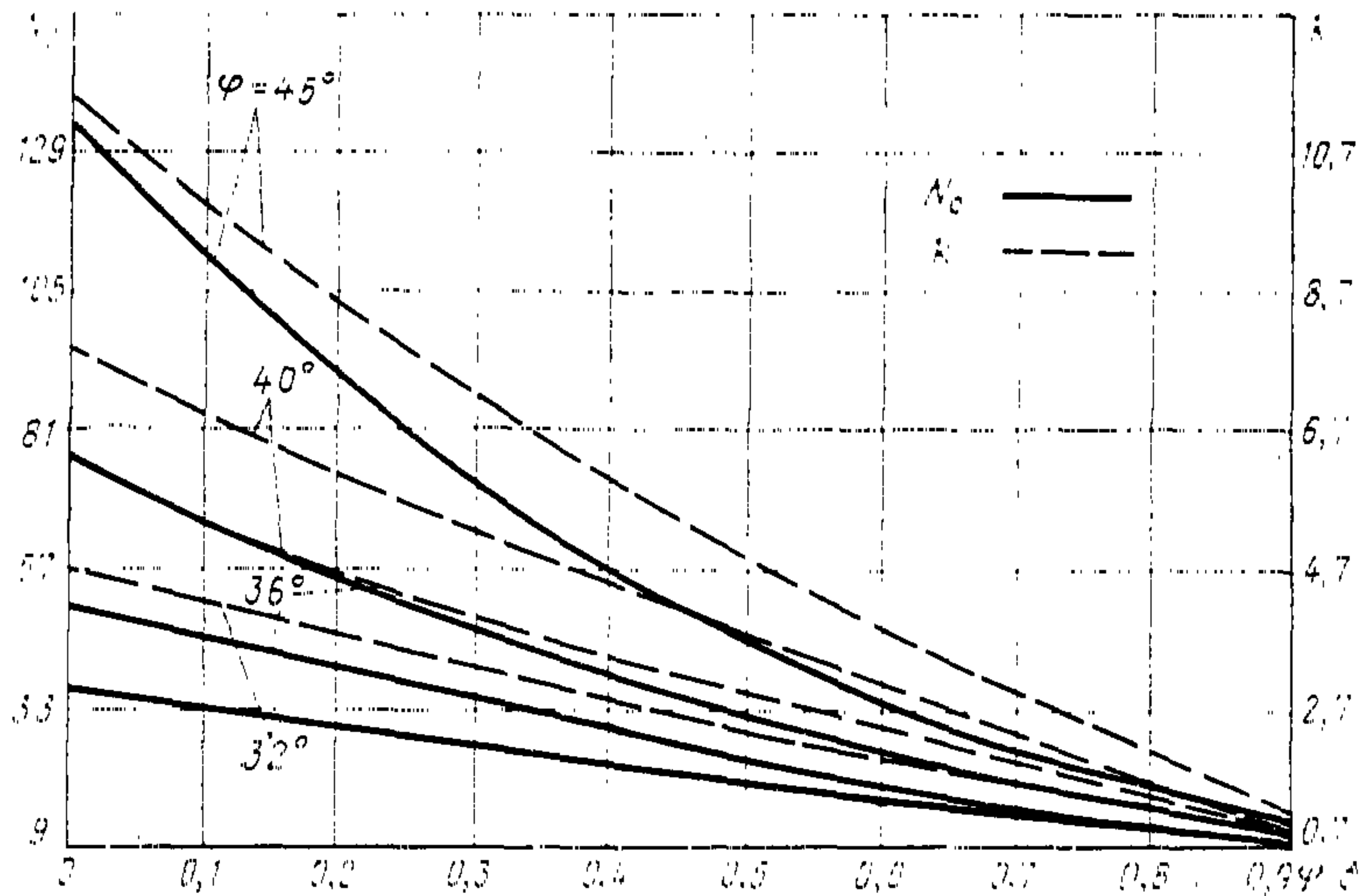
Рис. 19. График для определения безразмерных коэффициентов несущей способности N_c и k в зависимости от угла внутреннего трения \varphi и угла наклона \delta' силы R_{пр.р}
