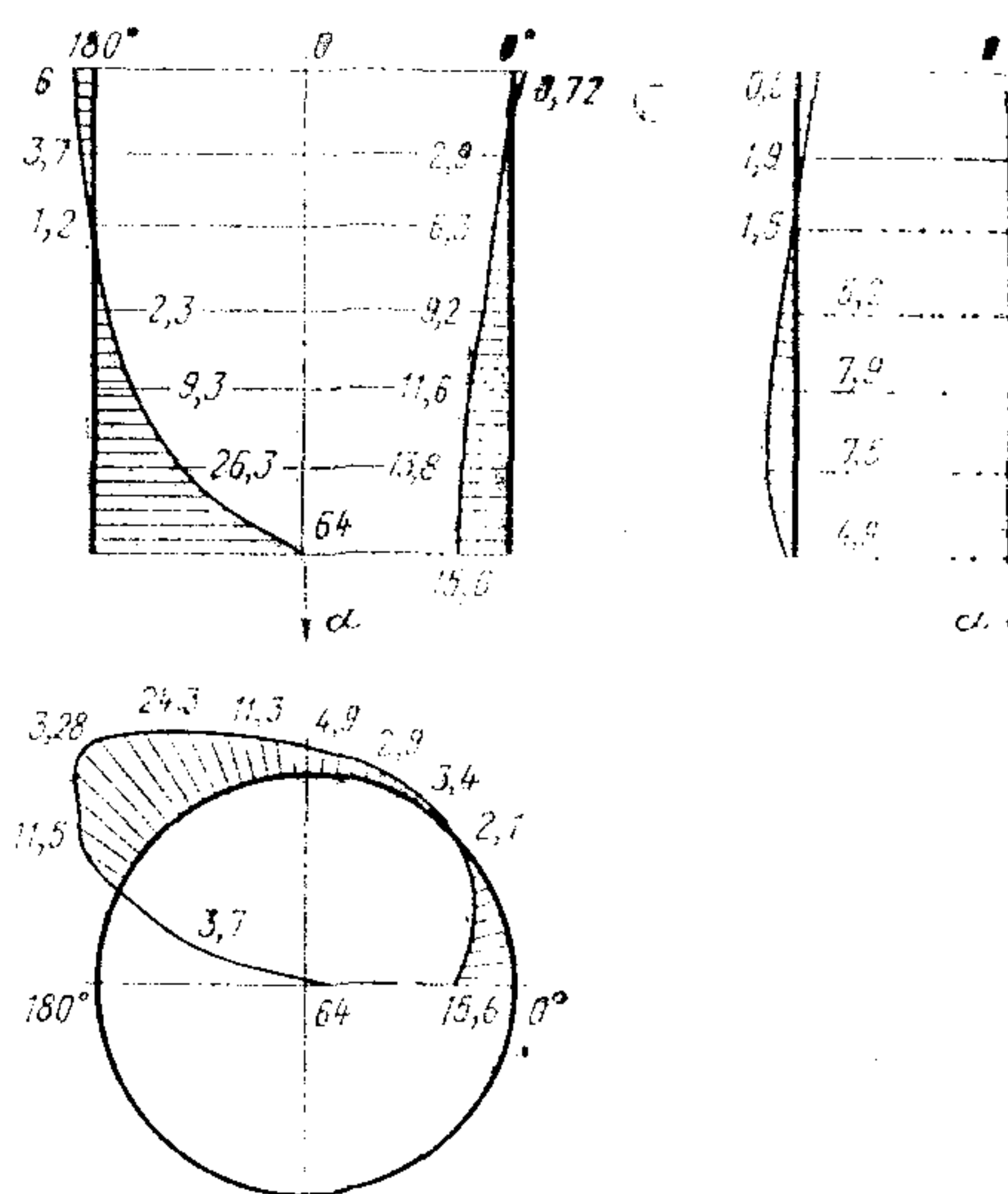
Рис. 23. Эпюра поперечных изгибающих моментов в оболочке M_\beta , кН·м
