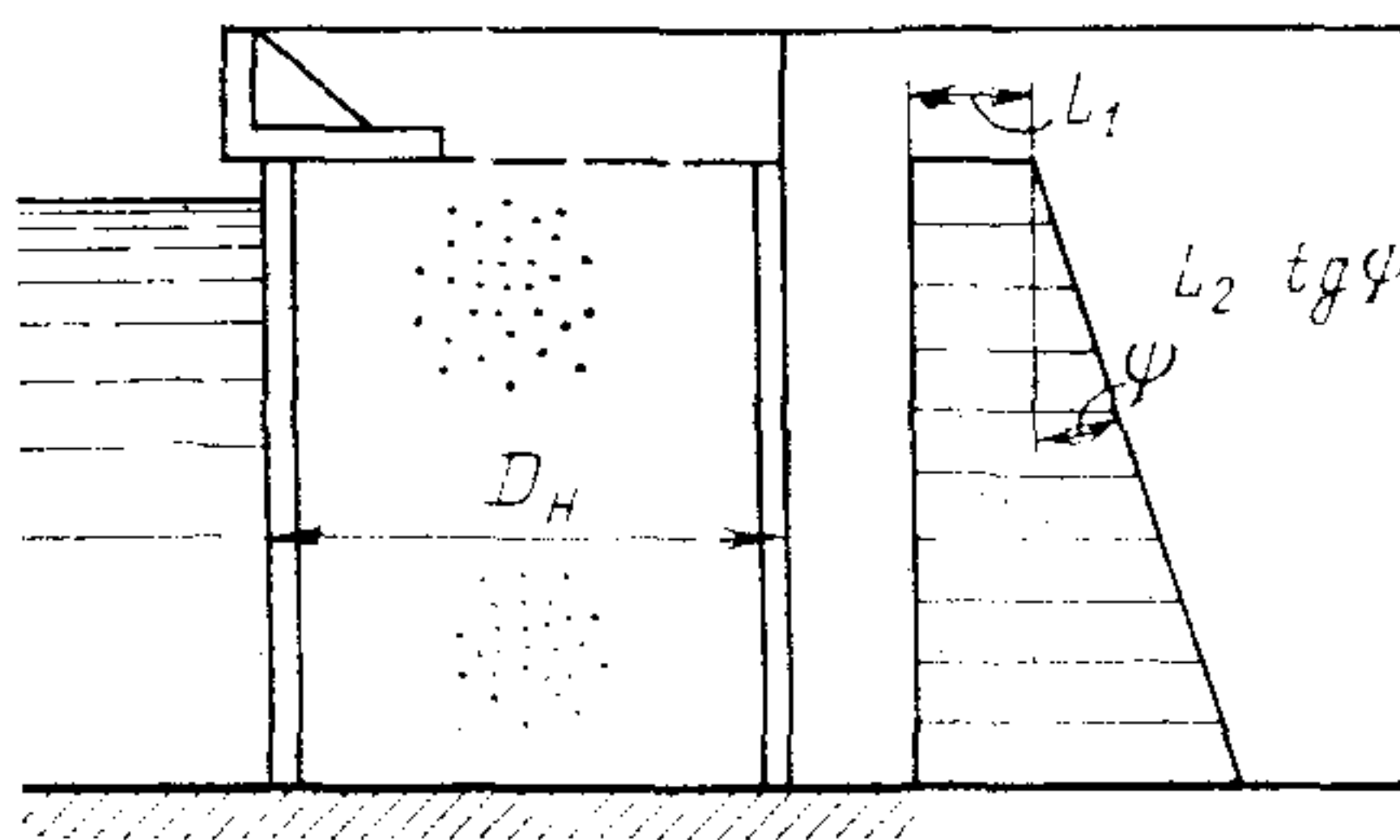
Рис. 7. Схема для определения параметров бокового давления
