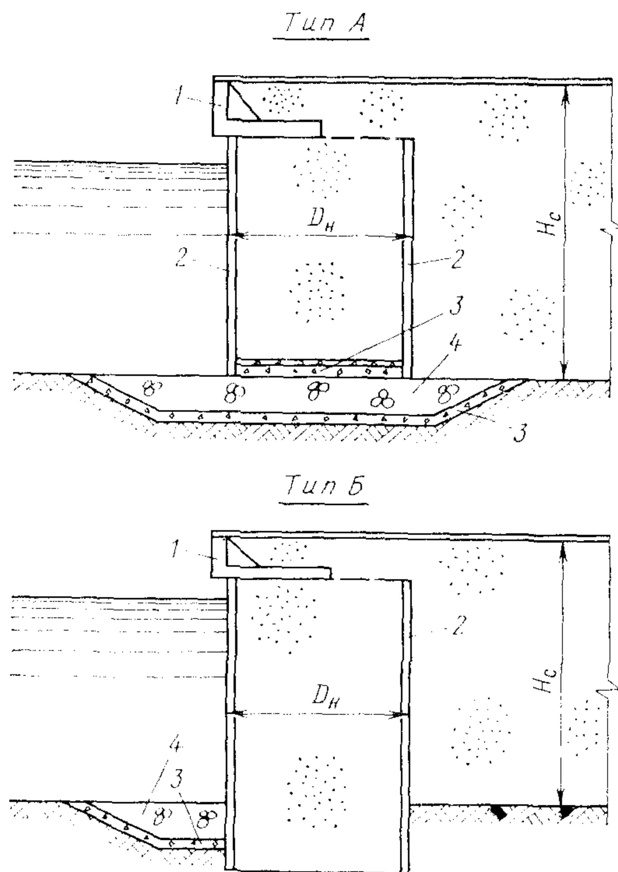
Рис. 1. Причальные сооружения из оболочек большого диаметра: 1 — верхнее строение; 2 — оболочка; 3 — контрфильтр; 4 — каменная постель
