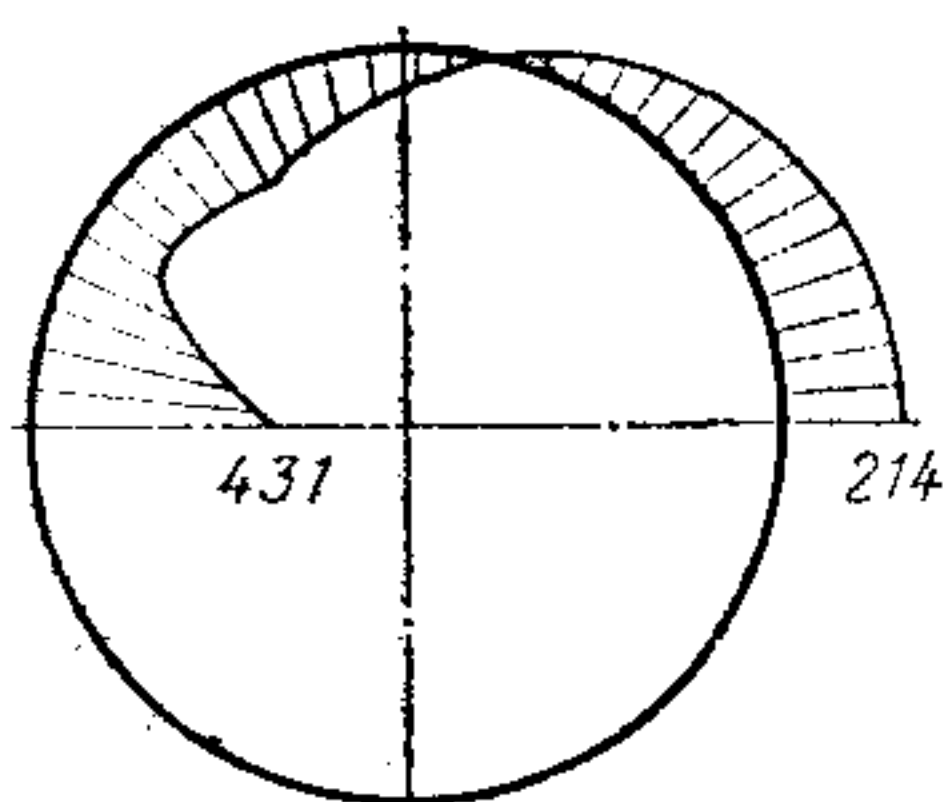
Рис. 24. Эпюра поперечных нормальных усилий в оболочке Т, кН/м
