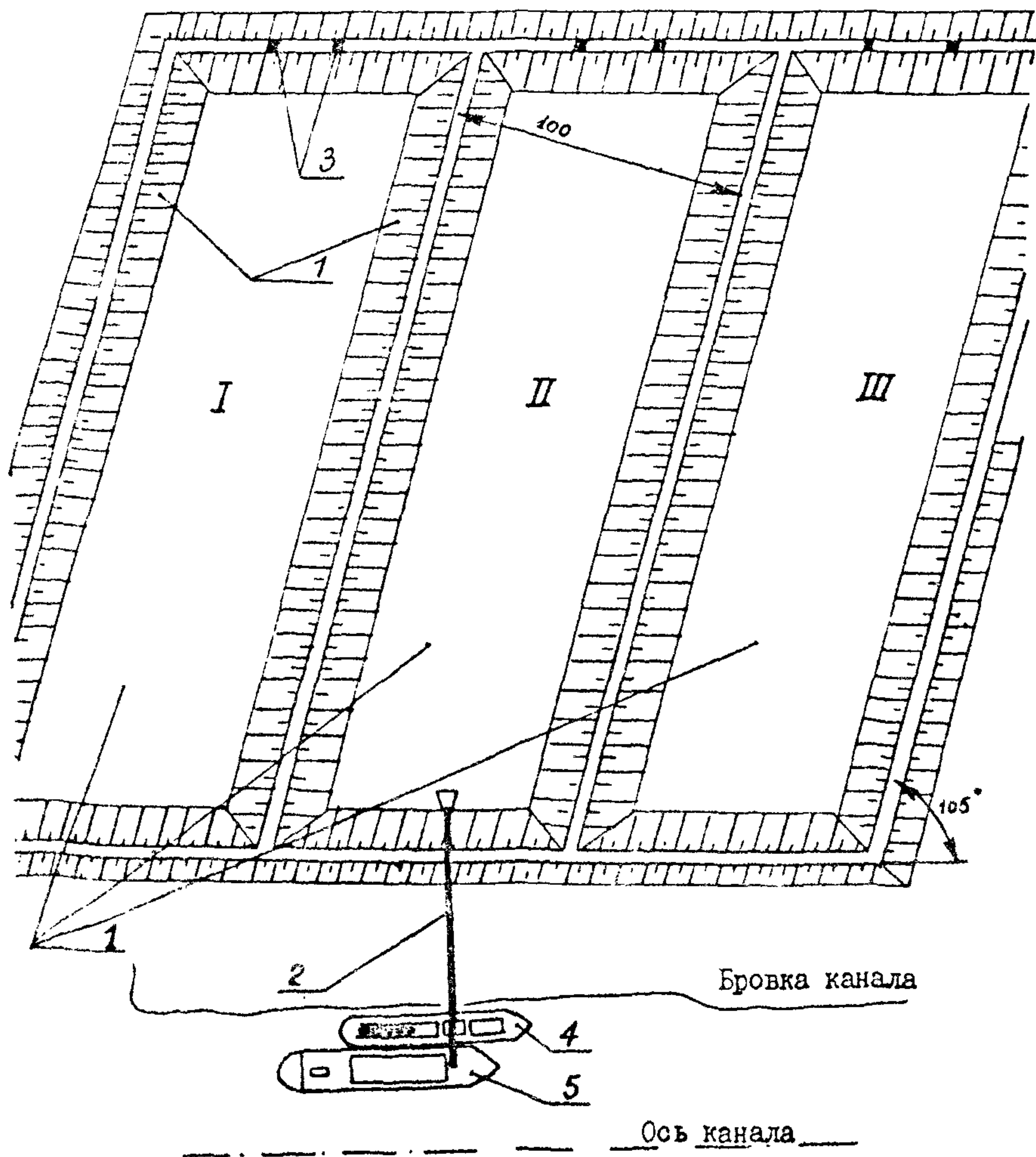
Рис. 3. Схема берегового отвала в порту Херсон: I–III – карты намыва; 1 – дамбы обвалования; 2 – пульпопровод; 3 – водосбросы; 4 – станция рефулирования; 5 – самоотвозный землесос
