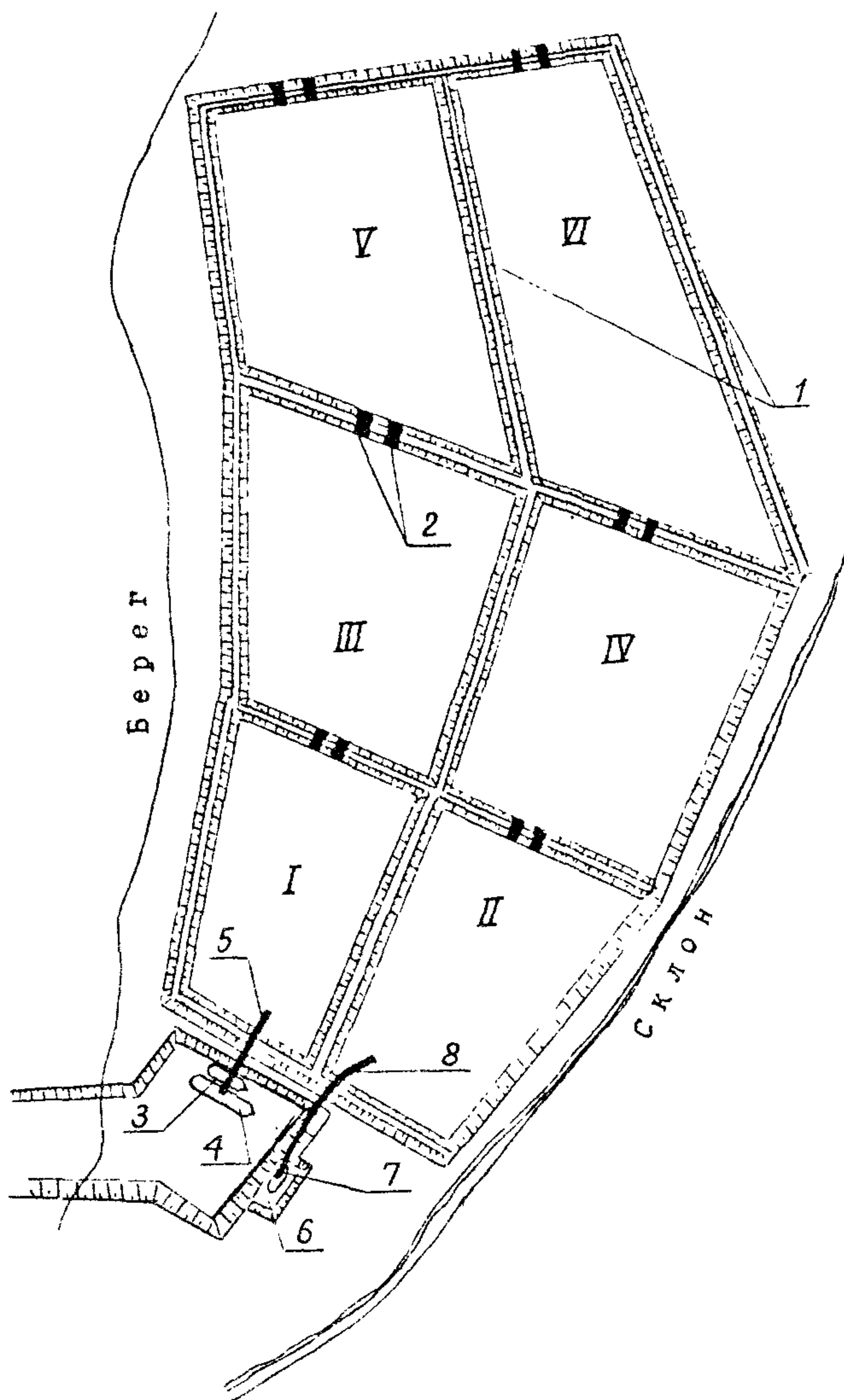
Рис. 4. Схема берегового отвала в порту Керчь: 1—УД — карты намыва; 1 — дамбы обвалования; 2 — водосбросы; 3 — плавучий причал; 4 — самоотвозный землесос; 5 — береговой пульпопровод; 6 — депозит; 7 — шаландоперегрузатель; 8 — плавучий пульпопровод
