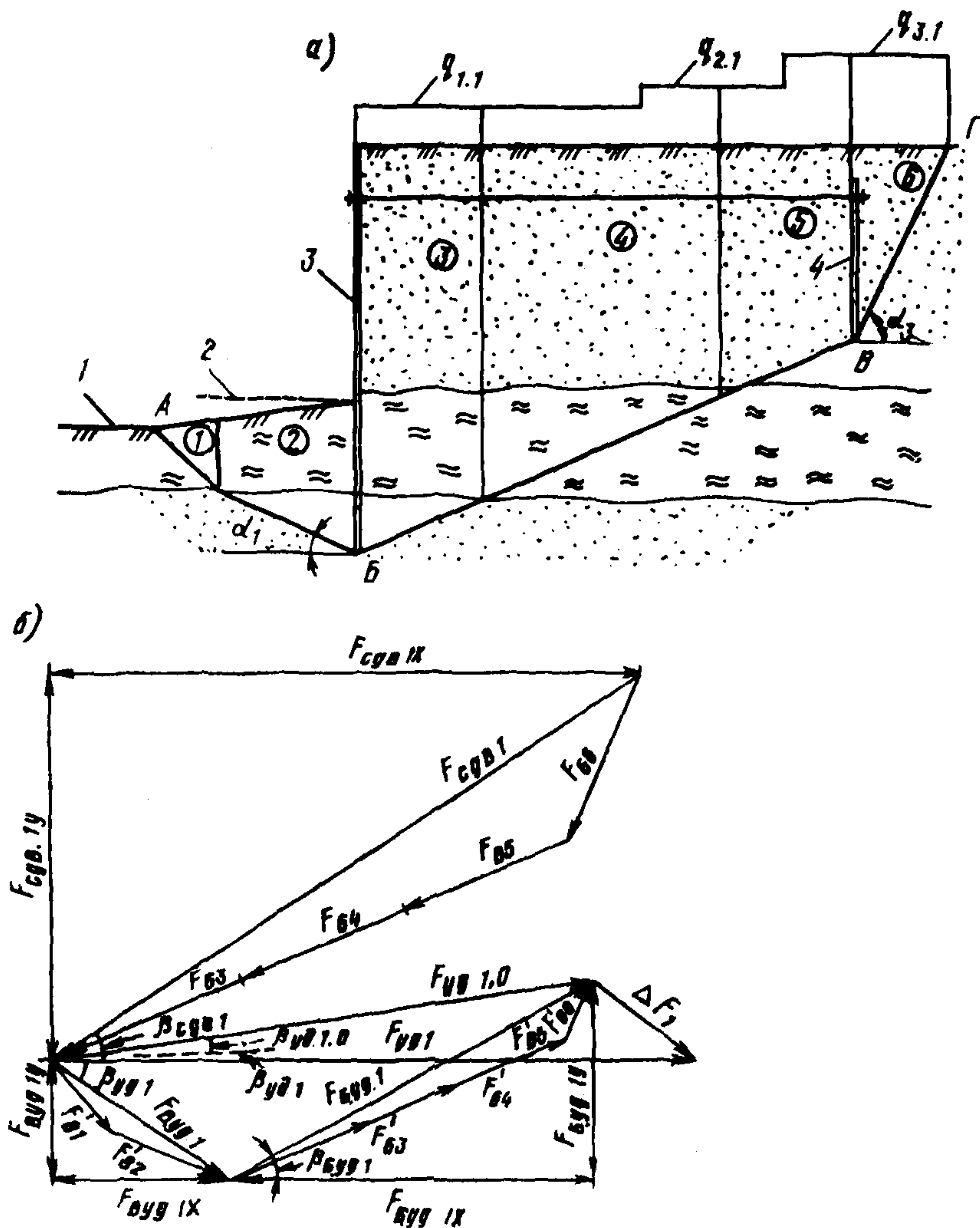
Рис. 2. Схема к определению равнодействующих сдвигающих и удерживающих сил:
