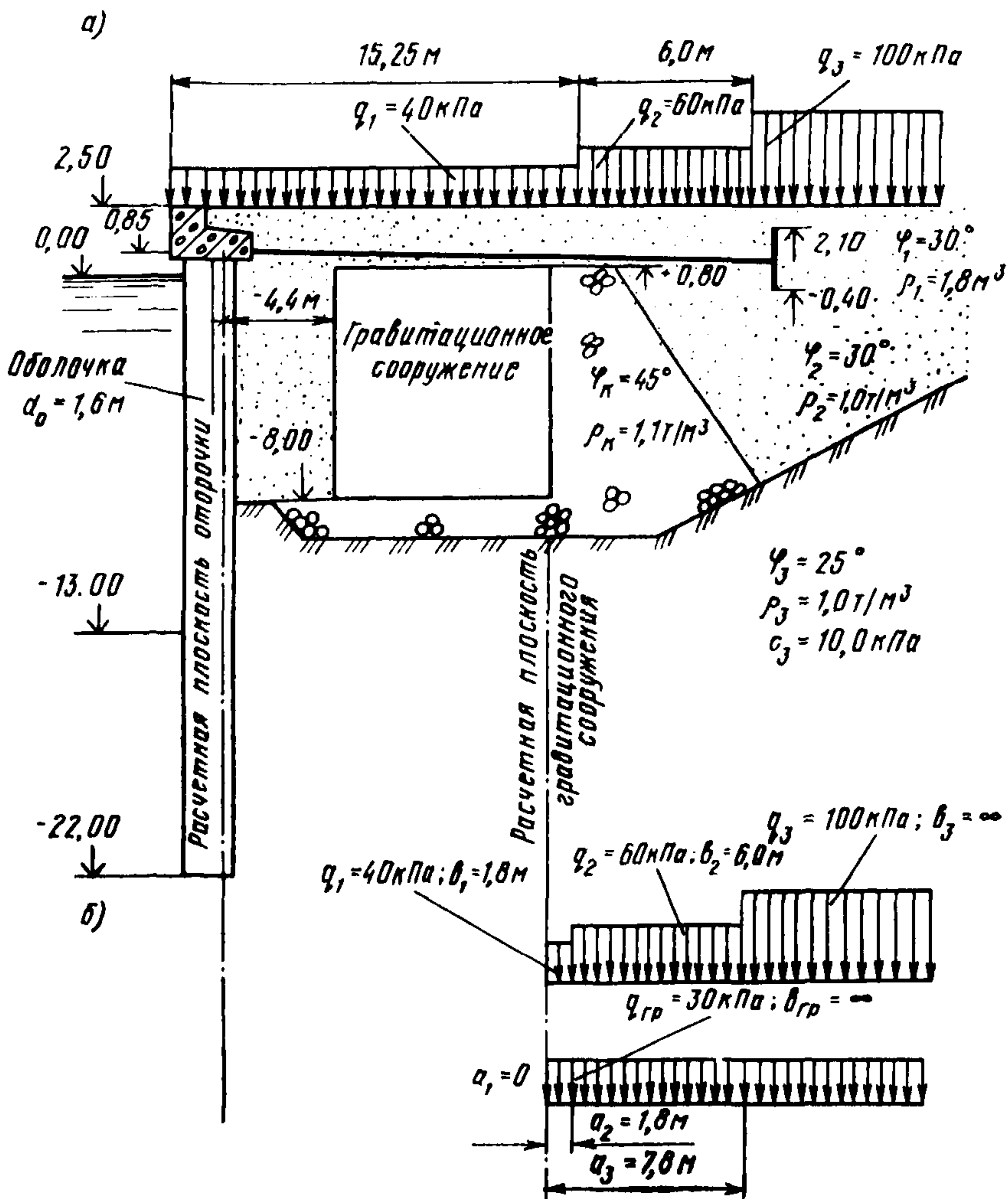
Рис. 4. Схема сооружения:
