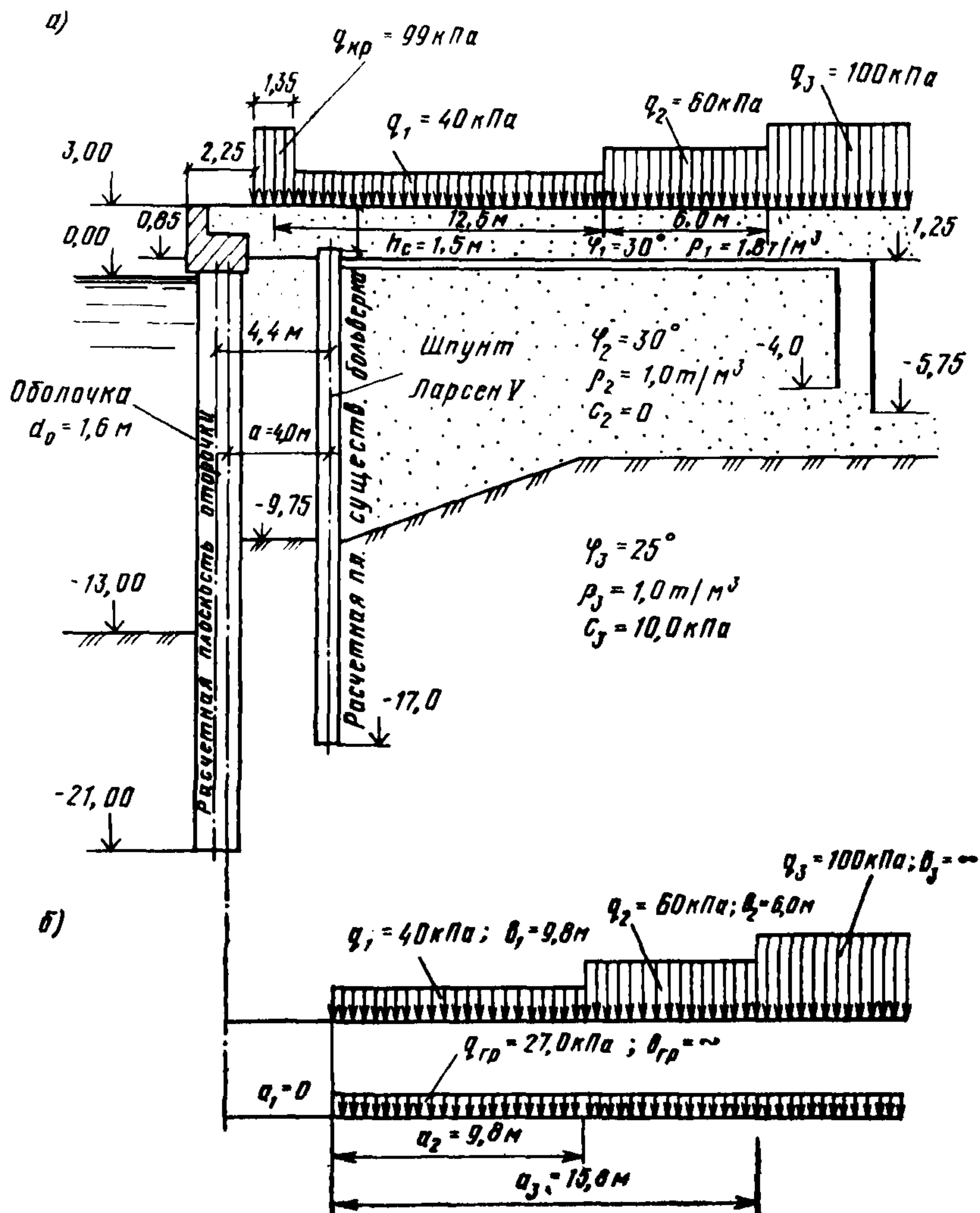
Рис. 3. Схема сооружения: а — конструктивная схема; б — схема расположения вертикальных нагрузок за расчетной плоскостью существующего бойверка
