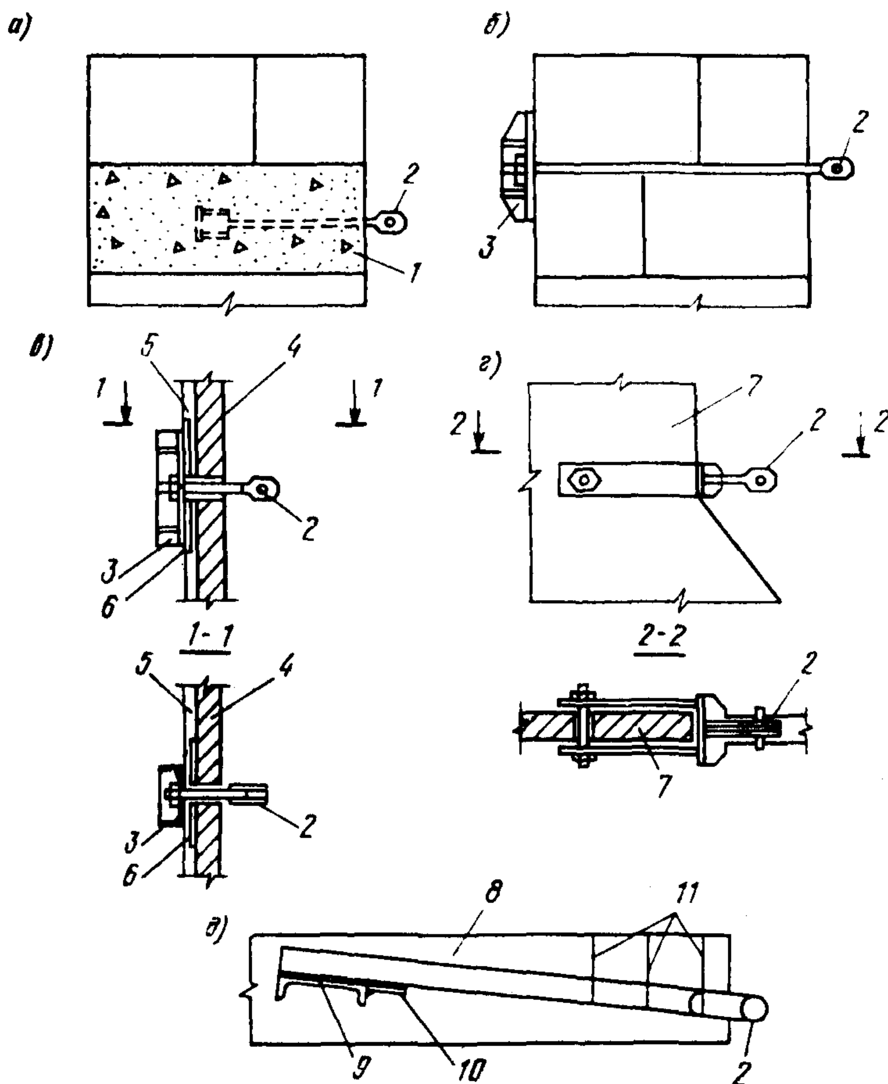
Рис. 4.1. Схемы крепления анкерных тяг к гравитационному сооружению:
