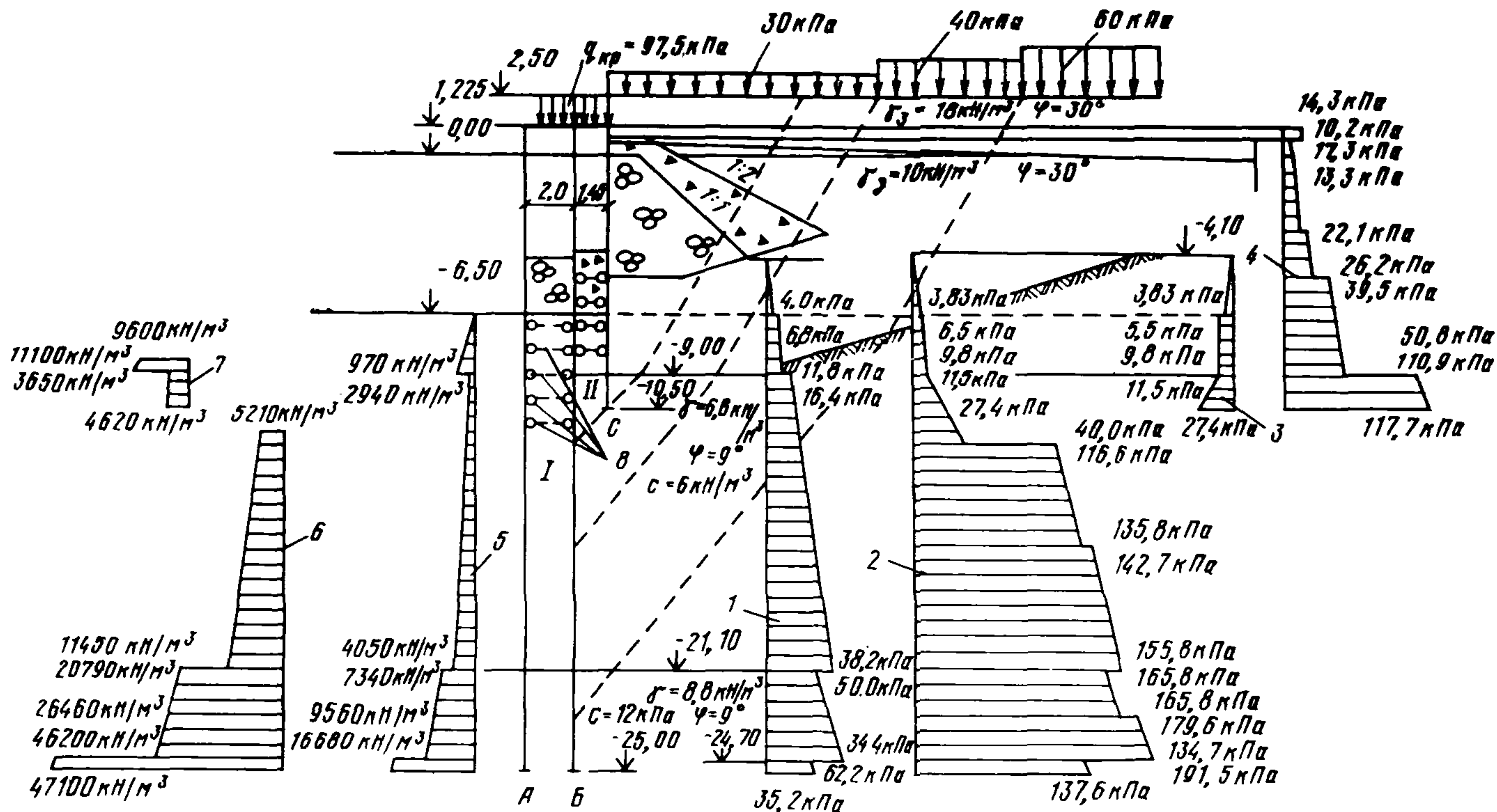
Рис. 2. Расчетная схема:
