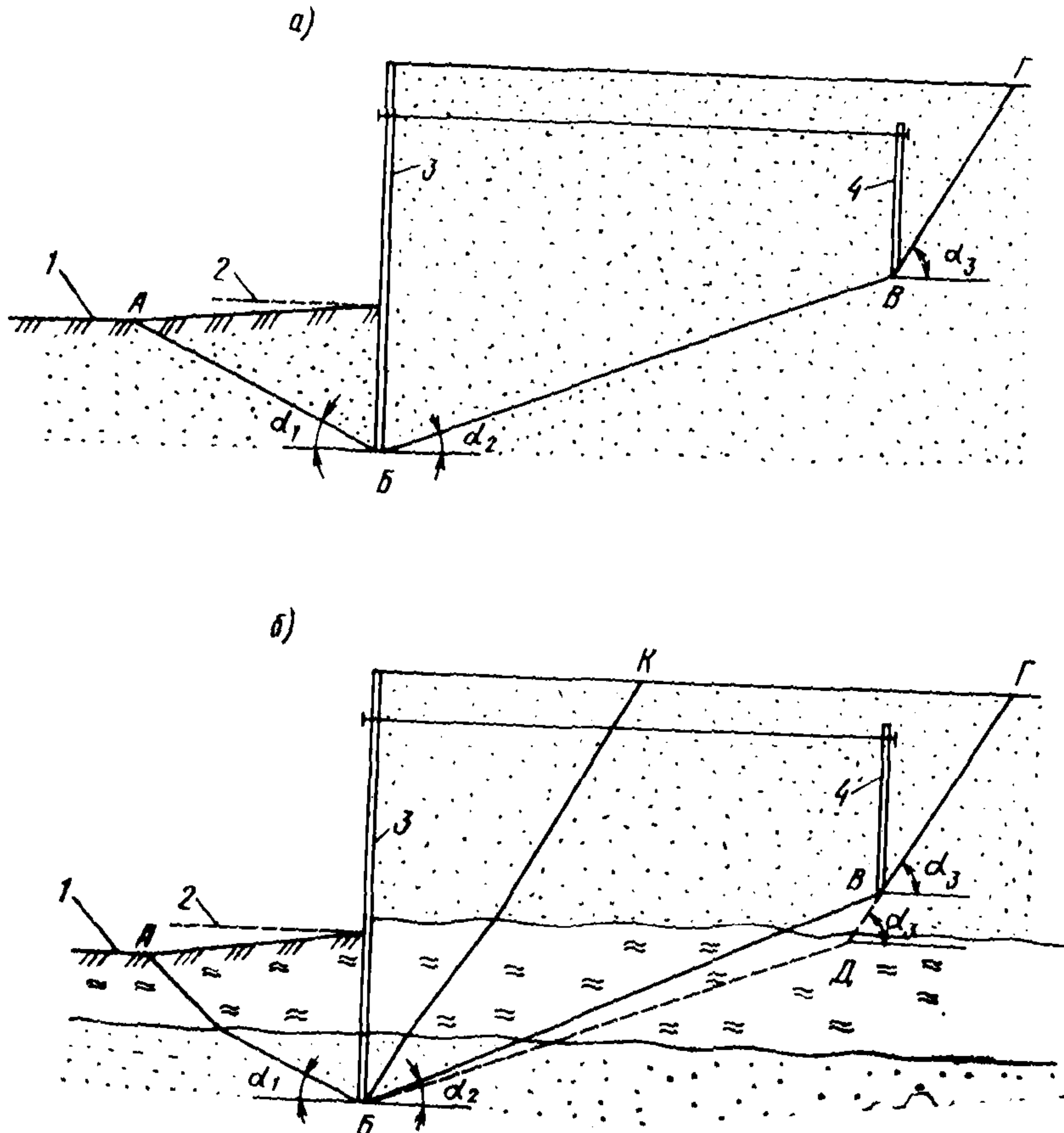
Рис. 1. Схемы расположения поверхности скольжения грунта основания:
