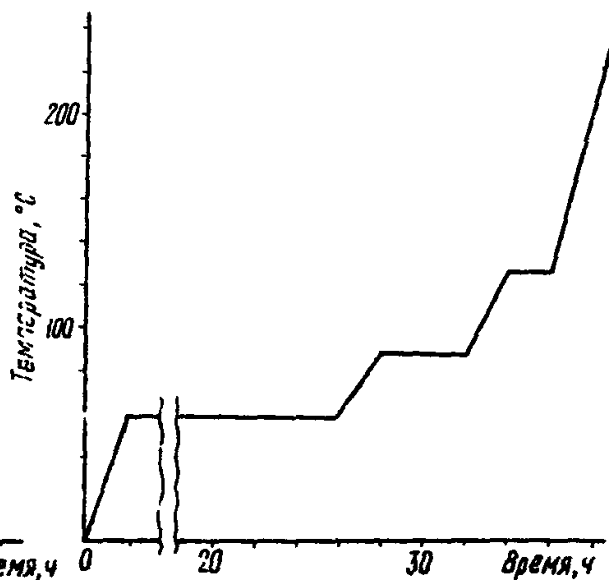
Рис.7. График сушки массы на алюмохромофосфатной связке (ХФ ЦБ Союзэнергоремонта)
