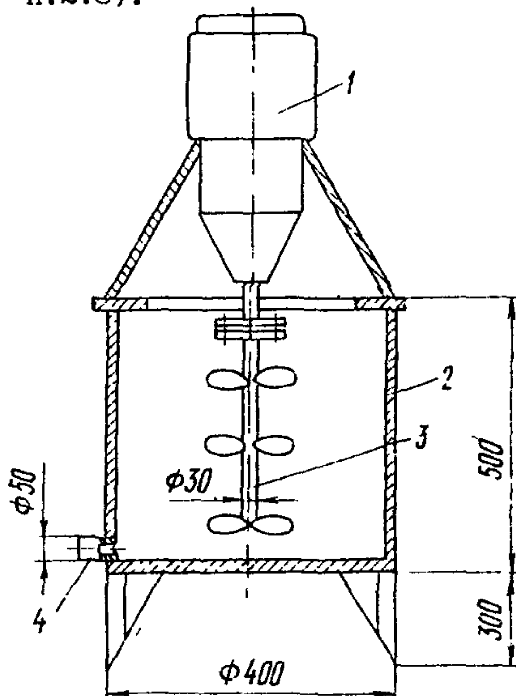
Рис.1. Смеситель для приготовления связки:
