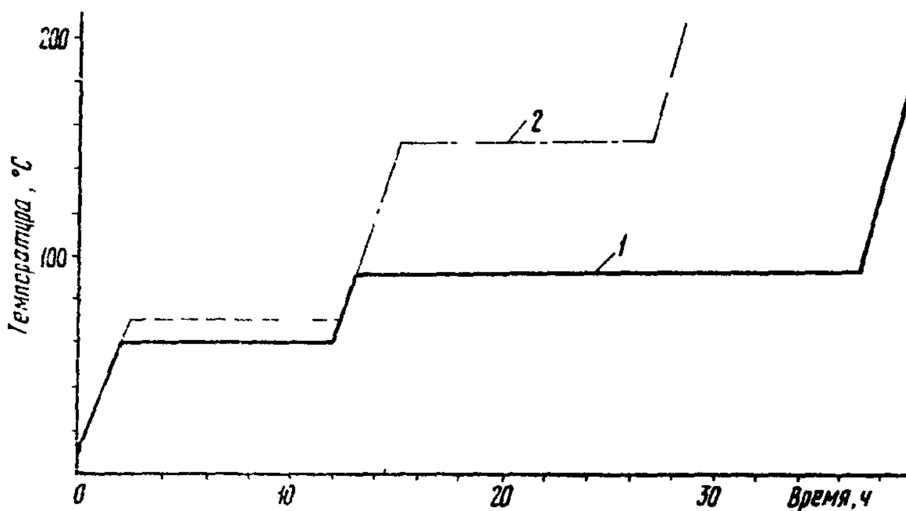
Рис.5. График сушки массы на ортофосфорной кислоте (ГО "Союзтехэнерго")
