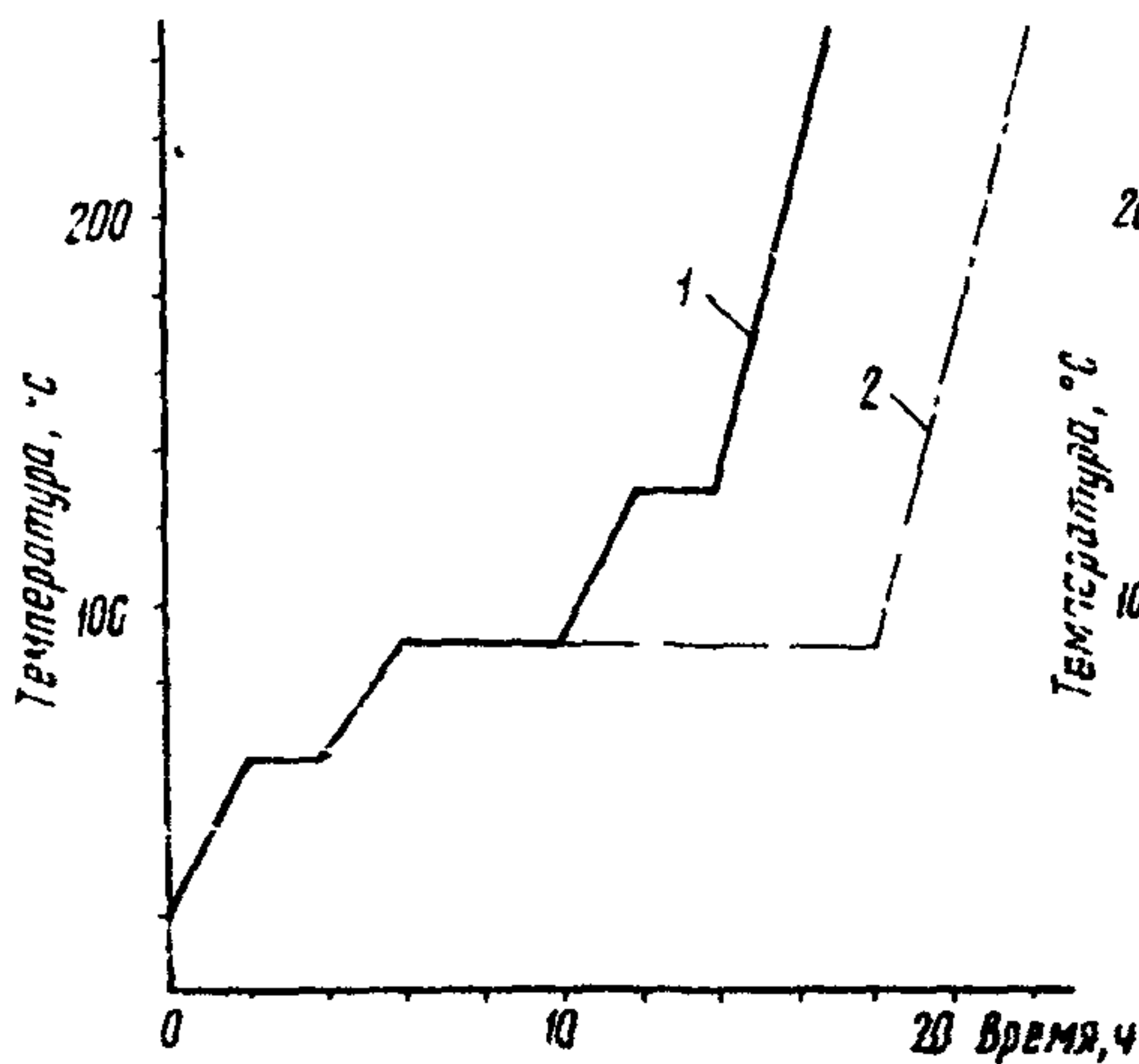
Рис.6. График сушки массы на кальций(бор)алюмофосфатной связке (УралВТИ)
