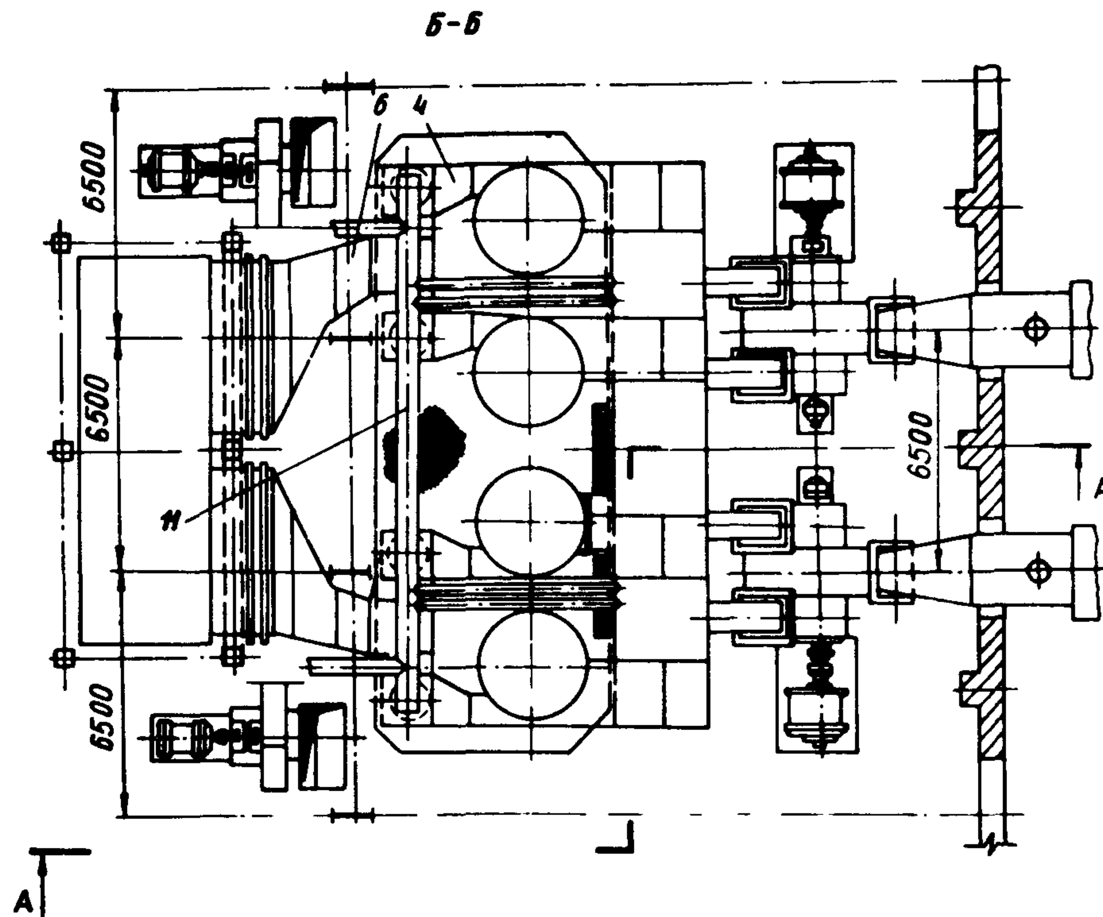
Рис.1. Компонировка МЗУ типа МВ-ИРО за котлоагрегатом паропроизводительностью 230 т/ч: 1 - труба Вентури; 2 - центробежный скруббер; 3 - колено; 4 - переход; 5 - патрубок входной; 6 - подводящие газоходы; 7 - отводящие газоходы; 8 - сборный короб; 9 - дымосос; 10 - форсунка; 11 - воздухопроводы СП; Г.В. - горячий воздух; Д.Г. - дымовые газы
