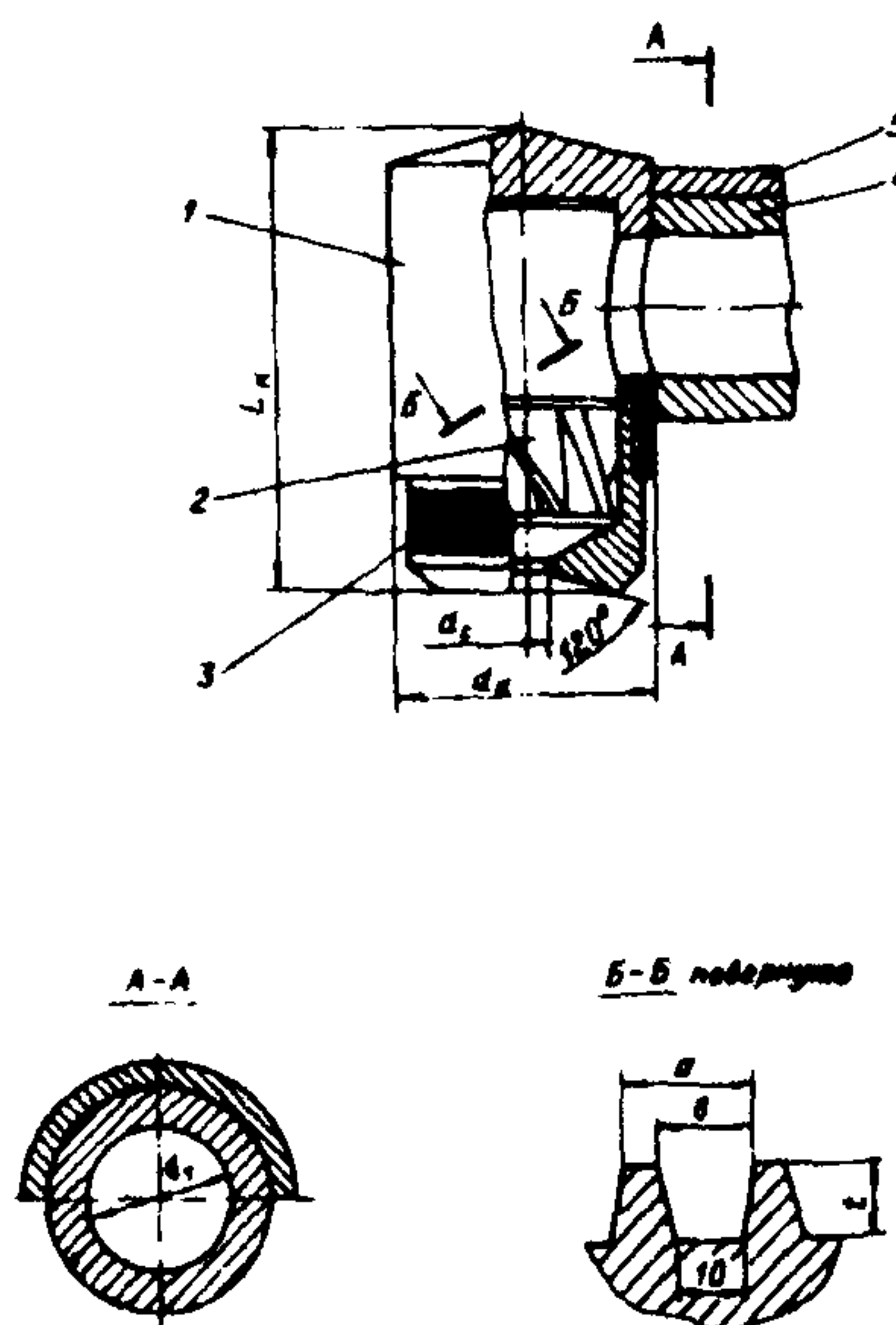
Рис.3. Центробежная механическая форсунка:
