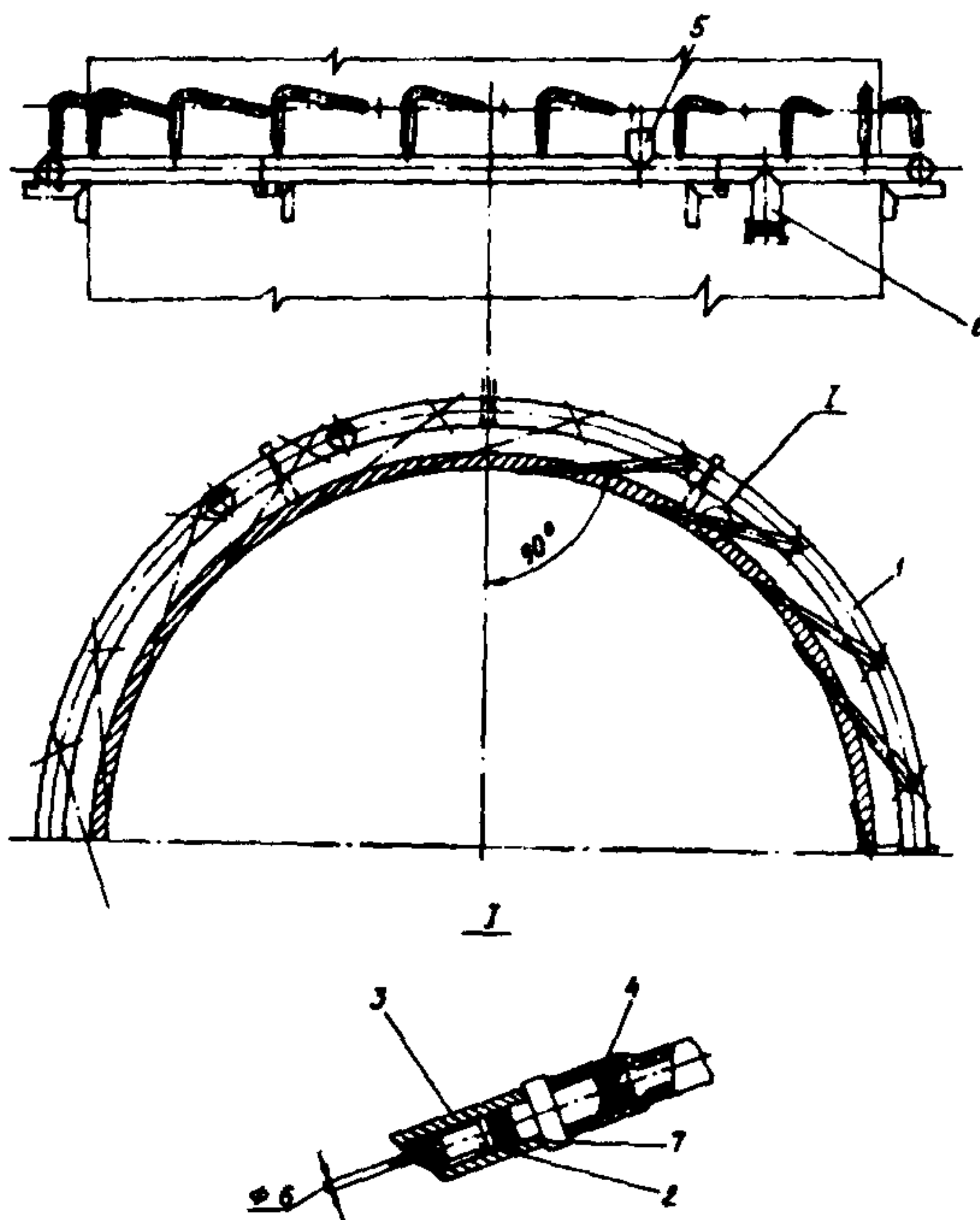
Рис.5. Система орошения ЦС:
