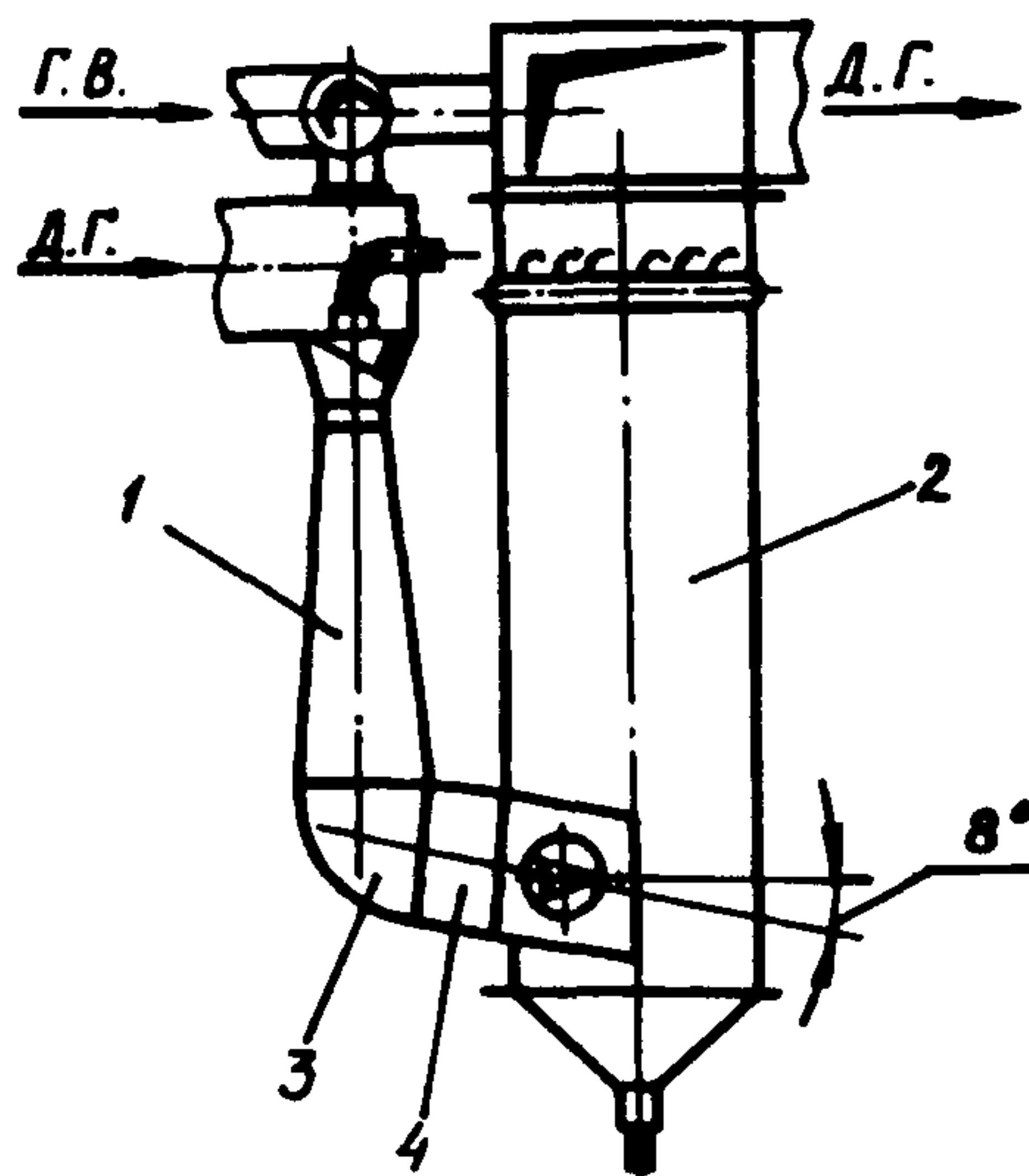
Рис.2. Золоуловитель МВ-ИРО:
