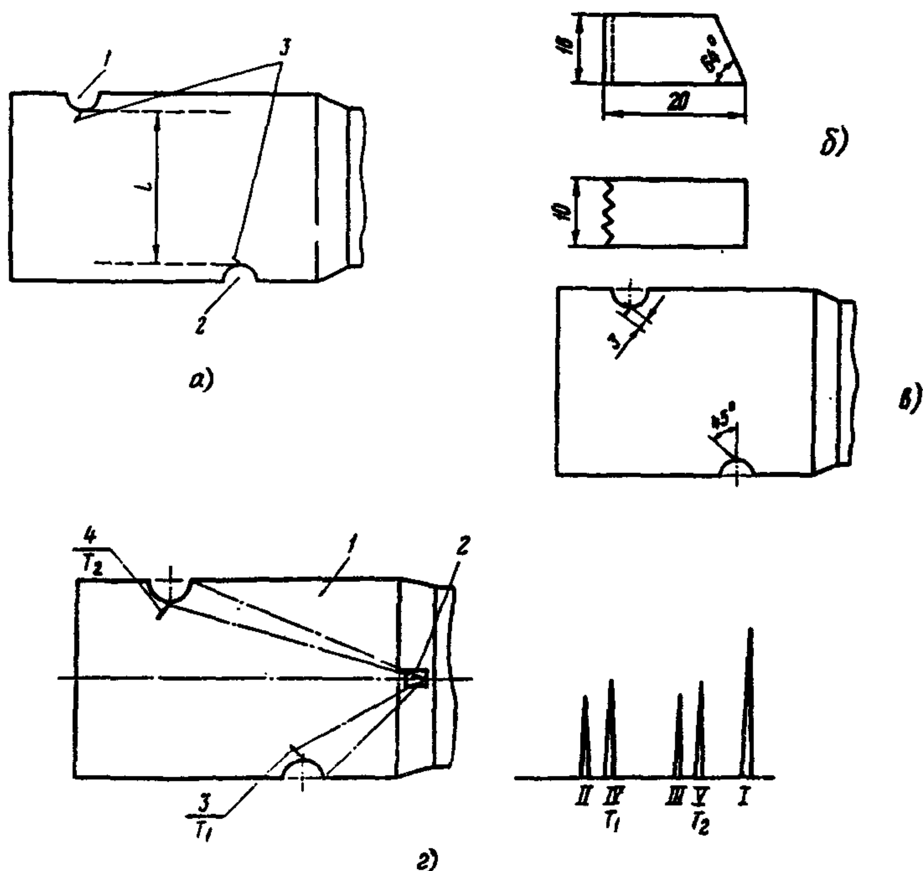
Рис. П.4. Ультразвуковая дефектоскопия вильчатого хвостовика лопаток:
