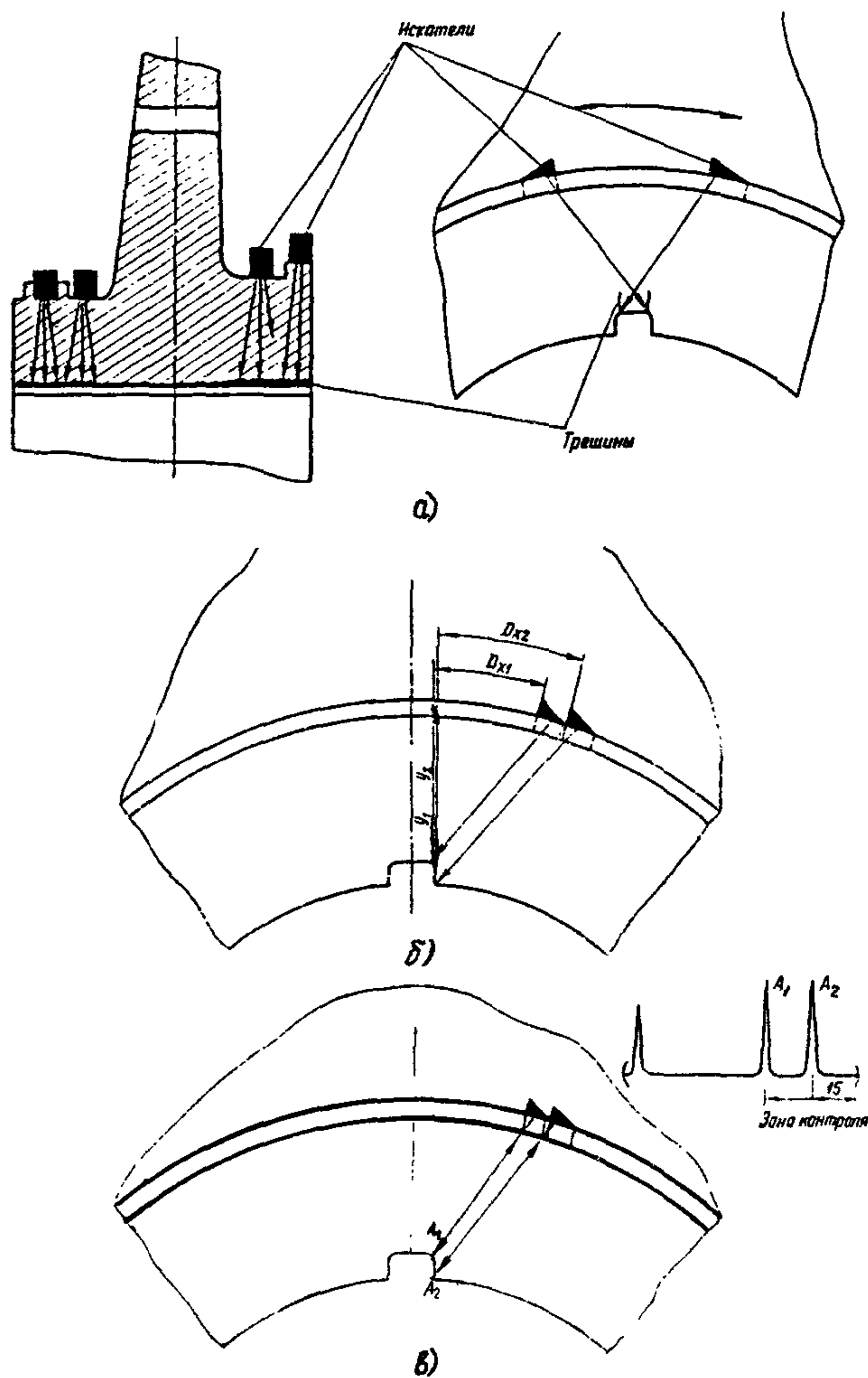
Рис. П.2.3. Дефектоскопия диска:
