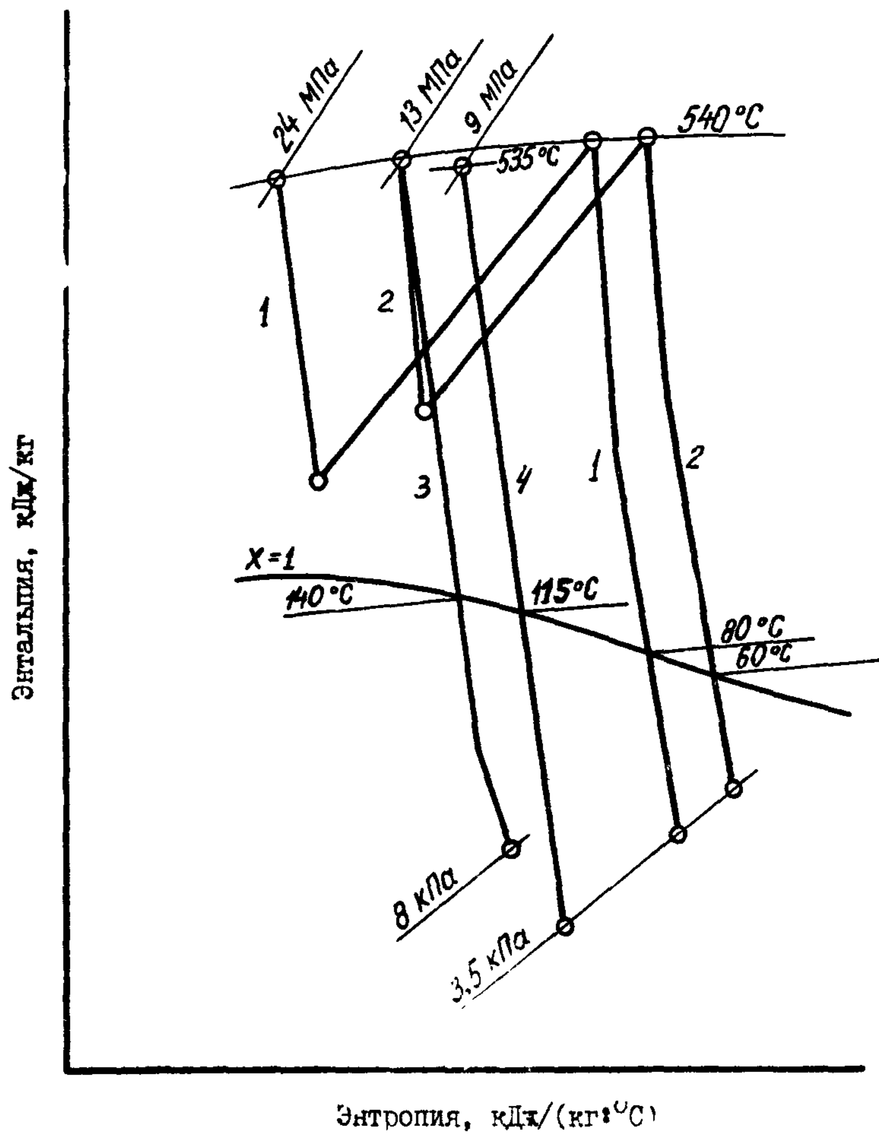
Рис. 4. Процессы расширения пара в турбинах
