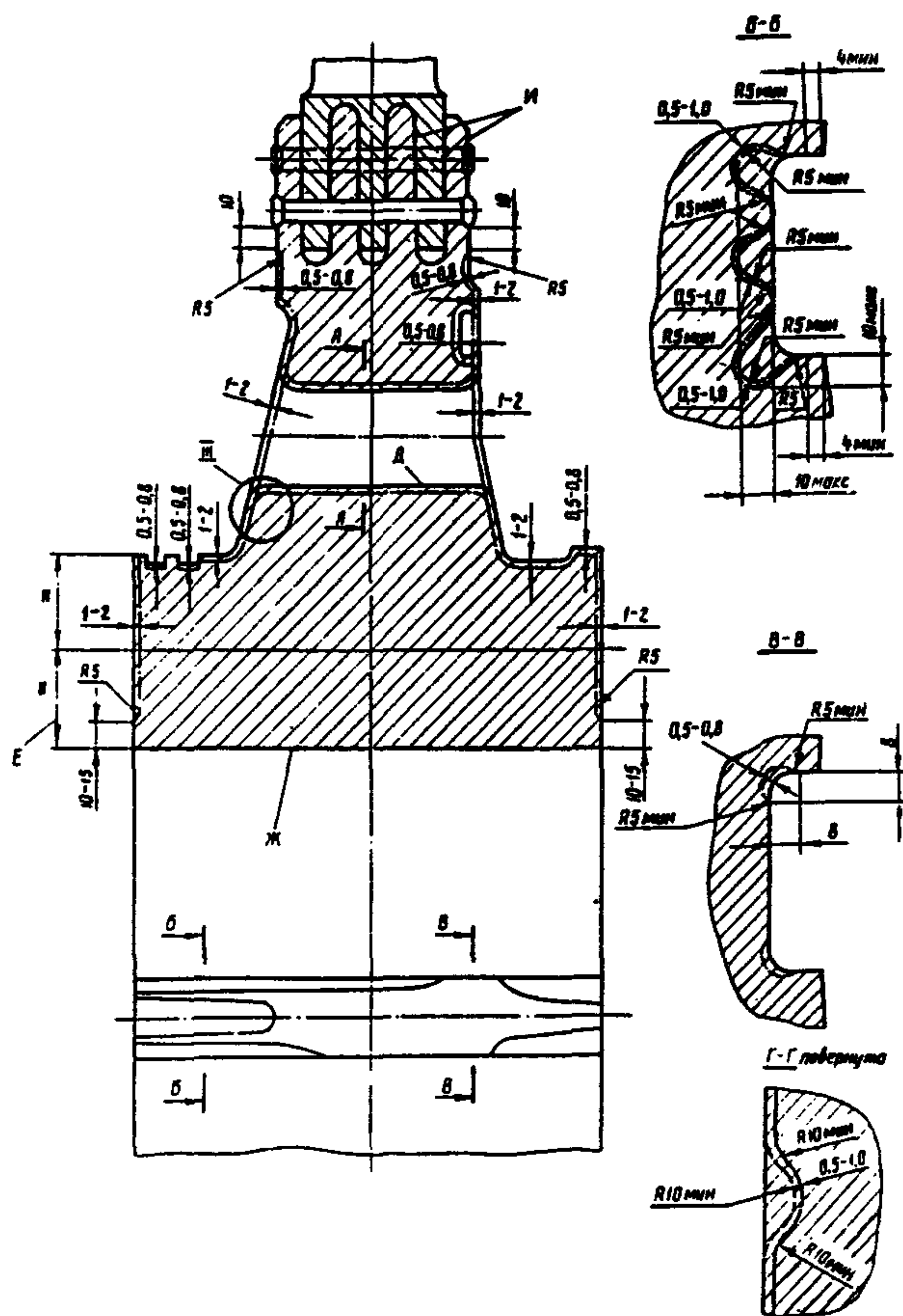
Рис. П.1.1. Диск турбины
