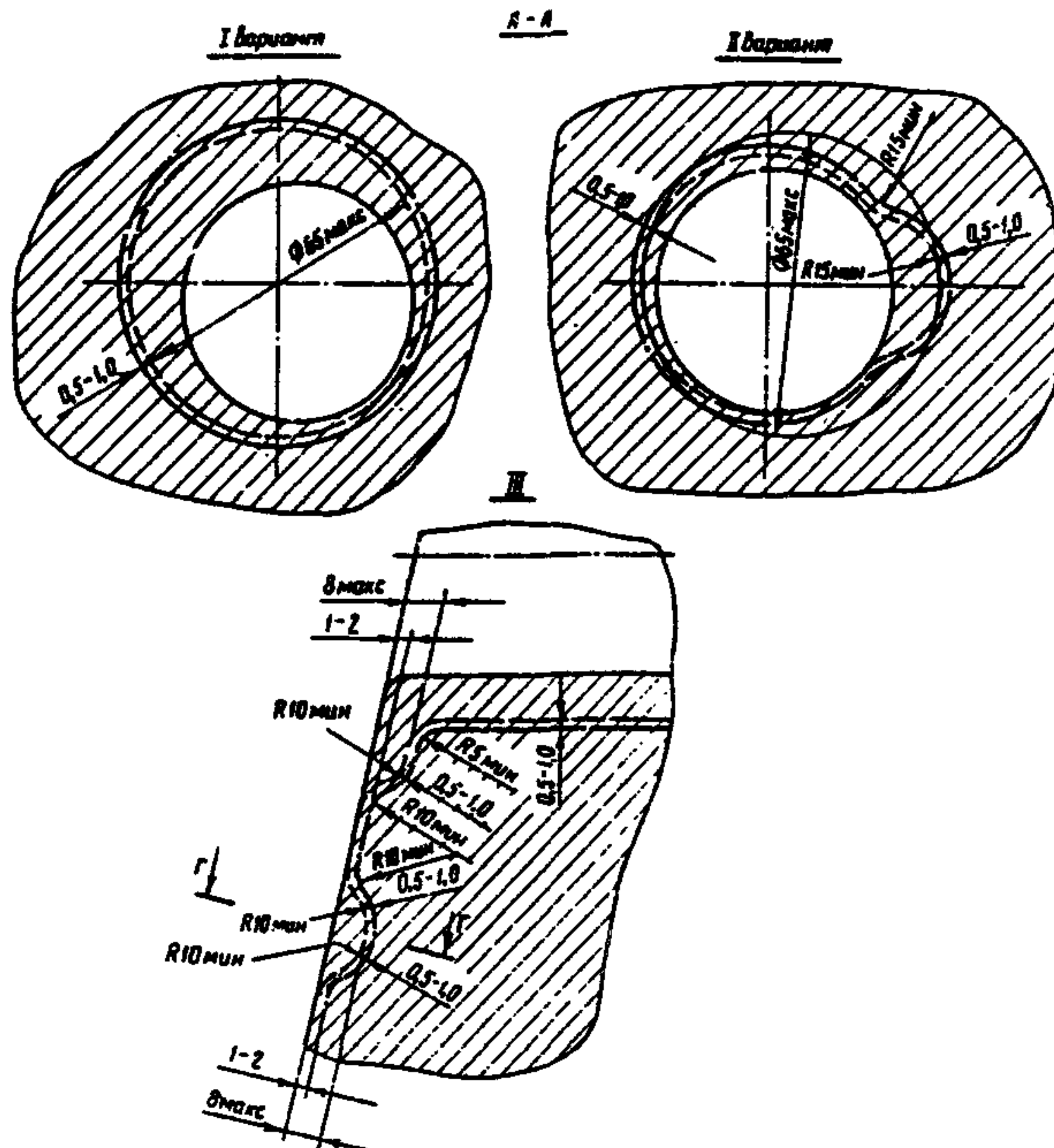
Рис. II.1.2. Обработка диска при ремонте 18-23-й ступеней турбины Т-100-130
