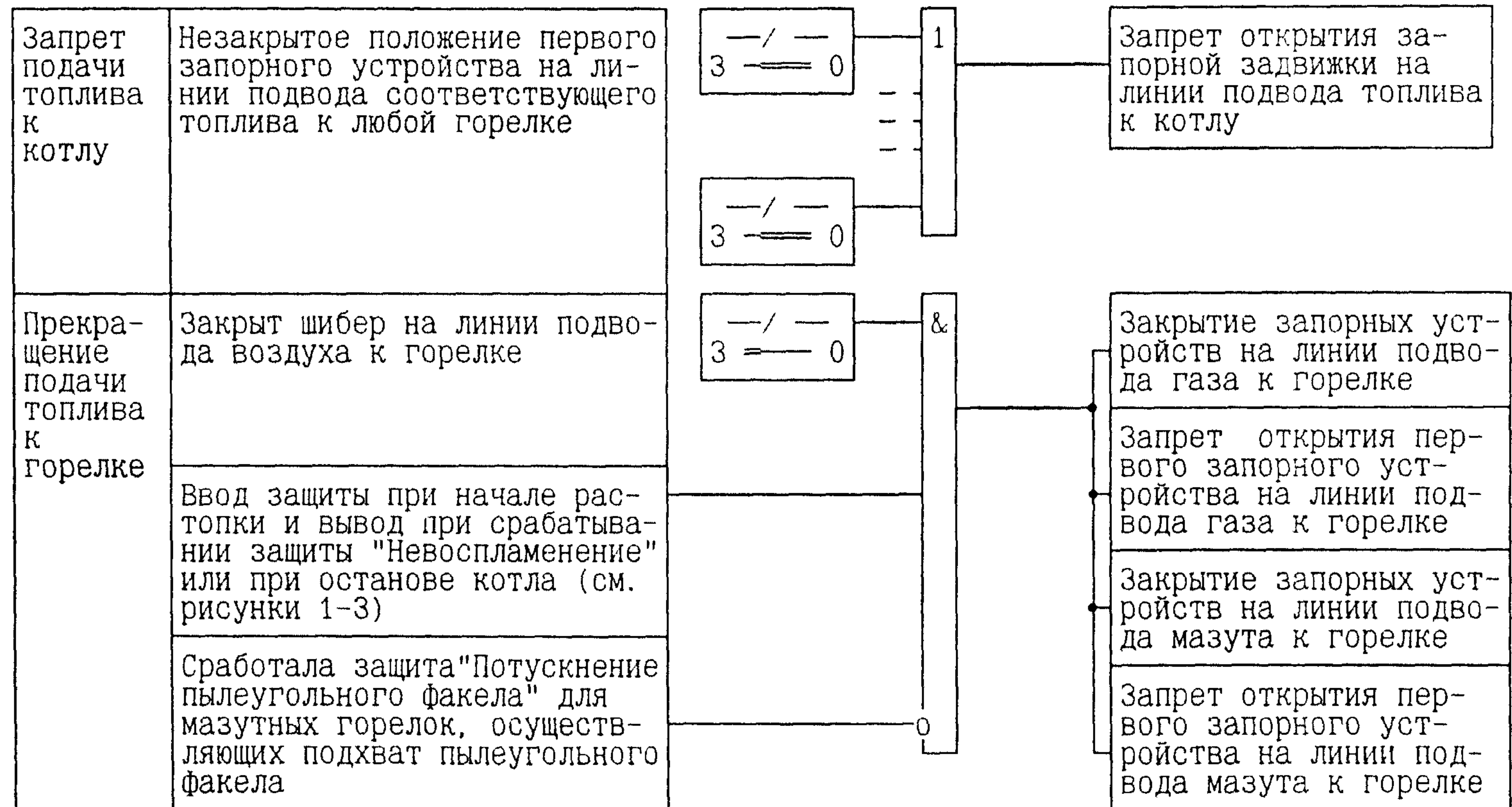
Рисунок 32 – Запрет подачи топлива к котлу. Запрет при закрытии воздушного шибер перед горелкой
