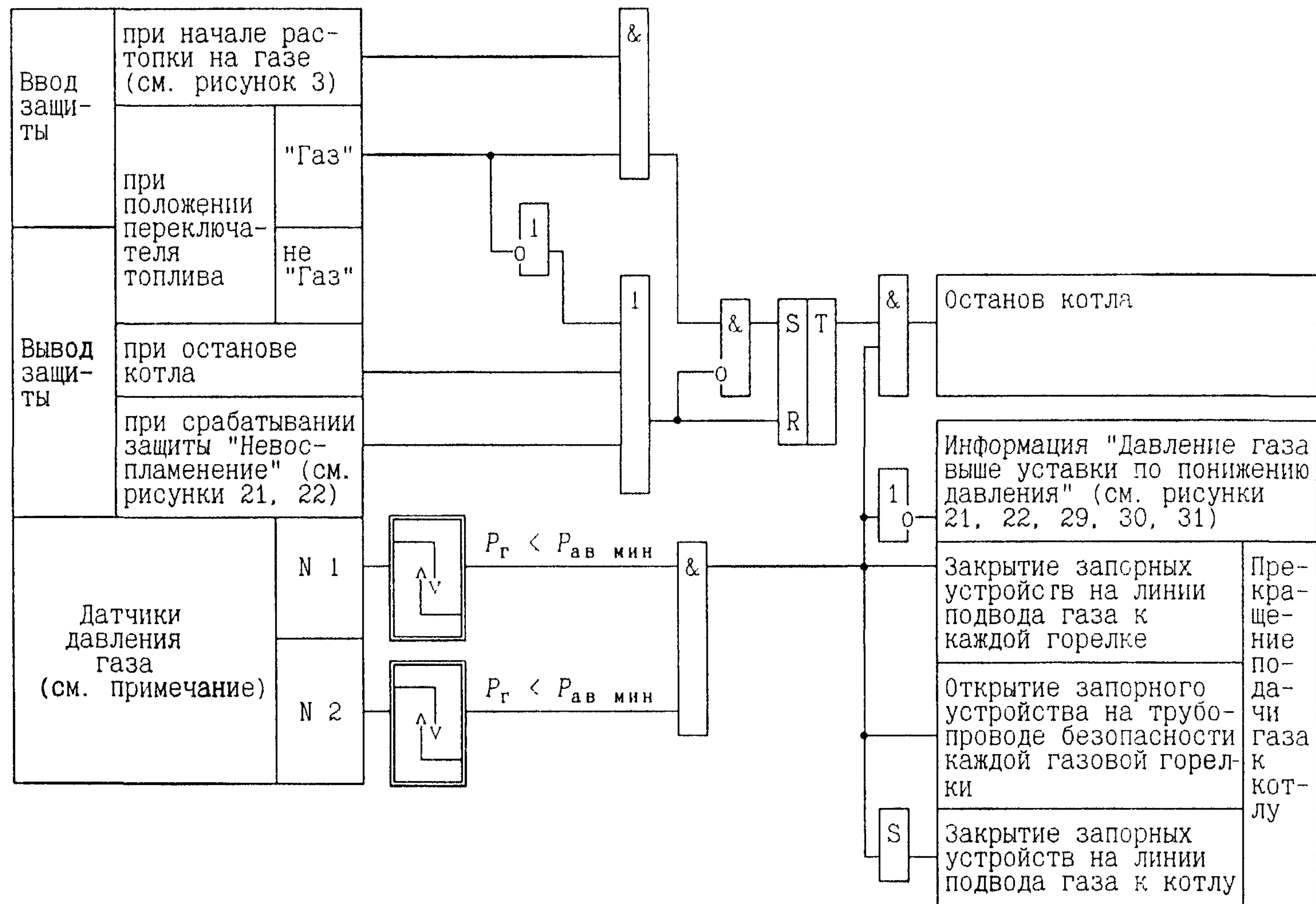
Рисунок 14 – Защита по понижению давления газа. Пылегазовый котел.
