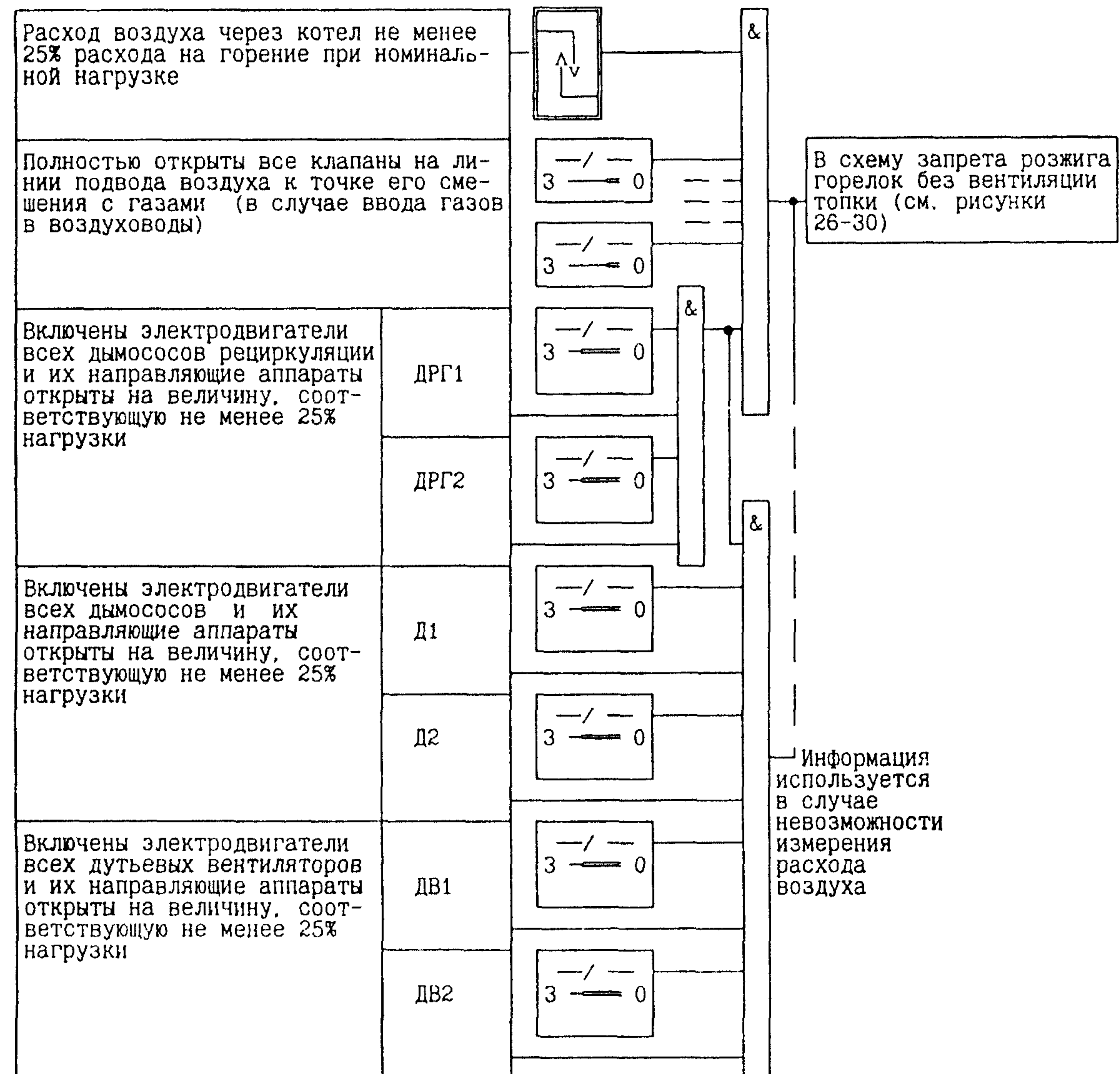
Рисунок 25 – Условия вентиляции топки
