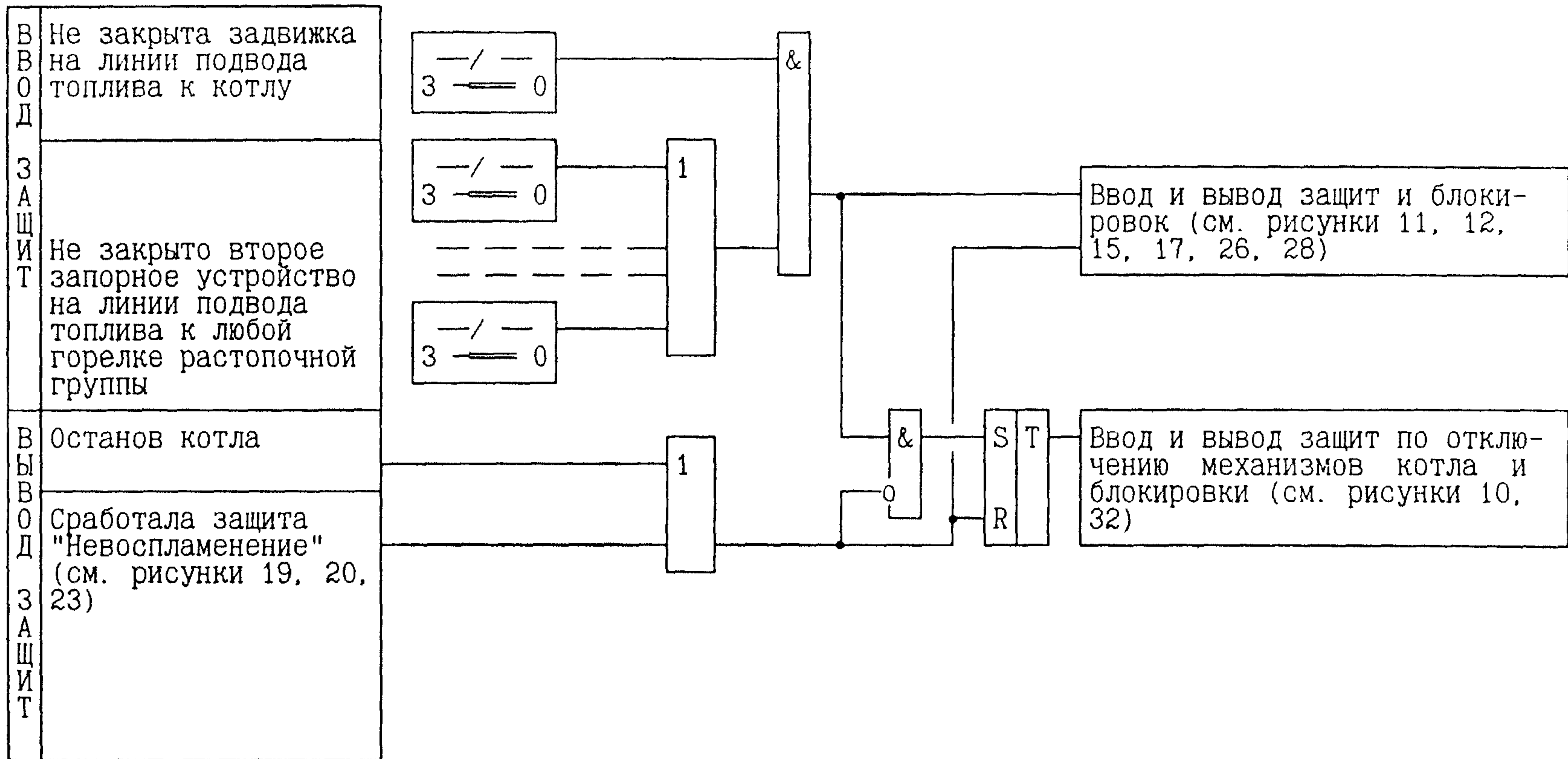
Рисунок 2 – Ввод защит при начале растопки и вывод после останова котла. Газовый котел без ПЗК у горелок, мазутный котел без ПЗК у горелок, пылеугольный котел
