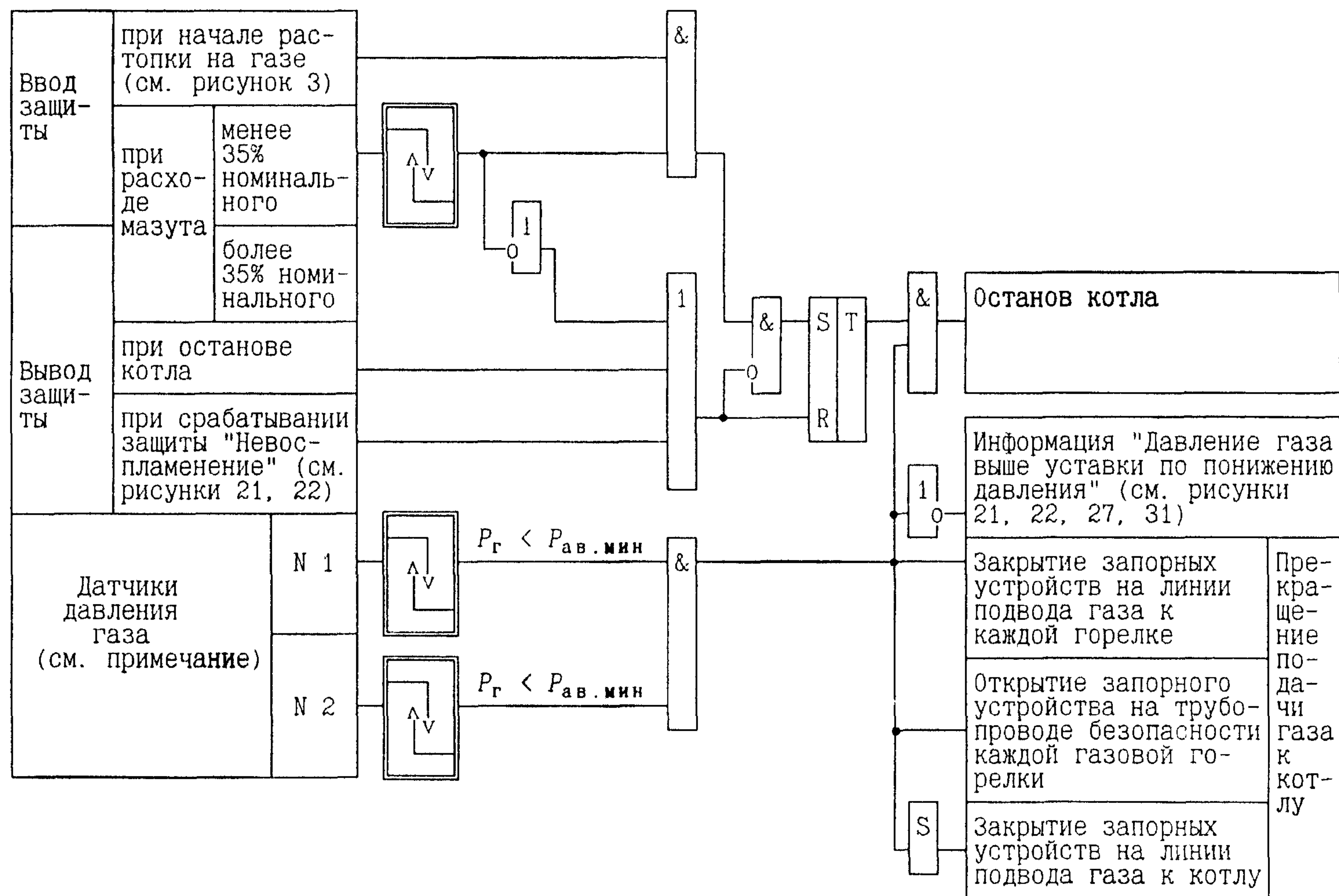
Рисунок 13 – Защита по понижению давления газа. Газомазутный котел.
