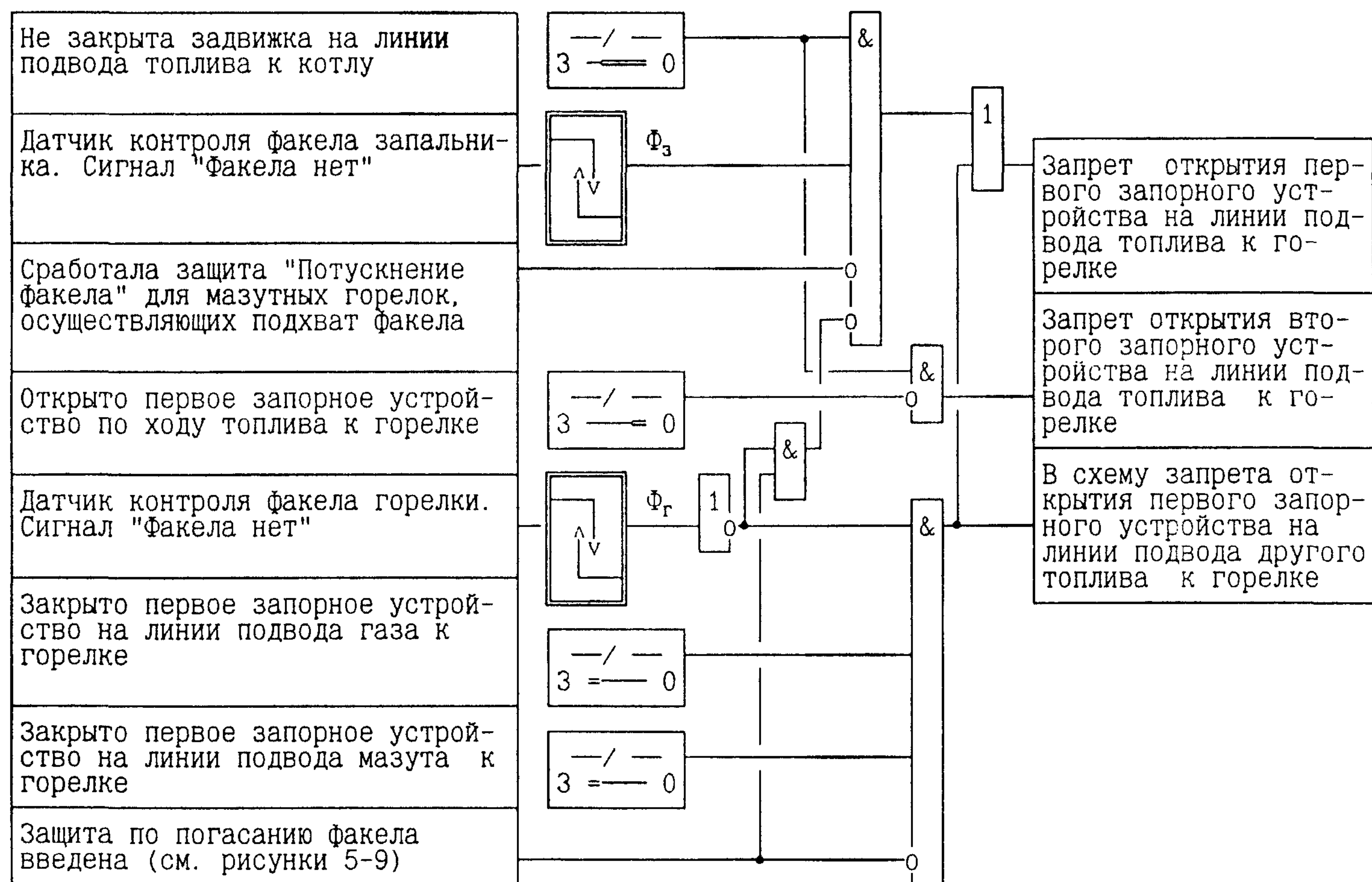
Рисунок 33 – Запреты при розжиге горелки.
