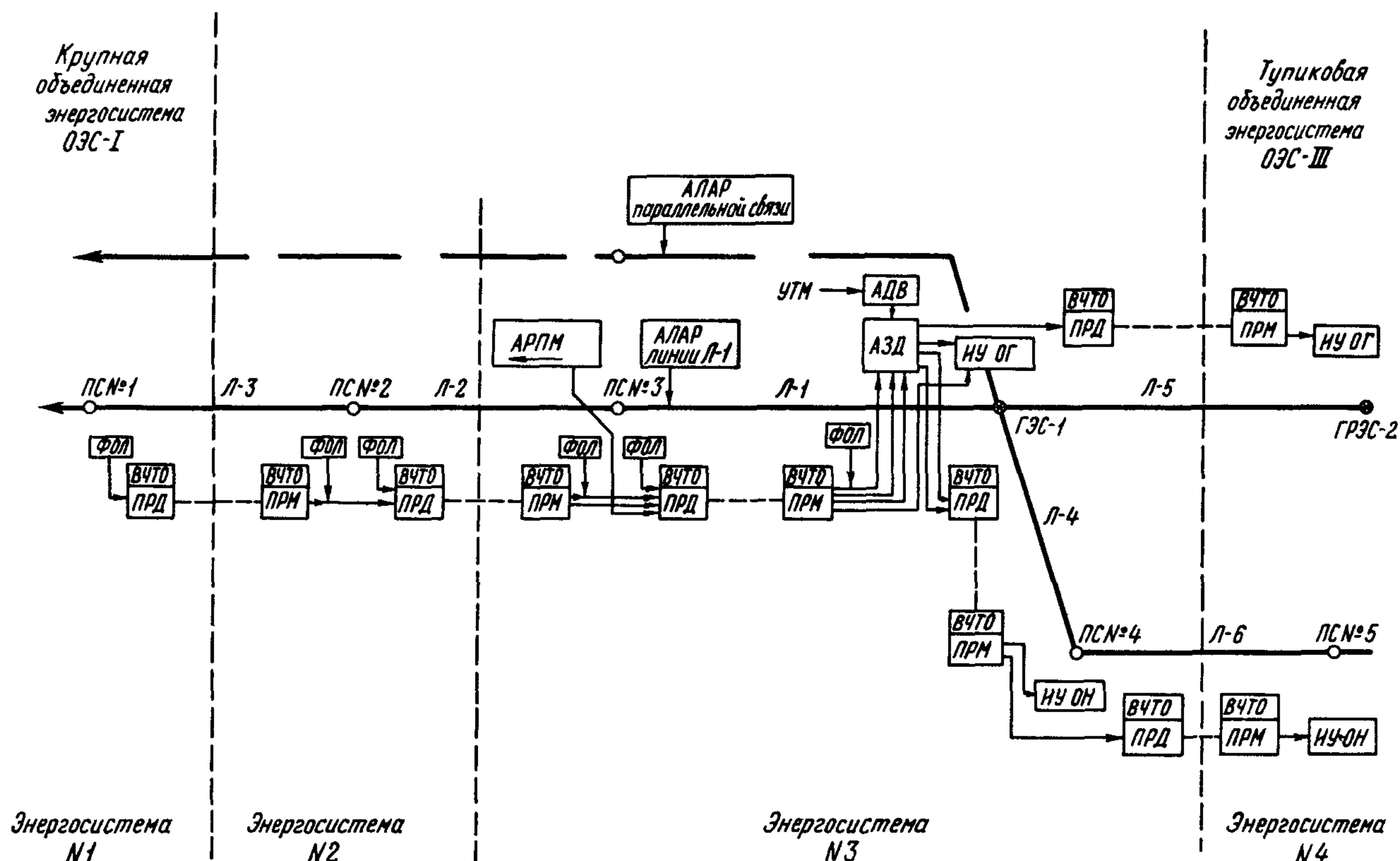
Поясняющая схема
