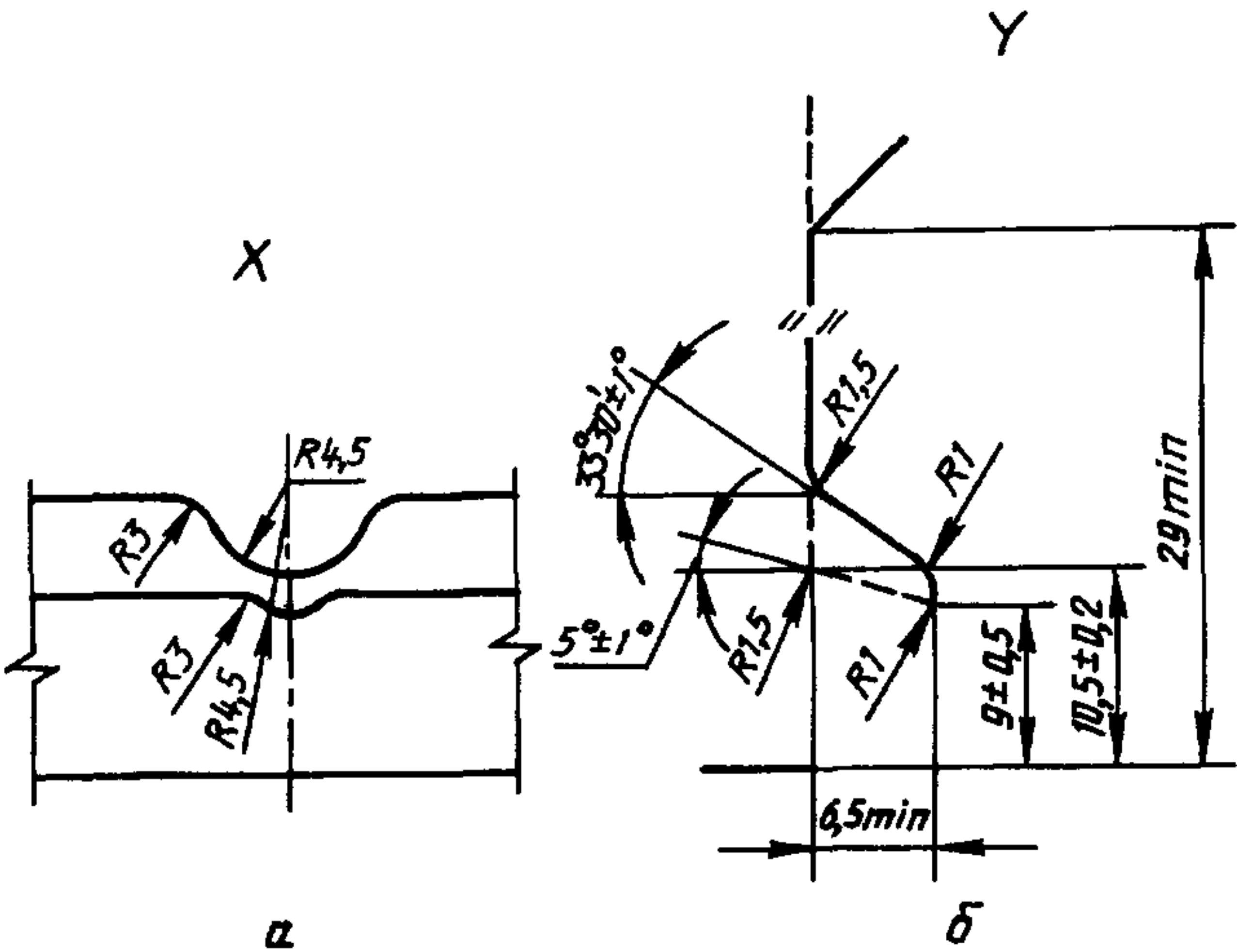
Деталь X — выемка
