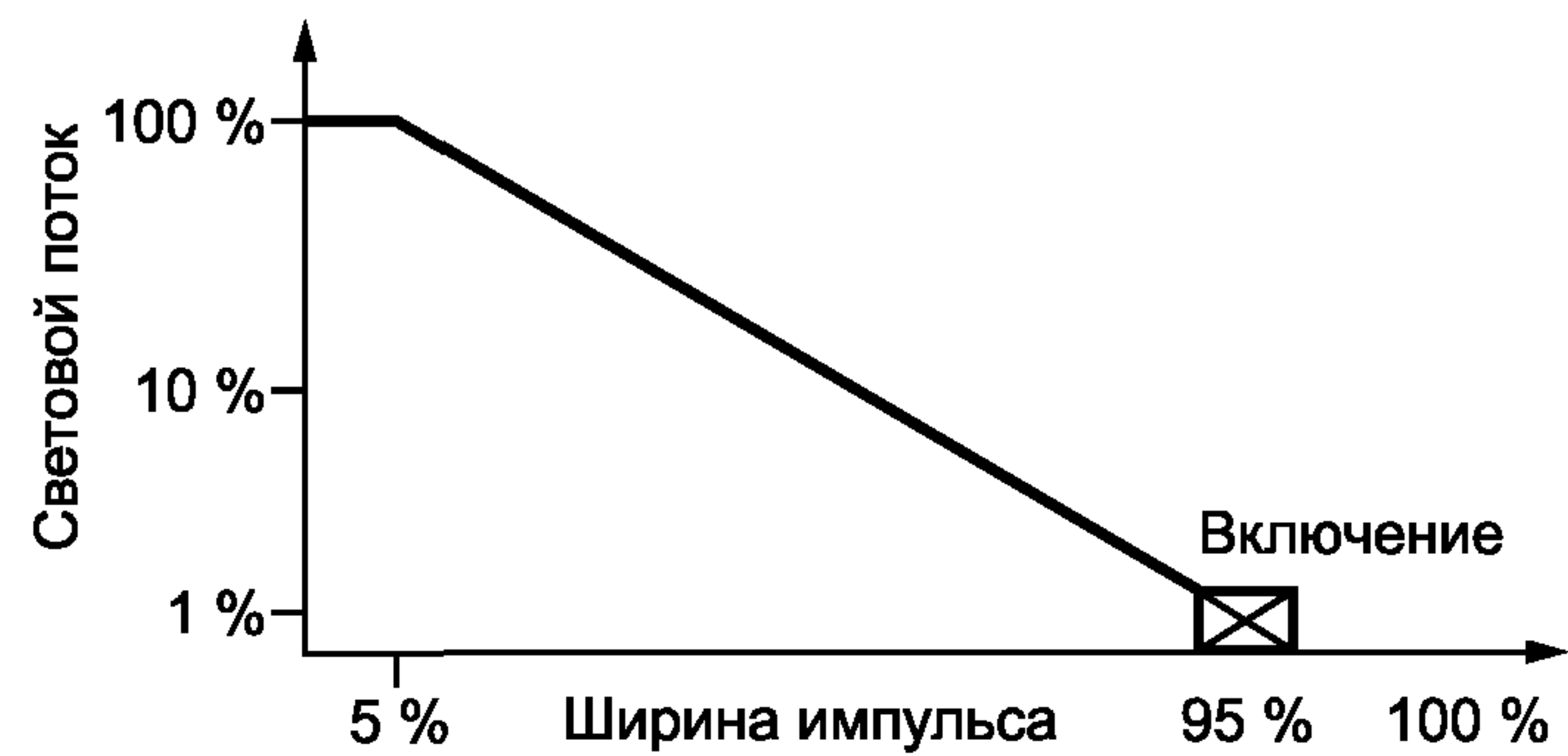
Кривая регулирования ПРА с минимальным световым потоком 1 %
