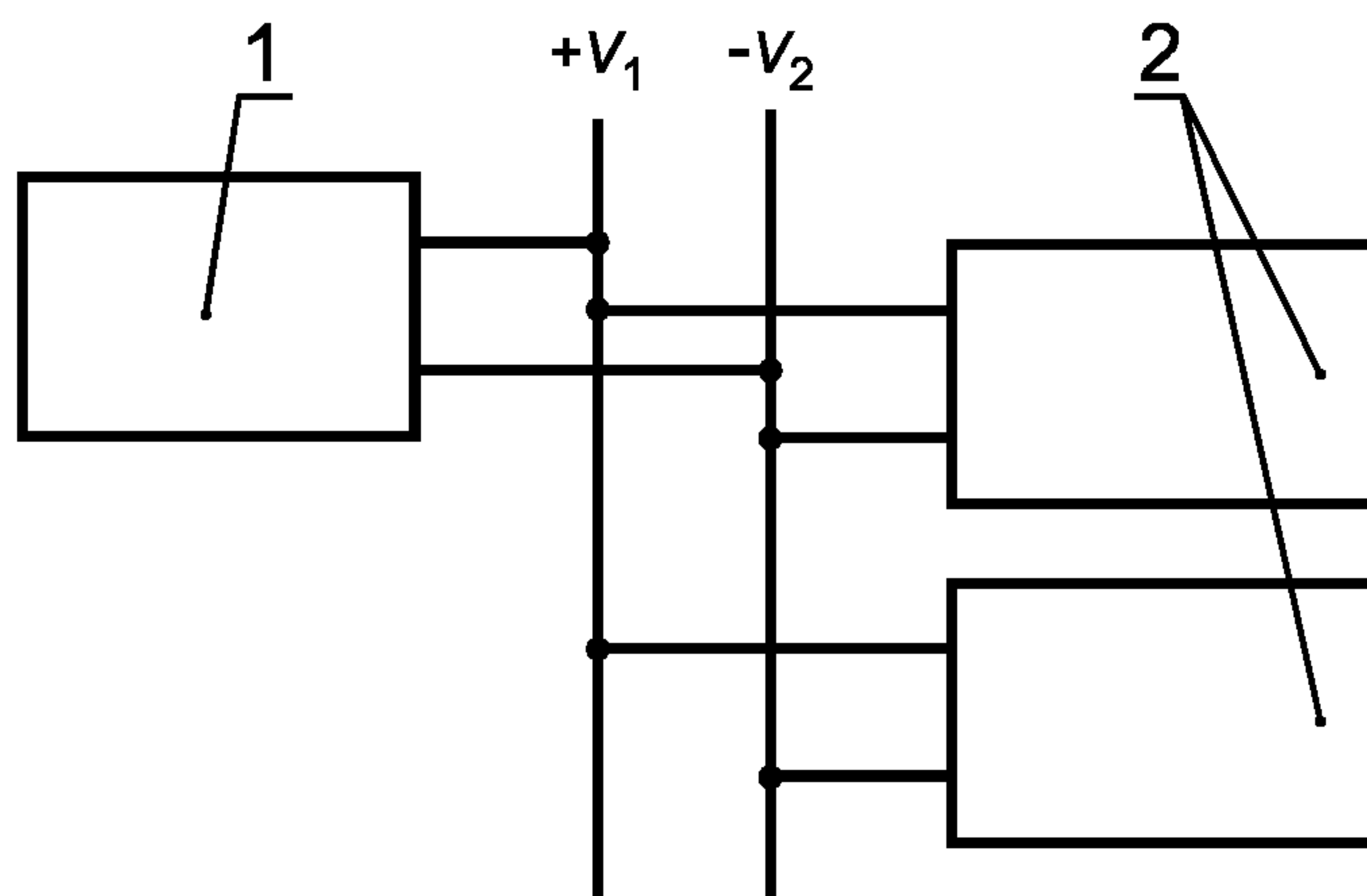
1 — блок управления; 2 — регулируемый ПРА
