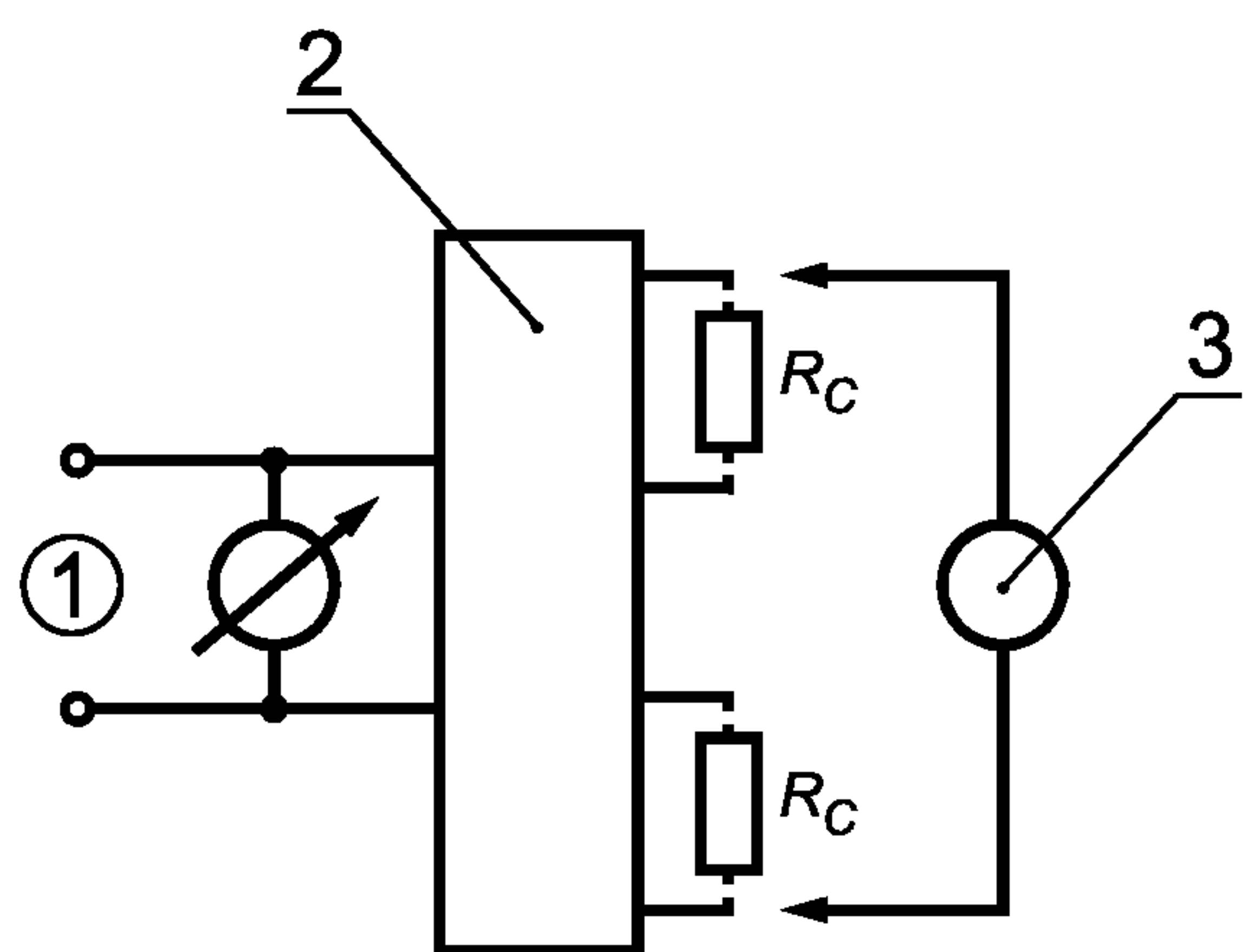
1 — сеть; 2 — испытуемый ПРА; 3 — измерительное устройство
