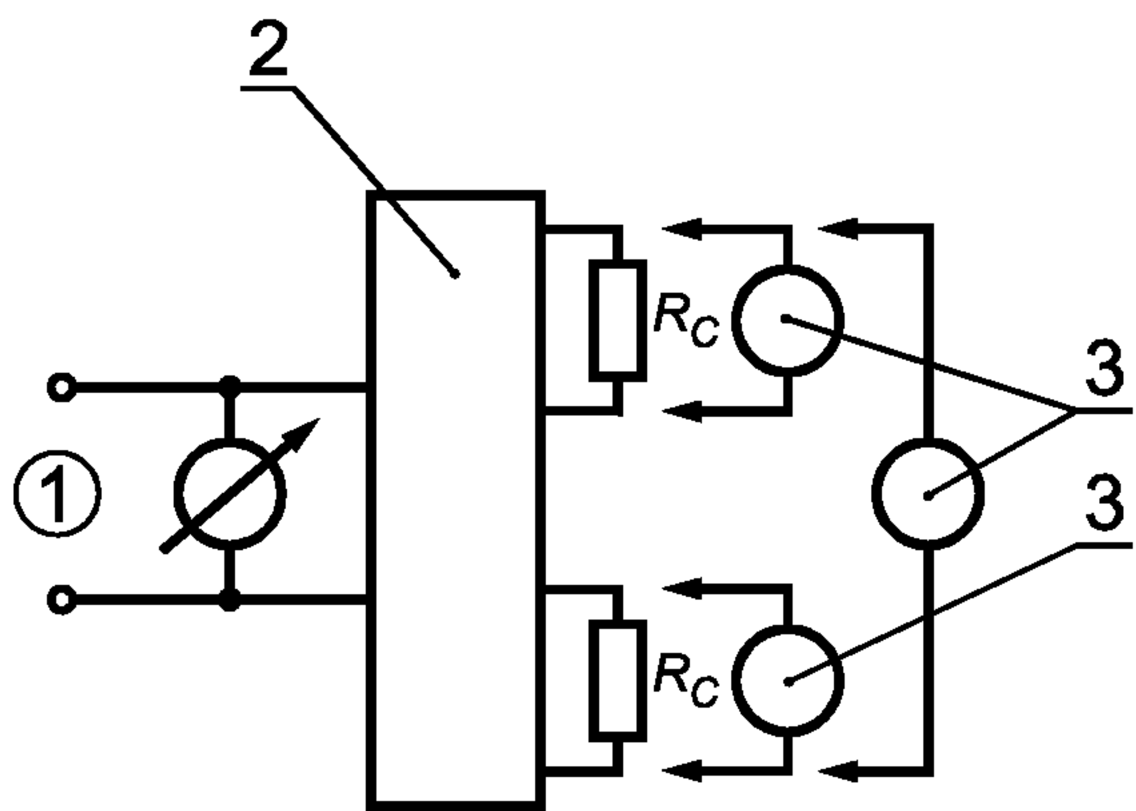
1 — сеть; 2 — испытуемый ПРА; 3 — измерительное устройство
