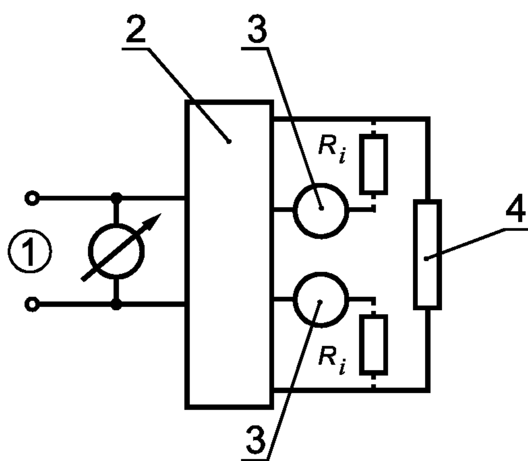
1 — сеть; 2 — испытуемый ПРА; 3 — измерительное устройство; 4 — лампа
