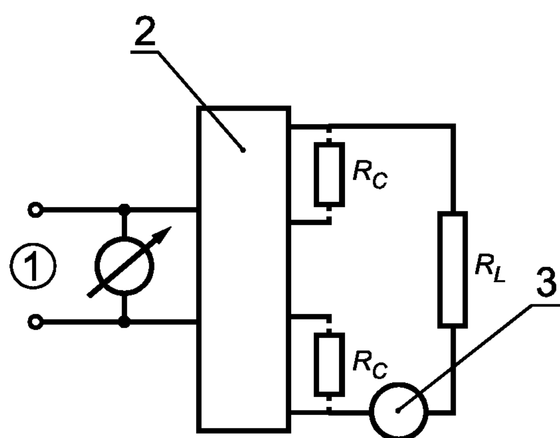
1 — сеть; 2 — испытуемый ПРА; 3 — измерительное устройство
