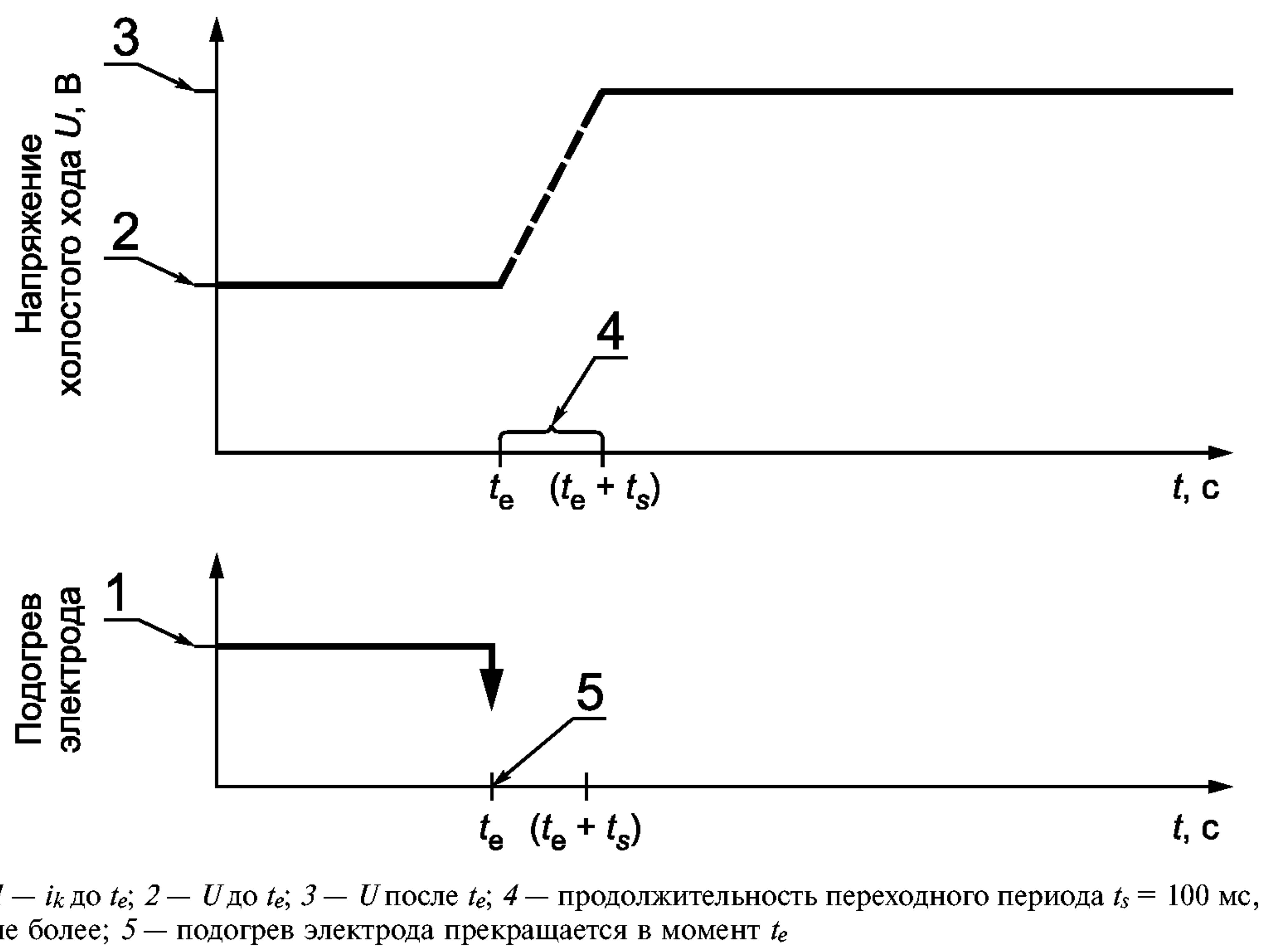
Рисунок 2.1 — ПРА, который прекращает ток предварительного подогрева при повышении напряжения холостого хода
