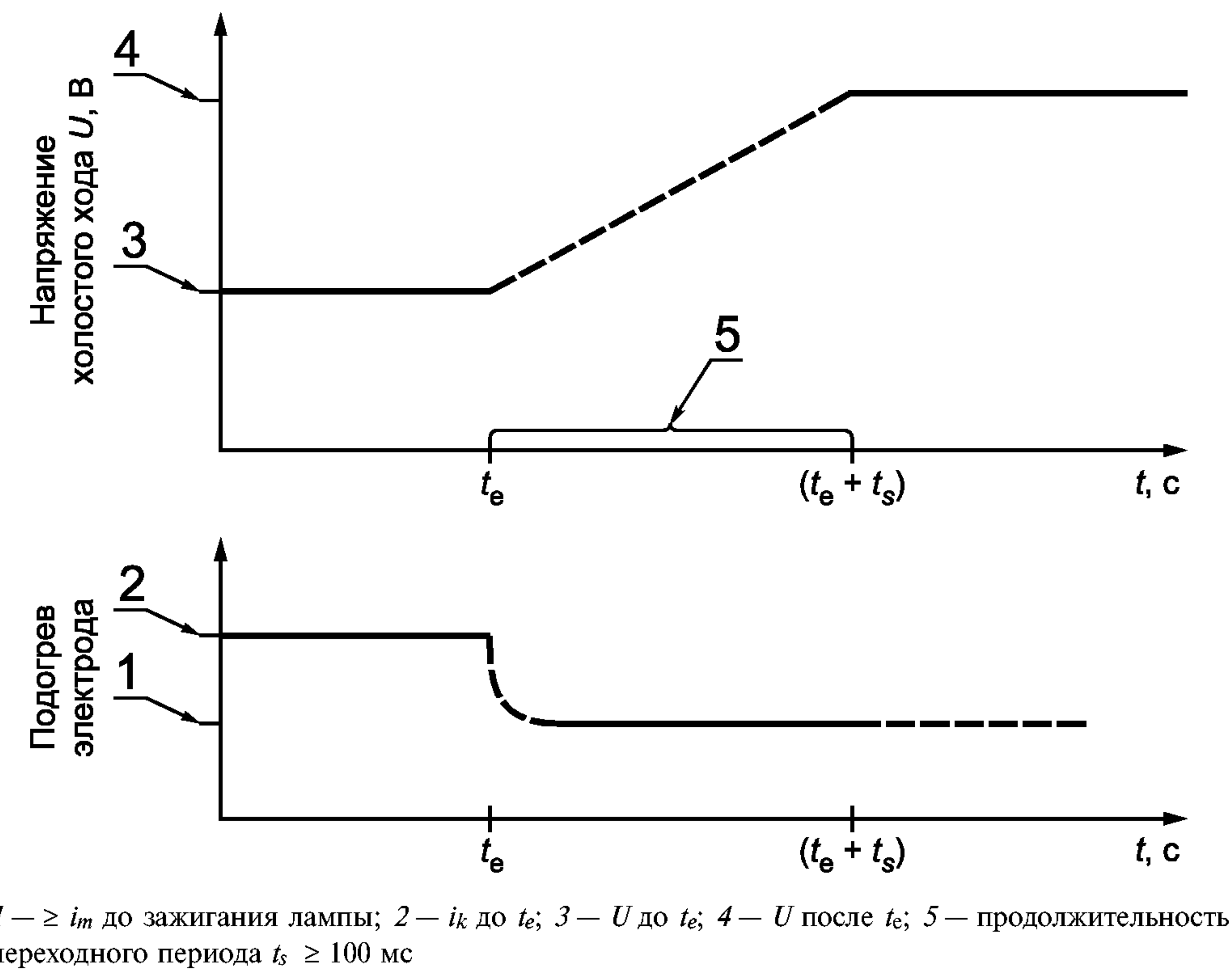
Рисунок 2.2 — ПРА, который имеет продолжительность переходного периода напряжения холостого хода > 100 мс
