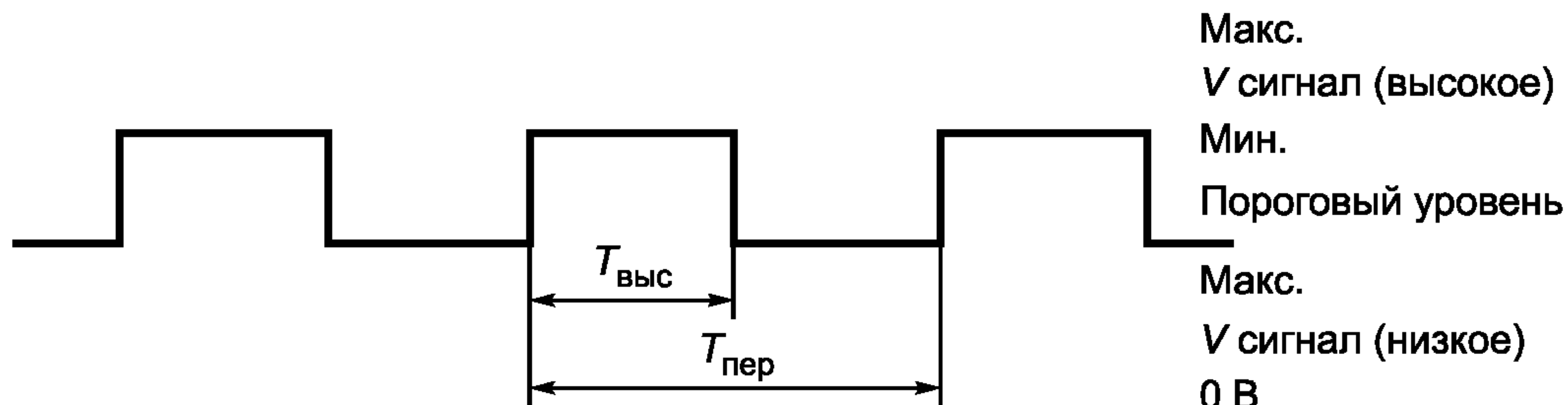
Типичный ШИМ сигнал
