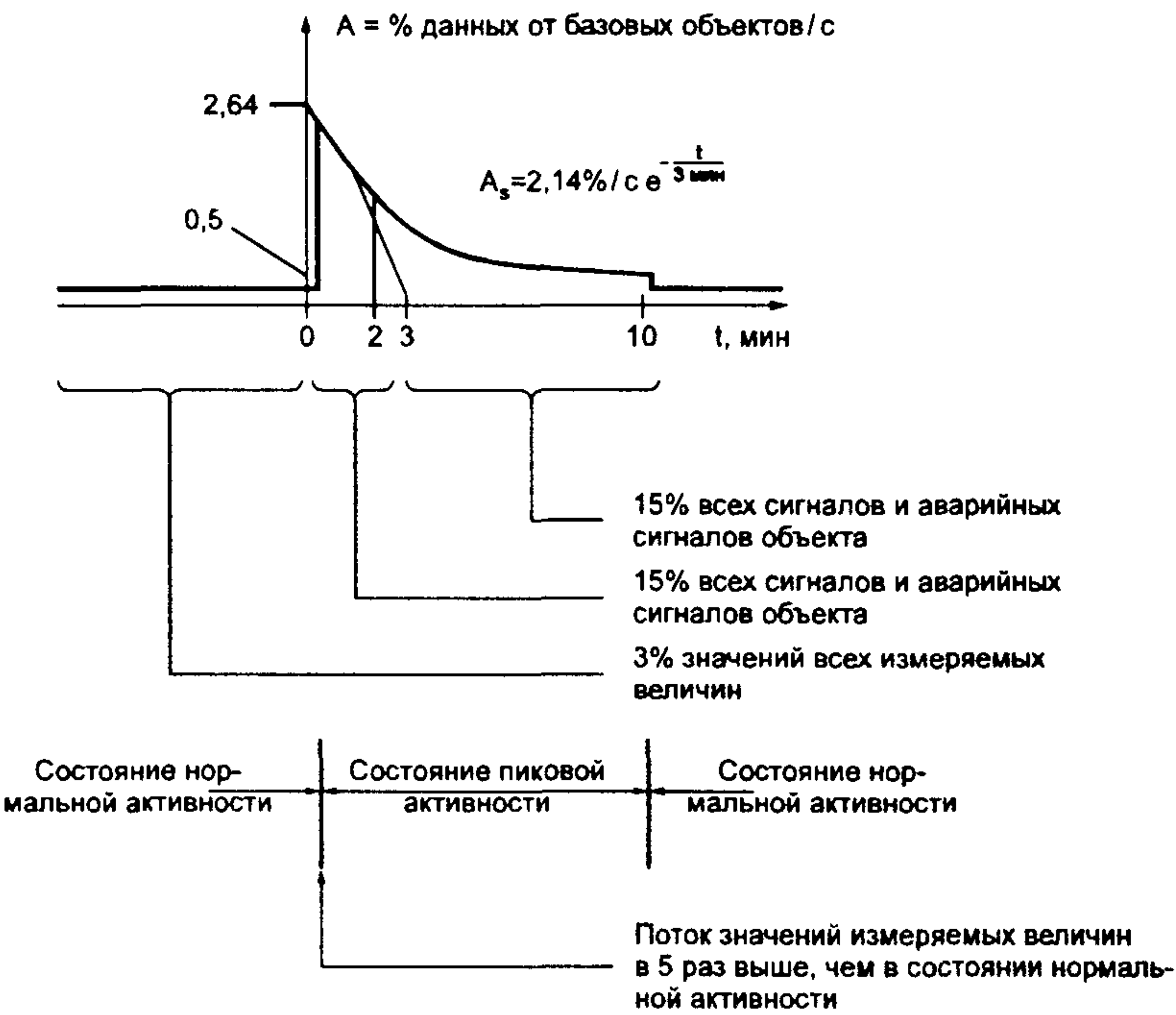
Рисунок А.1 — Определение расчетного потока данных
