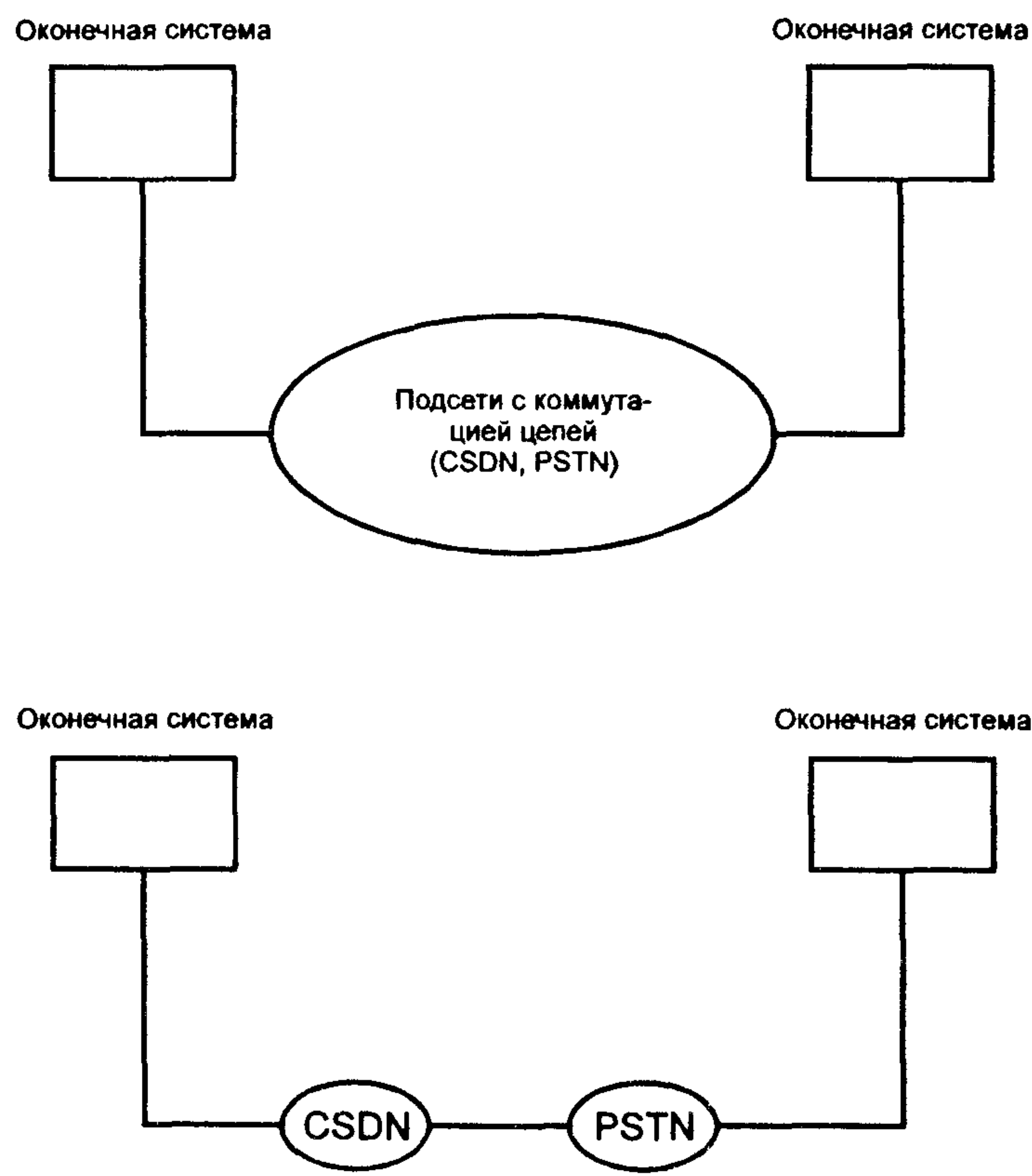
Рисунок 7 — Базовые структуры, основанные на коммутации цепей
