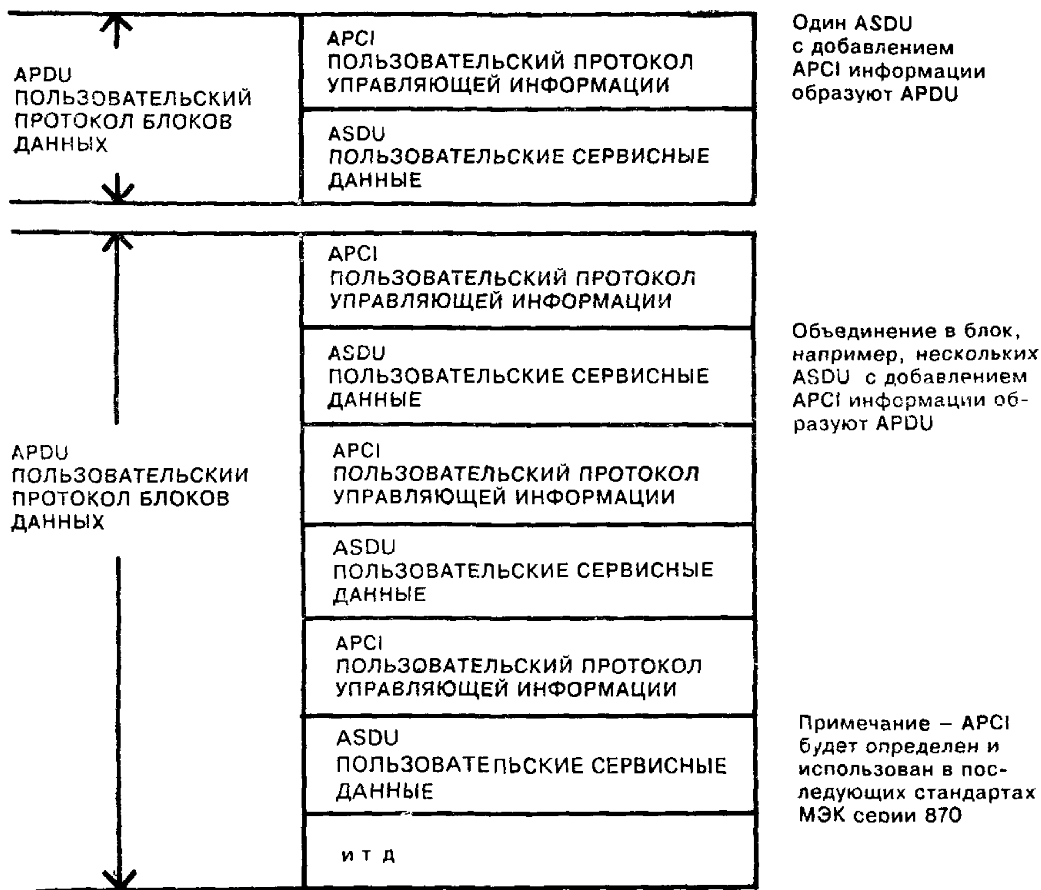
Рисунок 5 — Общая структура ПОЛЬЗОВАТЕЛЬСКОГО ПРОТОКОЛА БЛОКОВ ДАННЫХ
