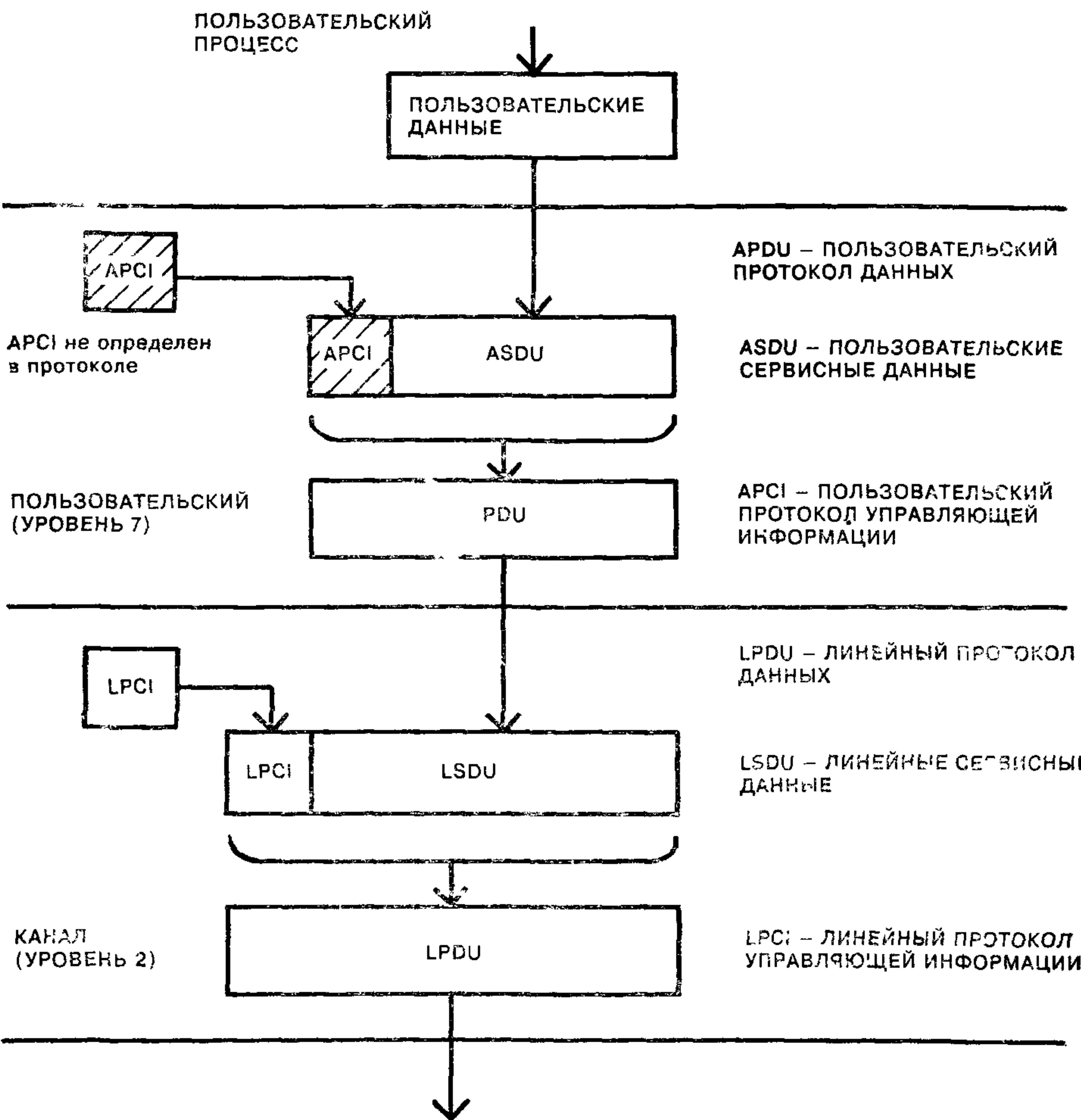
Рисунок 4 — Связи между блоками данных
