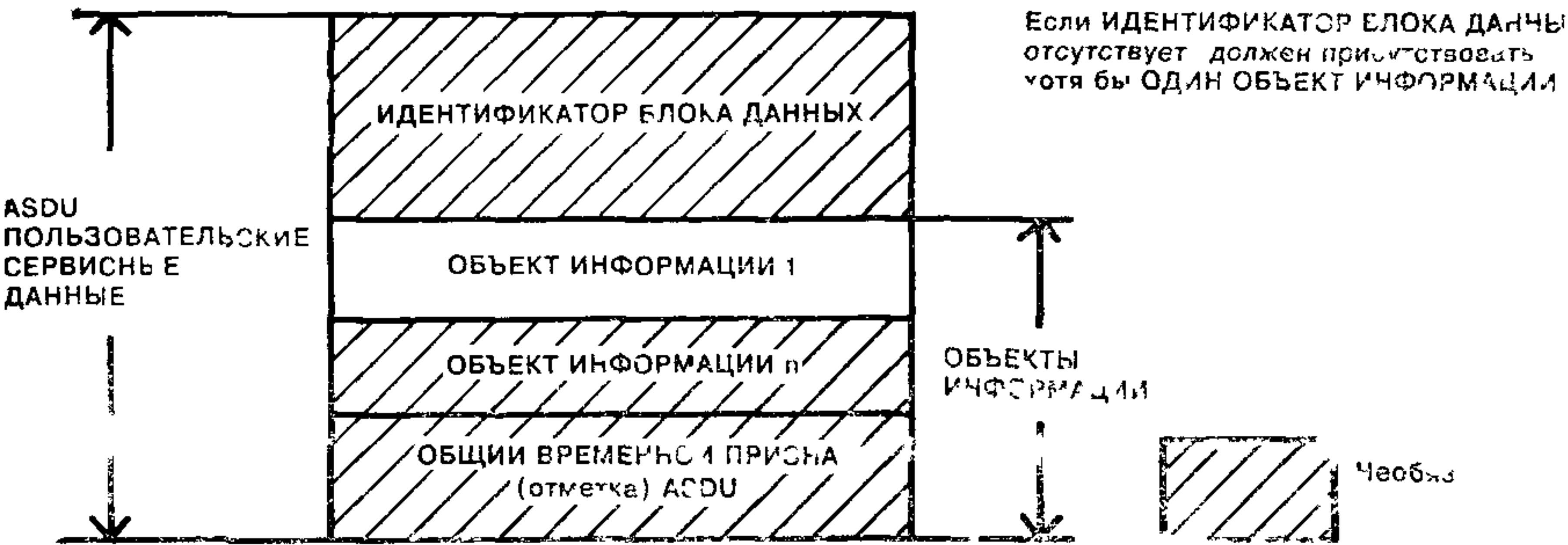
Рисунок 6 — Основная структура БЛОКА ПОЛЬЗОВАТЕЛЬСКИХ СЕРВИСНЫХ ДАННЫХ
