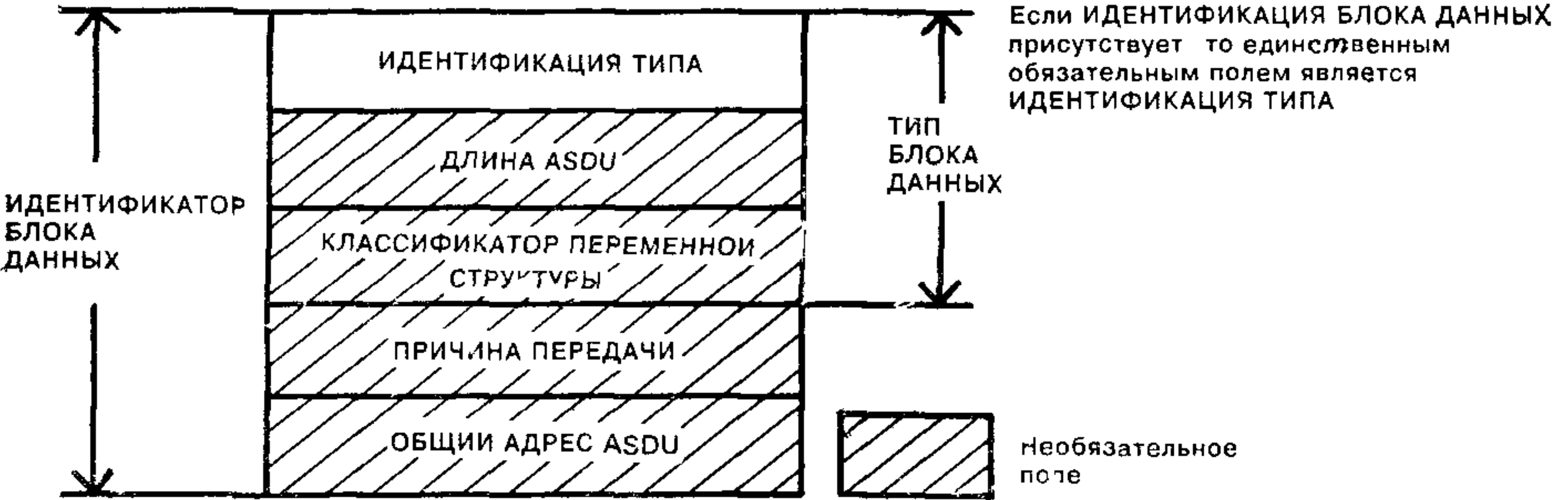
Рисунок 7 — Основная структура ИДЕНТИФИКАТОРА БЛОКА ДАННЫХ
