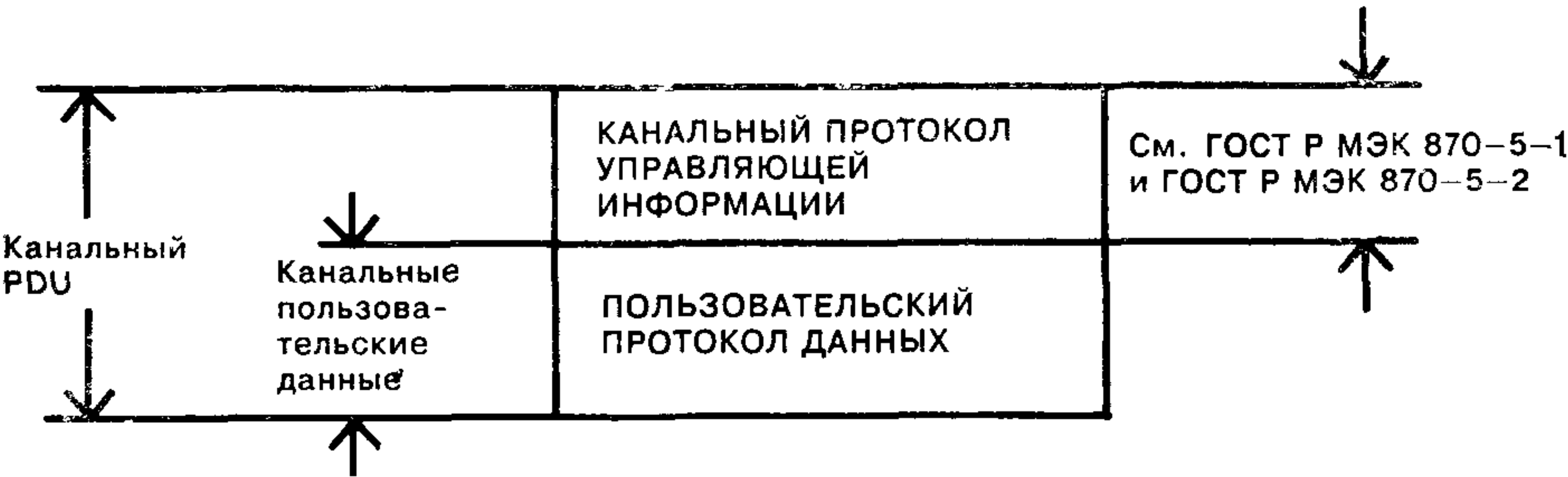
Рисунок 3 — Структура кадра для модели 2
