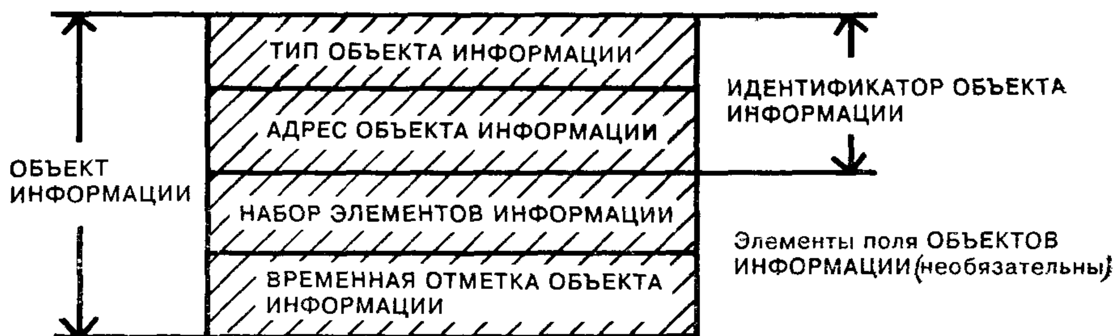
Рисунок 8 — Общая структура ОБЪЕКТА ИНФОРМАЦИИ
