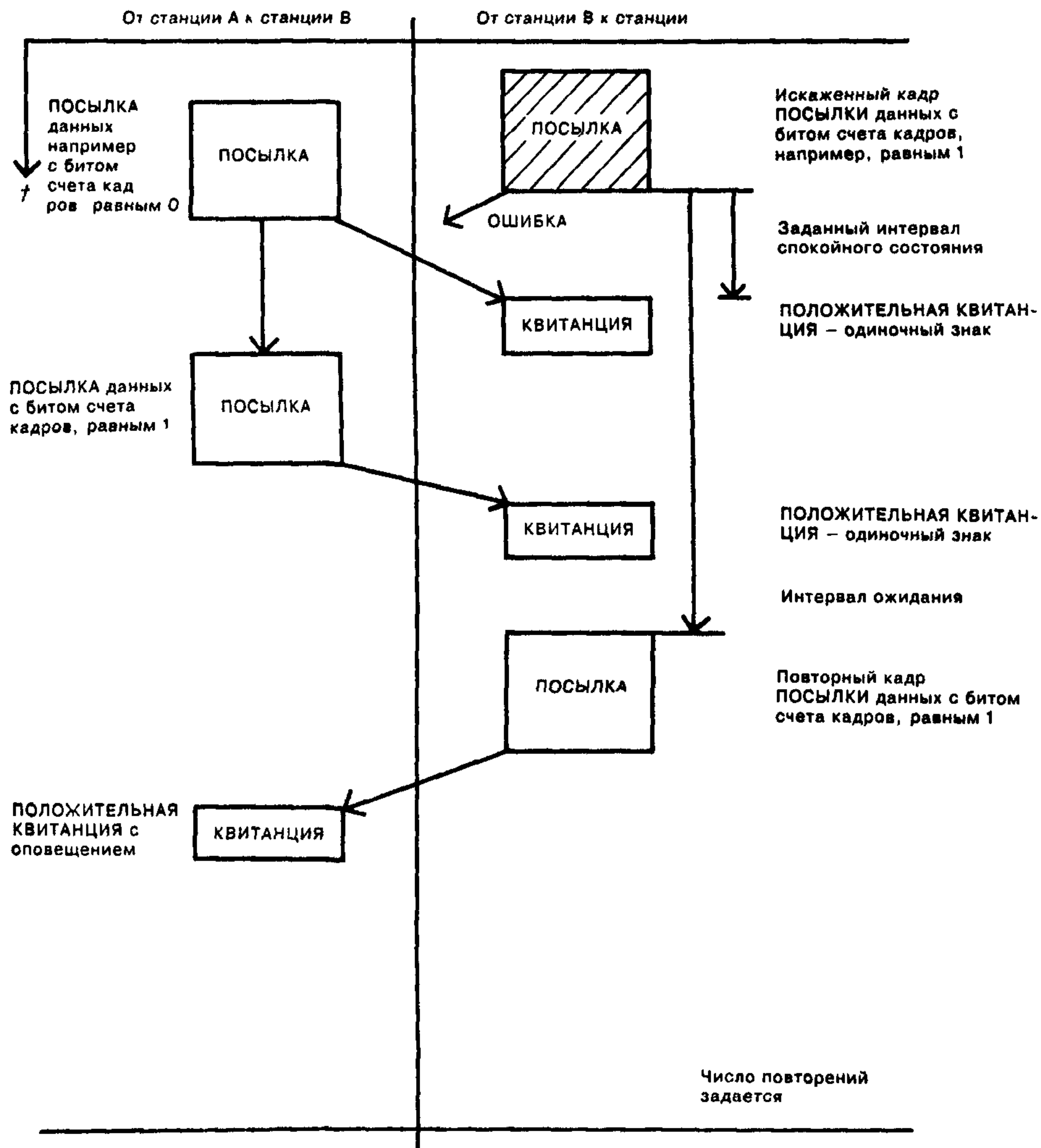
Рисунок 13 — Балансные процедуры передачи. Искаженный кадр ПОСЫЛКИ
