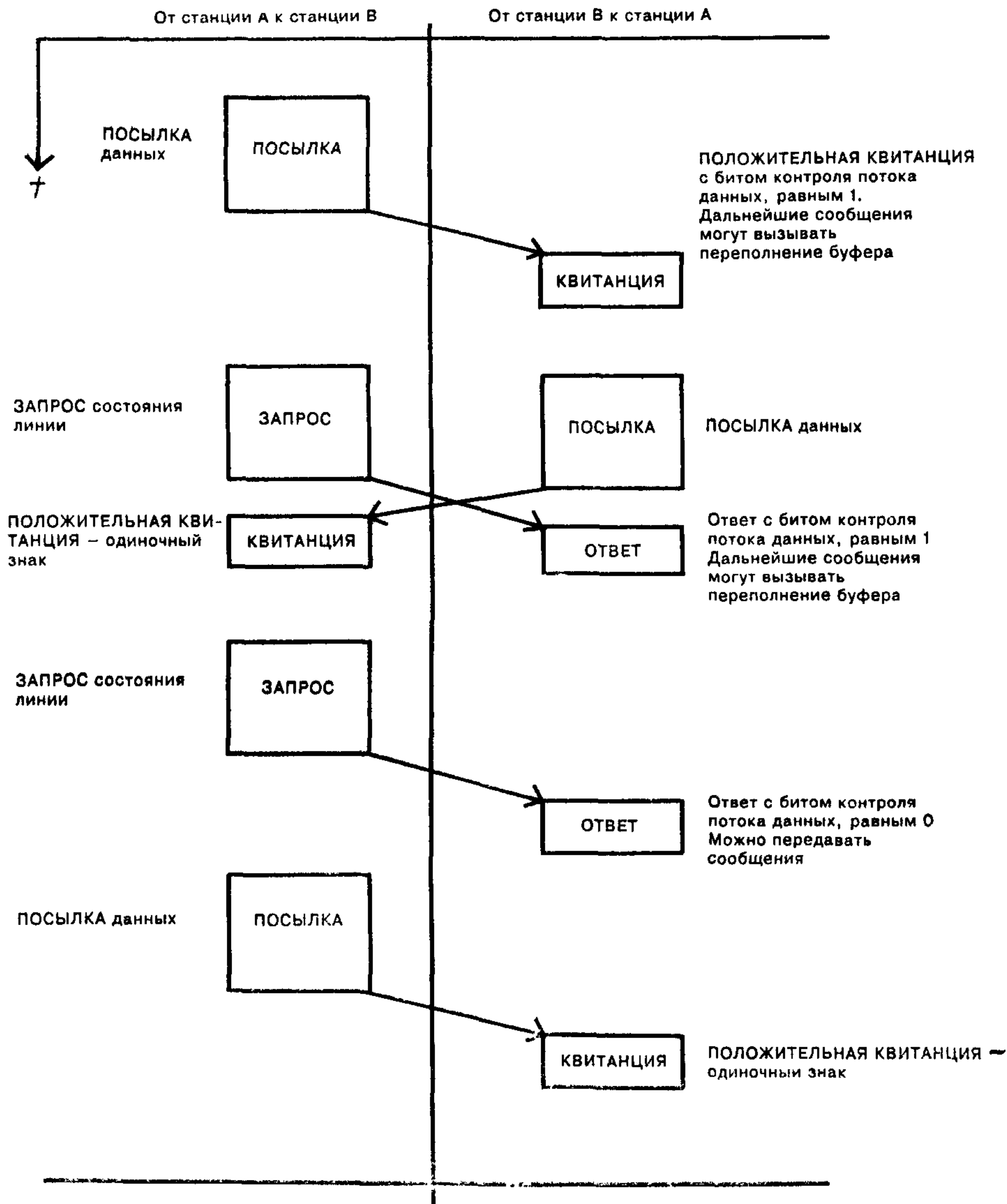
Рисунок 12 — Балансные процедуры передачи. Контроль потока данных
