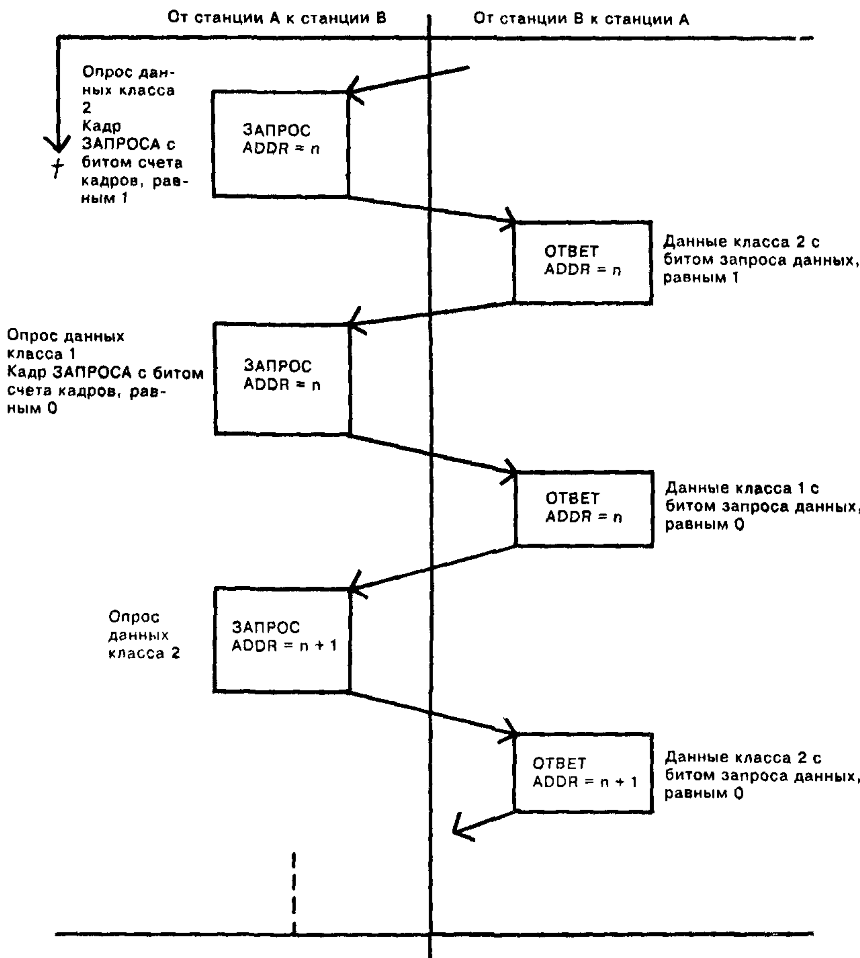
Рисунок 7 — Небалансные процедуры передачи, неискаженные процедуры ЗАПРОС/ОТВЕТ
