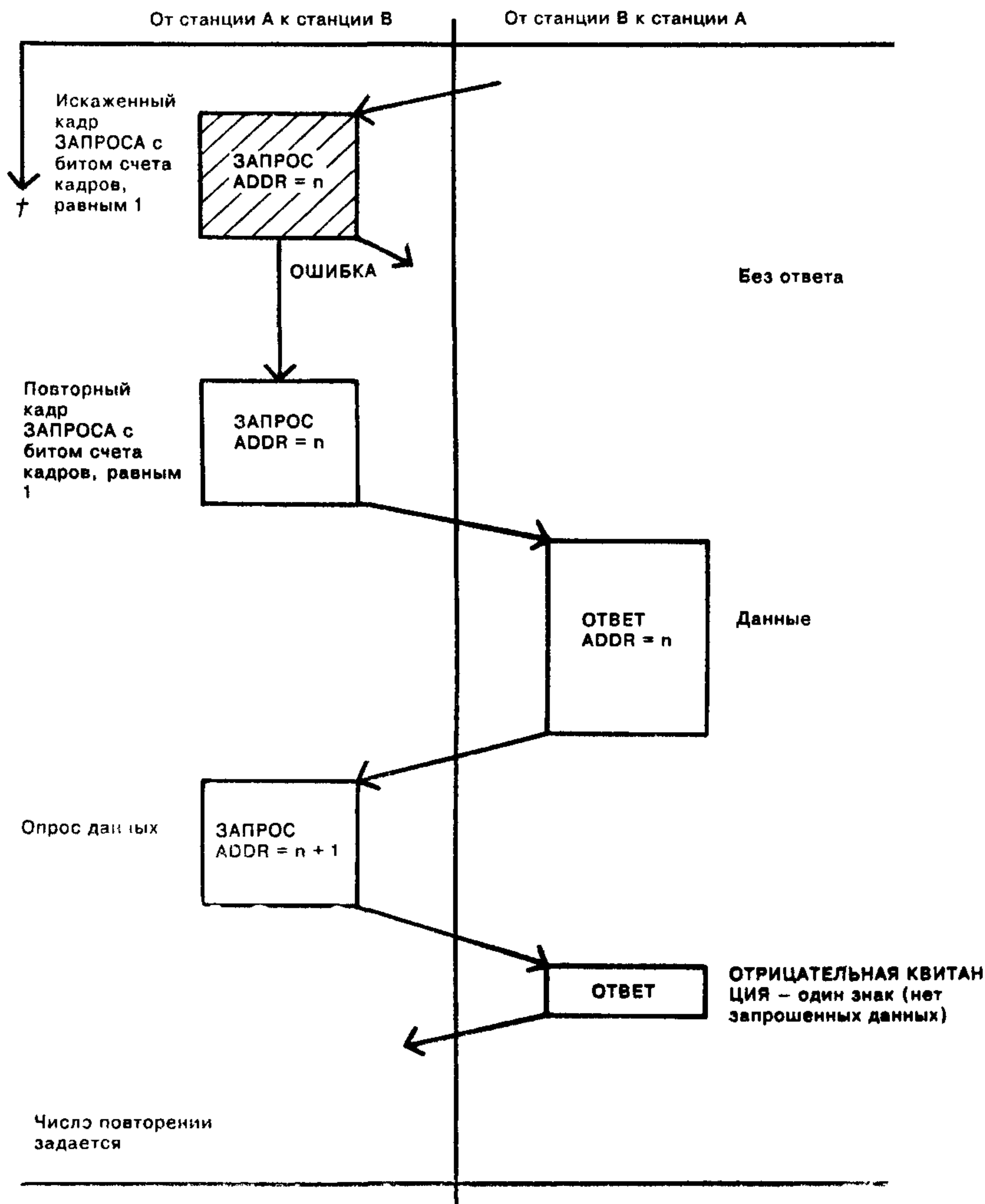
Рисунок 8 — Небалансные процедуры передачи ЗАПРОС/ОТВЕТ, кадр ЗАПРОСА искажен
