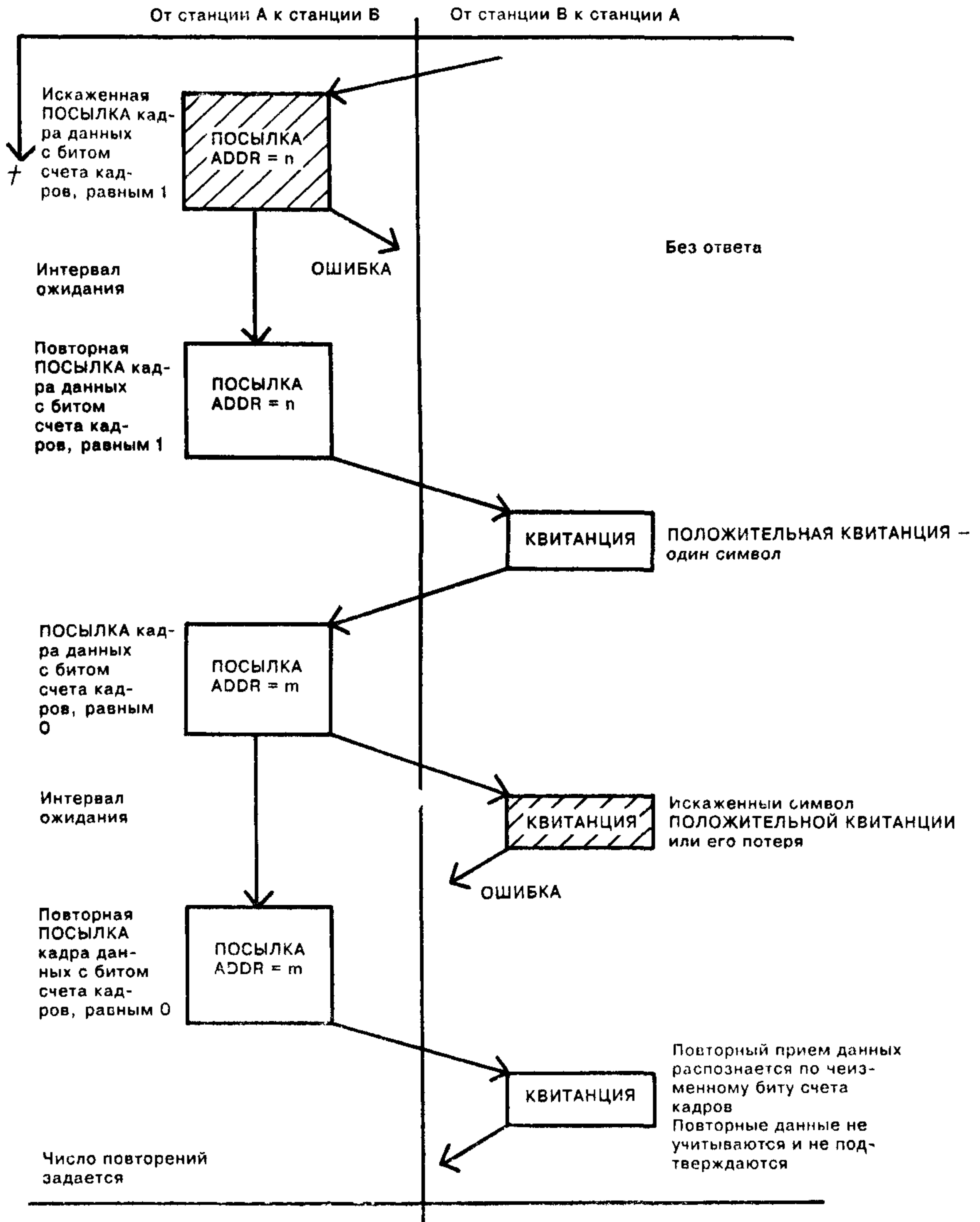
Рисунок 4 — Небалансные процедуры передачи, искаженные процедуры ПОСЫЛКА/ПОДТВЕРЖДЕНИЕ
