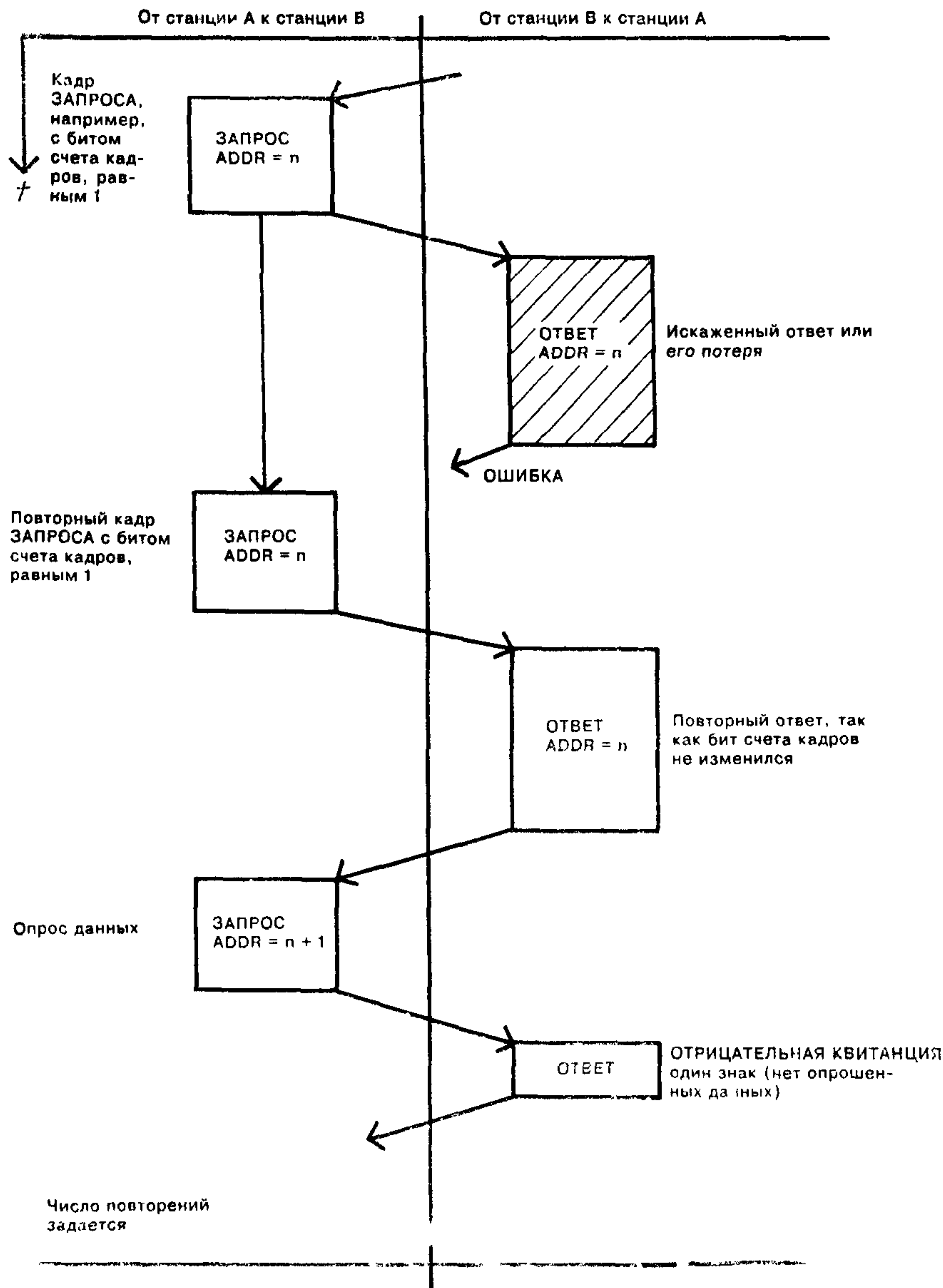
Рисунок 9 — Небалансные процедуры передачи ЗАПРОС/ОТВЕТ, кадр ОТВЕТА искажен
