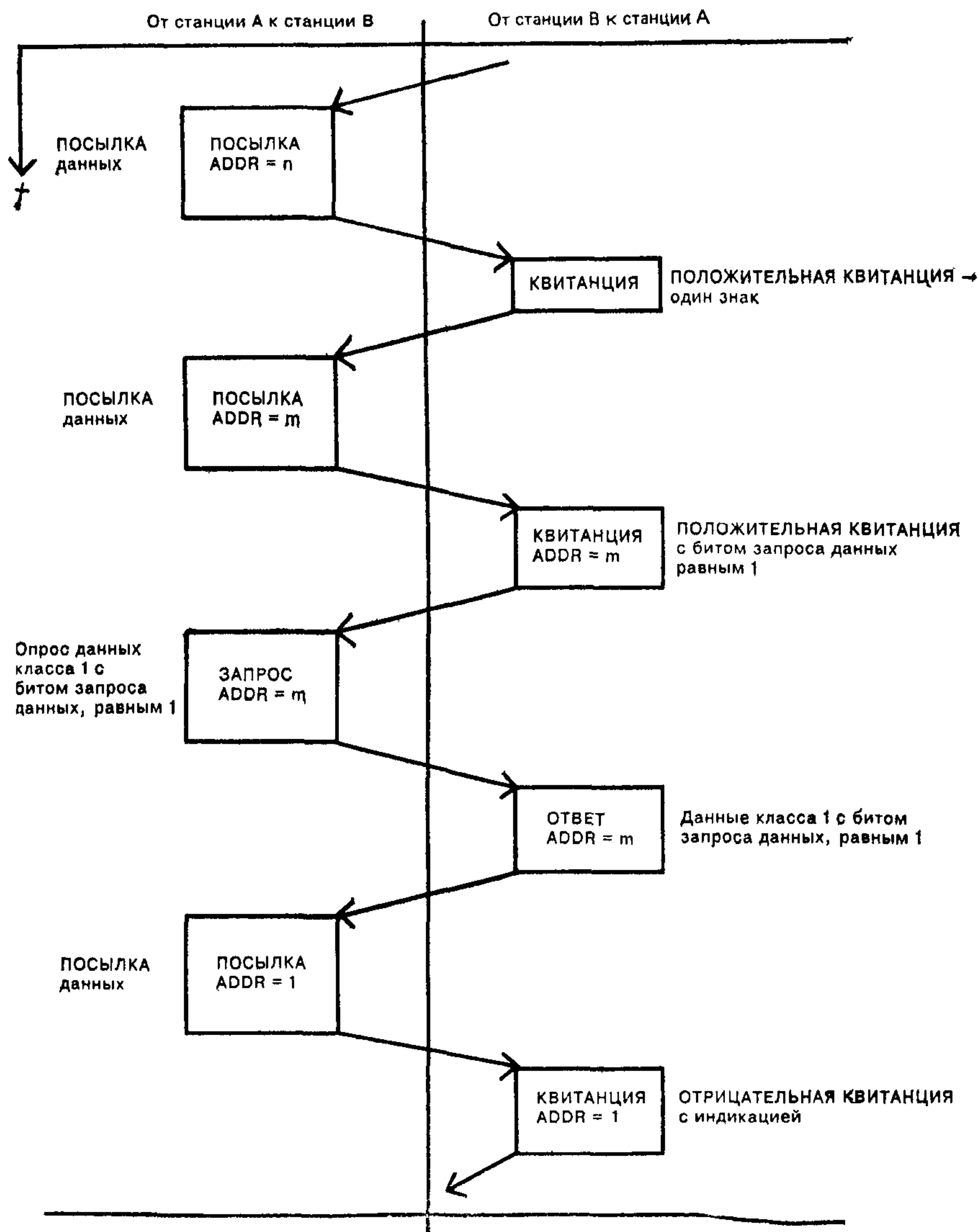
Рисунок 3 — Небалансные процедуры передачи, неискаженные процедуры ПОСЫЛКА/ПОДТВЕРЖДЕНИЕ
