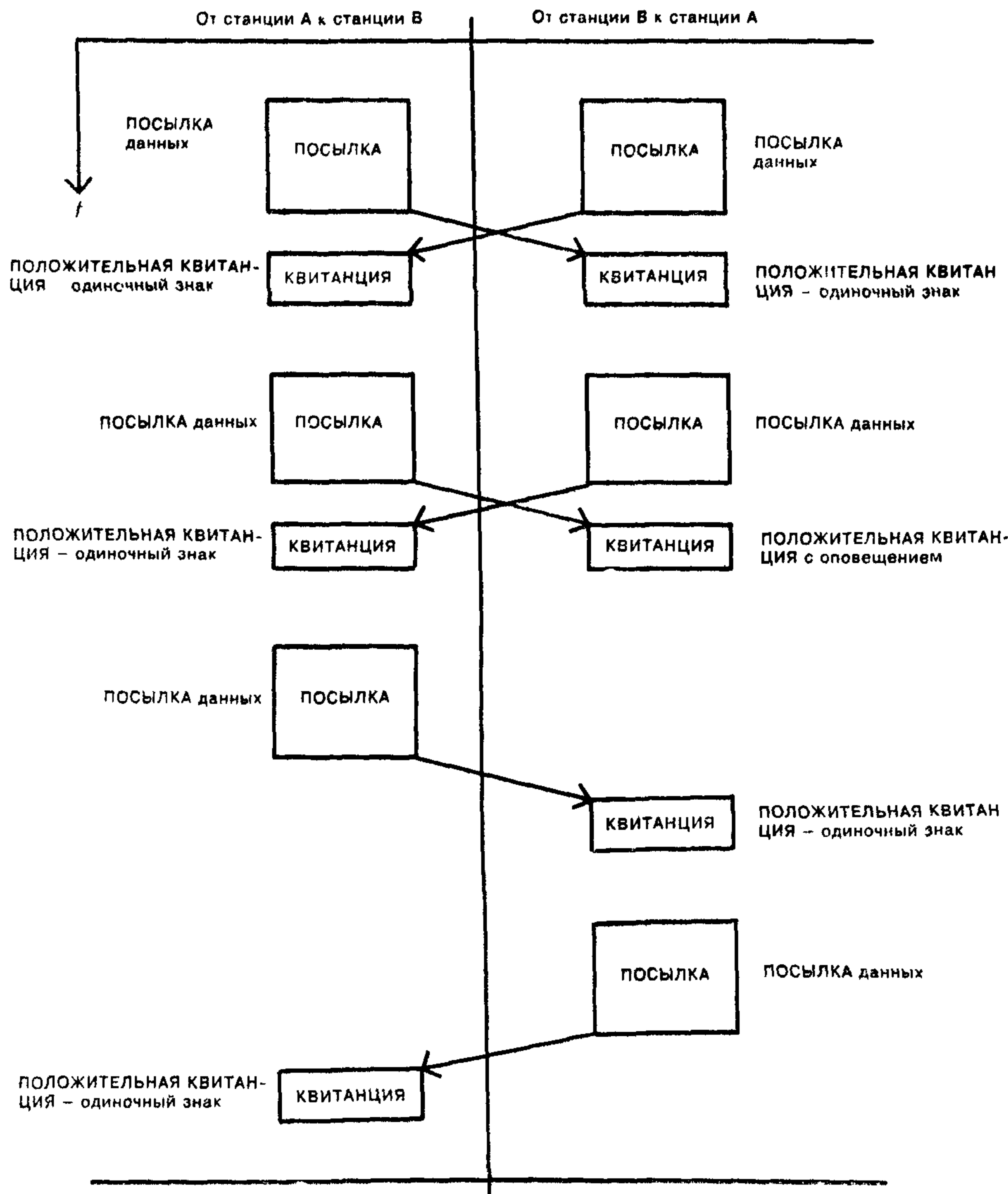
Рисунок 11 — Балансные процедуры передачи. Неисказенные процедуры ПОСЫЛКА/ПОДТВЕРЖДЕНИЕ
