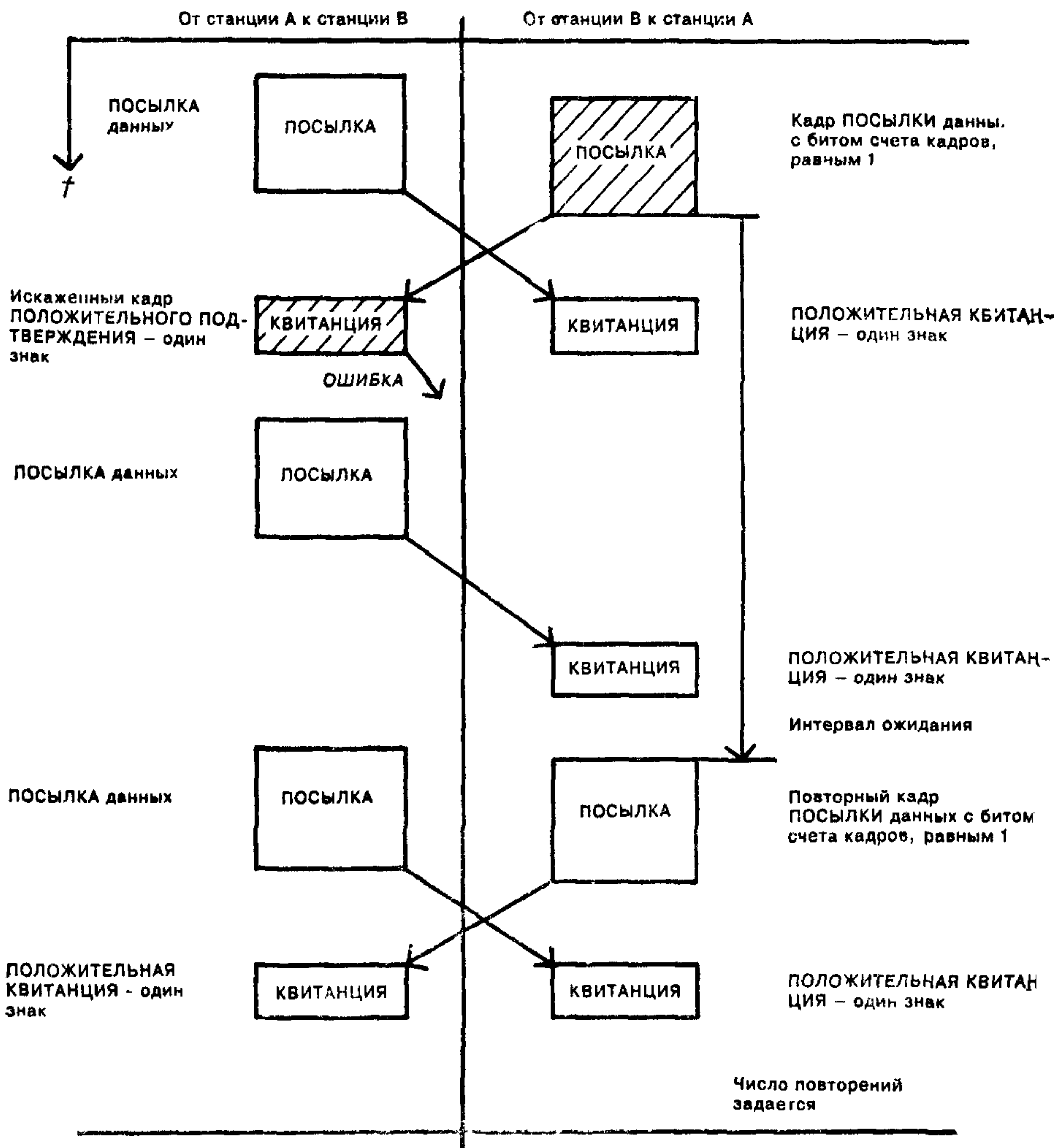
Рисунок 15 — Балансные процедуры передачи. Искаженный кадр ПОДТВЕРЖДЕНИЯ
