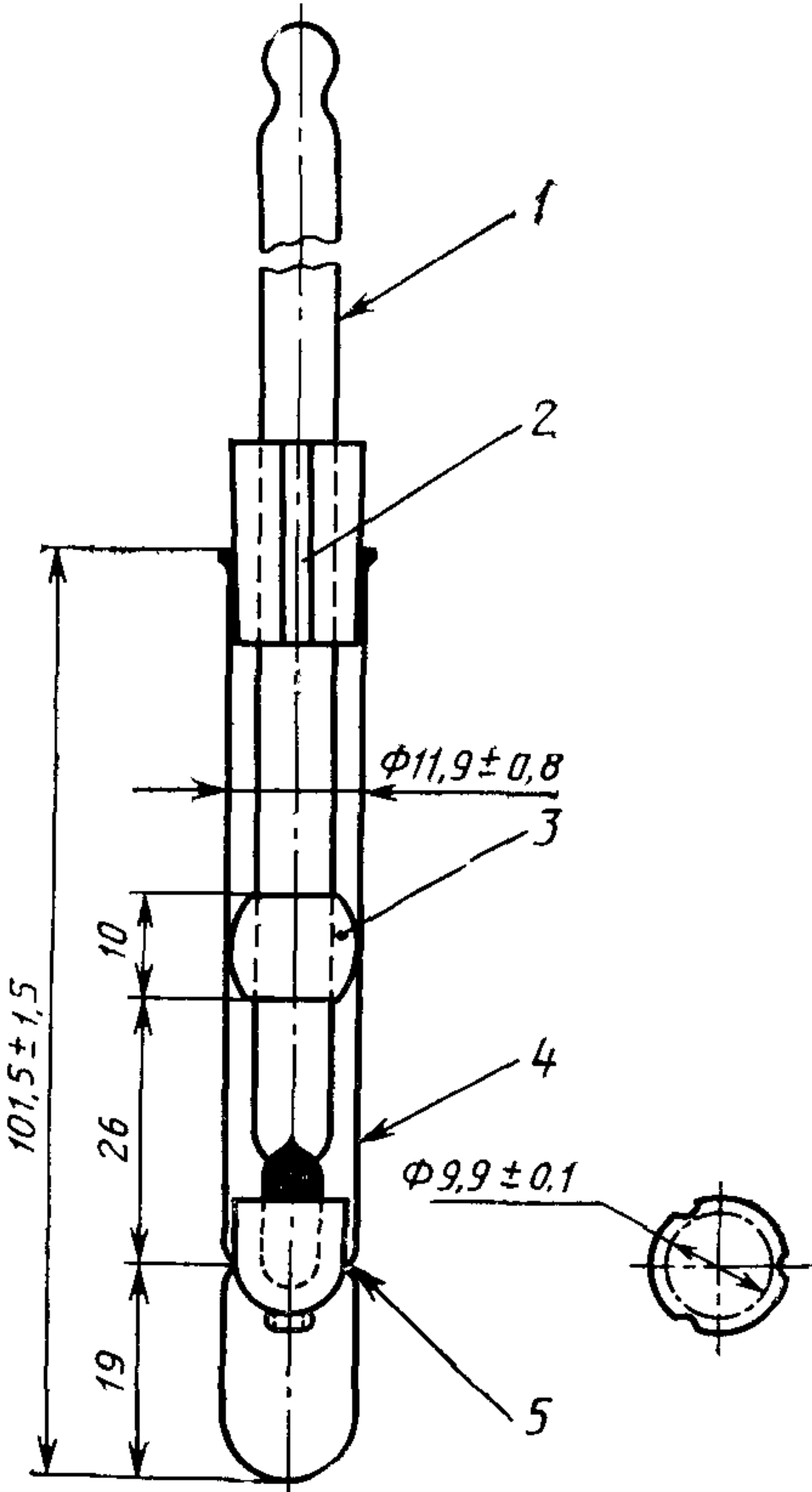
1 — термометр, 2 — прорезь в пробке для вентиляции; 3 — направляющая пробка для обеспечения необходимого зазора между термометром и пробиркой, 4 — пробирка из боросиликатного стекла, 5 — три равномерно расположенных углубления для удержания чашки
