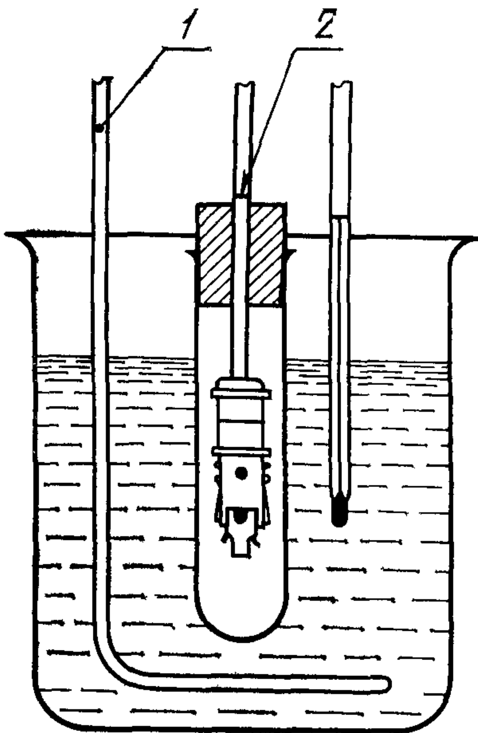
Рисунок 6 — Испытательное устройство
