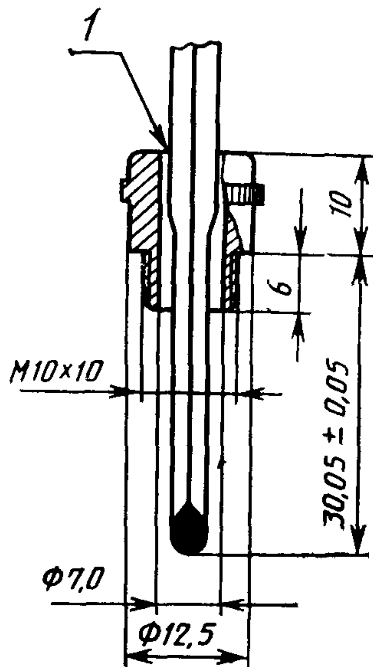
Рисунок 4 — Термометр и муфта
