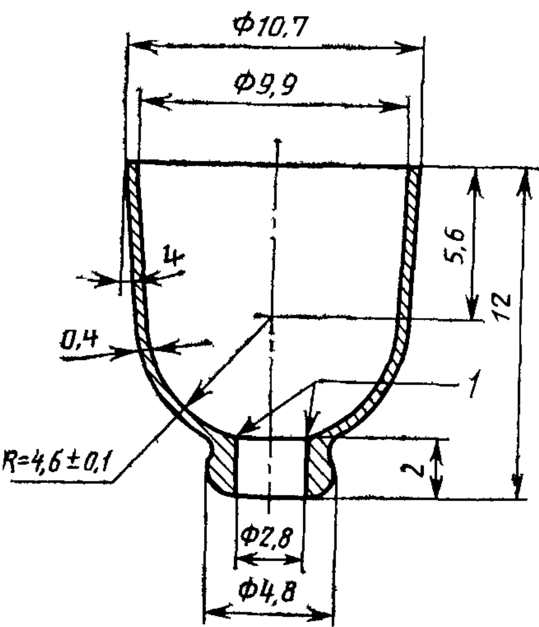
1 — острый край (удалены только заусенцы) Рисунок 1 — Чашка
