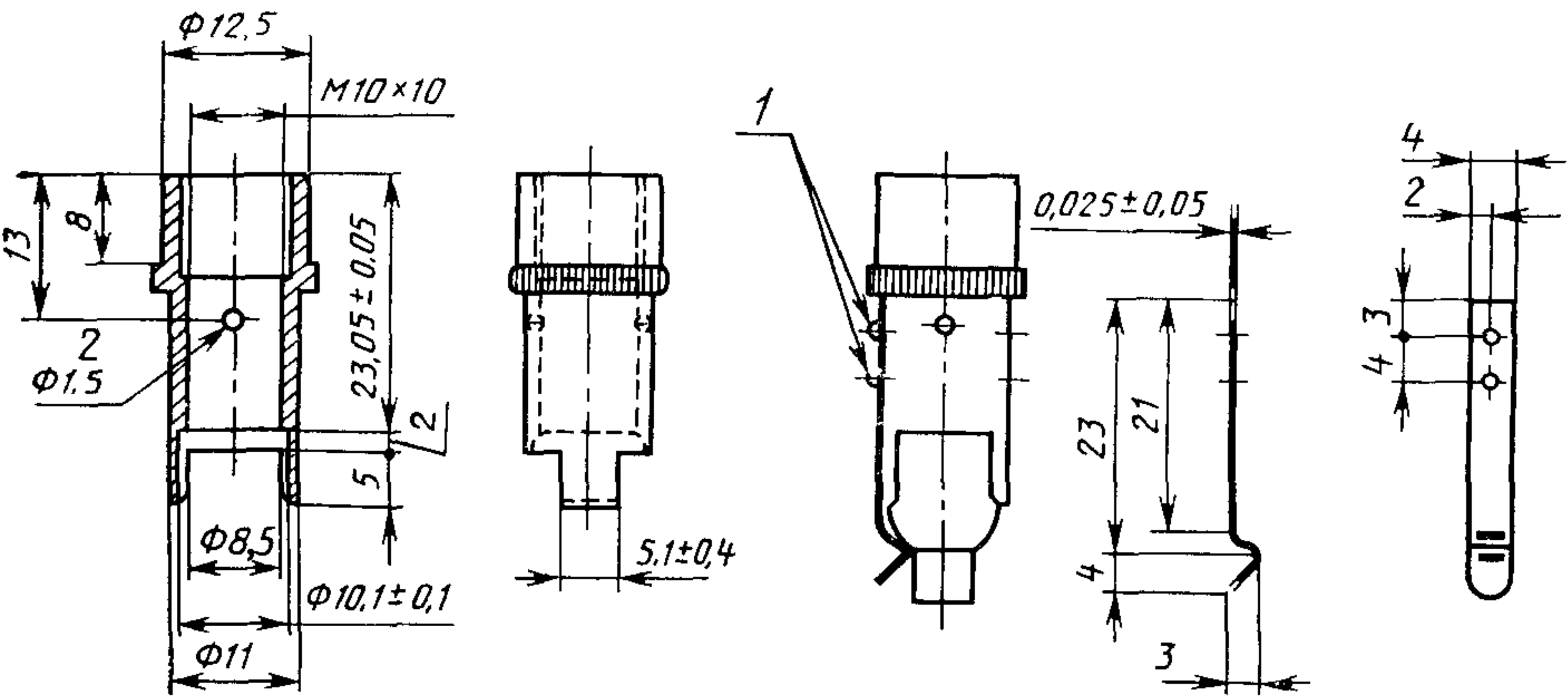
1 — наклейки или винты; 2 — отверстие Рисунок 5 — Корпус
