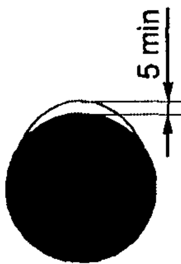
Рисунок А.1б — Чрезмерный слой пыли, имеющий температуру самовоспламенения менее 250 °С, на верхней поверхности оборудования
