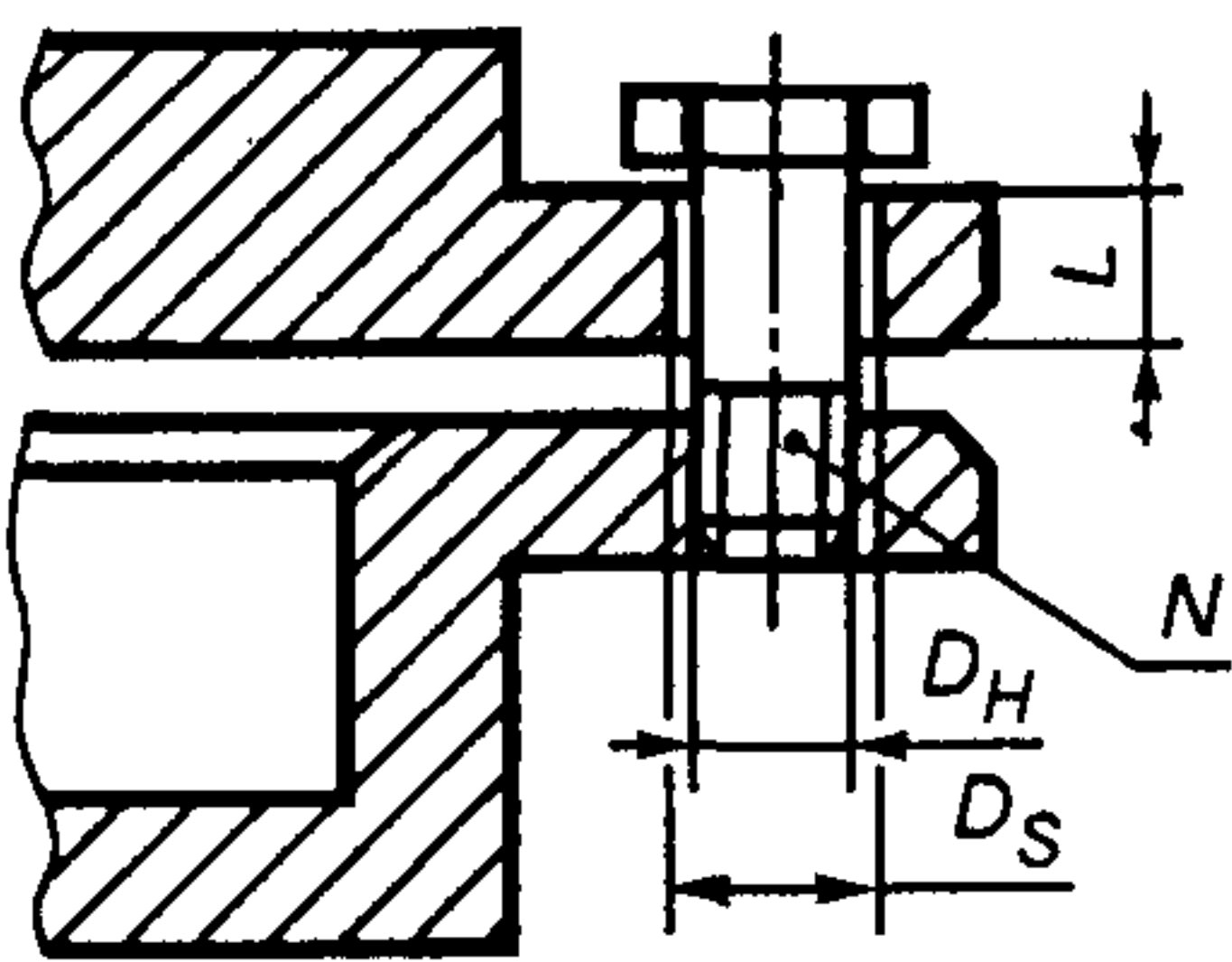
Рисунок 6 — Промежуток в болтовом отверстии
