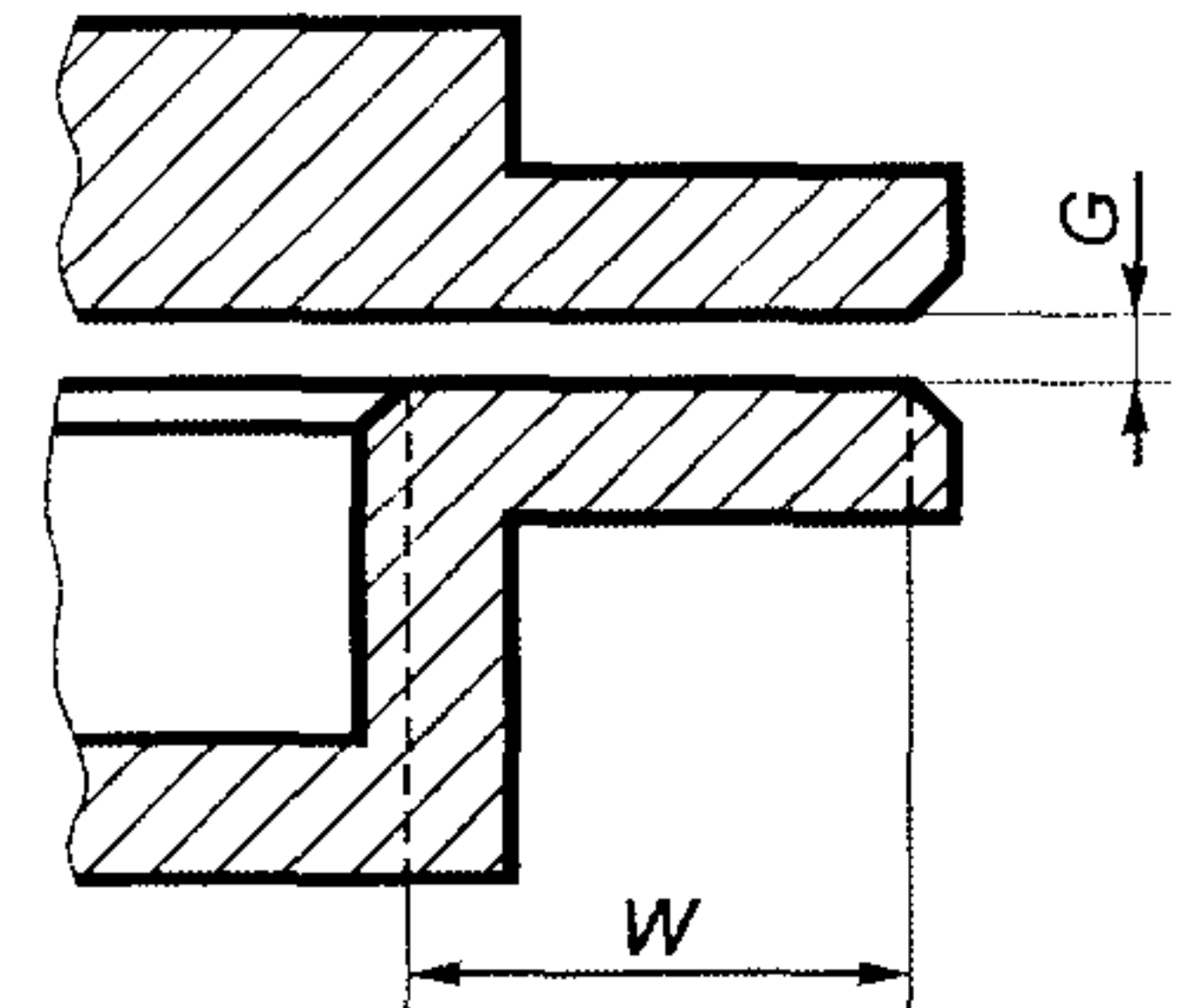
Рисунок 2 — Плоское соединение
