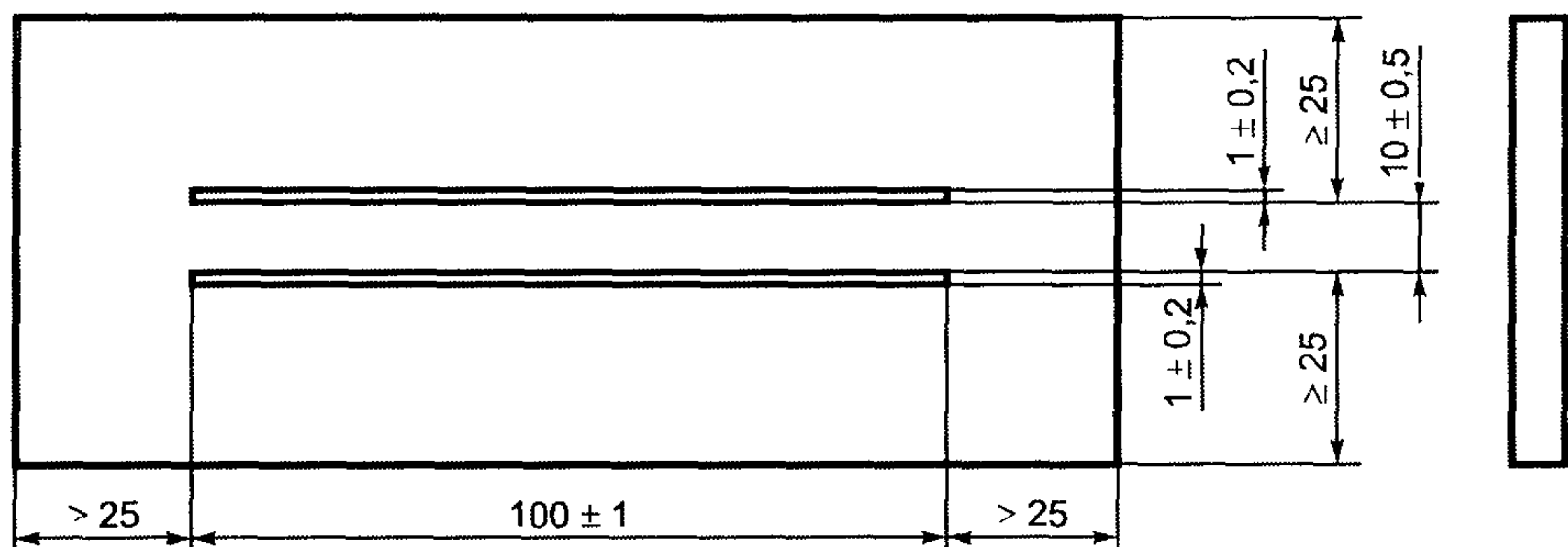
Рисунок 7 — Испытуемый образец с электродами
