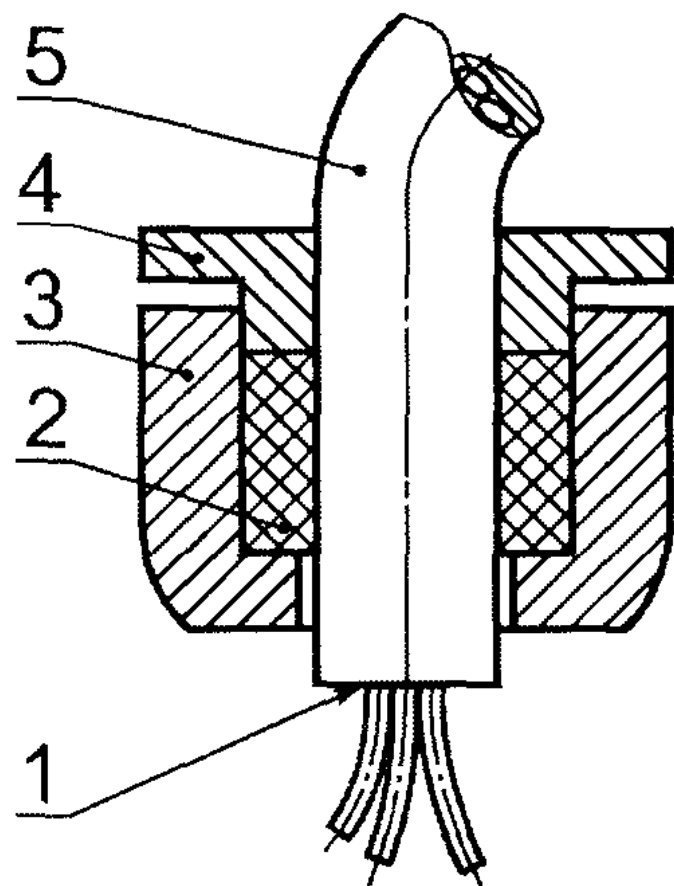
1 — место перехода проводов; 2 — уплотняющие кольцо; 3 — корпус кабельного ввода; 4 — зажимное кольцо с кольцевым ободком; 5 — кабель
