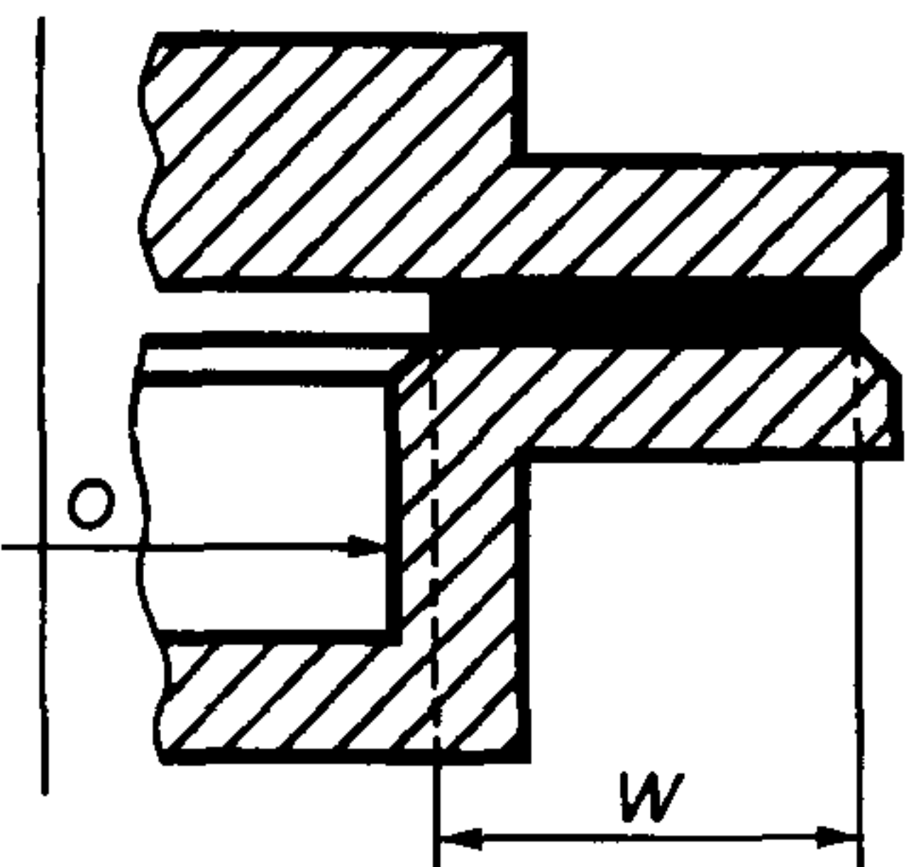
Рисунок 4 — Соединение с прокладкой
