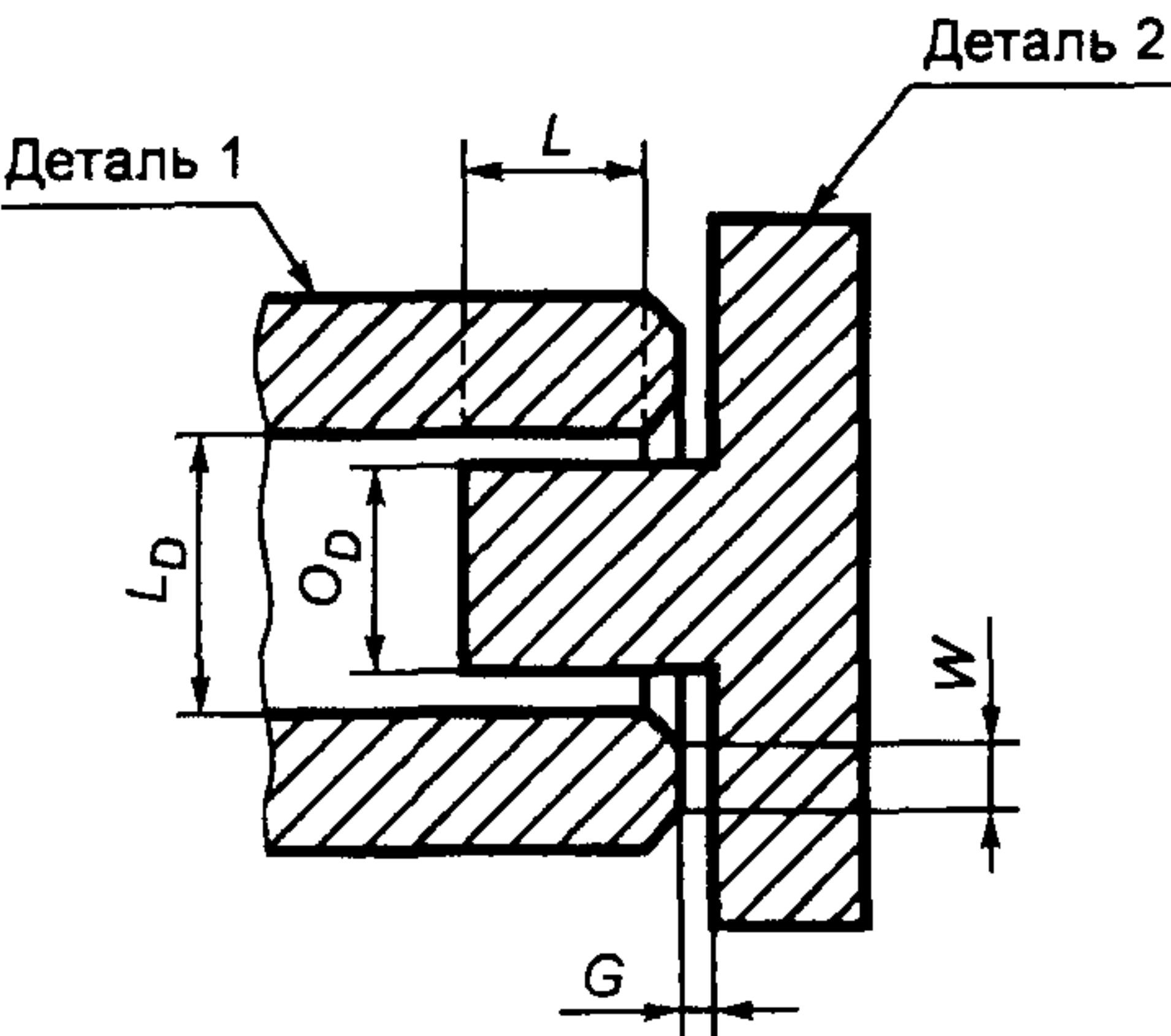
Рисунок 3 — Цилиндрическое соединение
