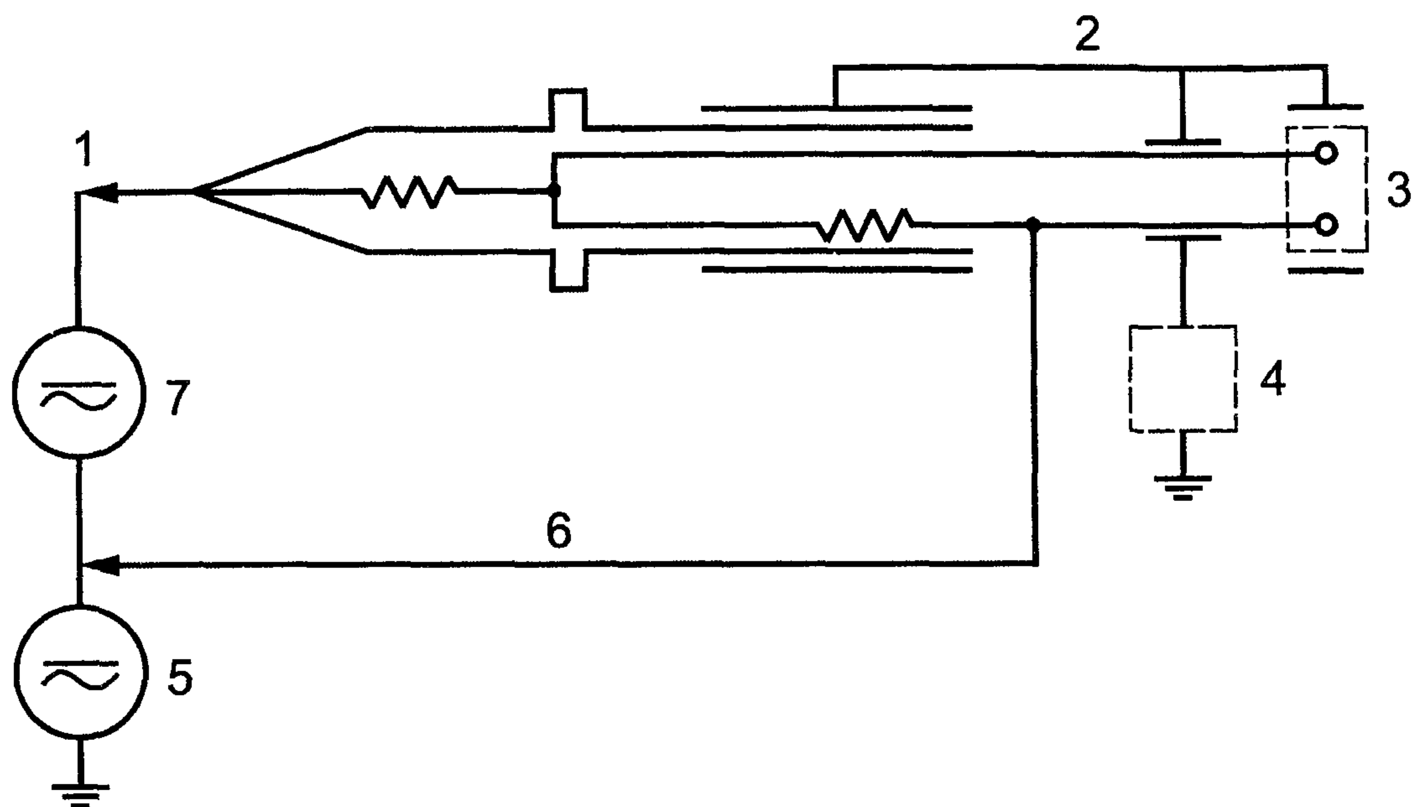
1 — наконечник щупа; 2 — металлическая фольга (см. рисунок 105); 3 — контрольно-измерительный прибор или электрическое оборудование или эквивалентный импеданс; 4 — схема измерения допустимой силы тока (см. рисунок А.1); 5 — источник максимального номинального напряжения опорного соединителя; 6 — опорный соединитель (если предусмотрен); 7 — источник максимального номинального напряжения
