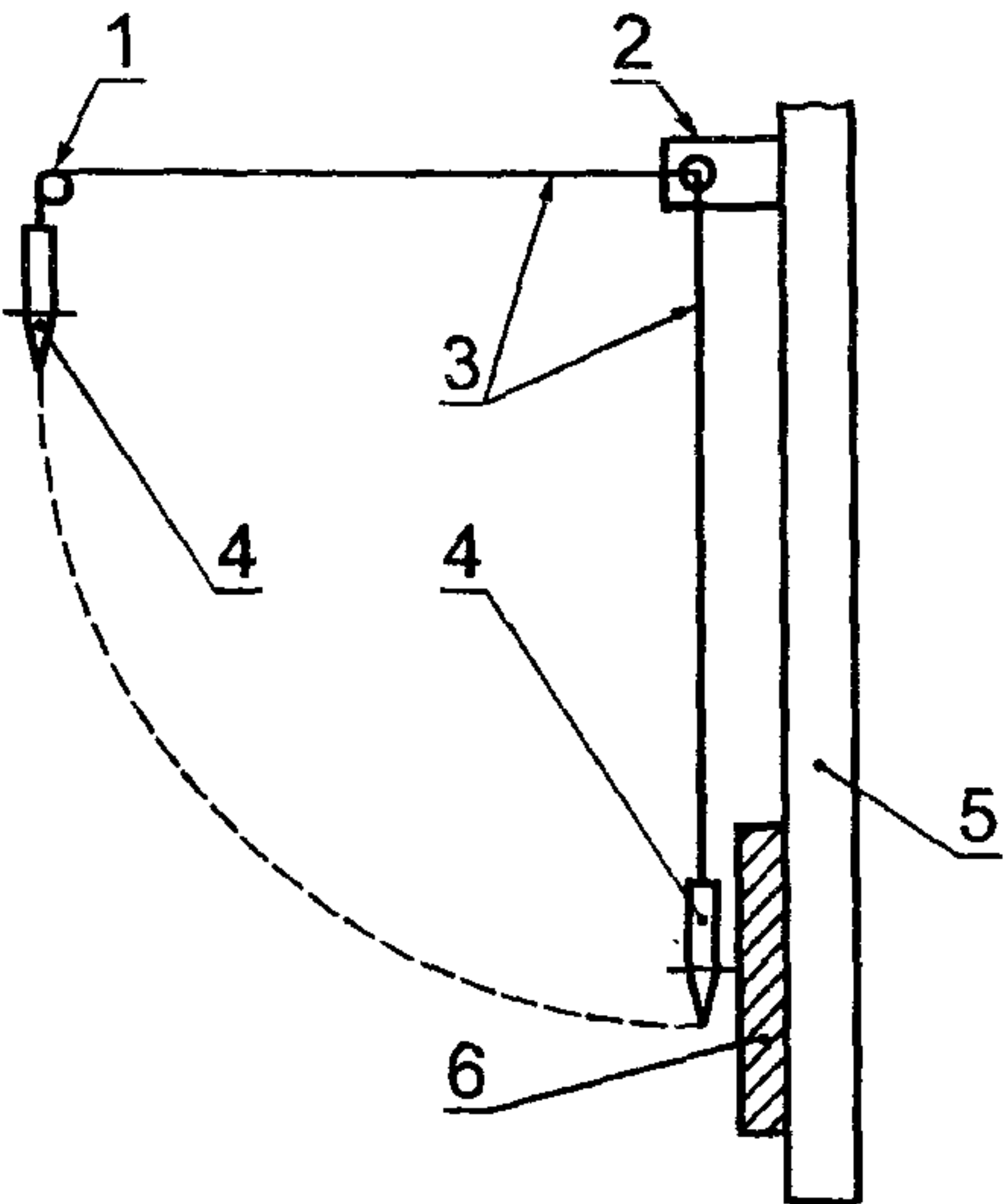
1 — исходная точка; 2 — точка крепления; 3 — шнур; 4 — электрический щуп; 5 — стена; 6 — доска из твердых пород дерева
