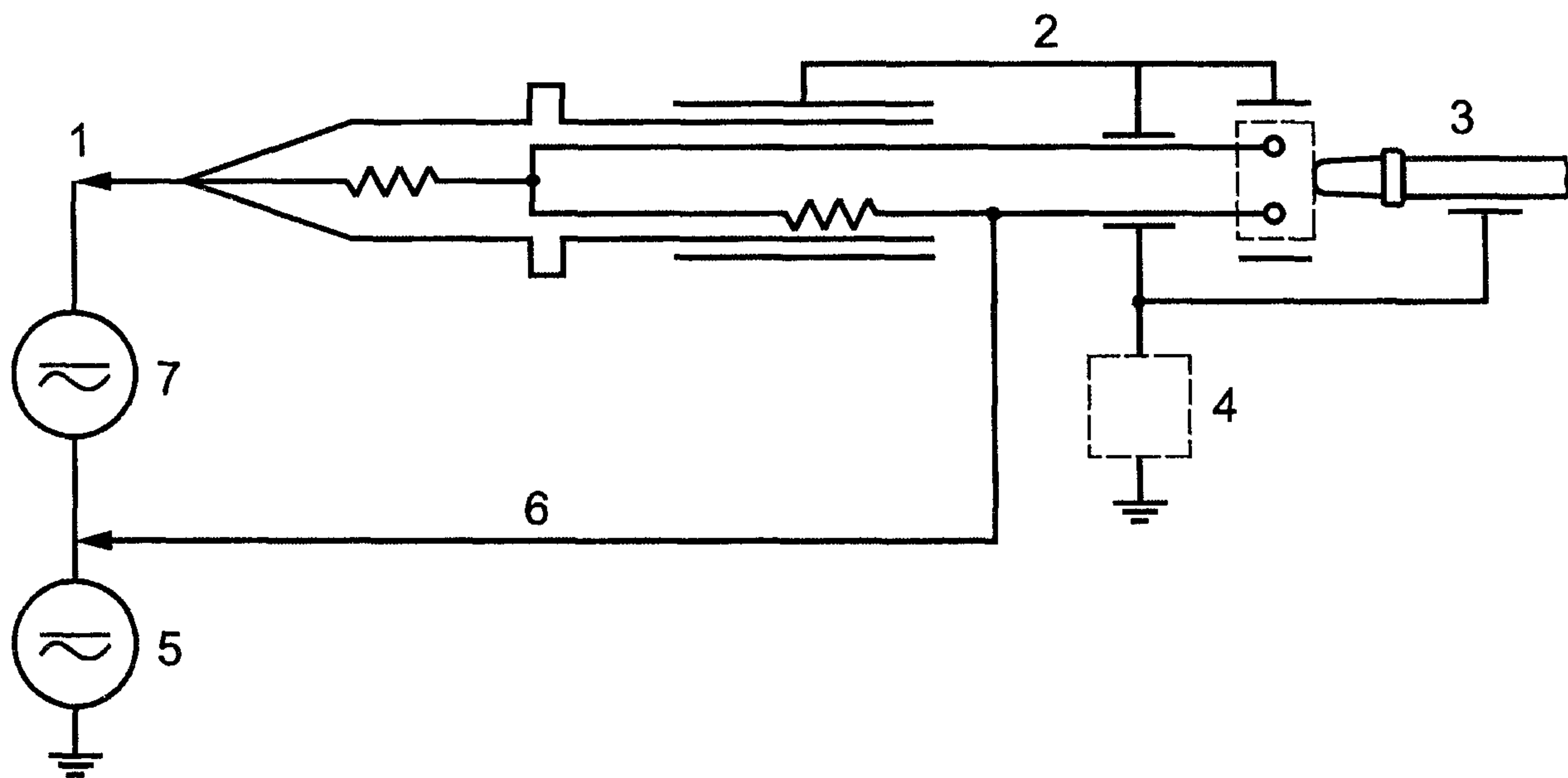
1 — наконечник щупа; 2 — металлическая фольга (см. рисунок 105); 3 — электрод, форма и размер которого те же, что у испытательного пальца; 4 — схема измерения допустимой силы тока (см. рисунок А.1); 5 — источник максимального номинального напряжения опорного соединителя; 6 — опорный соединитель (если предусмотрен); 7 — источник максимального номинального напряжения
