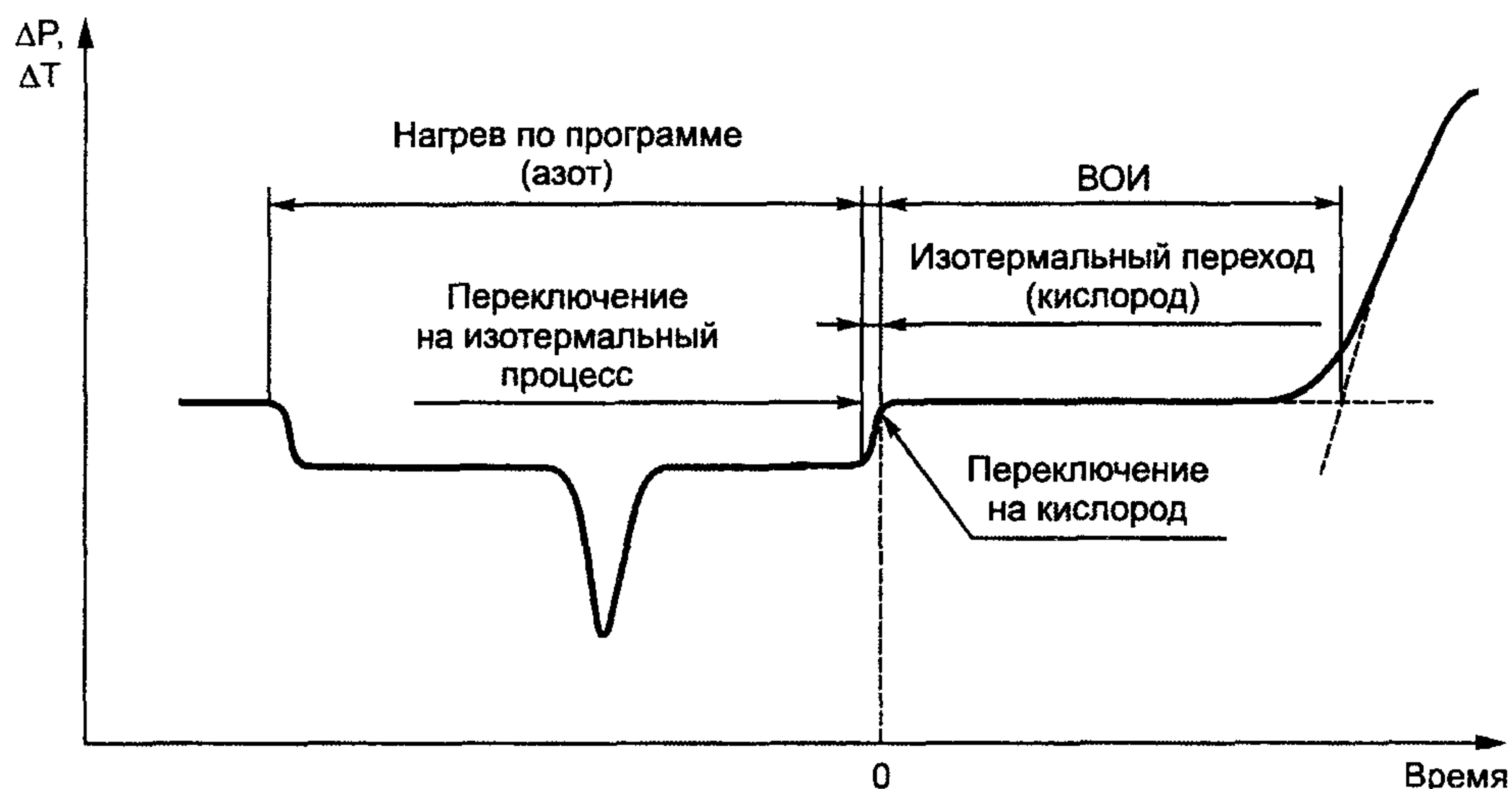
Рисунок В.2 — Определение ВОИ по термограмме
