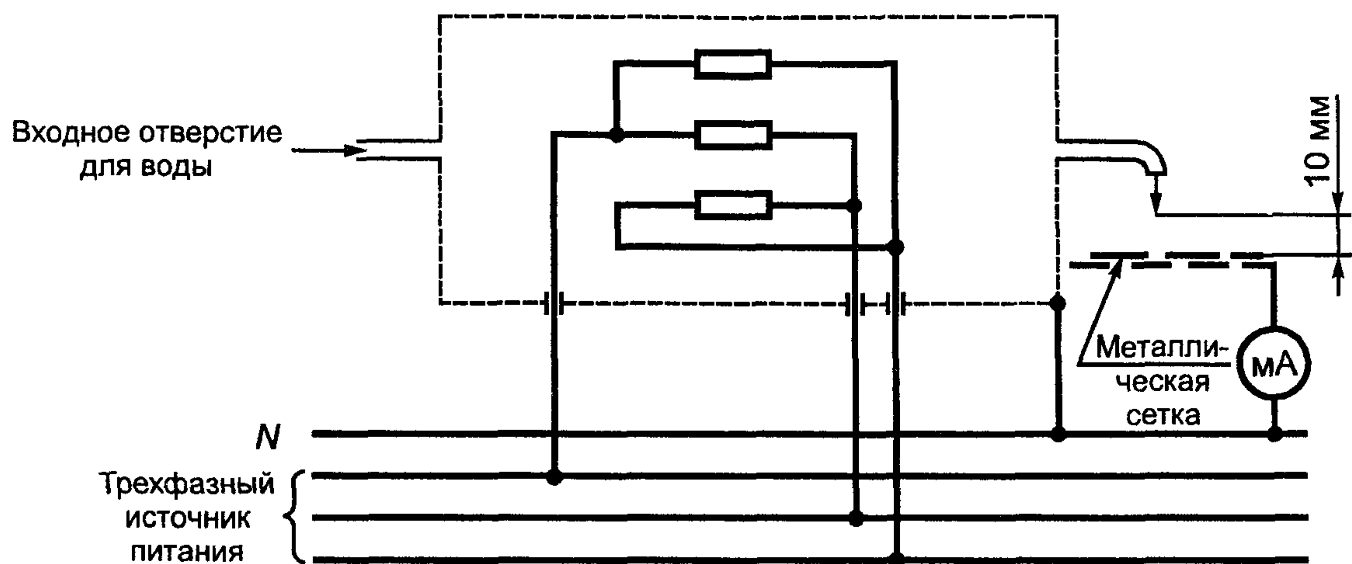
Рисунок 102 — Схема дополнительного измерения тока утечки при рабочей температуре для трехфазных водонагревателей класса I с открытым элементом
