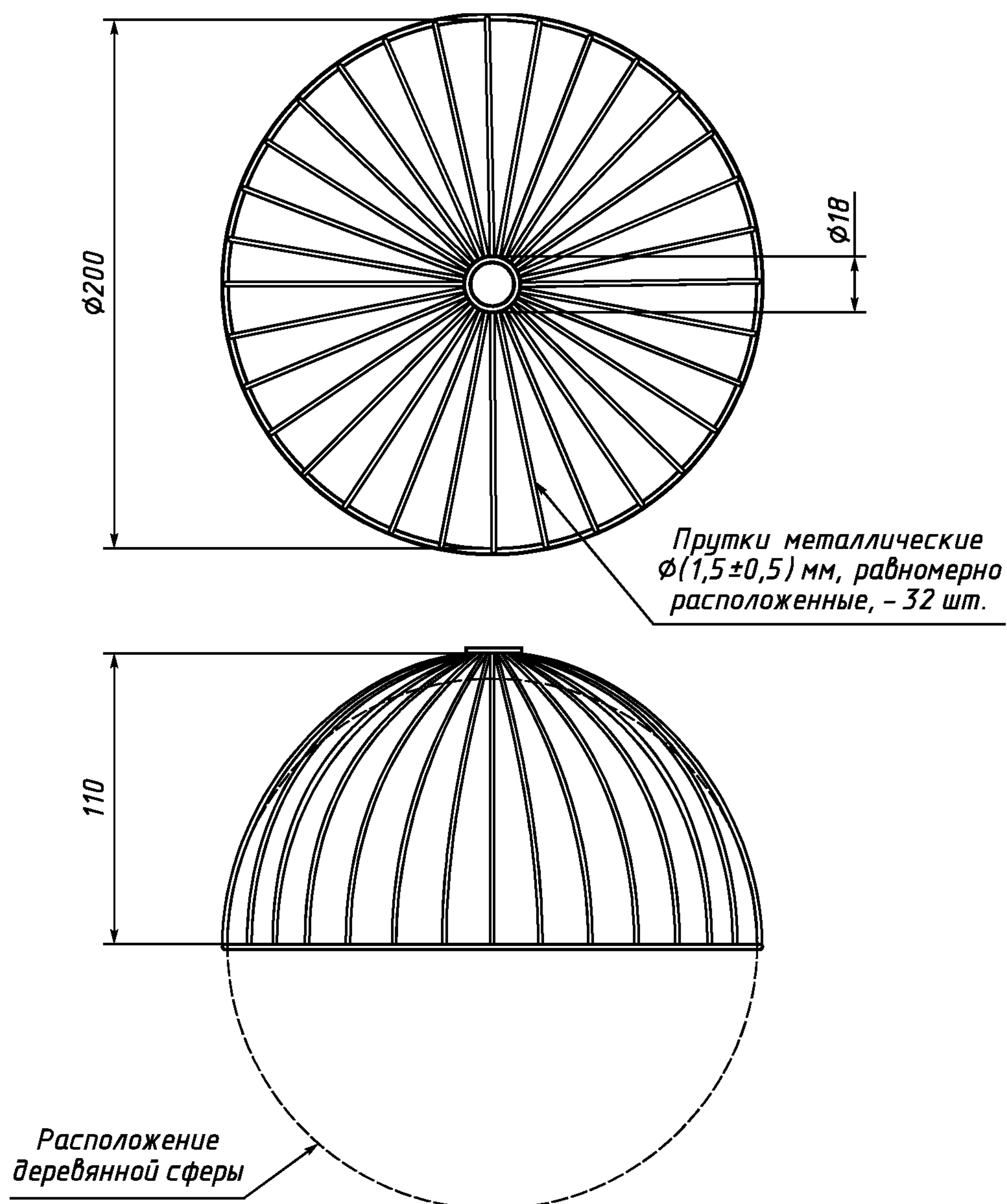
Рисунок 101 — Защитная решетка из металлических прутков
