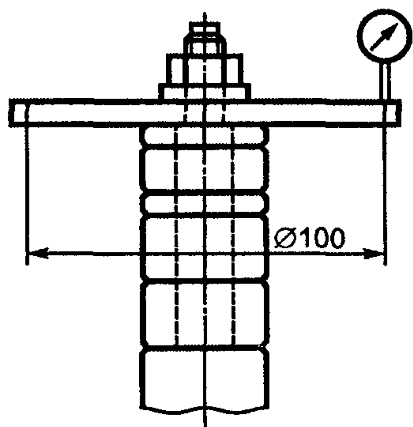
Рисунок 103 — Испытание на биение дистанционных колец шпинделя
