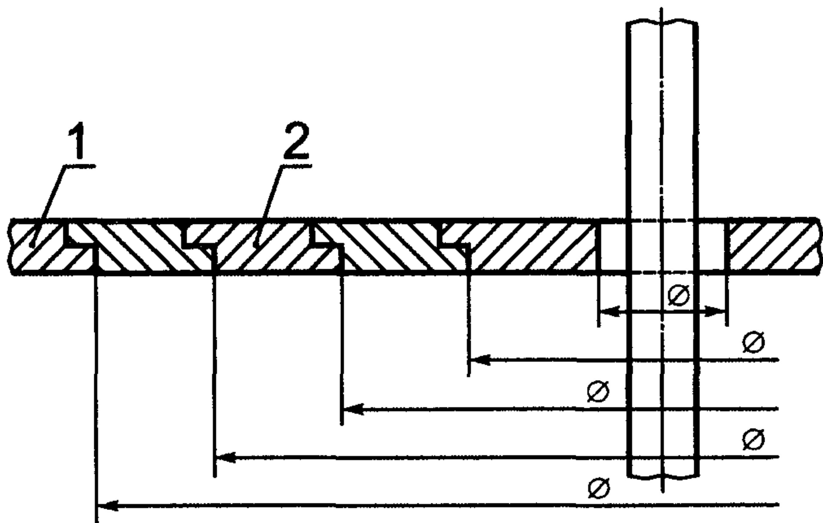
1 — стол; 2 — вставка стола
