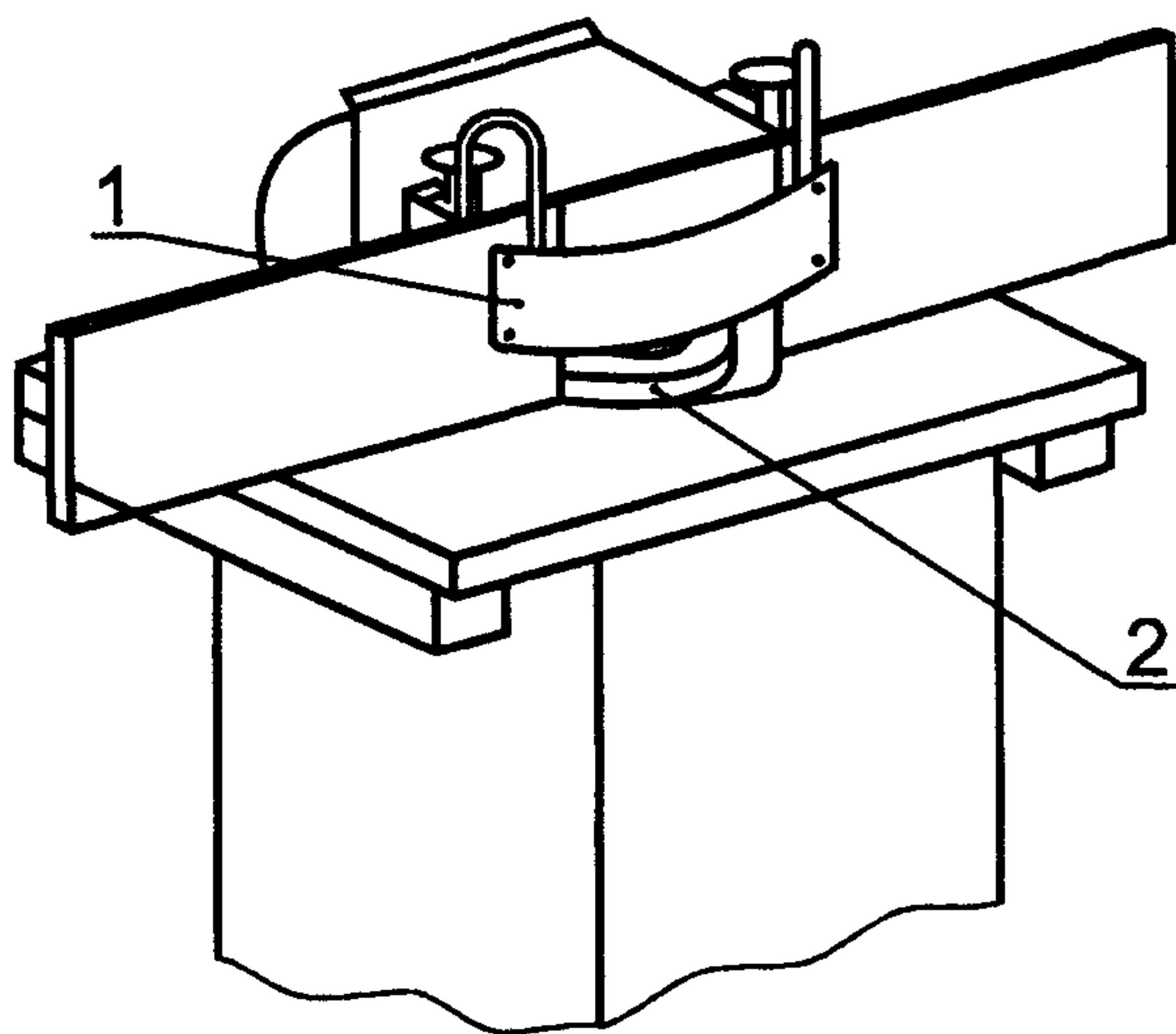
1 — защитный кожух; 2 — режущий узел
