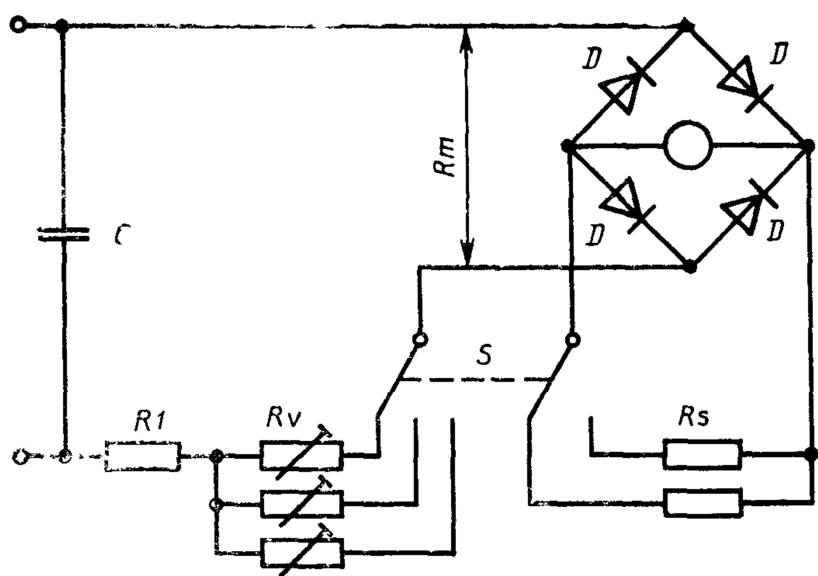
Рисунок 1A1 — Схема цепи для измерения тока утечки
