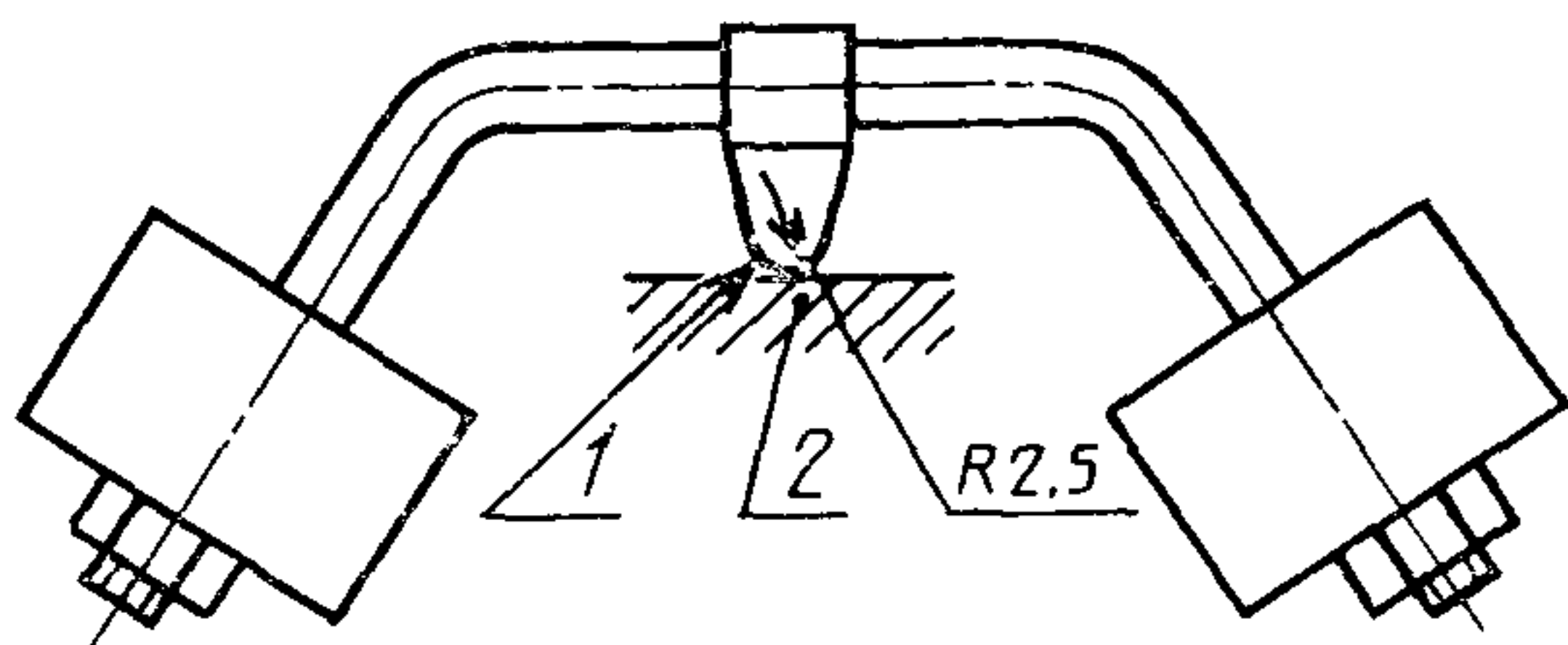
1—сферическая часть; 2—образец
