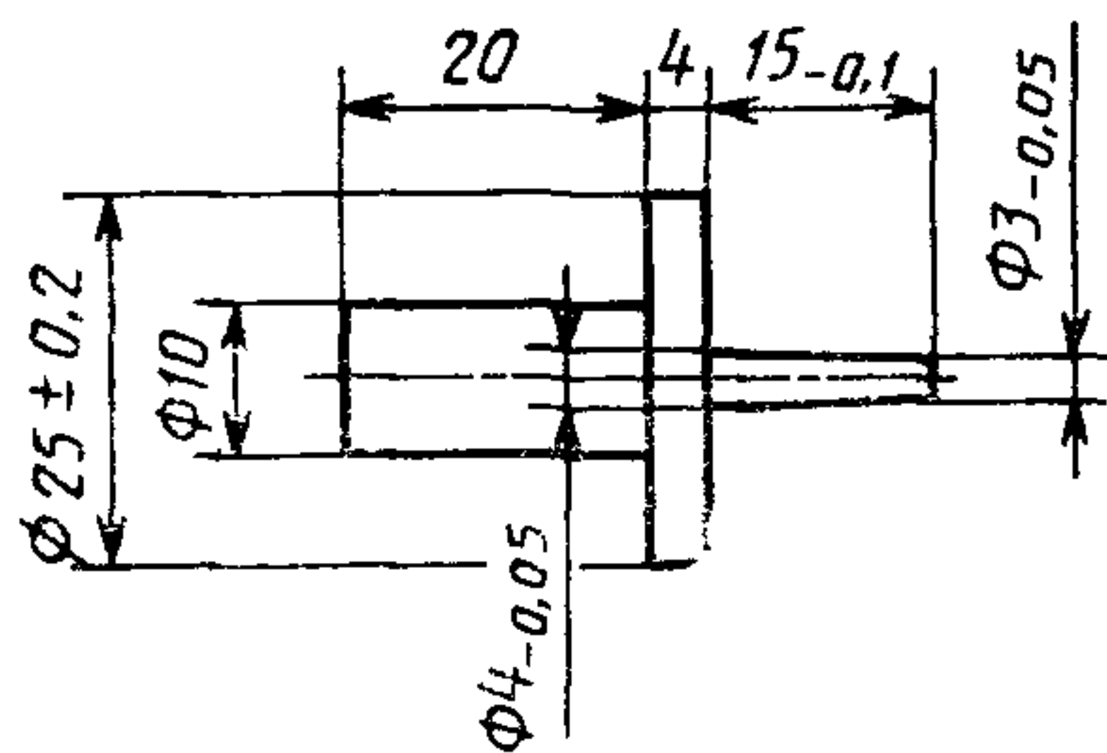
Рисунок 2 — Испытательный щуп
