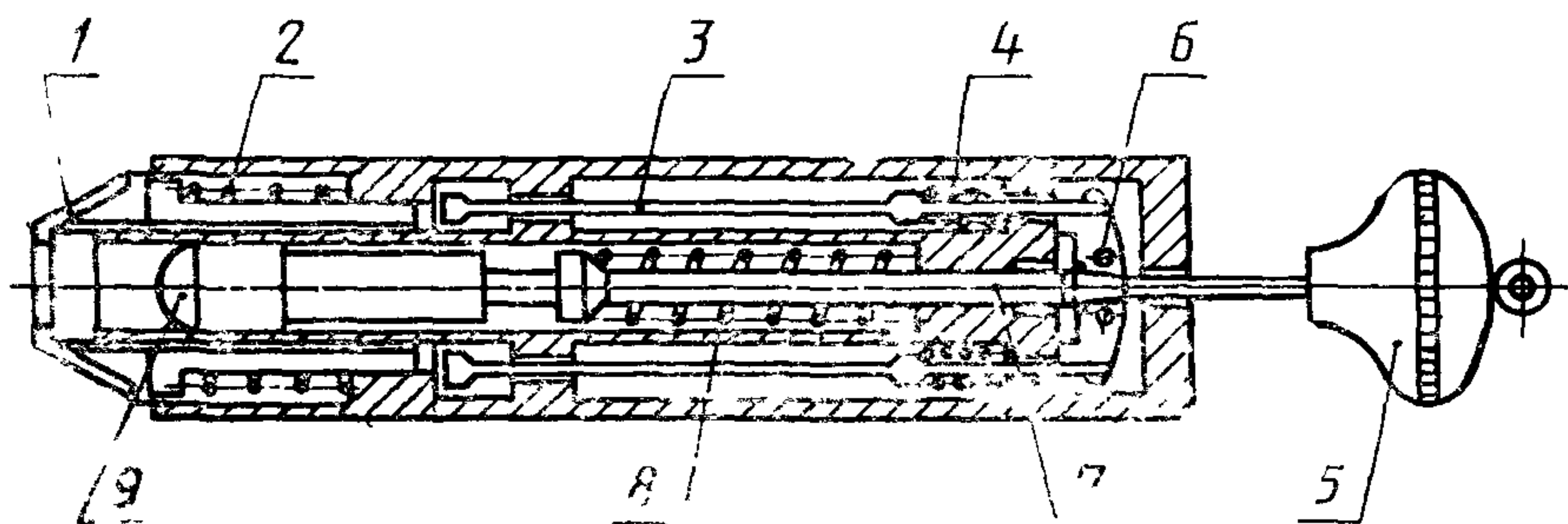
1—спусковой конус; 2—пружина конуса; 3—стержень спускового механизма; 4—пружина спускового механизма; 5—натяжная кнопка; 6—спусковой зажим; 7—стержень ударника; 8—пружина ударника; 9—головка ударника
