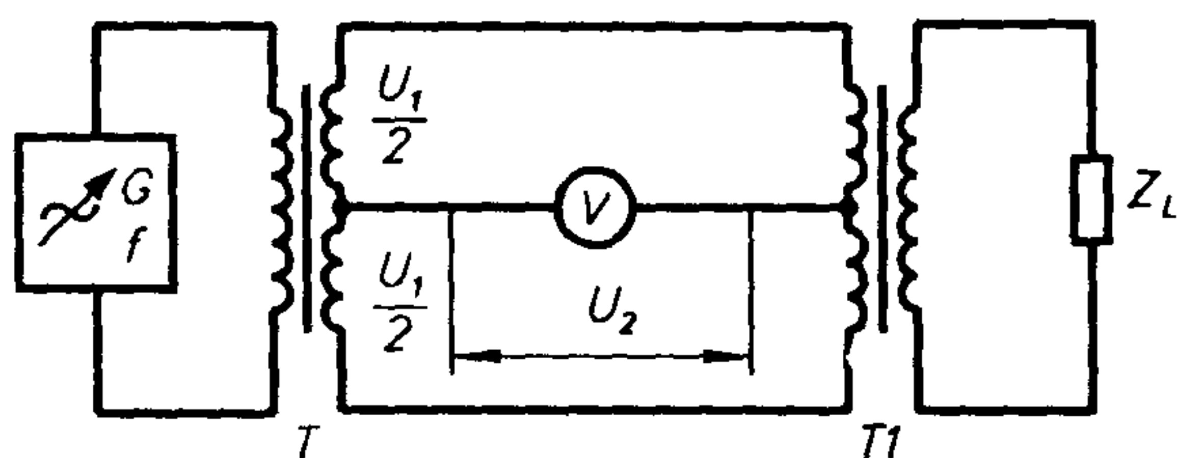
T1 — испытуемый трансформатор
