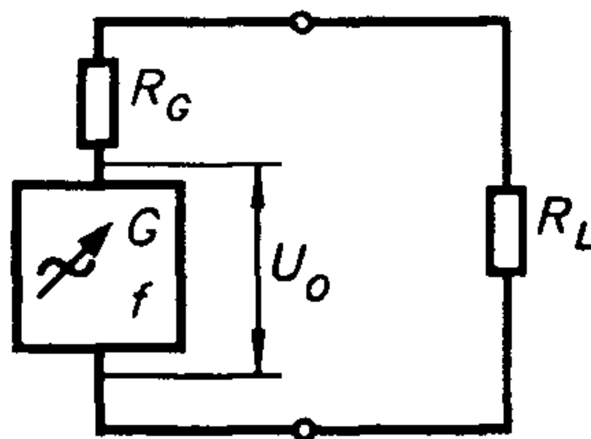
Рисунок 17 — Иллюстрация потерь от несогласования
