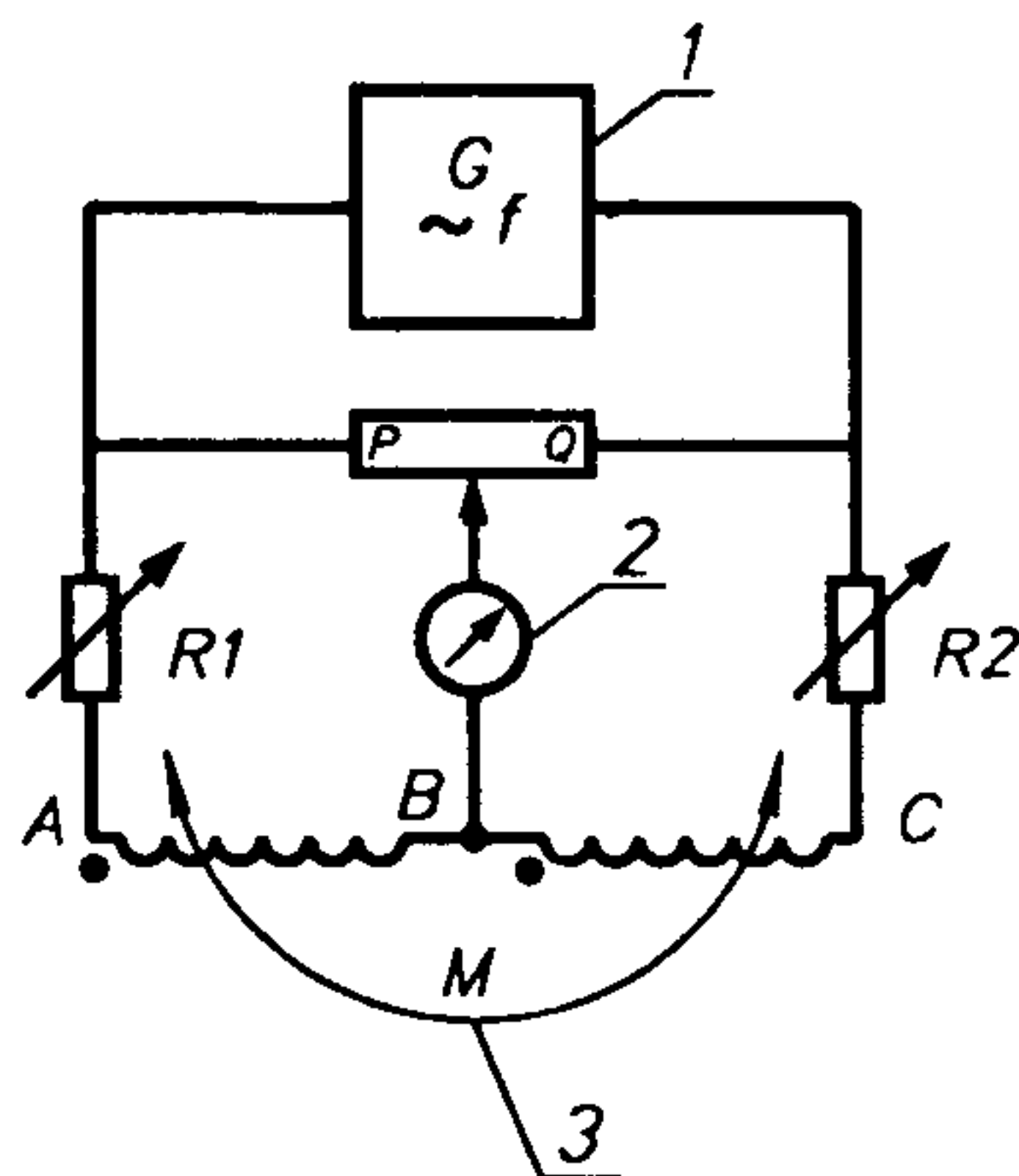
P и Q — декадные элементы чисто омического сопротивления; R1 и R2 — переменные резисторы с чисто омическим сопротивлением; 1 — симметричный источник питания; 2 — детектор с высоким импедансом; 3 — испытуемый компонент.
