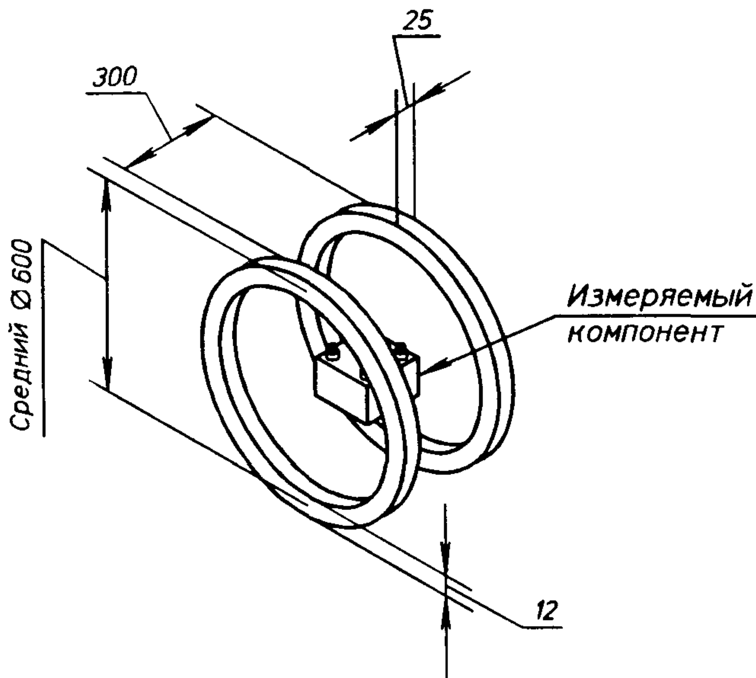
Рисунок 22 — Кольца Гельмгольца
