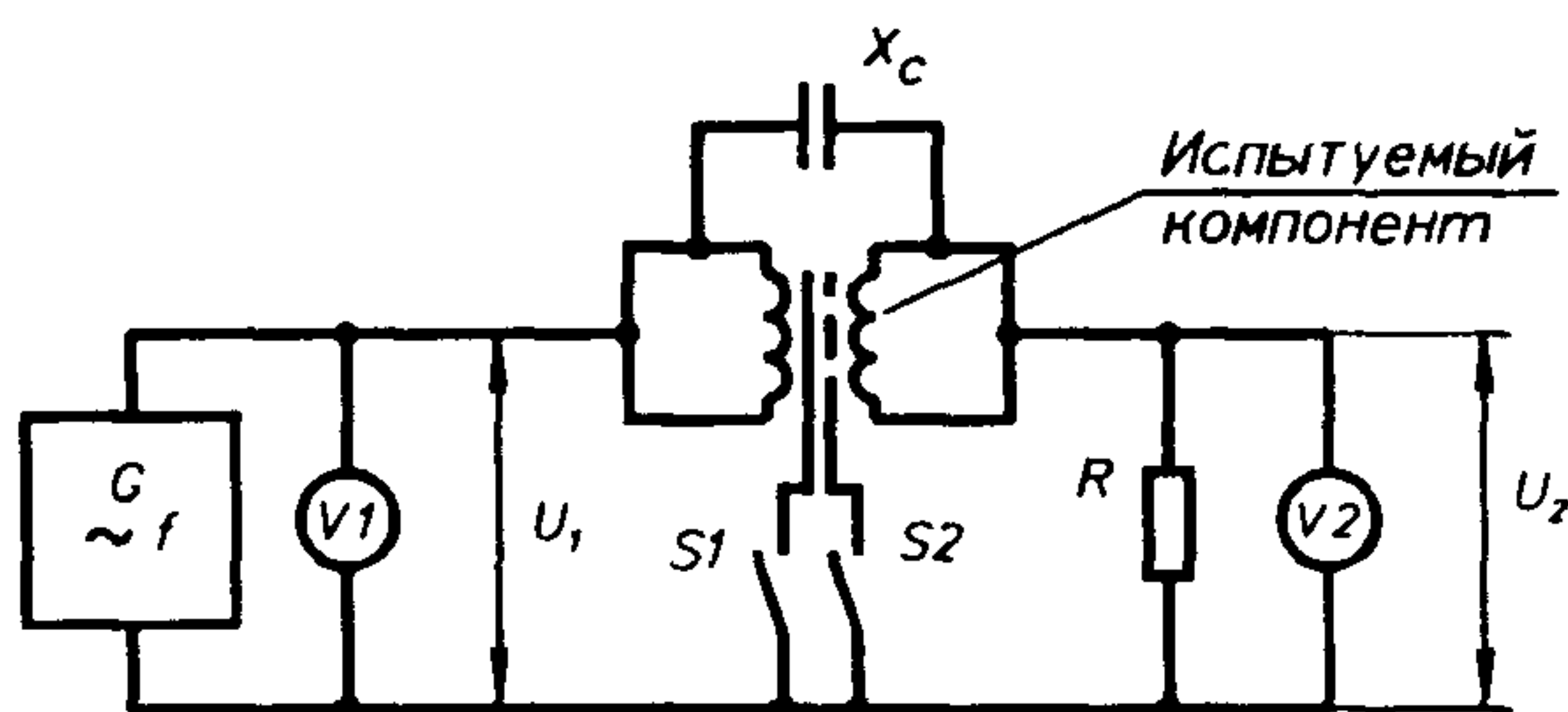
Рисунок 10 — Схема для определения межобмоточной емкости
