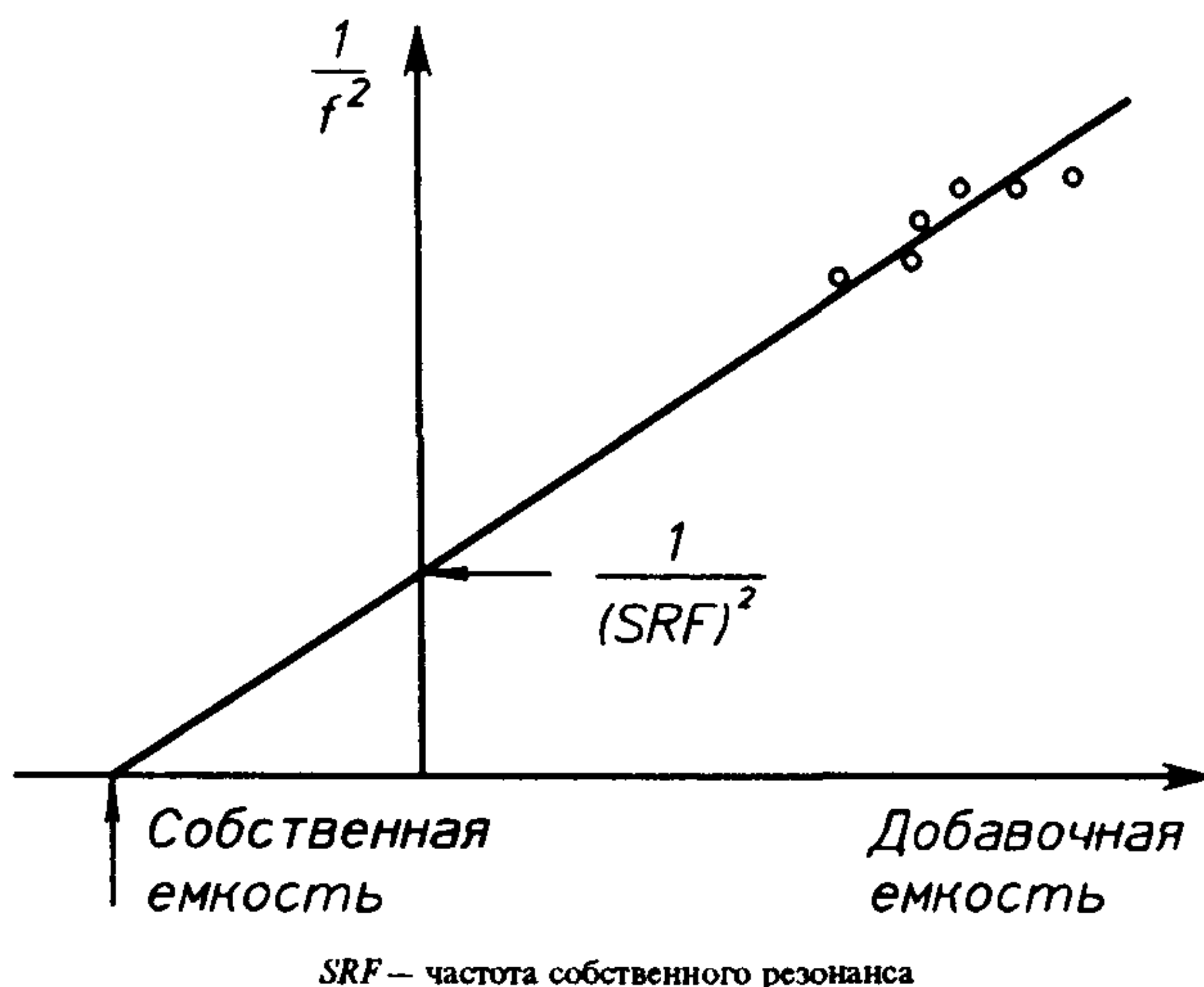
Рисунок 9 — Типичный график для определения собственной емкости
