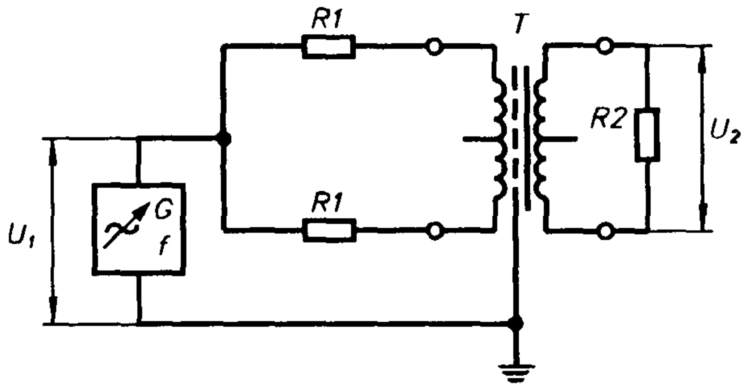
T — испытуемый трансформатор
