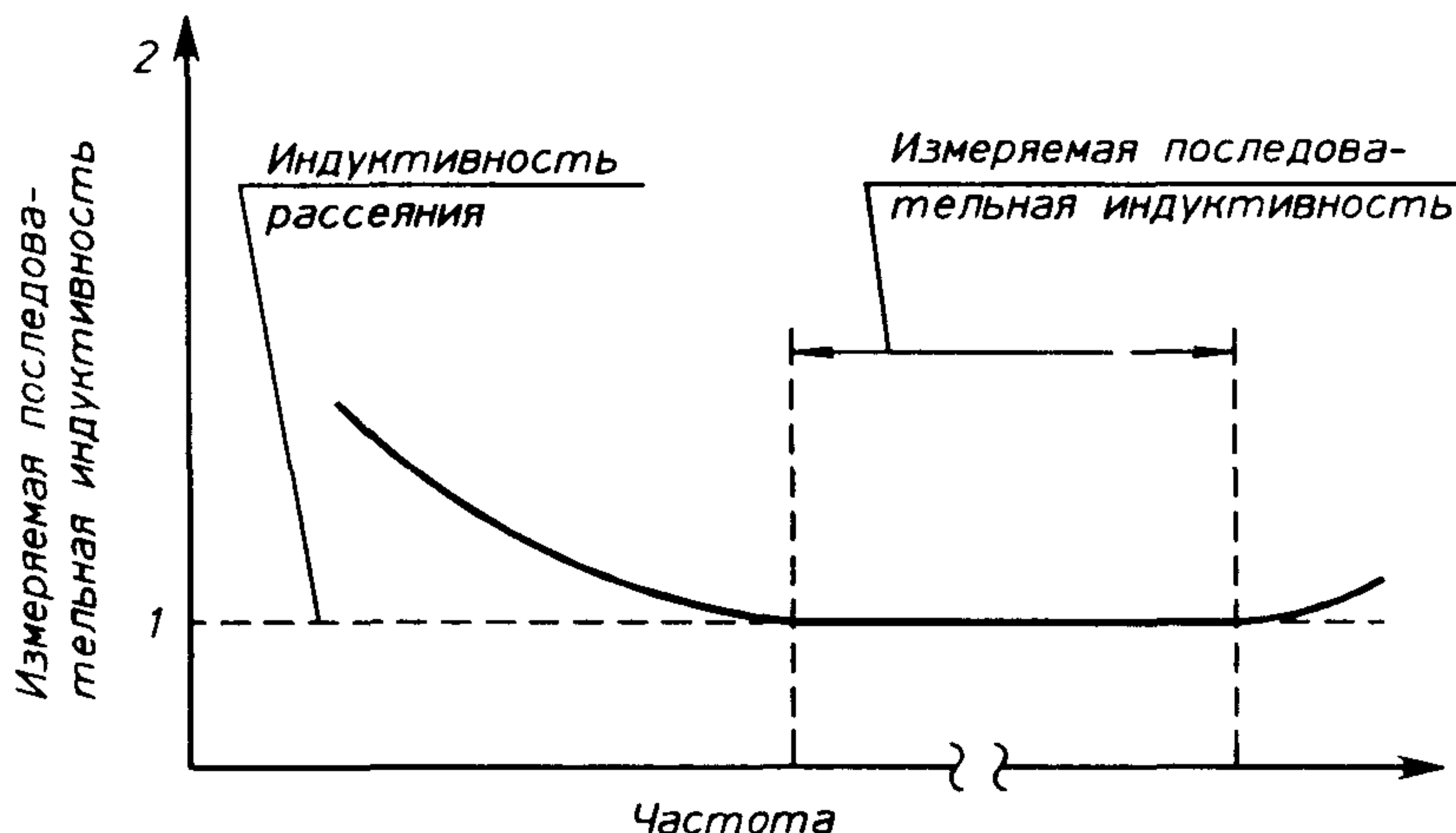
Рисунок 4 — Зависимость измеряемой последовательной индуктивности от частоты
