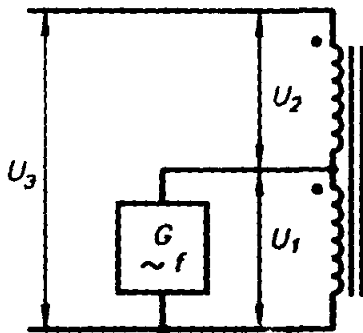
Рисунок 21 — Проверка фаз (полярности) путем измерения напряжений
