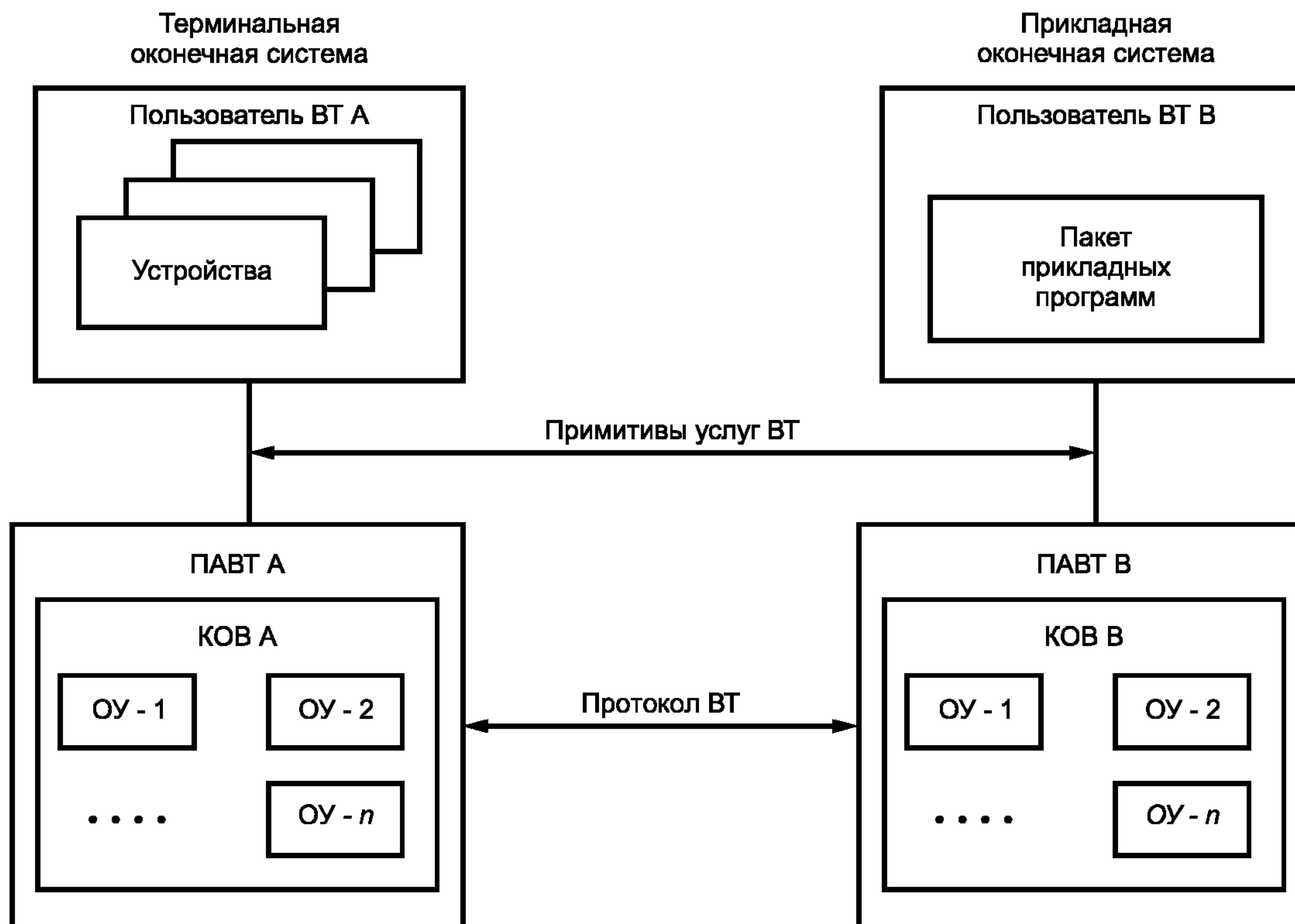
Рисунок 2 — Объекты управления в модели протокола ВТ
