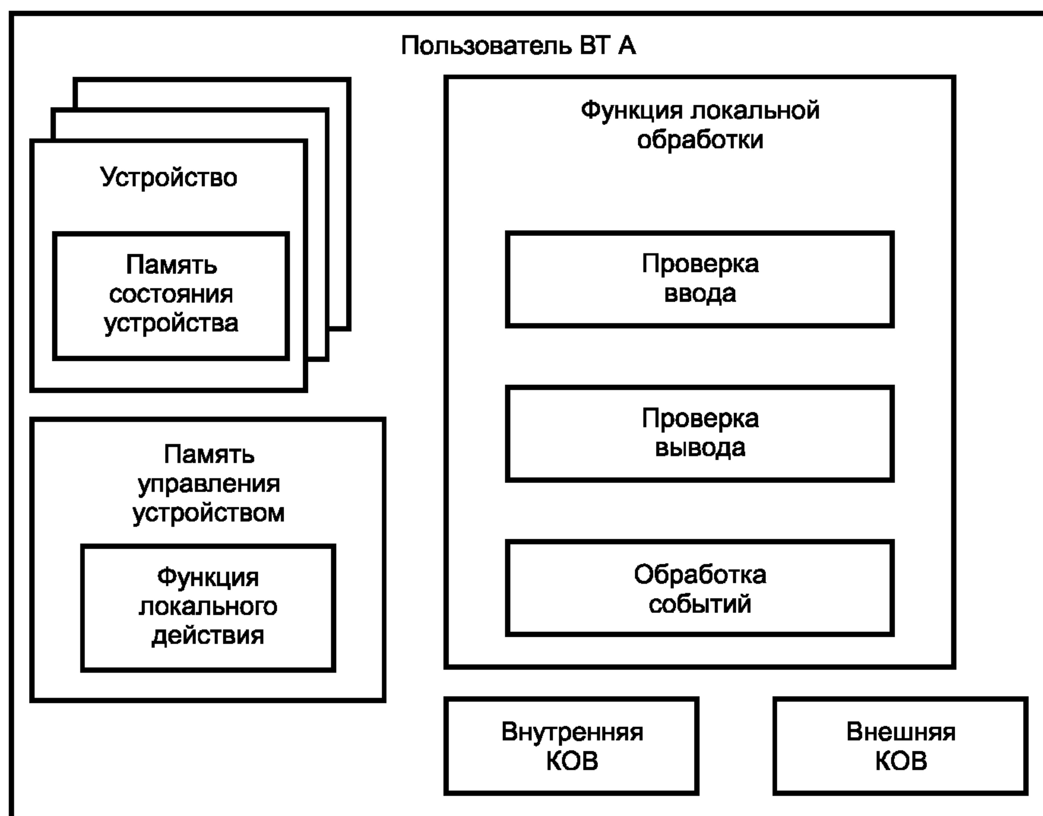
Рисунок 3 — Структура терминального пользователя ВТ
