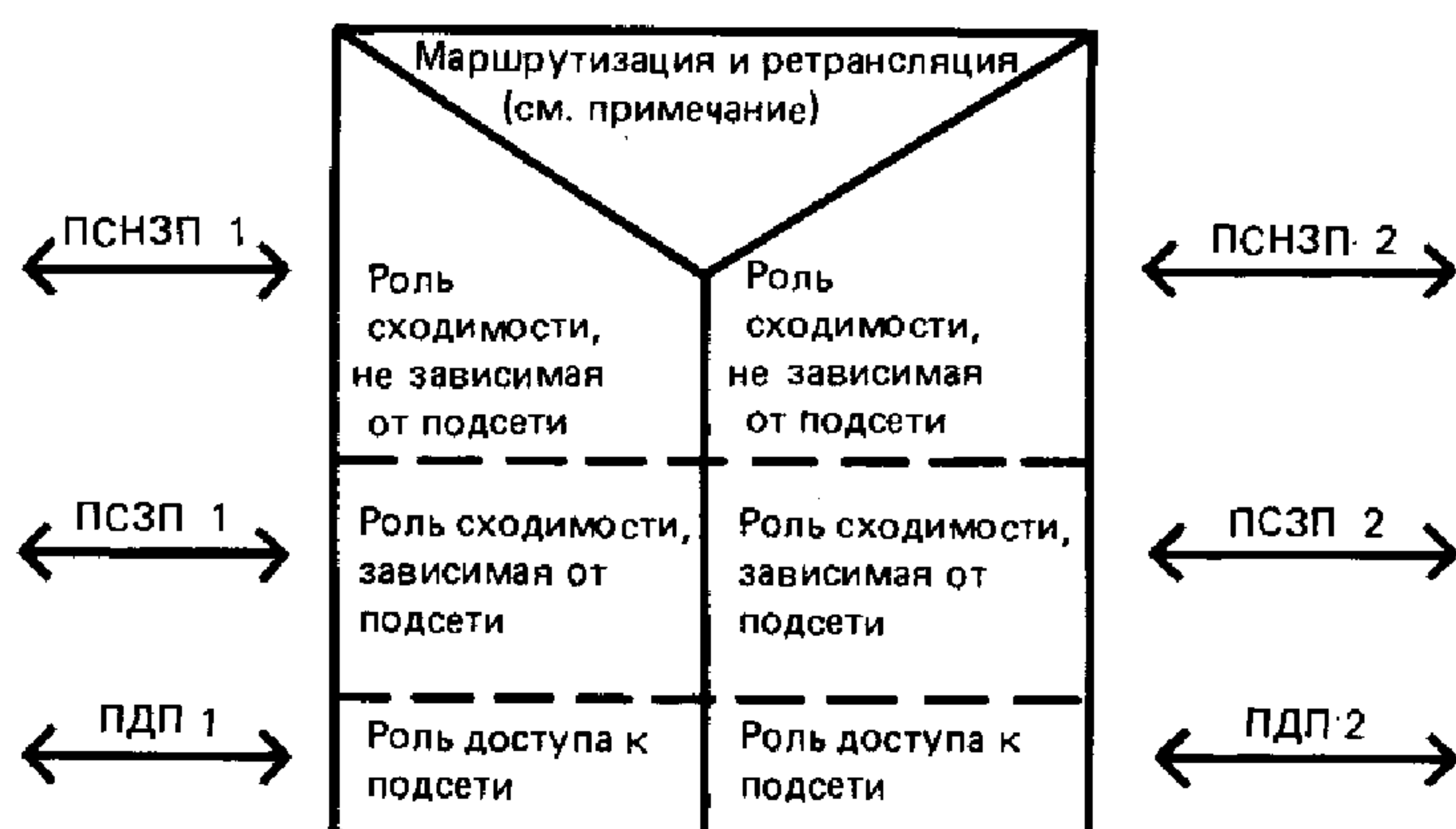
Рисунок 6 — Протокольные правила сетевого уровня
