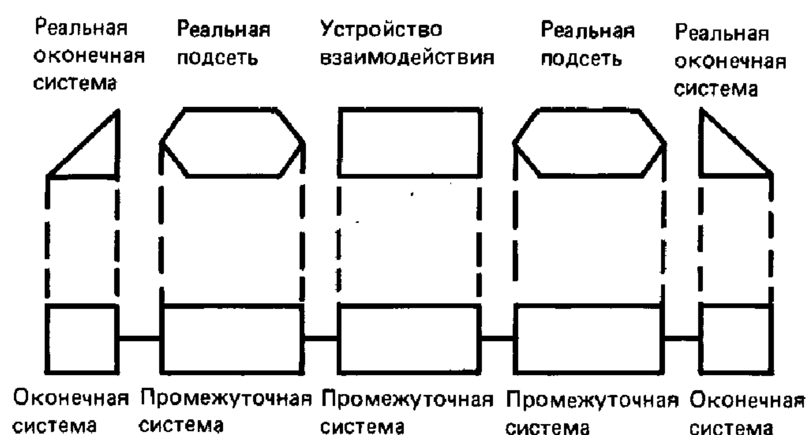
Рисунок 4 — Взаимосвязь реальных подсетей посредством отдельного устройства взаимодействия
