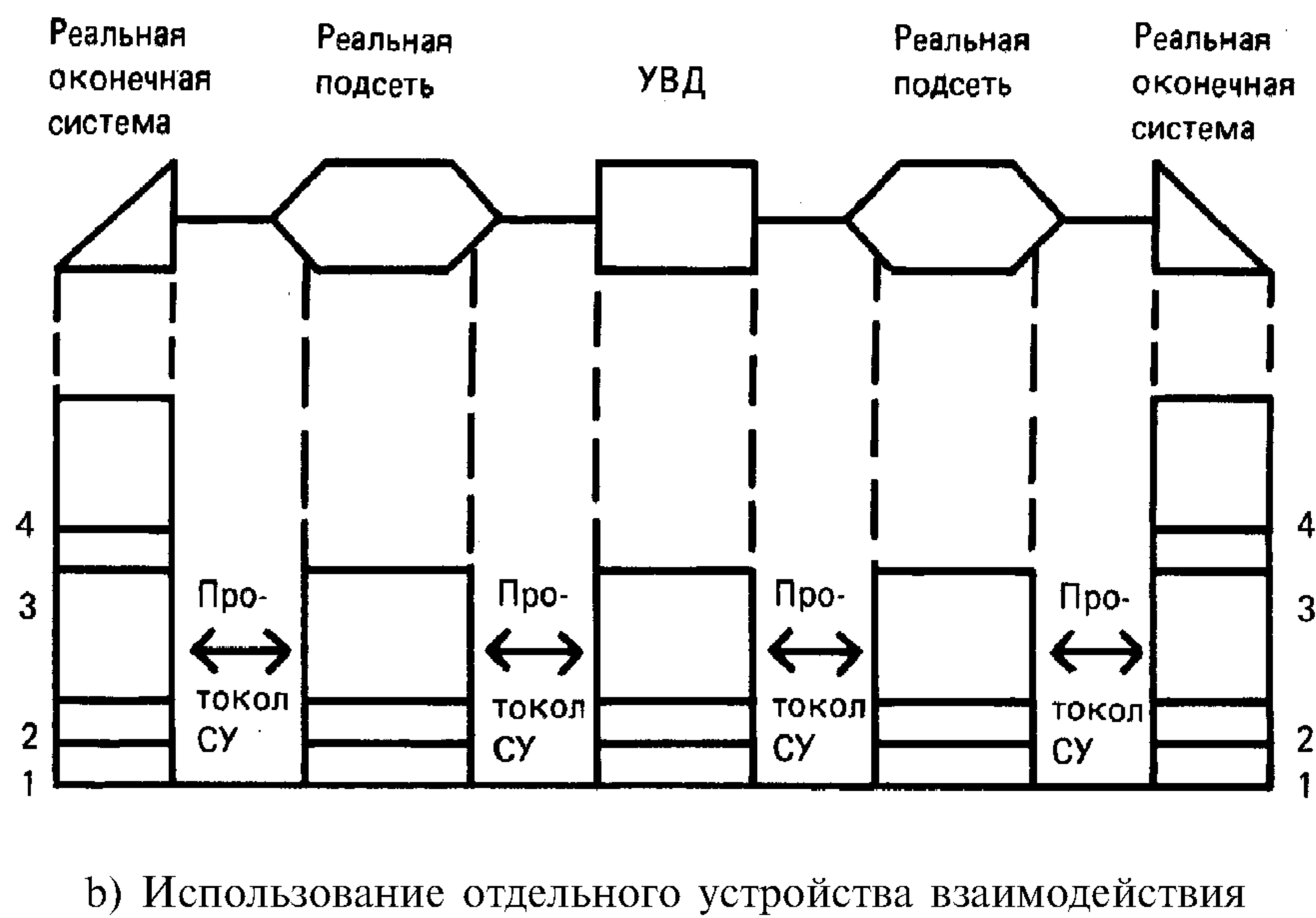
Рисунок 9 — Взаимосвязь подсетей, использующих один протокол сетевого уровня для обеспечения УСУ УС или УСУ БУС через две подсети УС или БУС
