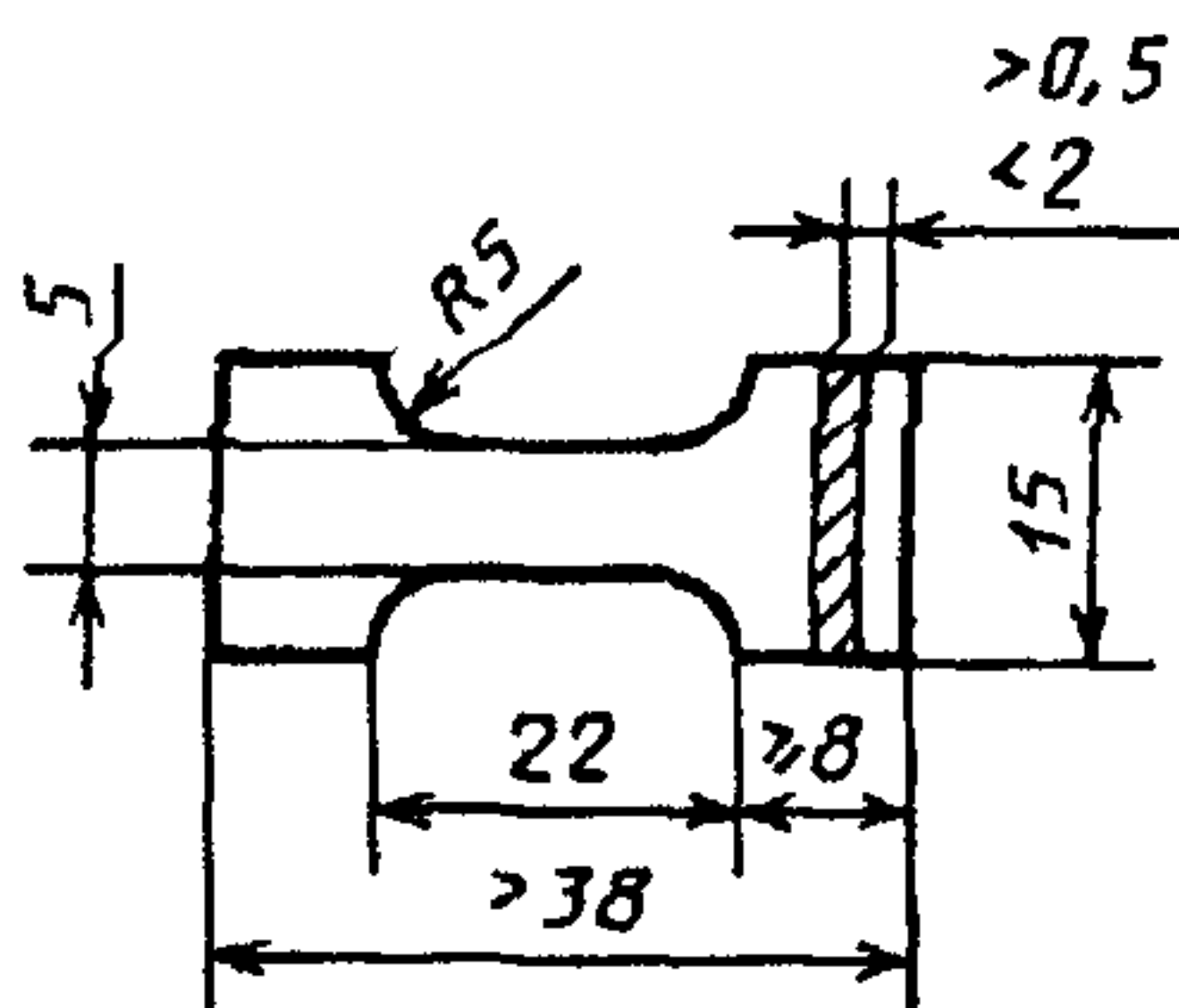
Рисунок 10 — Образец из ПТФЭ
