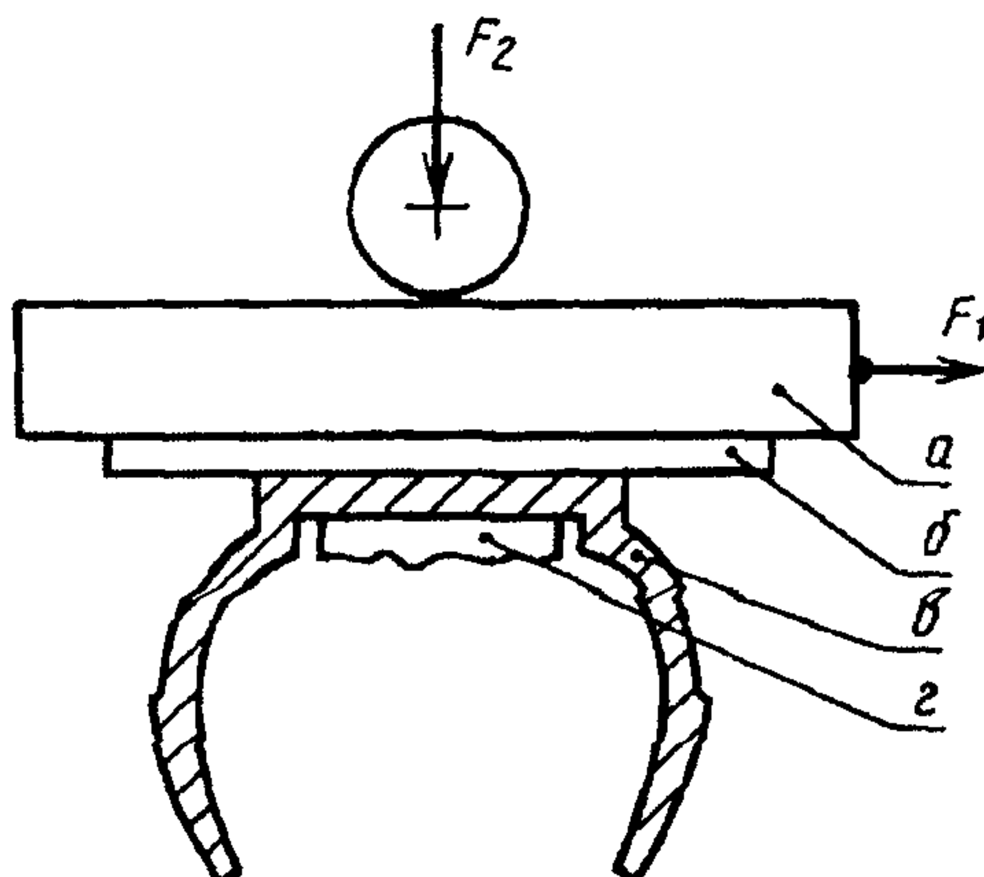
Рисунок 10 — Образец из ПТФЭ
