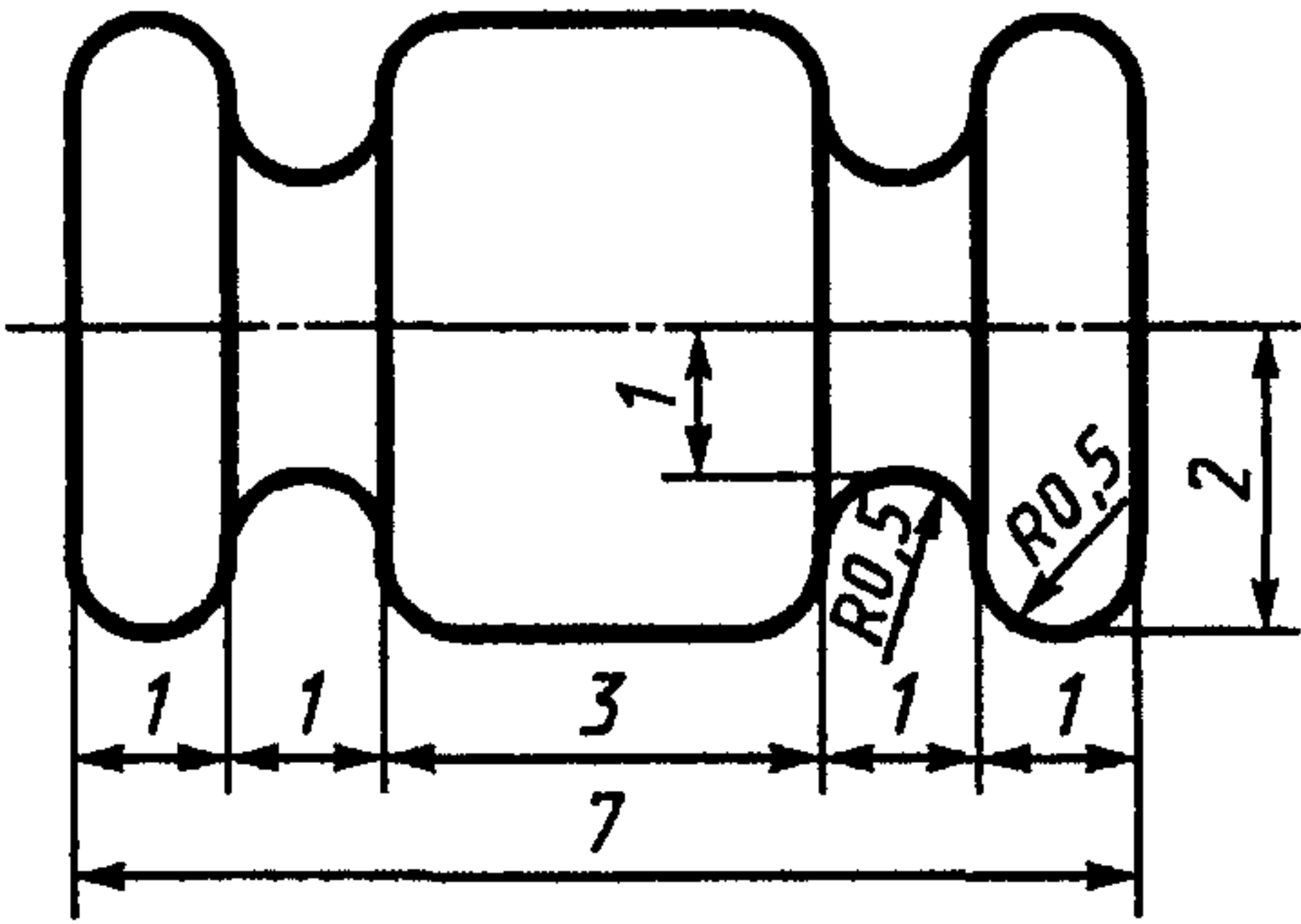
Рисунок Б.1 — Специальный цилиндр с пазами
