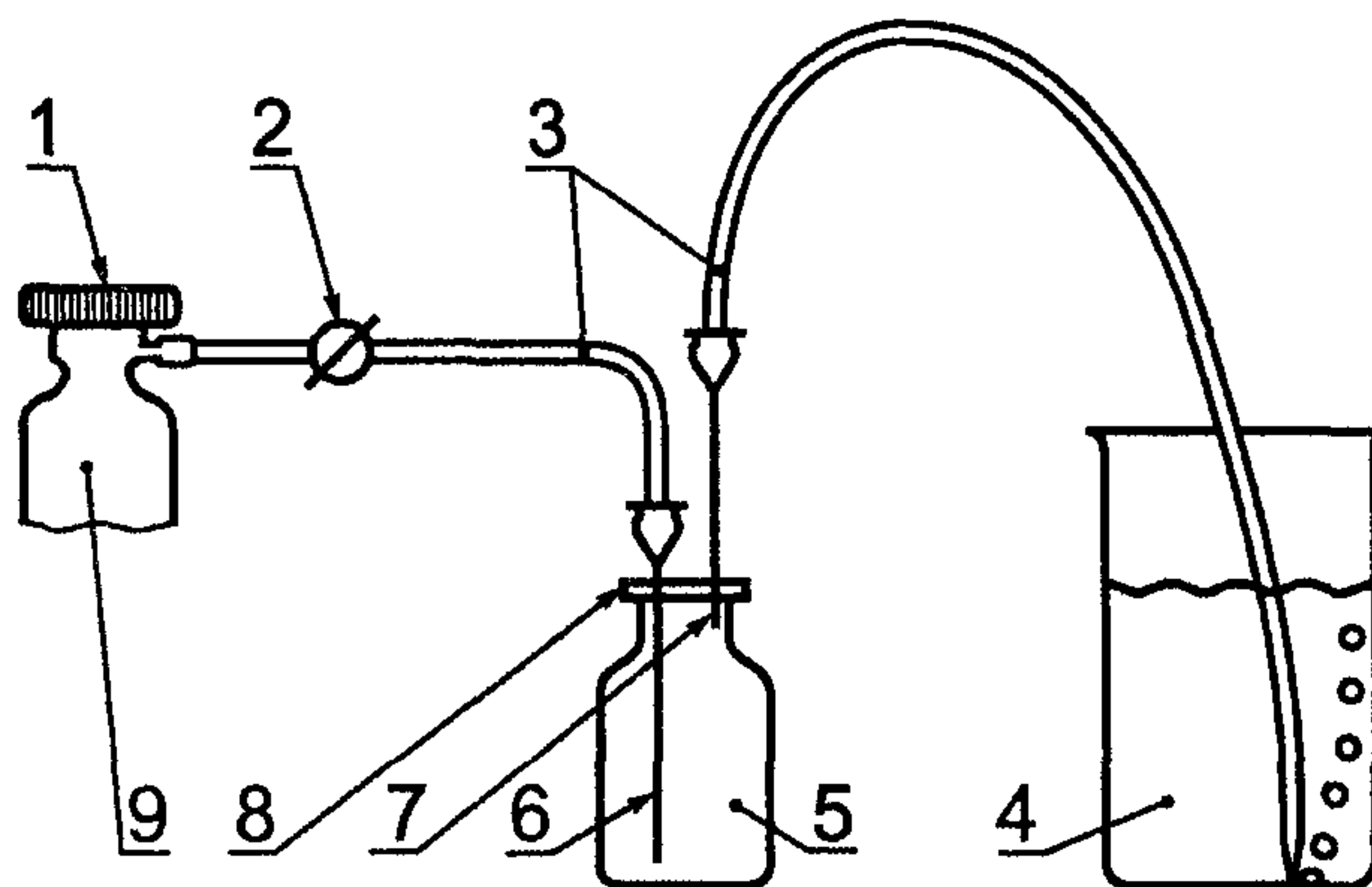
1 — клапан; 2 — регулятор; 3 — трубки ПВХ; 4 — стакан с водой; 5 — флакон; 6 — входная игла 1; 7 — выходная игла 2; 8 — закручивающаяся крышка с ПТЭФ прокладкой; 9 — баллон с газообразным ЭО
