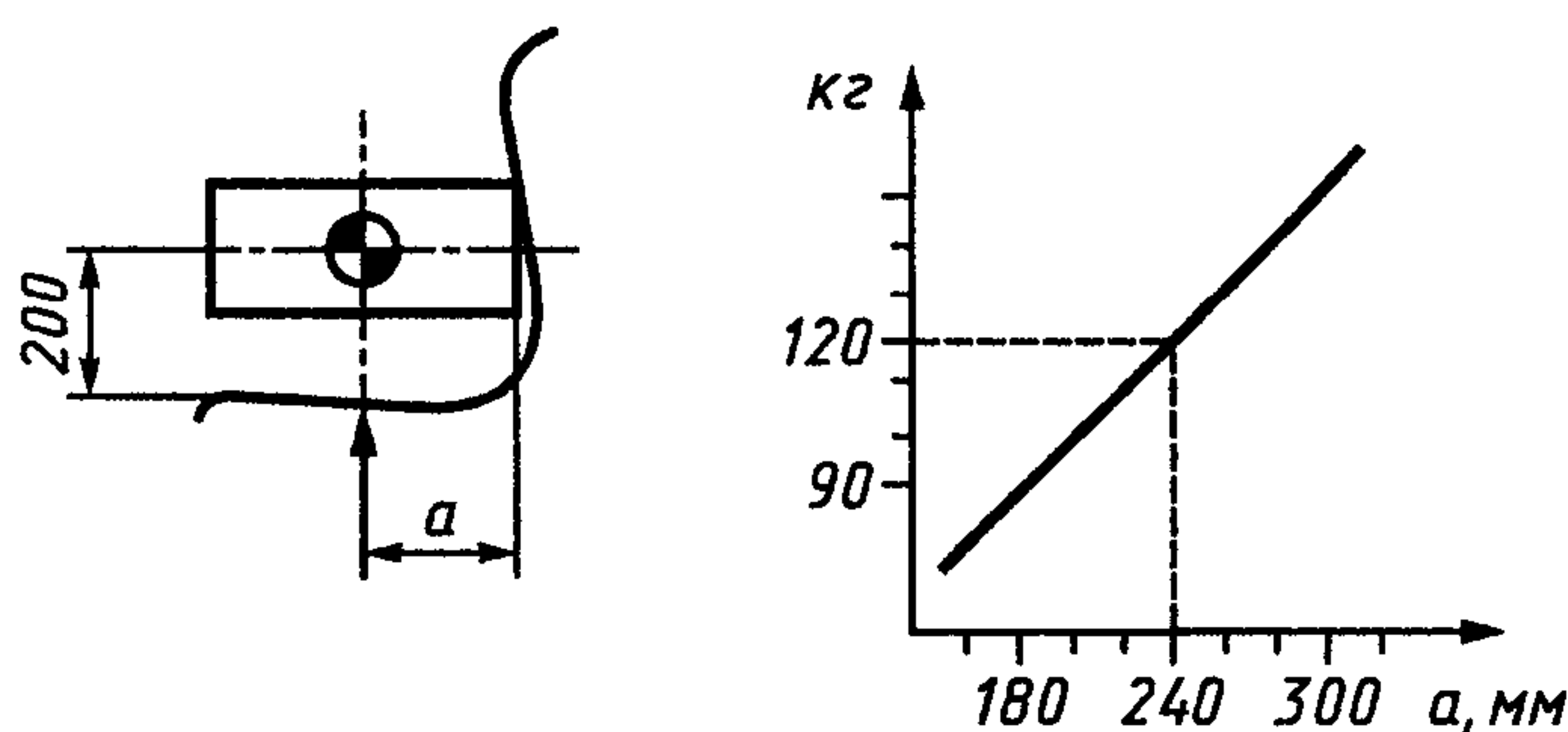
Рисунок 8 — Расположение нагрузки на жестком сиденье
