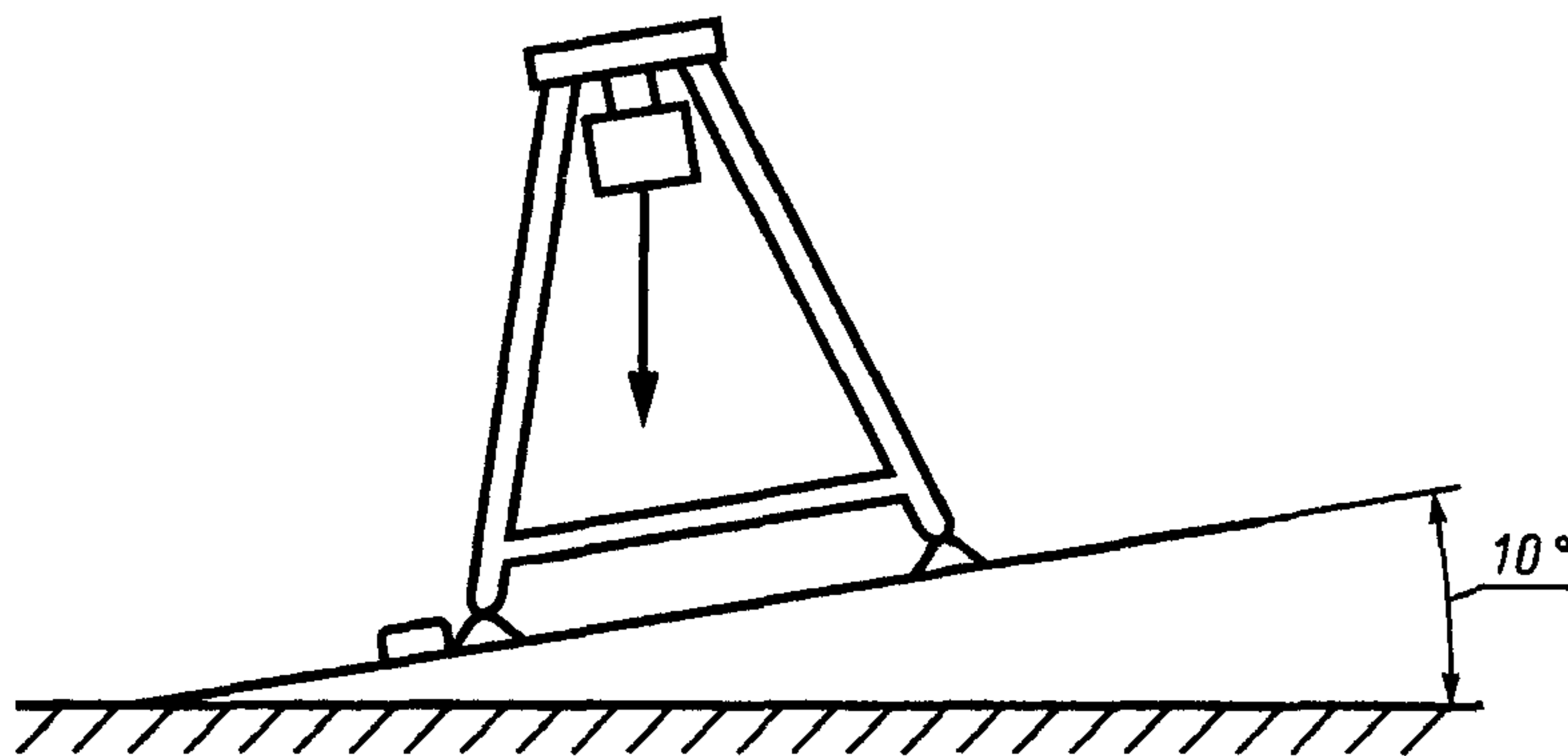
Рисунок 11 — Испытание на статическую прочность свободностоящего подъемника
