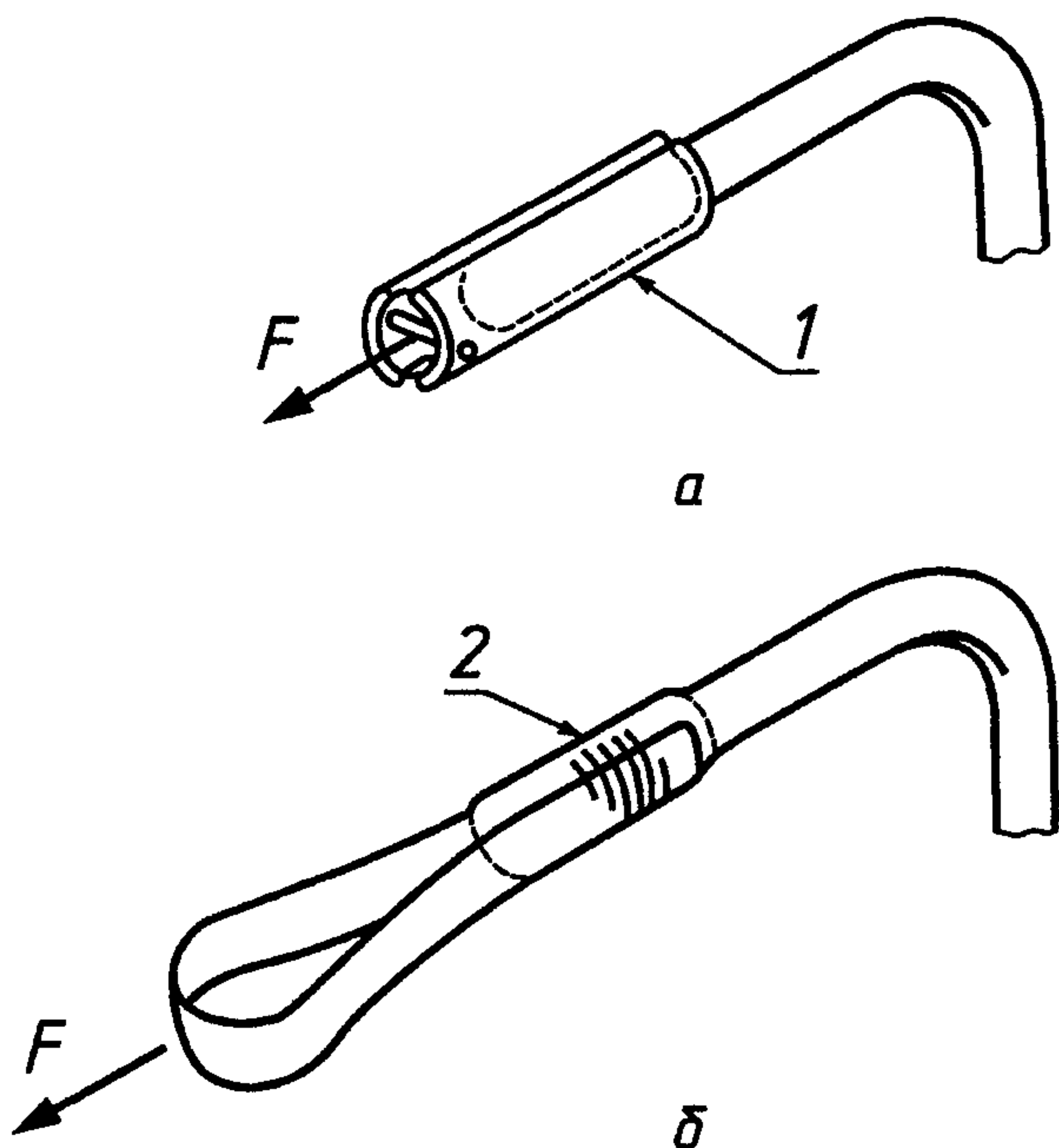
а, б — варианты исполнения устройств к рукояткам для приложения испытательной нагрузки F
