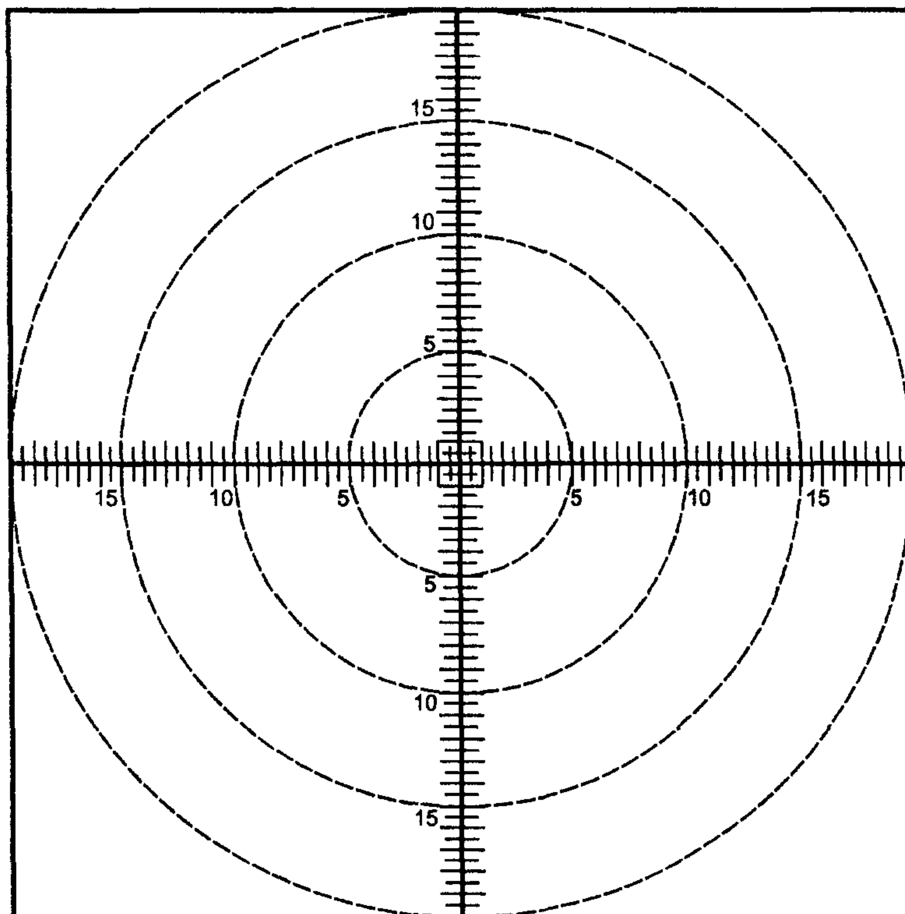
Рисунок 1 — ТЕСТ-ОБЪЕКТ для определения ДИСТОРСИИ ИЗОБРАЖЕНИЯ
