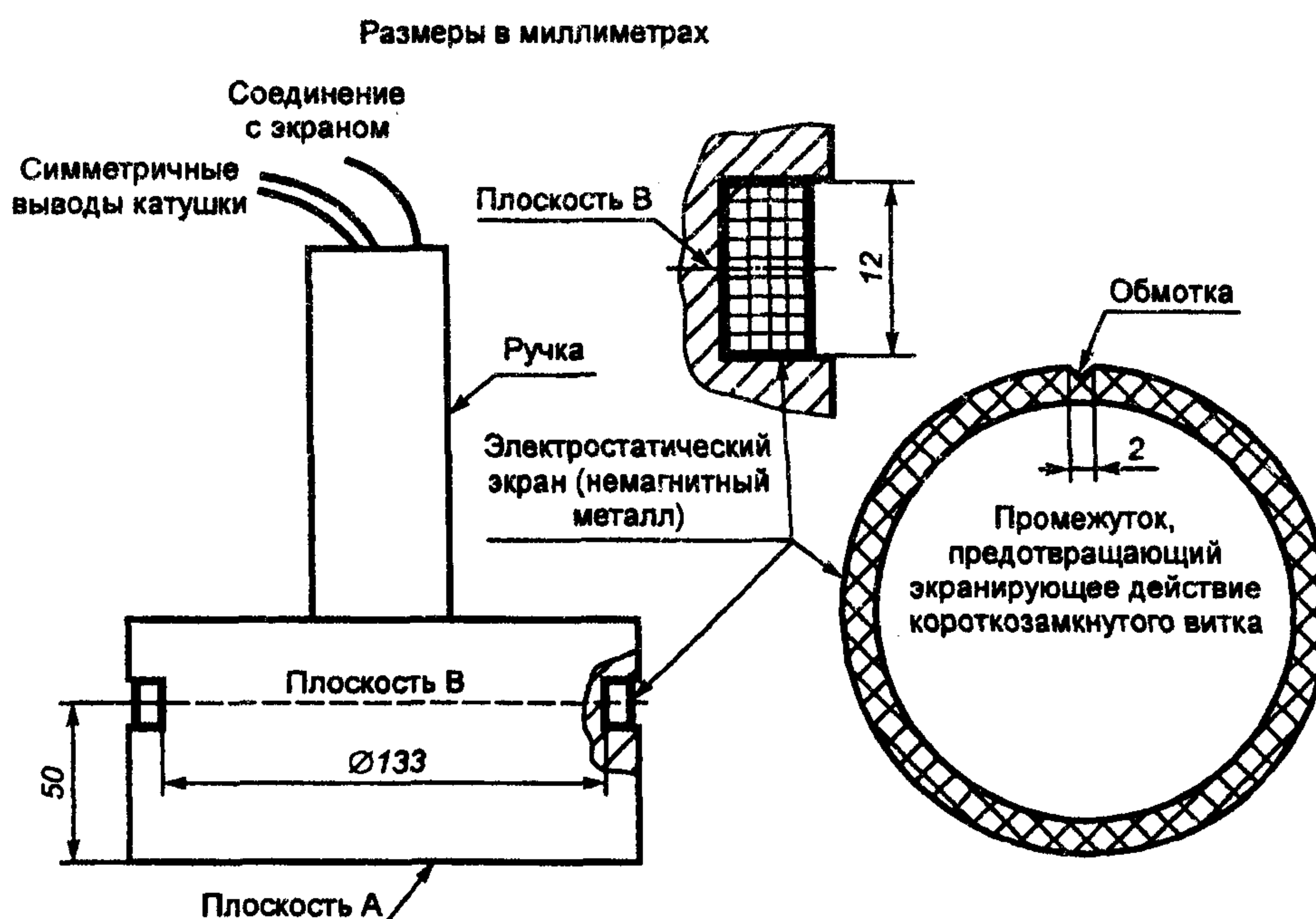
Рисунок А.1 — Конструкция рамочного датчика
