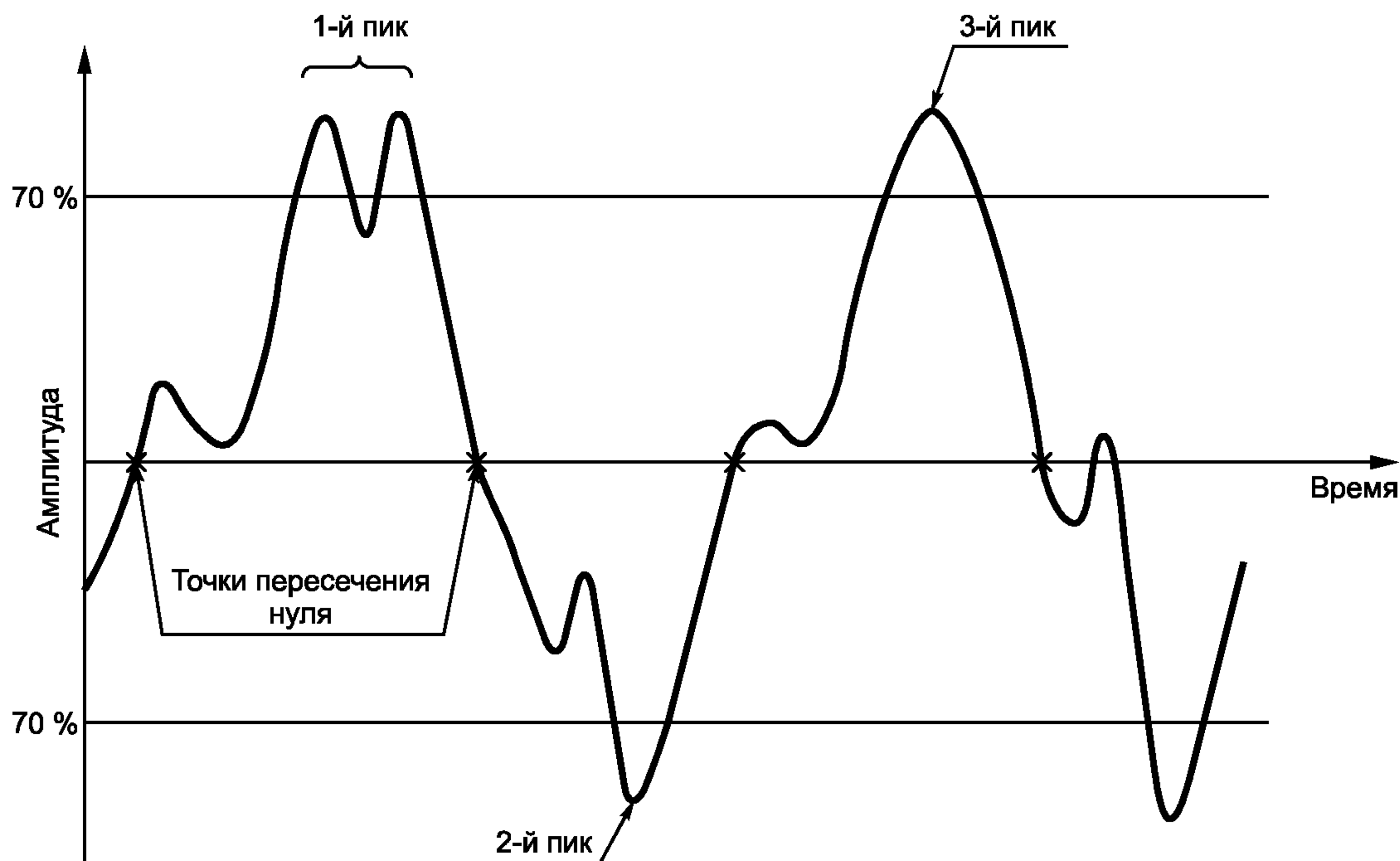
Рисунок 2 — Пример обнаружения пиков отклика, превышающих пороговое значение (70 %)
