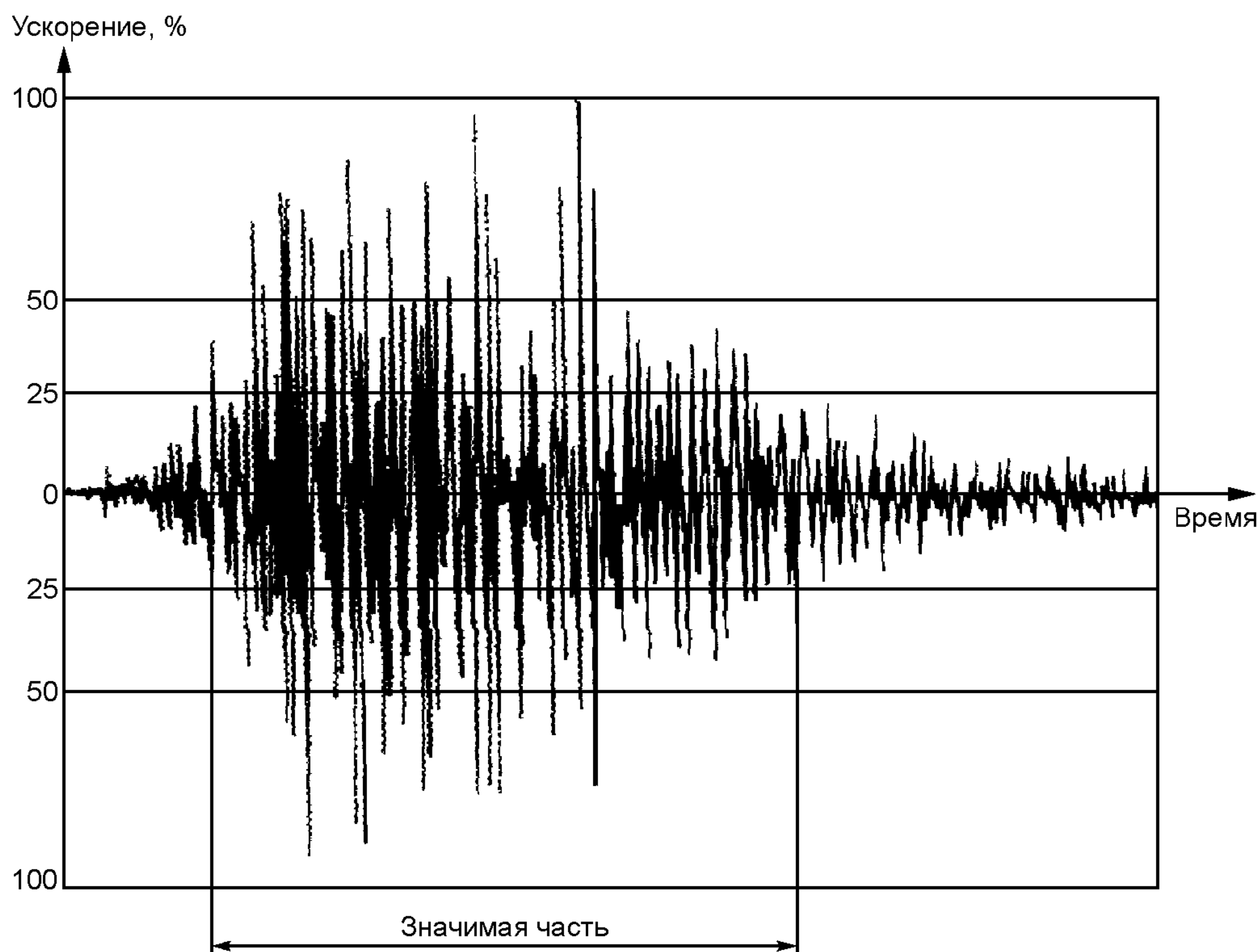
Рисунок 4 — Типичная форма акселерограммы
