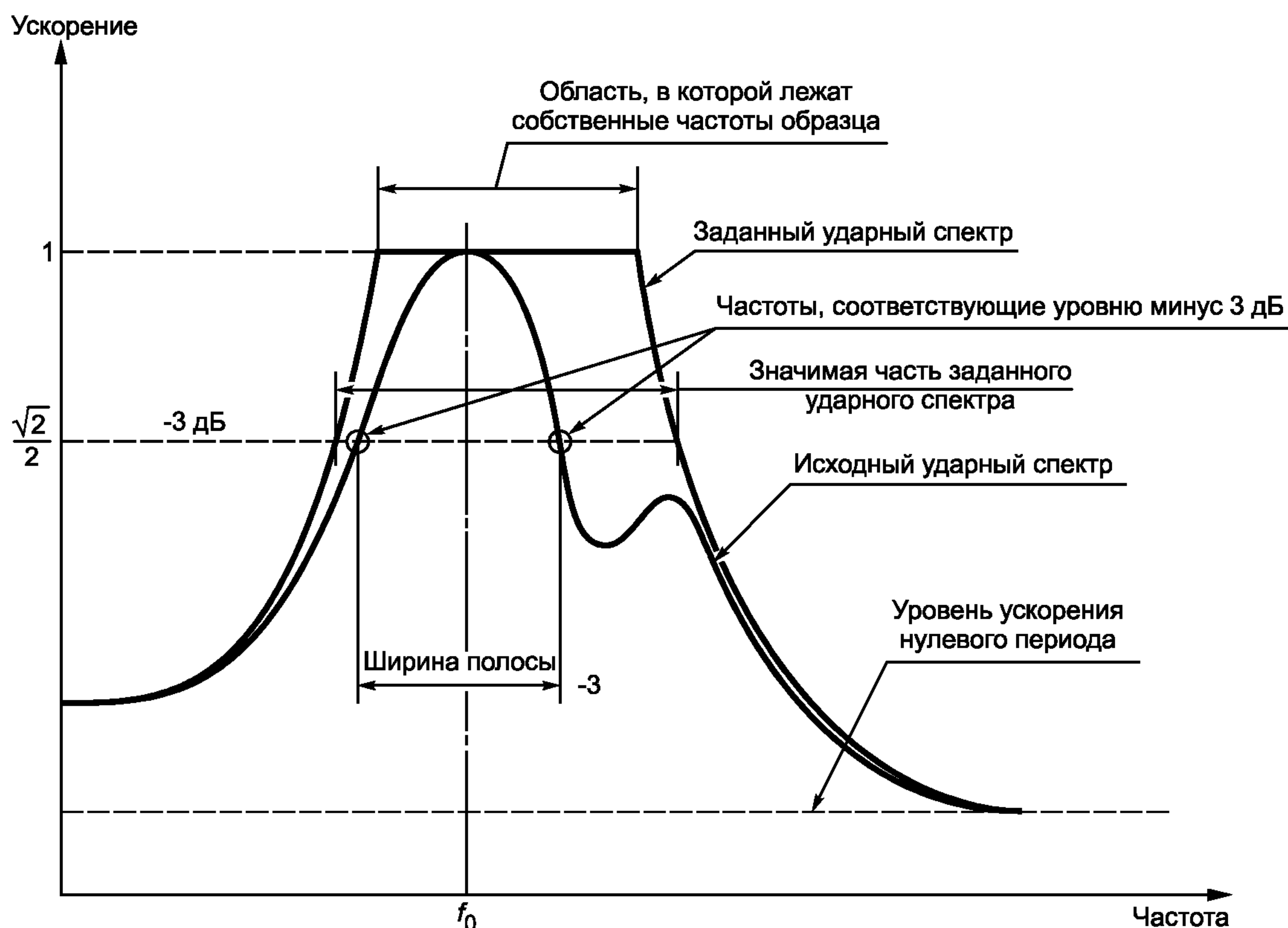
Рисунок 3 — Типичная огибающая спектра ответа
