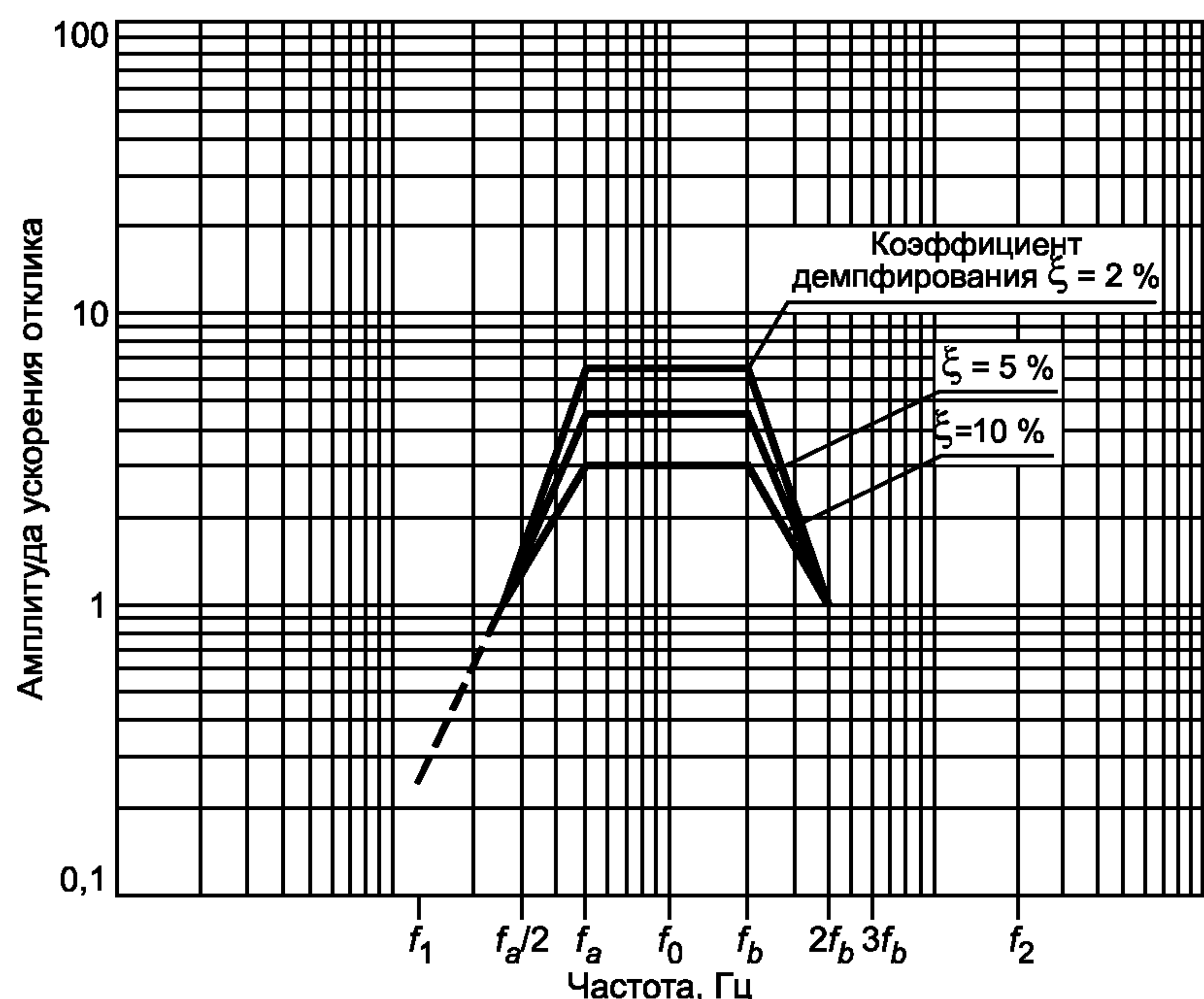
Рисунок — Категория 2. Рекомендуемый вид заданного спектра ответа
