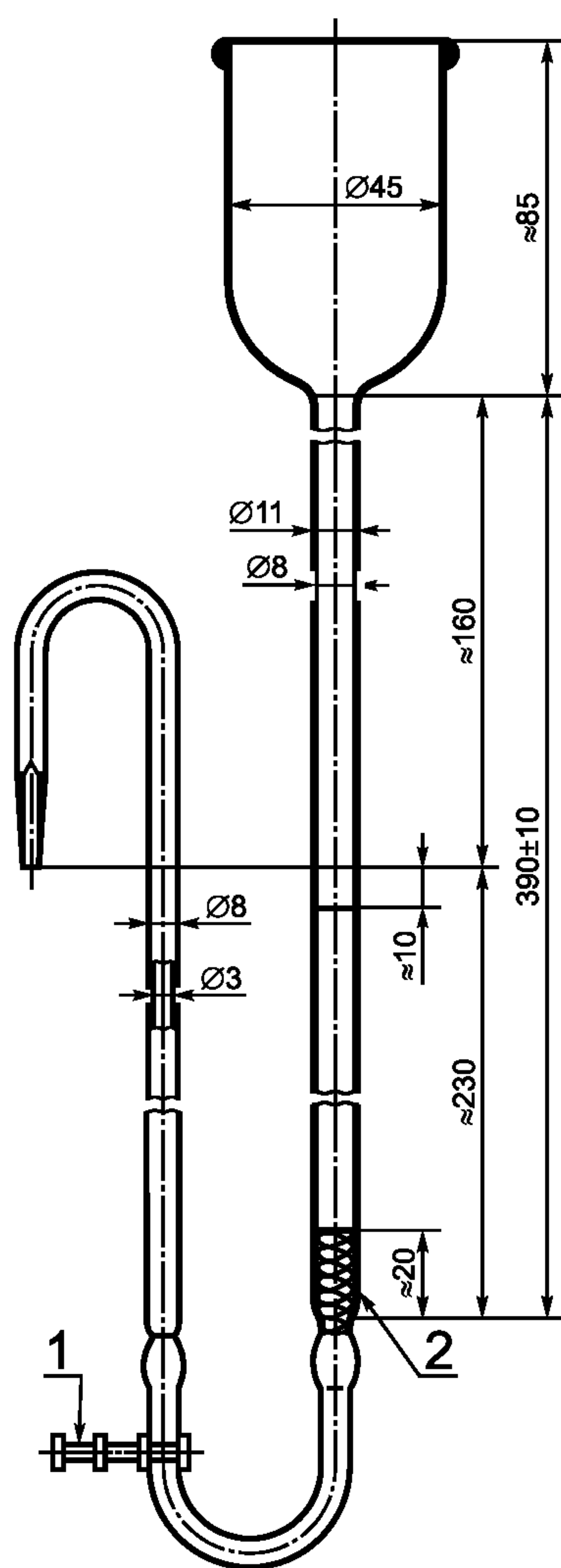
1 — зажим с винтом; 2 — прокладка из стекловаты
