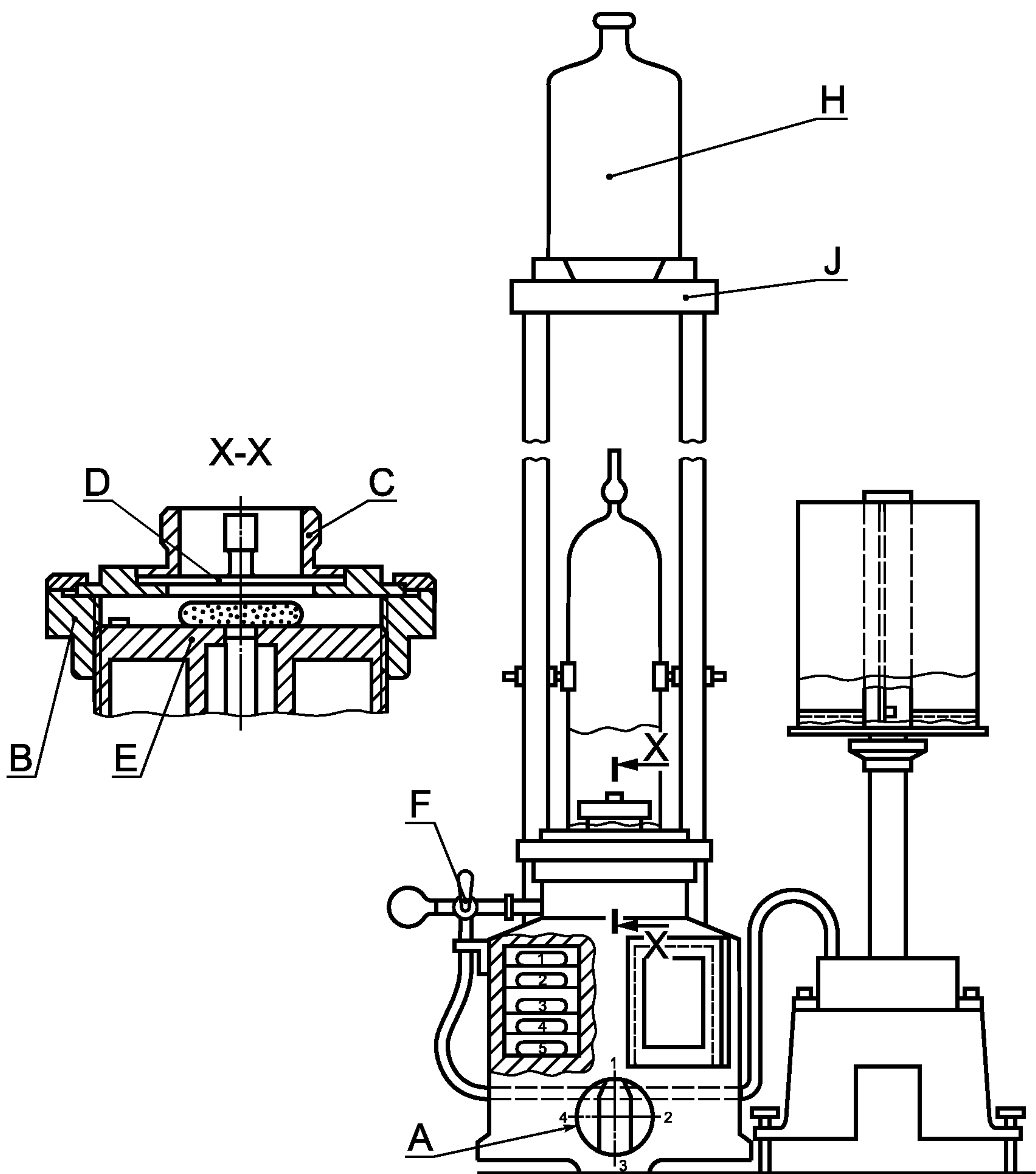
Рисунок 1 — Альвеограф (старая модель)
