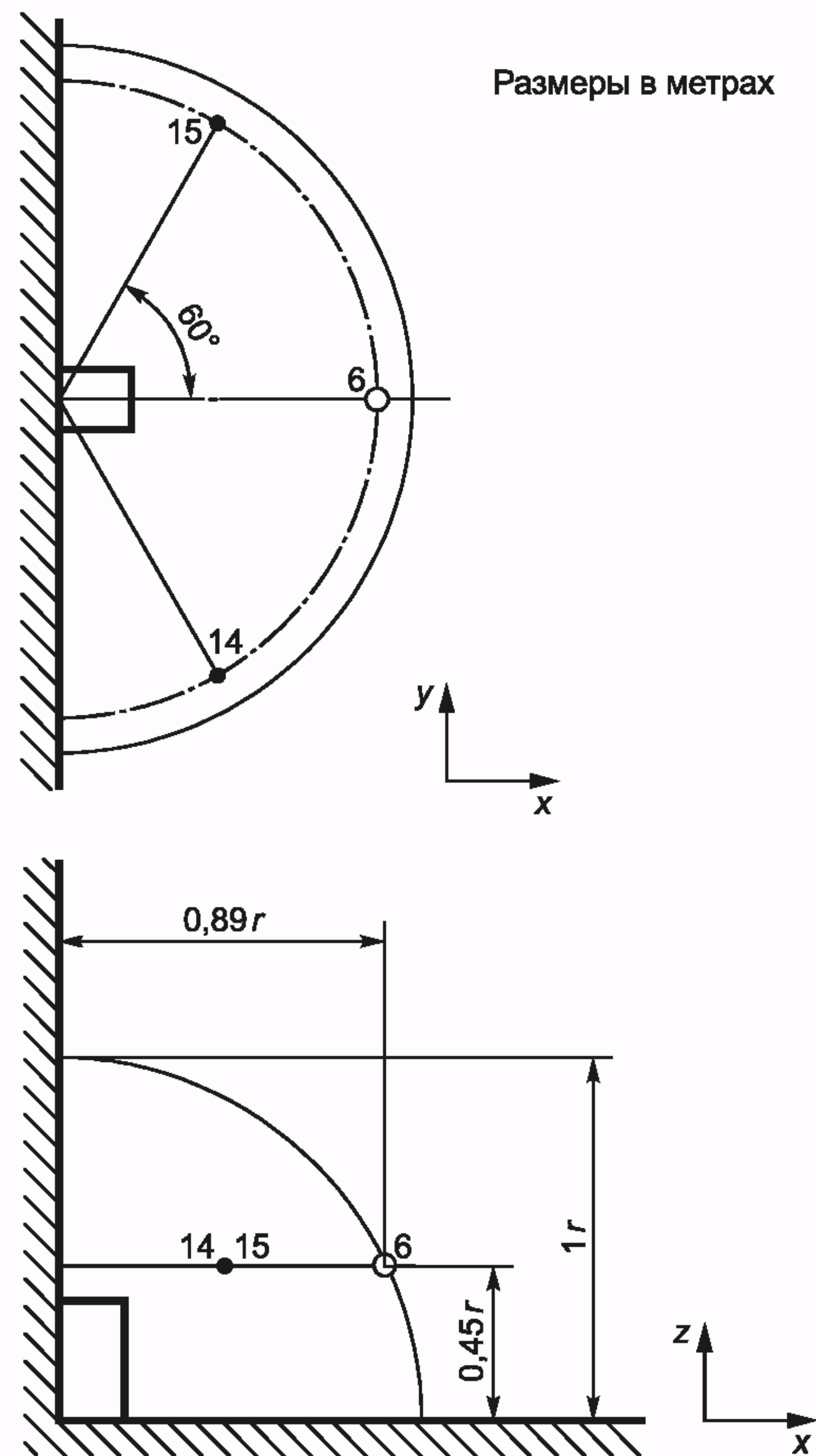
4, 5, 6, 10 — основные точки измерения Рисунок Б.1 — Основные точки измерения на полусферической измерительной поверхности
