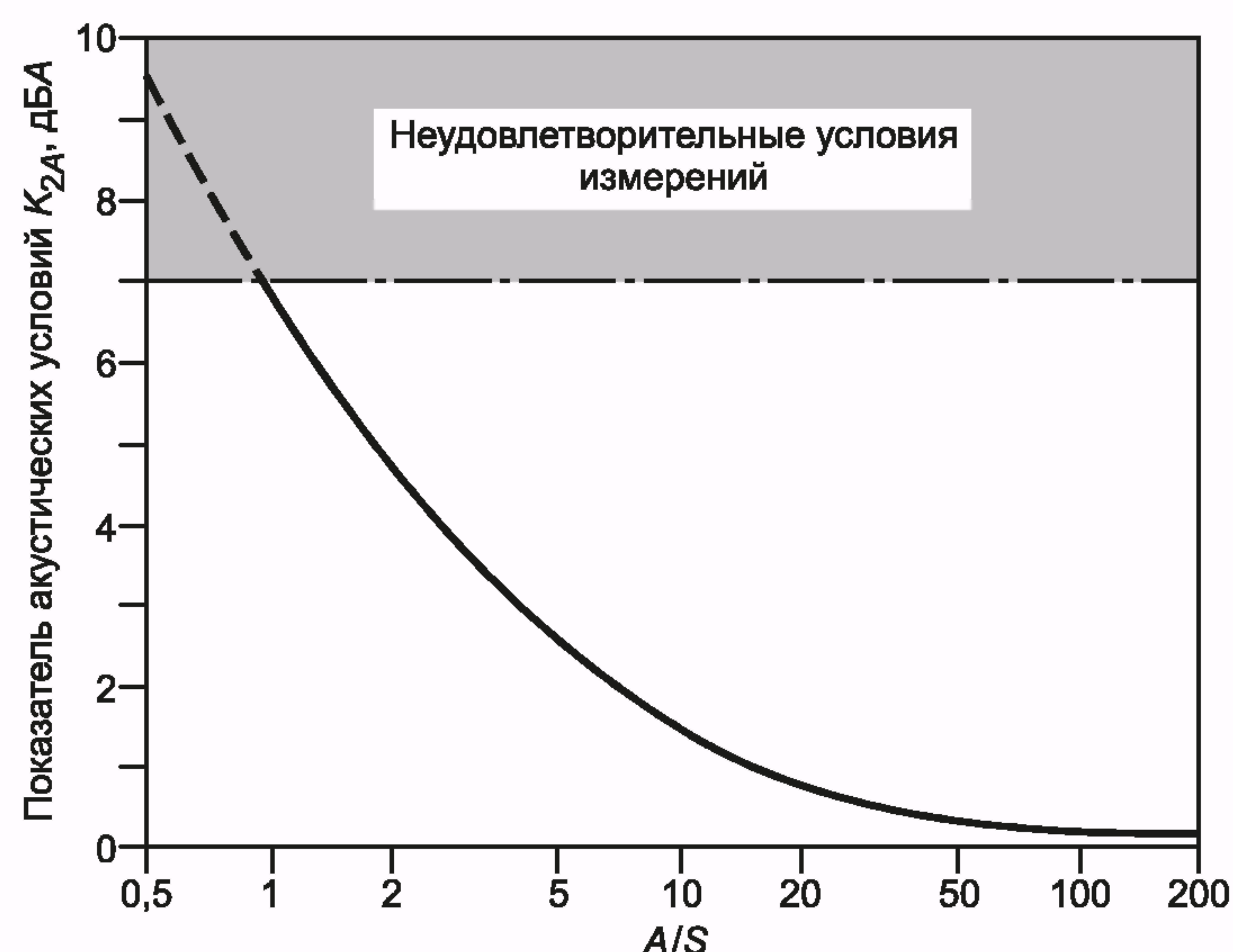
Рисунок А.1 — Показатель акустических условий K_{2A}
