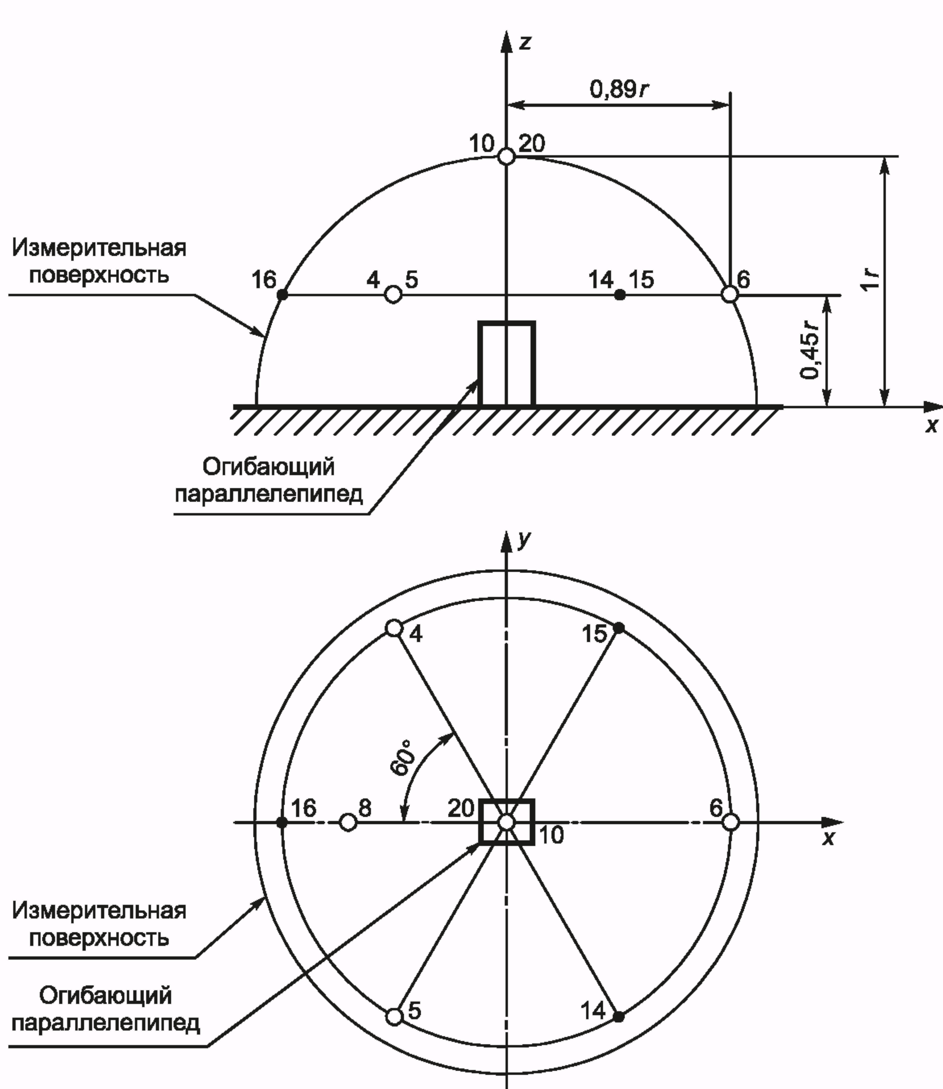
4, 5, 6, 10 — основные точки измерения Рисунок Б.1 — Основные точки измерения на полусферической измерительной поверхности
