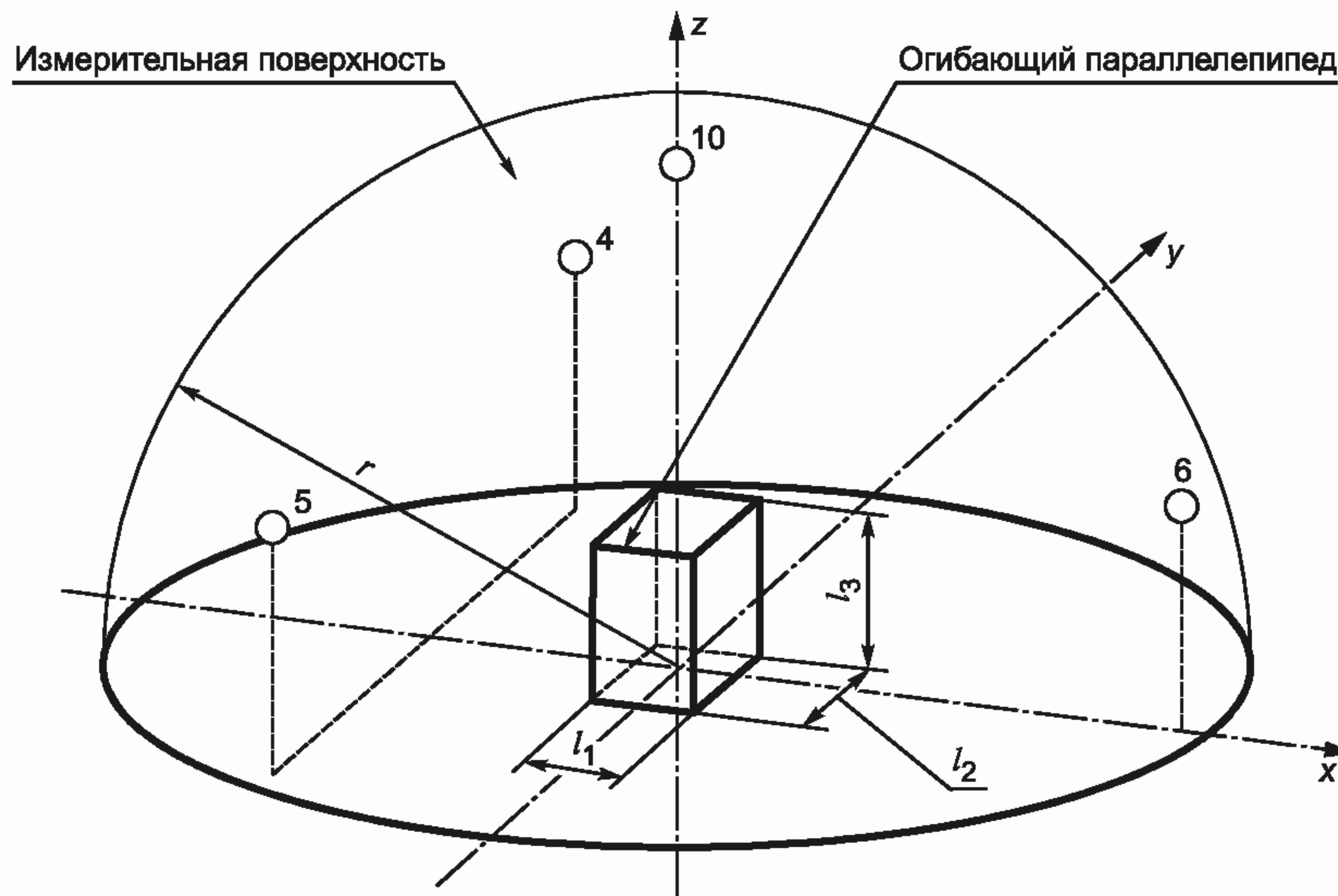
4, 5, 6, 10 — основные точки измерения Рисунок Б.1 — Основные точки измерения на полусферической измерительной поверхности
